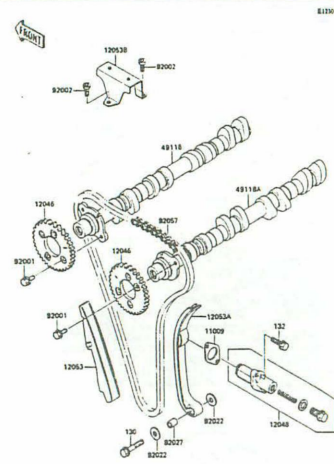
Camshaft/Tensioner
