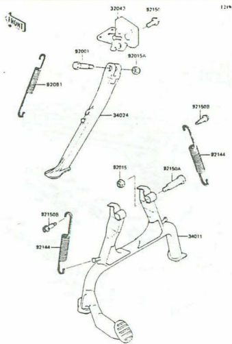
E-10 Stand
