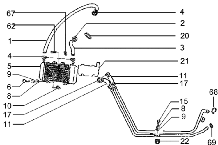
Kühlsystem
