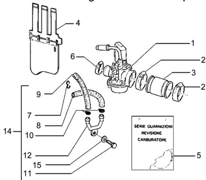
Vergaser / Drosselkörper
