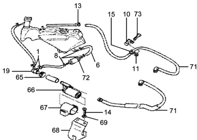
Kraftstoffanlage PureJet
