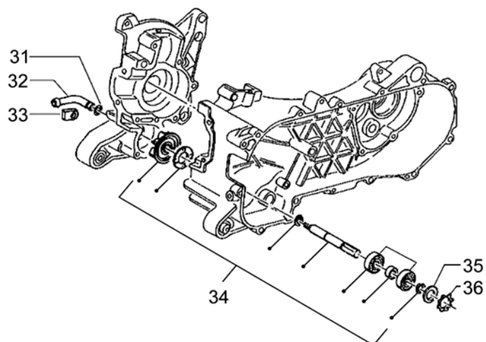
Wasserpumpe
