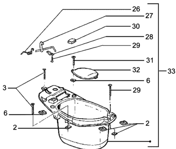
Helmfach
