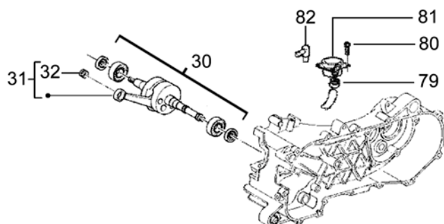
Kurbelwelle
