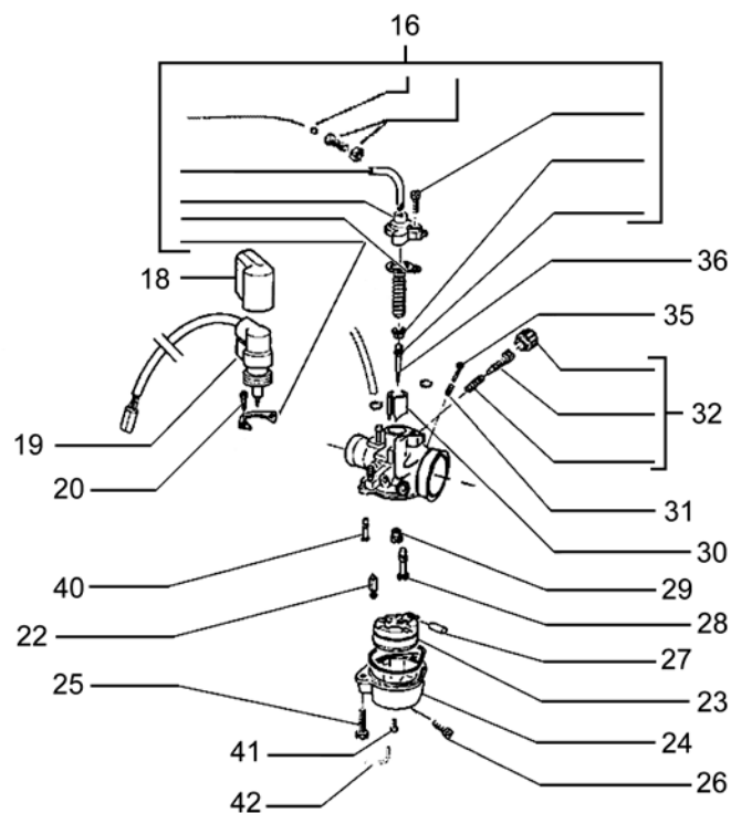
Vergaser
