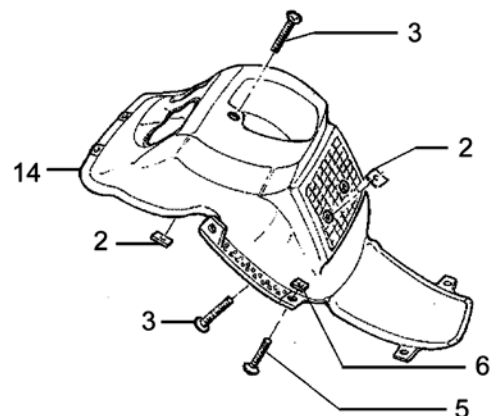
Verkleidung unten
