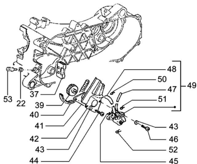
Ölpumpe
