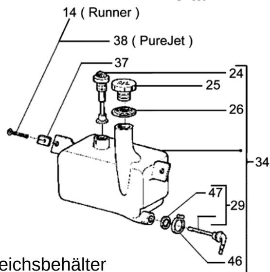
Öltank
