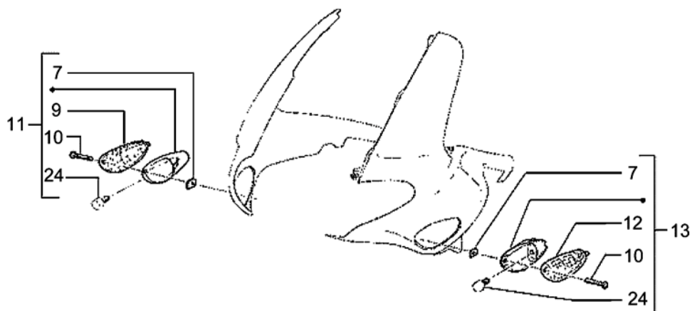
Blinker vorne
