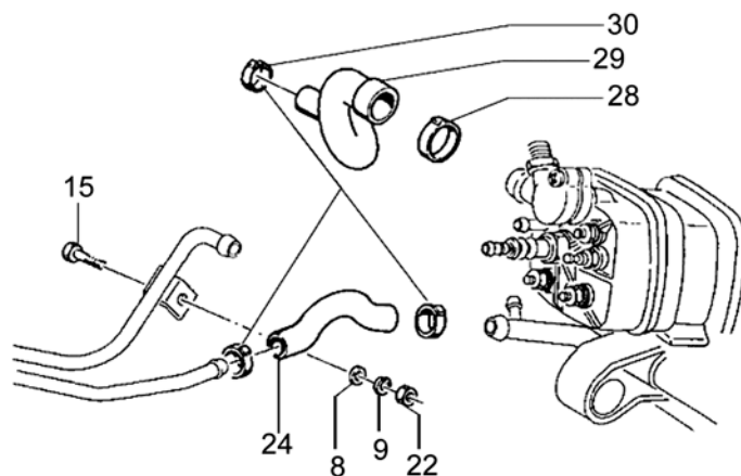
Kühlsystem
