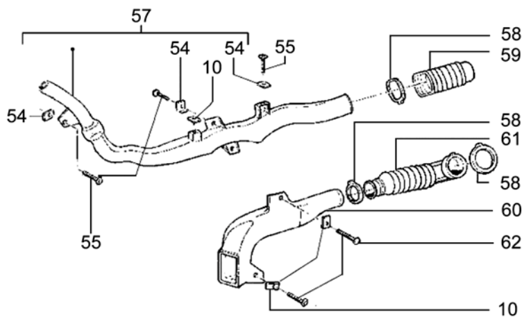
Kühlleitung / Ansaugrohr
