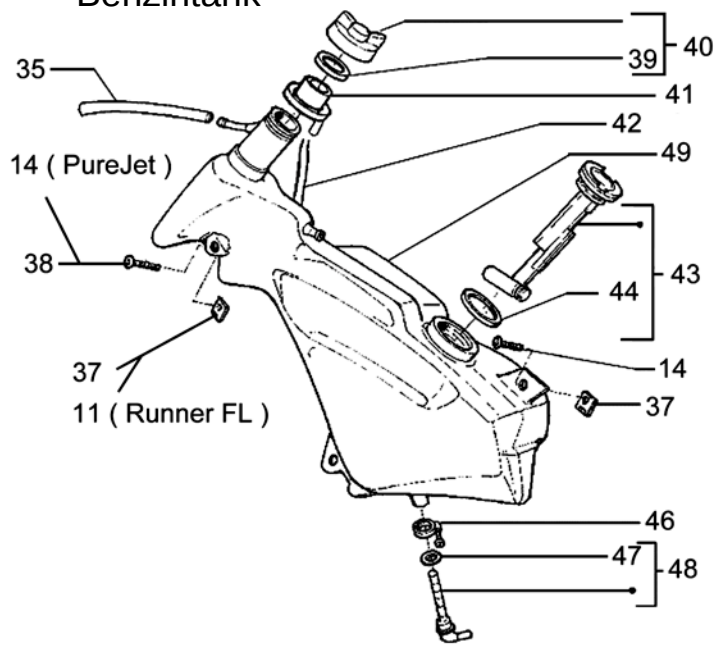
Benzintank
