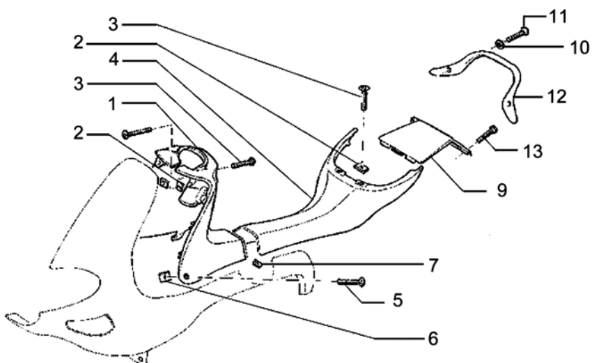
Verkleidung Fußraum
