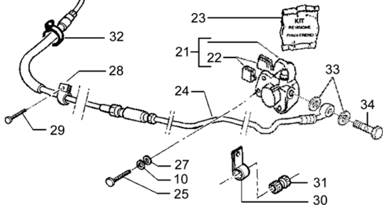
Bremszange
