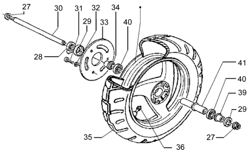
Vorderrad
