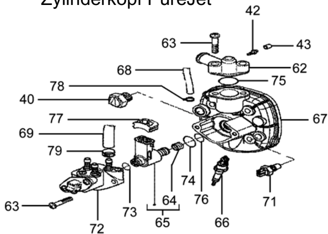
Zylinderkopf PureJet
