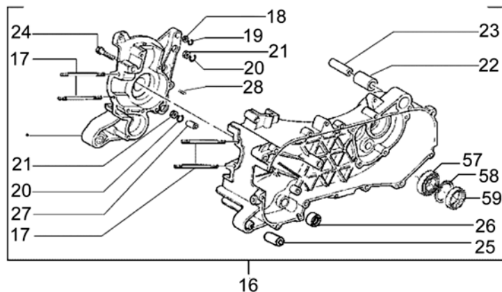
Kurbelwellengehäuse
