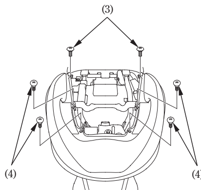
(3) Tornillos A (4) Tornillos B
