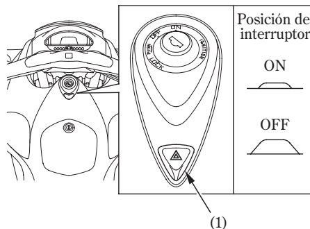
(1) Interruptor de aviso de peligro
