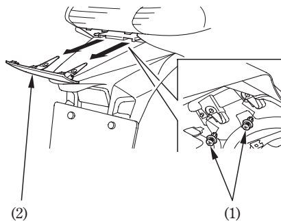
(1) Sujetadores A (2) Carenado central trasero
