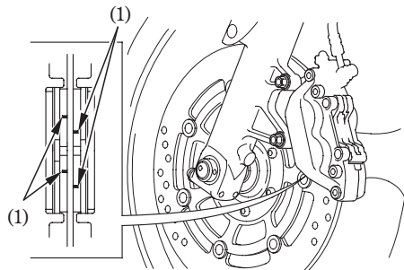
(1) Ranuras
