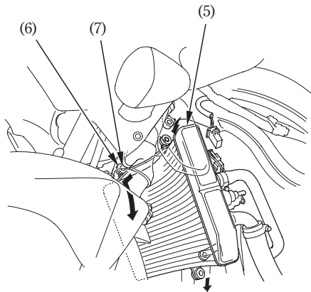
(5) Radiador (6) Arandela
