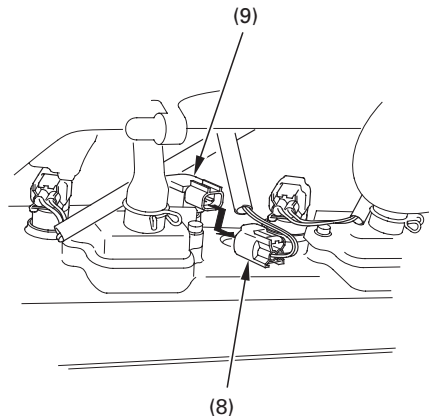
(8) Connettori bobine di accensione (9) Bobine di accensione
