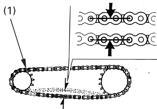
(1) Catena di trasmissione
