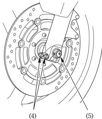
(4) Pernos de retención del eje (5) Semieje delantero
