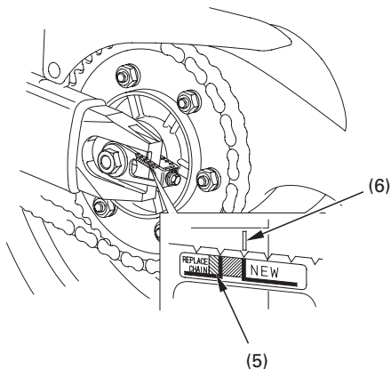
(5) Zona rossa
