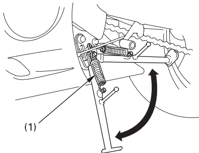
(1) Molla del cavalletto
