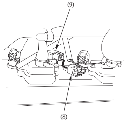
(8) Conectores de las bobinas de encendido (9) Bobinas de encendido
