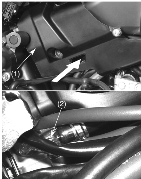
(1) Cubierta
