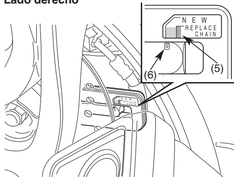
(5) Zona roja
