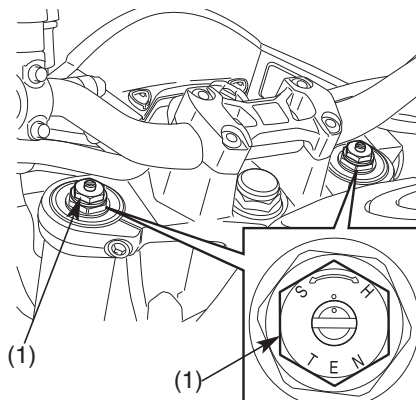
(1) Regulación precarga
