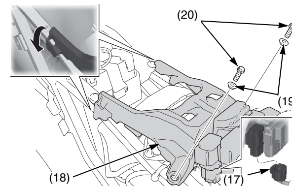
(17) conector del relé de encendido/motor de arranque (18) base de soporte del asiento (19) casquillos (20) tornillos de montaje de la base de soporte del asiento
