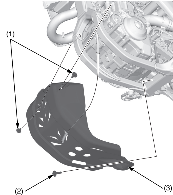
(1) arandelas/tornillos A del protector del motor (2) arandela/tornillos B del protector del motor (3) protector del motor
