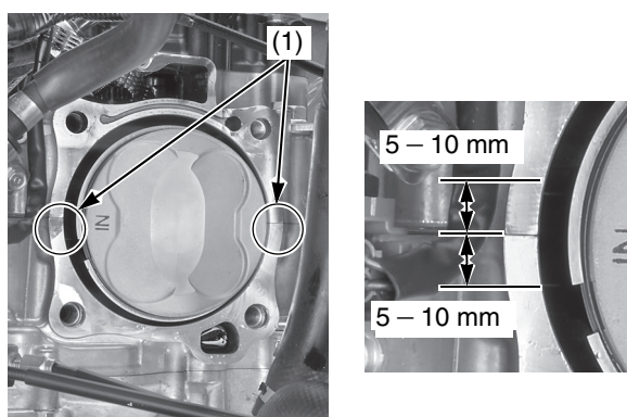
(1) superficie de acoplamiento del cilindro
