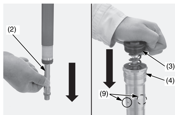
(2) barra del pistón del amortiguador de la horquilla (3) conjunto de tornillos de la horquilla (4) conjunto del amortiguador de la horquilla (9) orificios de lubricación de la horquilla
