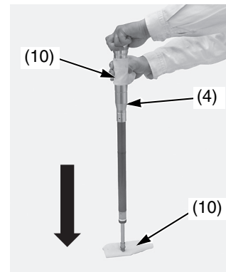
(4) conjunto del amortiguador de la horquilla (10) trapo de taller de la horquilla
