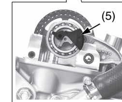
(5) peso del descompresor (8) corona del árbol de levas (6) árbol de levas (9) cojinete del árbol de levas izquierdo (7) cadena de distribución (10) culata
