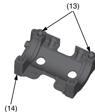
(13) pasadores (14) soporte del árbol de levas
