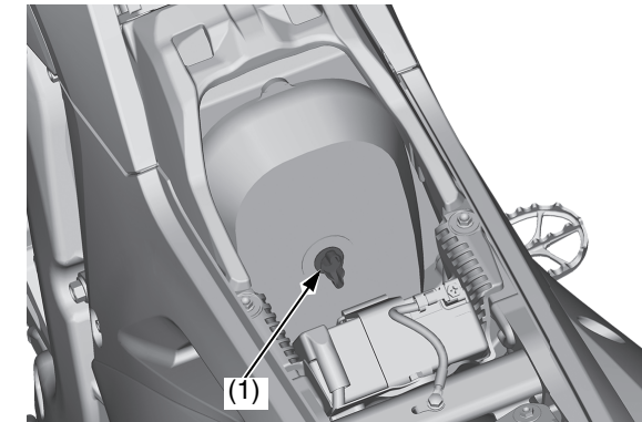
(1) tornillo de fijación del filtro de aire
