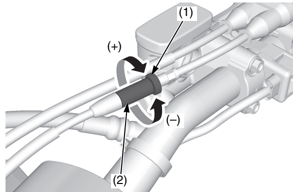
(1) contratuerca (2) mando de ajuste (+) aumento de holgura (-) reducción de holgura
