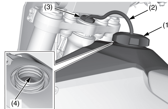
(1) tapón de llenado de combustible (2) respiradero
