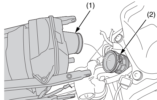
(1) caja del filtro de aire (2) tubo de conexión del filtro de aire
