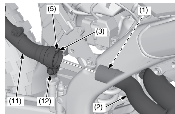
(1) junta (2) tubo de escape (3) recorte (5) lengüeta (11) silenciador derecho (12) abrazadera del silenciador derecho
