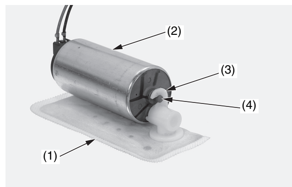
(1) filtro de la bomba de combustible (2) conjunto de la bomba de combustible (3) gancho (4) refuerzo de la junta de combustible
