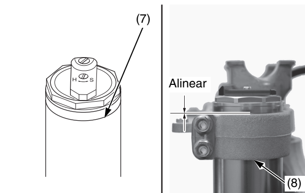
(7) ranura
