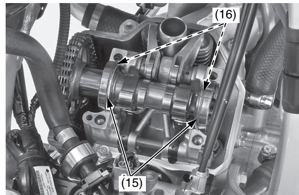
(15) anillos de ajuste (16) ranuras del cojinete del árbol de levas
