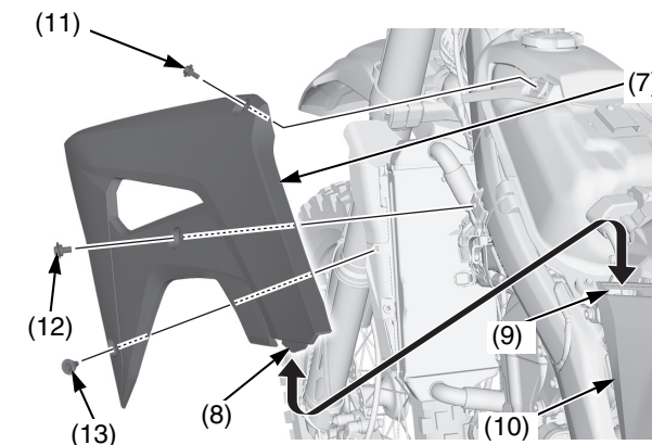
(7) cubierta (8) lengüeta (9) ranura (10) tapa del filtro de aire (11) tornillo C de la cubierta (12) tornillo B de la cubierta (13) tornillo A de la cubierta
