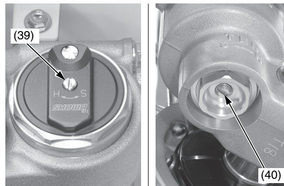
(39) mando de ajuste de amortiguación en compresión (40) mando de ajuste de amortiguación en extensión
