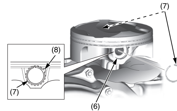
(6) bulón del pistón (8) corte del pistón (7) clips del bulón del pistón (nuevos)
