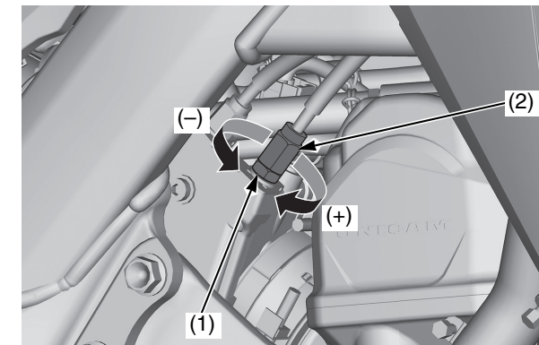
(1) contratuerca (2) mando de ajuste (+) aumento de holgura (-) reducción de holgura
