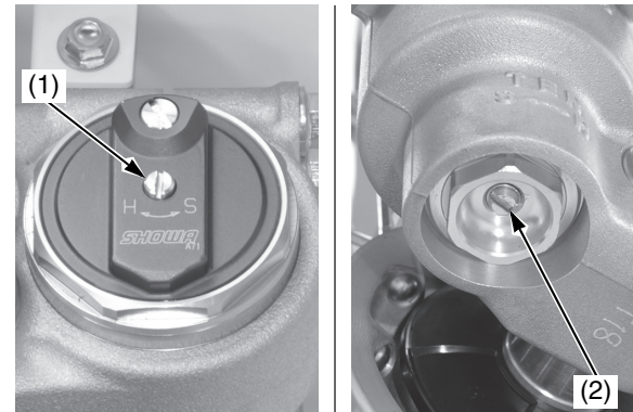
(1) tornillo del mando de ajuste de la amortiguación en compresión
