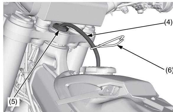
(4) respiradero (5) tuerca del vástago de dirección (6) abrazadera de manguera
