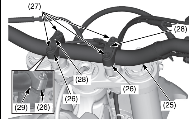
(25) manillar (26) soportes superiores del manillar (27) tornillos del soporte superior del manillar (28) marcas de punzón (29) marca de pintura
