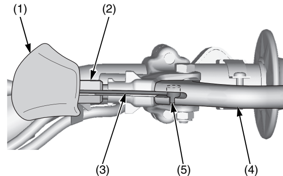
(1) guardapolvo (2) mando de ajuste (3) cable del embrague (4) maneta de embrague (5) extremo del cable del embrague
