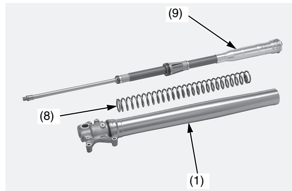
(1) conjunto de la horquilla (9) conjunto del amortiguador de la horquilla (8) resorte de la horquilla
