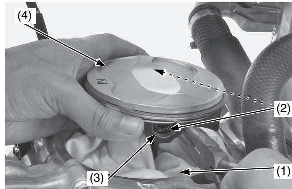
(1) trapos de taller (3) bulón del pistón (2) clips del bulón del pistón (4) pistón
