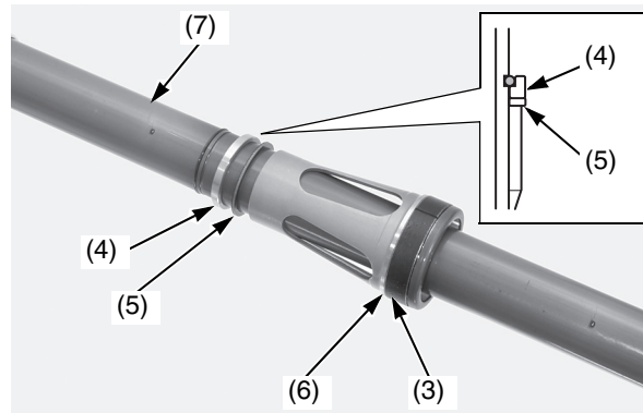
(3) casquillo de la deslizadera (6) casquillo de asiento del muelle (4) tope del asiento (7) amortiguador de la horquilla (5) anillo de apoyo
