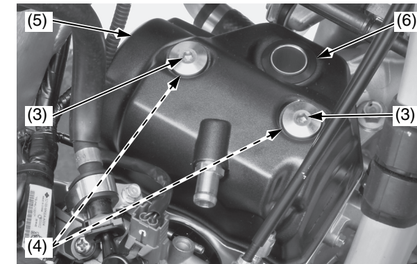
(3) tornillos huecos de la tapa de la culata (4) juntas de goma de la tapa de la culata (5) tapa de la culata (6) empaquetadura del orificio de la bujía
