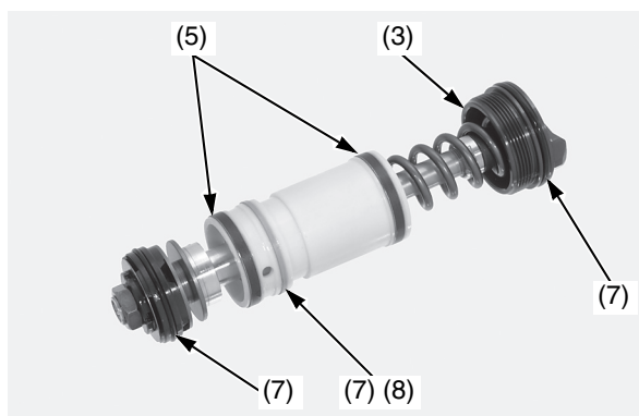
(3) conjunto de tornillos de la horquilla (5) casquillos de los tornillos de la horquilla (7) juntas tóricas (nuevas) (8) anillo de pistón (nuevo)
