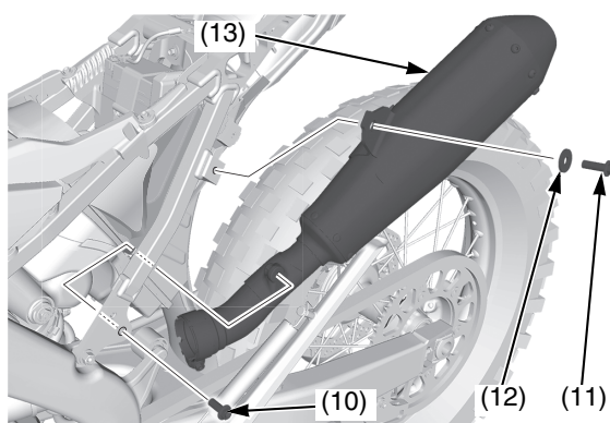
(10) tornillo A de montaje del silenciador izquierdo (11) tornillo B de montaje del silenciador izquierdo (12) arandela (13) silenciador izquierdo
