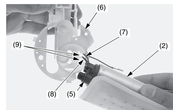
(2) conjunto de la bomba de combustible (5) junta tórica (nueva) (6) soporte de la unidad de la bomba de combustible (7) cable rojo (8) cable negro (9) ranuras
