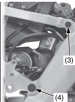
(3) tornillos superiores del subchasis (4) tornillos inferiores del subchasis
