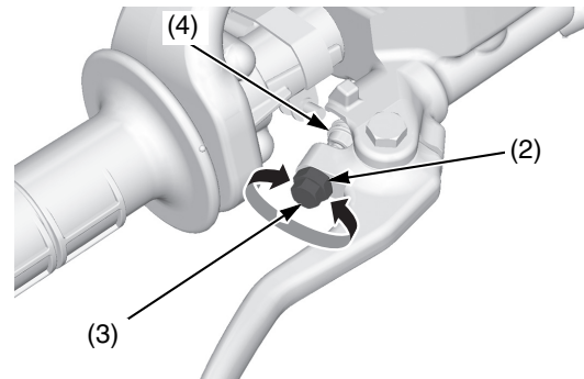
(2) contratuerca (4) brazo de impacto (3) mando de ajuste
