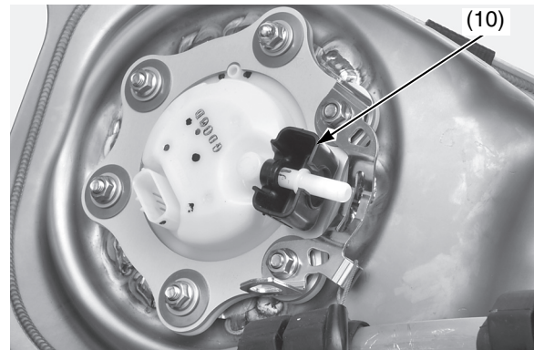
(10) tapa de goma
