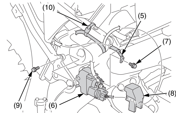
(5) borne del cable de la batería (6) interruptor magnético de arranque (7) tornillo de los terminales del cable de la batería (8) tapa del interruptor magnético de arranque (9) tornillo de sujeción del interruptor magnético de arranque (10) brida de plástico
