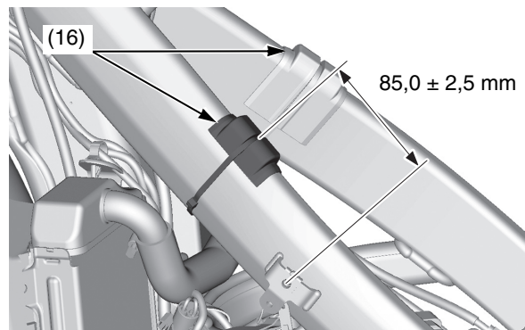
(16) gomas de amortiguación
