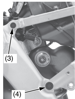
(3) tornillos superiores del subchasis (4) tornillos inferiores del subchasis
