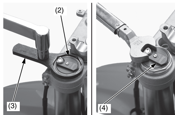
(2) conjunto del amortiguador de la horquilla (3) llave para contratuerca (4) conjunto de tornillos de la horquilla
