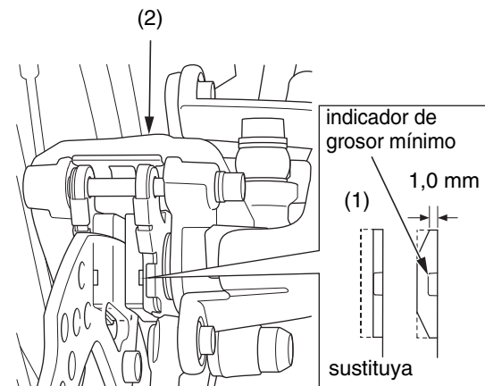
(1) pastillas de freno (2) pinza de freno trasero
