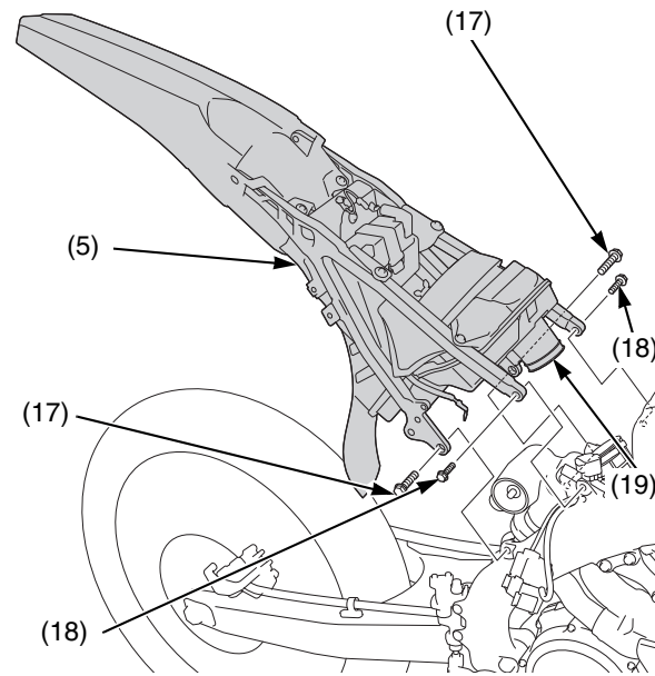
(5) subchasis (17) tornillos inferiores del subchasis (18) tornillos superiores del subchasis (19) tubo de conexión del filtro de aire
