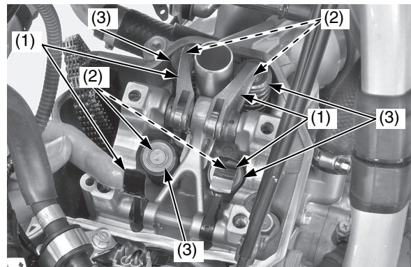
(1) balancines (3) retenedores de resorte de válvula (2) suplementos
