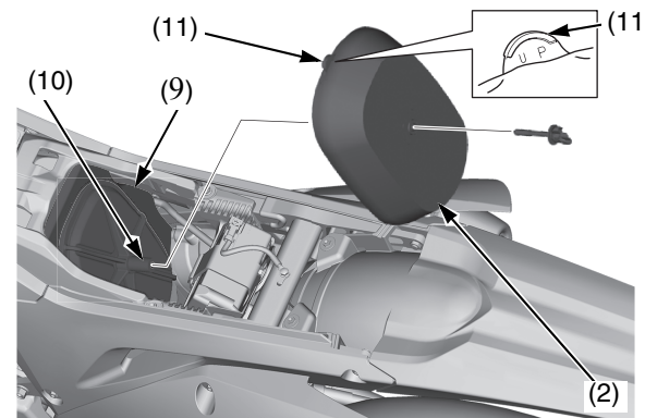
(2) conjunto del filtro de aire (9) área de contacto (10) soporte de la caja del filtro de aire (11) lengüeta con marca "UP" (arriba)
