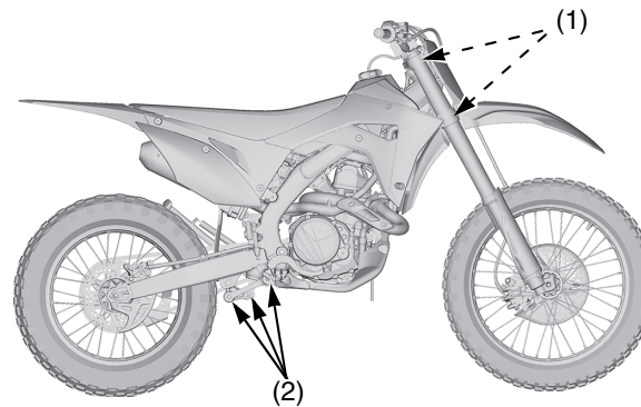
(1) rodamientos de la pipa de dirección (2) puntos de pivote de la suspensión
