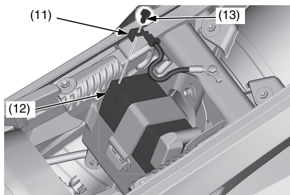
(11) borne negativo (–) (12) batería (13) tornillo del borne negativo (–)
