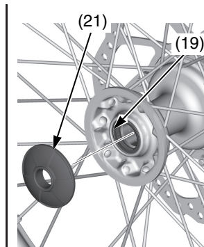
(21) casquillo de lado derecho
