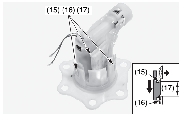
(15) ganchos (16) lengüetas
