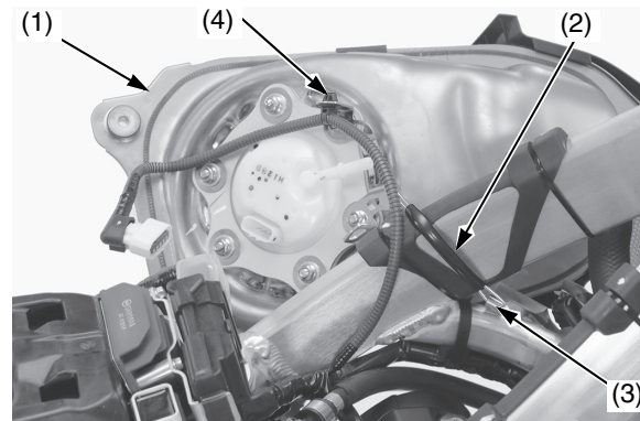
(1) depósito de combustible (3) gancho del bastidor (2) cable de tope (4) clip de la abrazadera del mazo de cables
