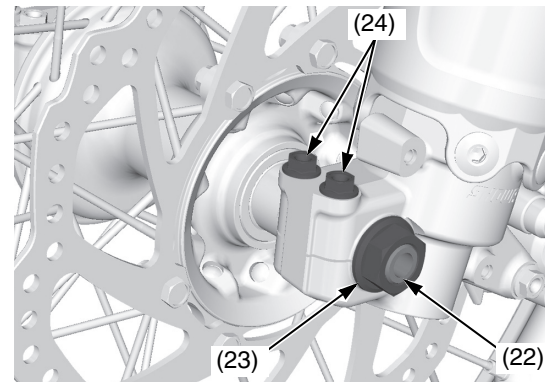
(22) eje delantero (23) tuerca del eje delantero (24) tornillos de bloqueo izquierdos del eje
