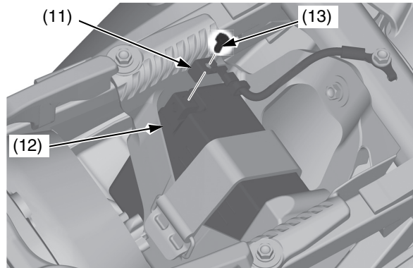
(11) borne negativo (-) (12) batería (13) tornillo del borne negativo (-)
