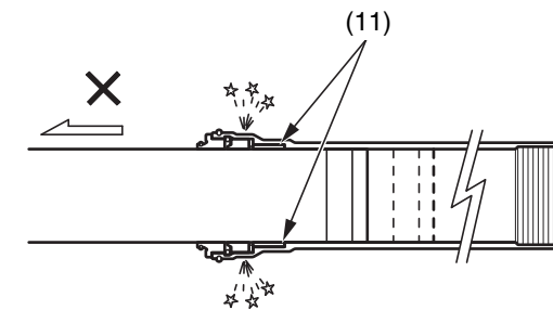
(11) casquillo guía
