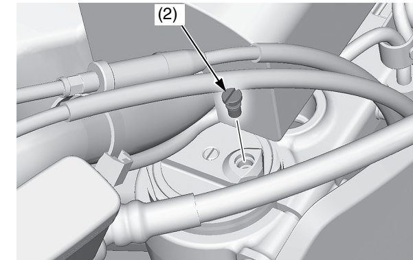
(2) tornillo de liberación de presión
