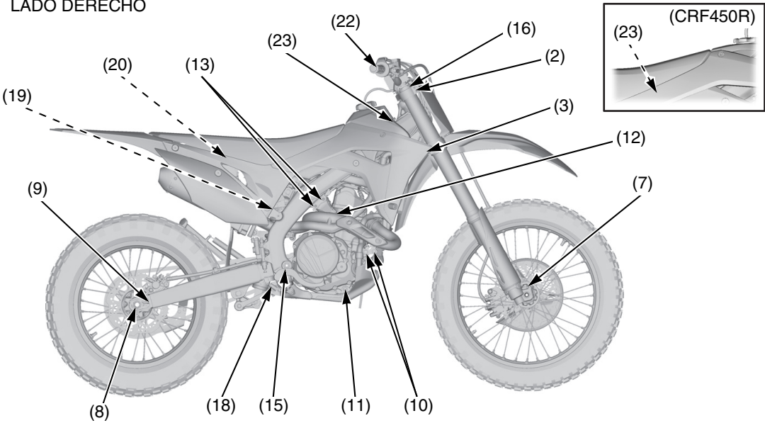
LADO DERECHO
