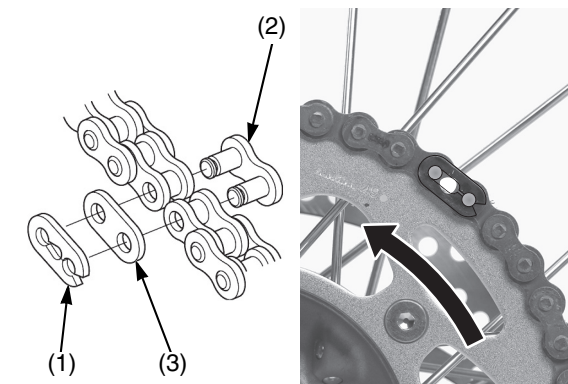
(1) circlip del eslabón de cierre (2) eslabón de cierre (3) placa de eslabón
