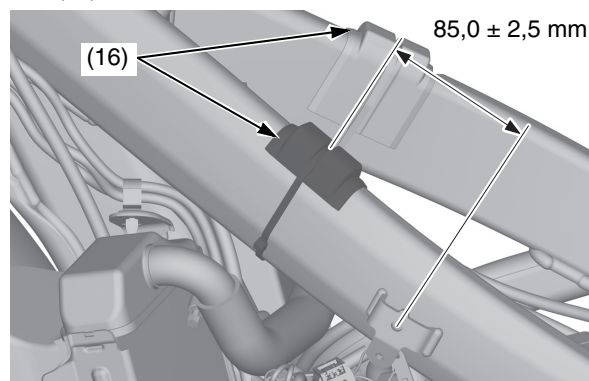
(16) gomas de amortiguación
