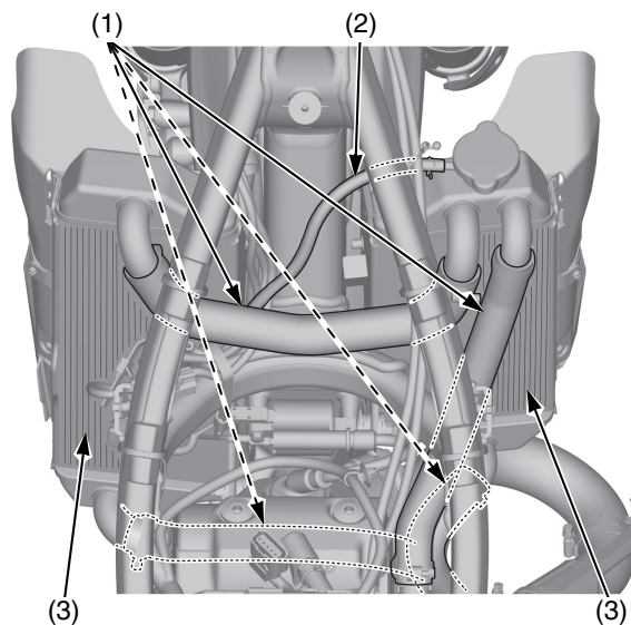
(1) manguitos del radiador (3) aletas del radiador (2) manguito de rebose
