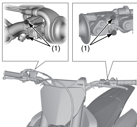
(1) tornillos de montaje de la maneta
