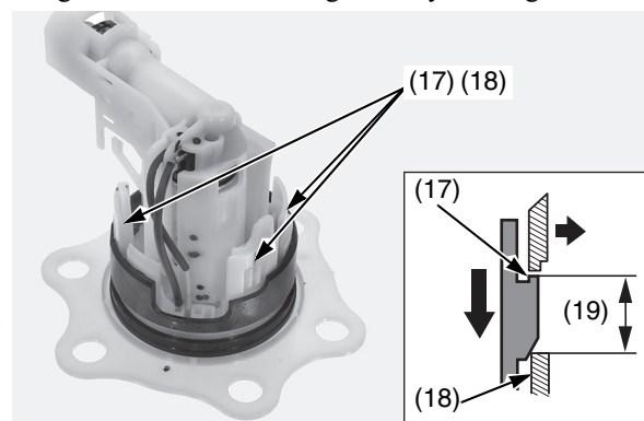
(17) ganchos (18) lengüetas
