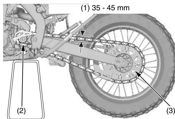
(1) holgura de la cadena de transmisión (3) corona (2) piñón
