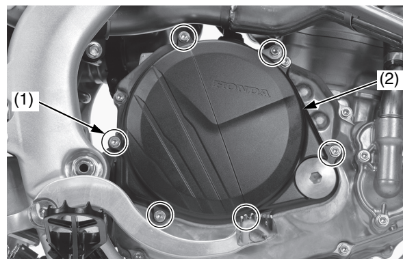
(1) tornillos de la tapa del embrague (2) tapa del embrague
