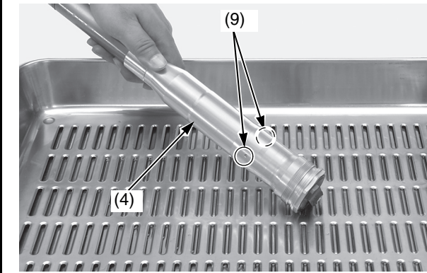
(4) conjunto del amortiguador de la horquilla (9) orificios de lubricación
