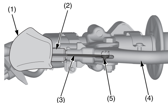
(1) guardapolvo (2) mando de ajuste (3) cable del embrague (4) maneta de embrague (5) extremo del cable del embrague
