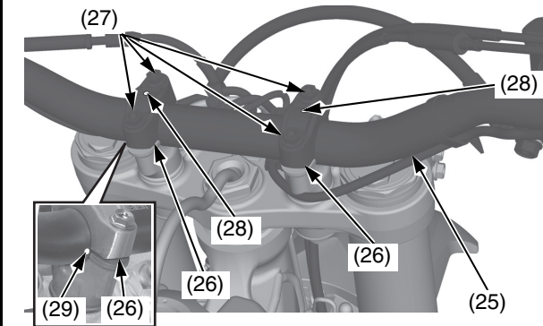
(25) manillar (26) soportes superiores del manillar (27) tornillos del soporte superior del manillar (28) marcas de punzón (29) marca de pintura
