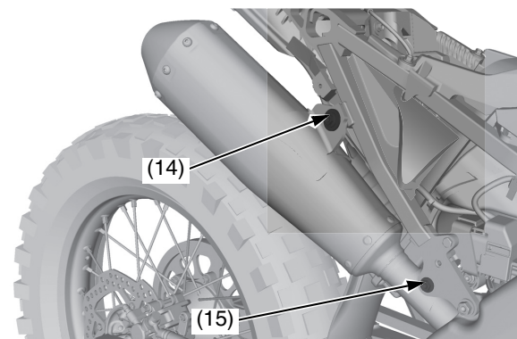
(14) tornillo de montaje B del silenciador derecho (15) tornillo de montaje A del silenciador derecho
