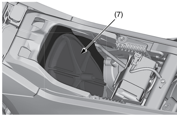
(7) Caja del filtro de aire
