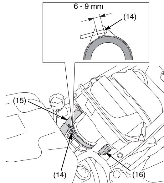
(14) tornillo de la abrazadera del tubo de conexión del filtro de aire (15) respiradero (16) conector del sensor IAT
