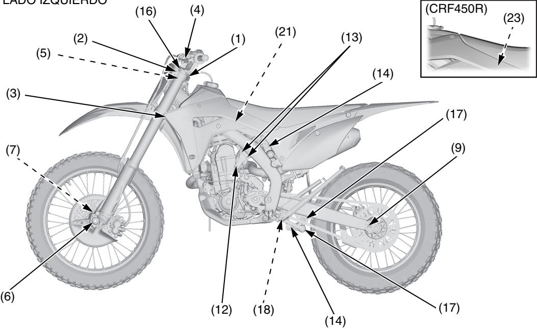
LADO IZQUIERDO
