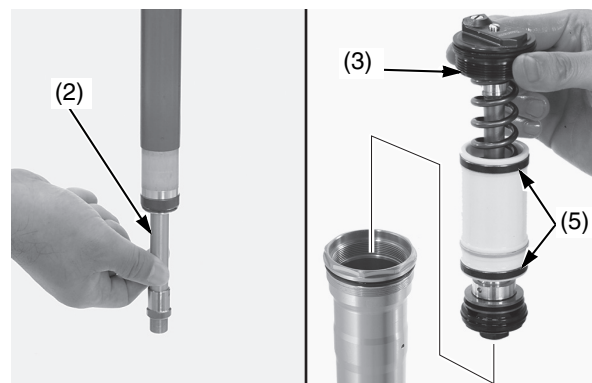
(2) barra del pistón del amortiguador de la horquilla (3) conjunto de tornillos de la horquilla (5) casquillos de los tornillos de la horquilla
