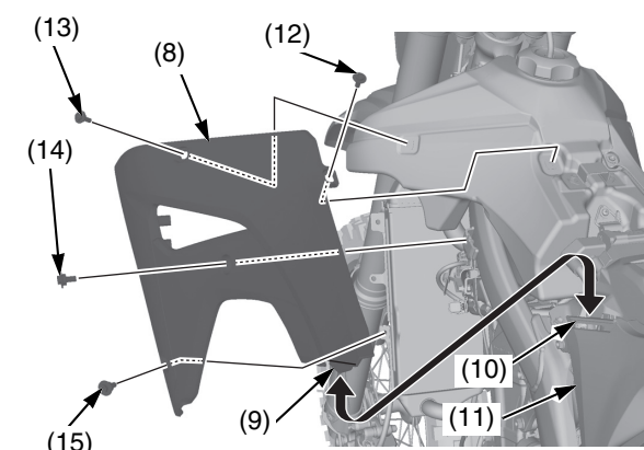
(8) cubierta (9) lengüeta (10) ranura (11) tapa del filtro de aire (12) tornillo D de la cubierta (13) tornillo C de la cubierta (14) tornillo B de la cubierta (15) tornillo A de la cubierta
