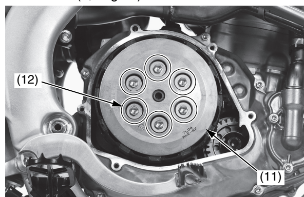
(11) prensa del embrague (12) muelles y tornillos del embrague
