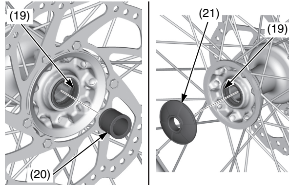
(19) labios del guardapolvos (20) casquillo del lado izquierdo (21) casquillo de lado derecho
