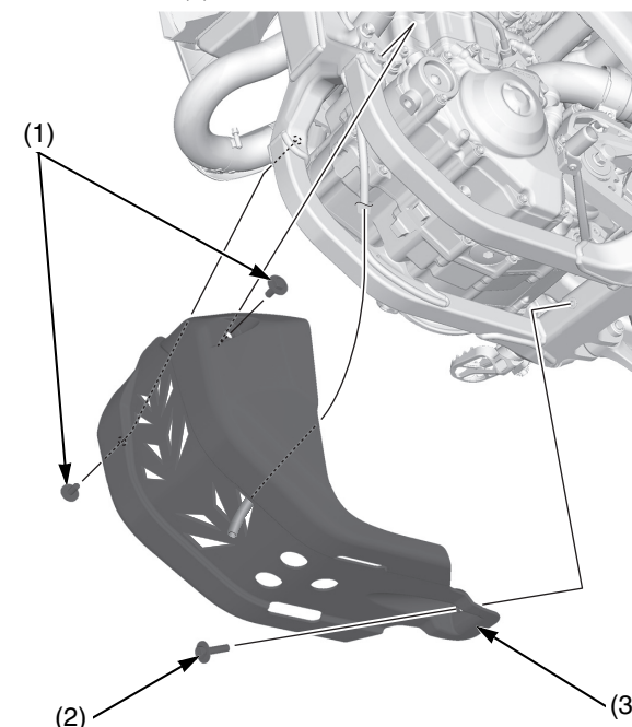
(1) arandelas/tornillos A del protector del motor (2) arandela/tornillos B del protector del motor (3) protector del motor
