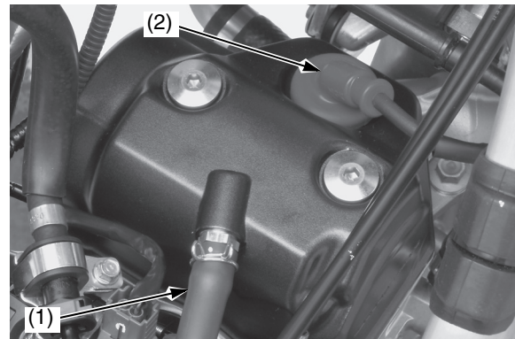
(1) respiradero
