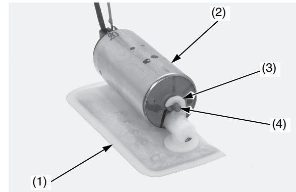
(1) filtro de la bomba de combustible (2) conjunto de la bomba de combustible (3) gancho (4) refuerzo de la junta
