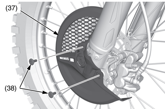
(37) tapa de disco (38) tornillos allen de la tapa del disco
