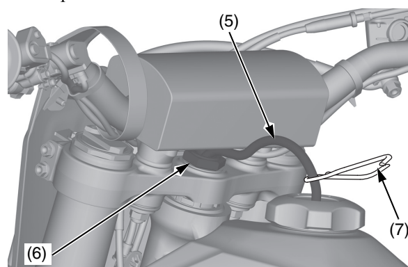
(5) respiradero (6) tuerca del vástago de dirección (7) abrazadera de manguera
