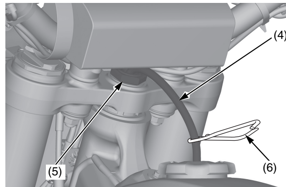
(4) respiradero (5) tuerca del vástago de dirección (6) abrazadera de manguera
