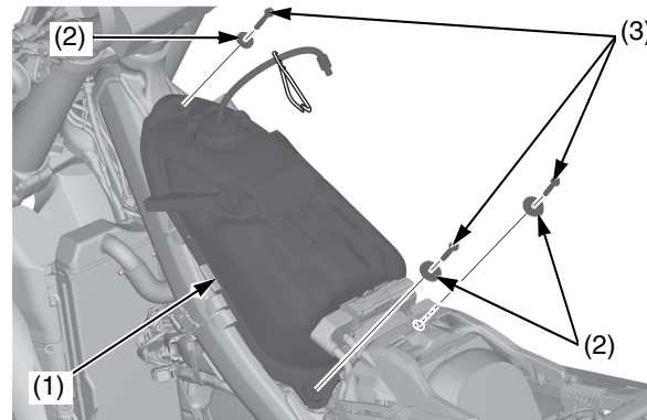
(1) depósito de combustible (2) arandelas (3) tornillos del depósito de combustible
