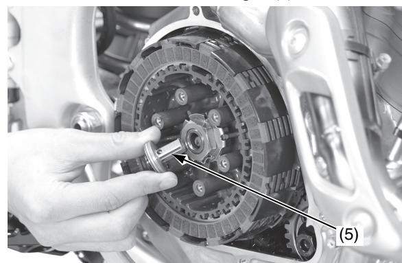
(5) elevador del embrague
