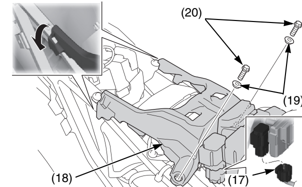
(17) conector del relé de encendido/motor de arranque (18) base de soporte del asiento (19) casquillos (20) tornillos de montaje de la base de soporte del asiento
