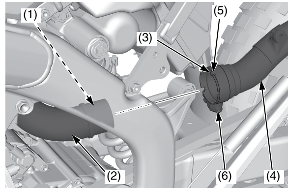
(1) junta (2) tubo de escape (3) recorte (4) silenciador izquierdo (5) lengüeta (6) abrazadera del silenciador izquierdo
