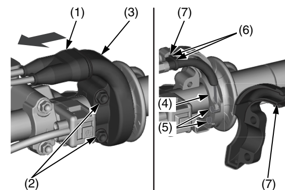
(1) guardapolvo (2) tornillos de la carcasa (3) caja del acelerador (4) tubo del acelerador (5) extremos del cable del acelerador (6) orejetas (7) ranuras
