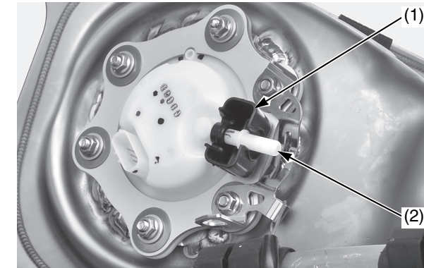
(1) tapa de goma (2) junta de combustible
