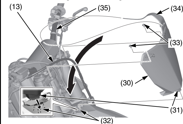
(13) latiguillo de freno (30) placa de matrícula (31) lengüeta (32) ranura (33) tornillos (34) lengüeta de la placa de matrícula (35) manillar
