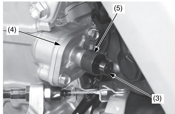
(3) tope de tensor (4) elevador del tensor de la cadena de distribución (5) maneta
