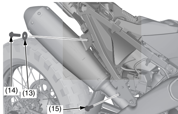
(13) arandela (14) tornillo de montaje B del silenciador derecho (15) tornillo de montaje A del silenciador derecho
