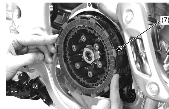
(7) discos del embrague, placas del embrague, aro cóncavo y asiento del muelle
