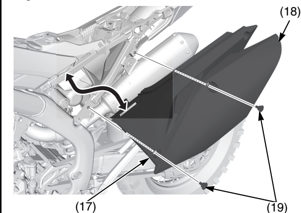
(17) tapas del filtro de aire (18) cubiertas laterales (19) tornillos
