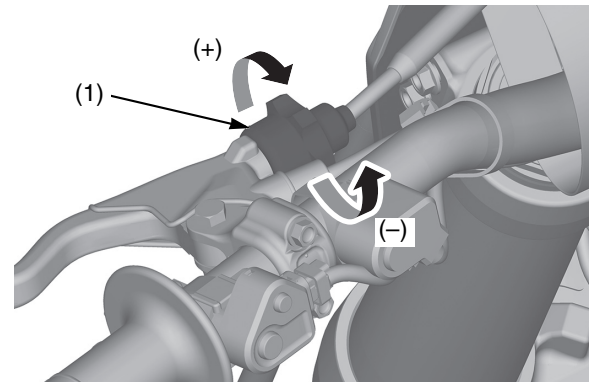
(1) mando de ajuste del extremo del cable
