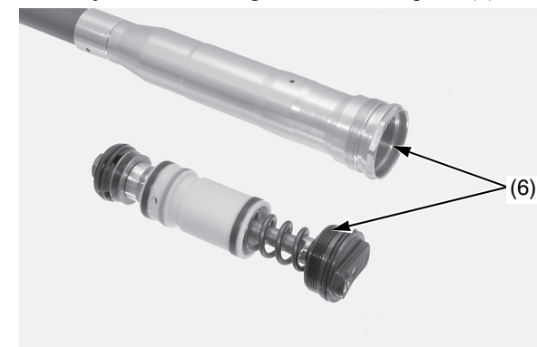
(6) tornillo de la horquilla y roscas del conjunto del amortiguador de la horquilla
