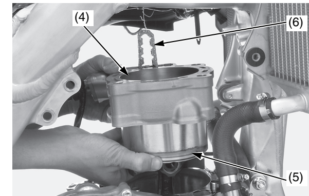
(4) diámetro del cilindro (5) segmentos (6) cadena de distribución
