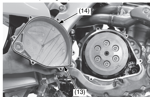
(13) junta tórica (nueva) (14) tapa del embrague
