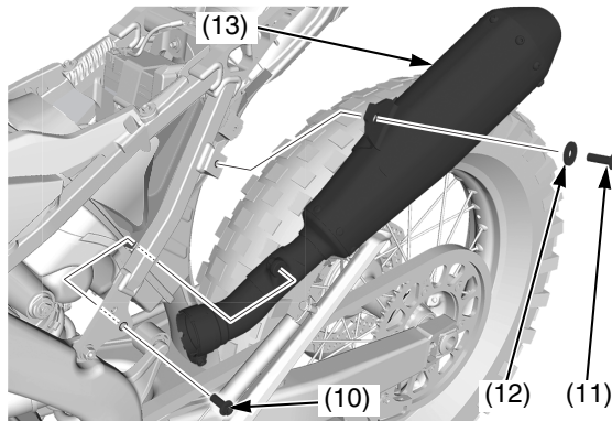
(10) tornillo A de montaje del silenciador izquierdo (11) tornillo B de montaje del silenciador izquierdo (12) arandela (13) silenciador izquierdo
