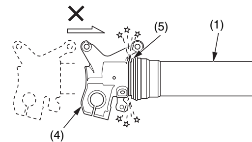
(1) tubo exterior (4) soporte del eje (5) guardapolvo de la horquilla
