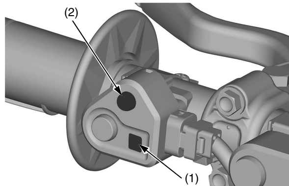
(1) indicador de modo del motor (azul) (2) botón de selección de modo del motor
