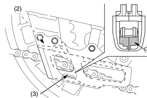
(2) deslizadera de la guía de la cadena (3) límite de desgaste
