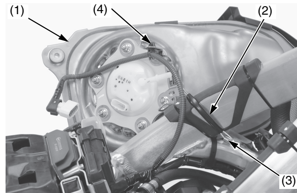
(1) depósito de combustible (3) gancho del bastidor (2) cable de tope (4) clip de la abrazadera del mazo de cables
