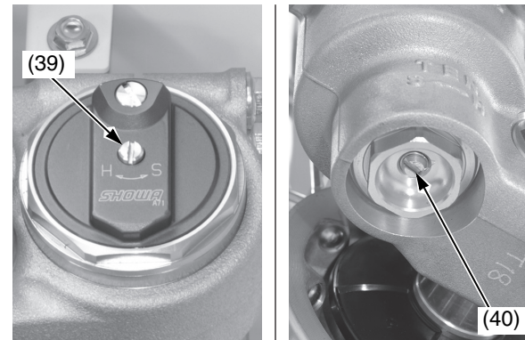
(39) mando de ajuste de amortiguación en compresión (40) mando de ajuste de amortiguación en extensión
