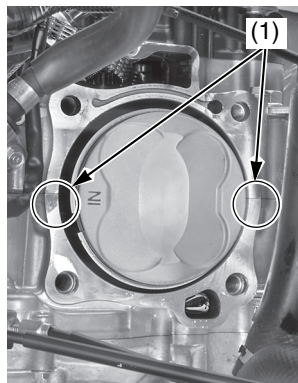
(1) superficie de acoplamiento del cilindro
