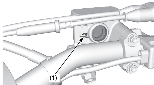
(1) marca LWR
