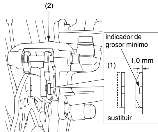
(1) pastillas de freno (2) pinza de freno trasero
