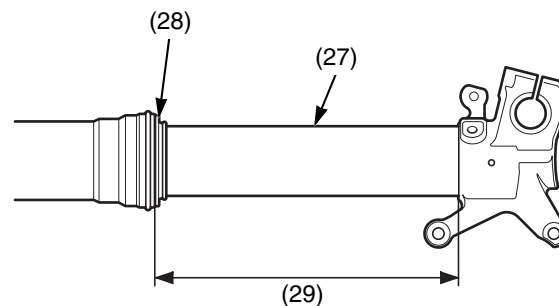
(27) superficie de deslizamiento (28) guardapolvo de la horquilla (29) longitud
