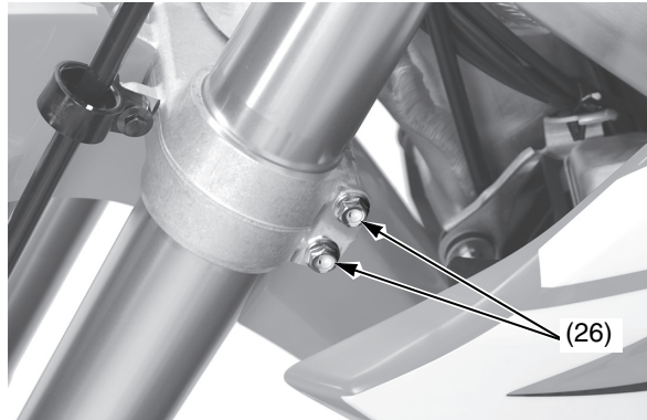
(26) tornillos de bloqueo inferiores del puente de la horquilla
