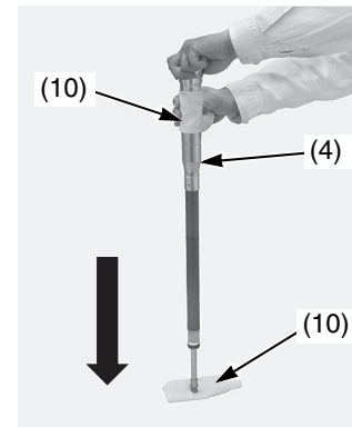
(4) conjunto del amortiguador de la horquilla (10) trapo de taller
