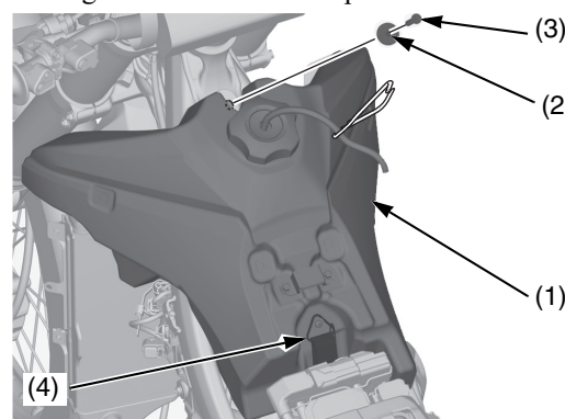
(1) depósito de combustible (2) casquillo (3) tornillo del depósito de combustible (4) banda del depósito de combustible
