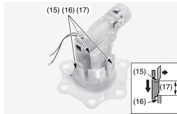
(15) ganchos (16) lengüetas
