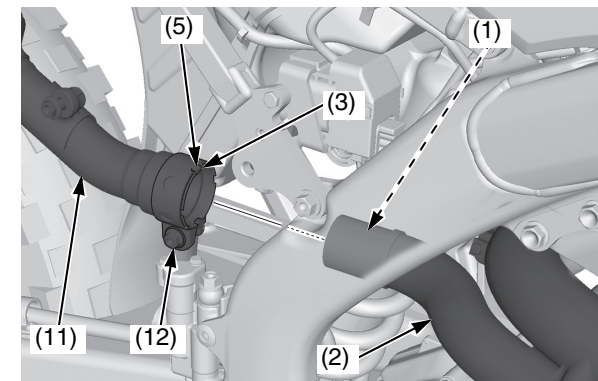
(1) junta (2) tubo de escape (3) recorte (5) lengüeta (11) silenciador derecho (12) abrazadera del silenciador derecho
