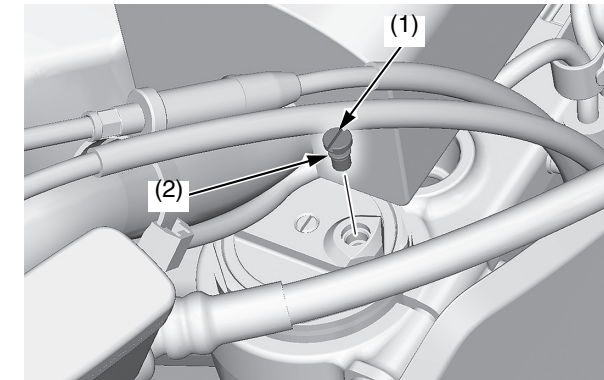
(1) tornillo de liberación de presión (2) junta tórica (nueva)
