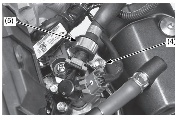
(4) tornillo
