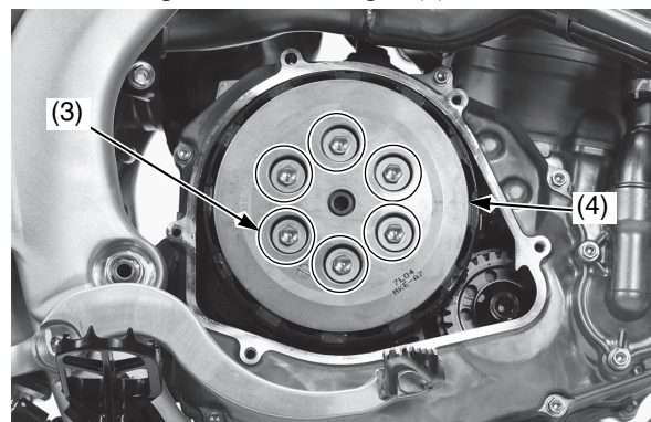
(3) tornillos de los muelles del embrague y muelles (4) prensa del embrague
