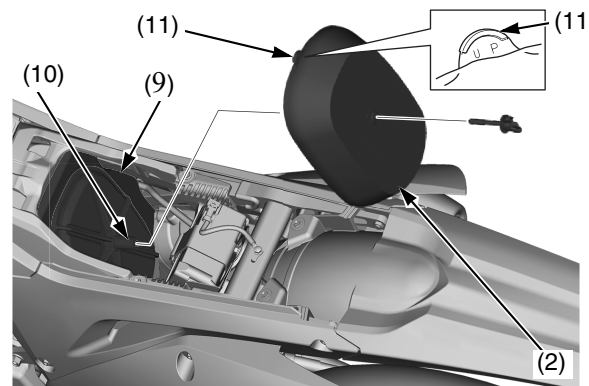
(2) conjunto del filtro de aire (9) área de contacto (10) soporte de la caja del filtro de aire (11) lengüeta con marca "UP" (arriba)
