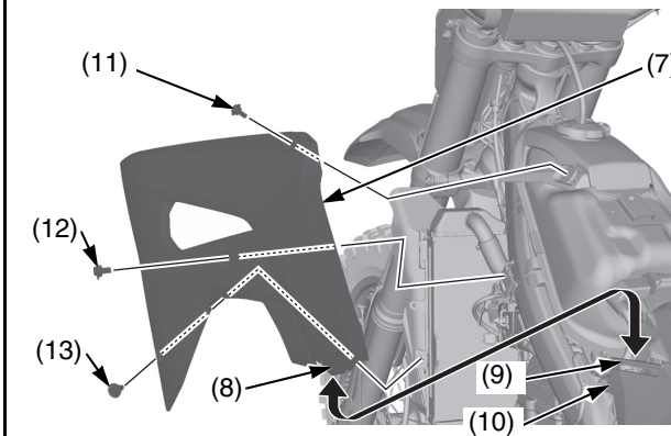
(7) cubierta (8) lengüeta (9) ranura (10) tapa del filtro de aire (11) tornillo C de la cubierta (12) tornillo B de la cubierta (13) tornillo A de la cubierta
