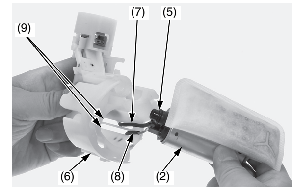
(2) conjunto de la bomba de combustible (5) junta tórica (nueva) (6) soporte de la unidad de la bomba de combustible (7) cable amarillo (8) cable verde (9) ranuras
