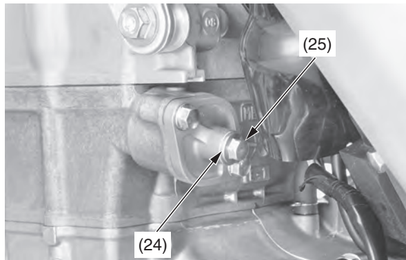
(24) arandela de sellado (nueva) (25) perno de la cubierta del alzador del tensor de la cadena de levas
