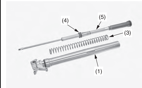
(1) conjunto de la horquilla (3) resorte de la horquilla (4) retenedor del resorte (5) conjunto del amortiguador de la horquilla
