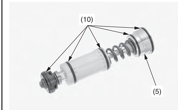
(5) conjunto de la tapa de la horquilla (10) juntas tóricas (nuevas)
