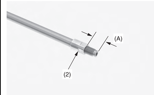
(2) contratuerca del perno central de la horquilla (A) longitud de la rosca
