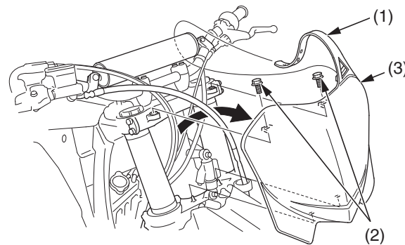
(1) lengüeta de la placa de la matrícula (2) pernos (3) matrícula
