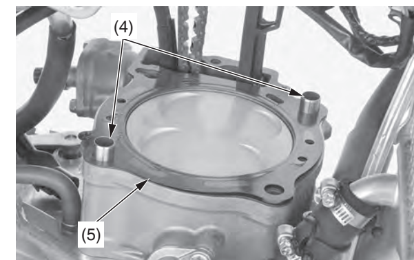
(4) pasadores cónicos (5) empaquetadura de la culata
