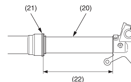
(20) superficie de deslizamiento (21) sello contra el polvo de la horquilla
