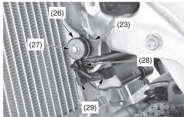
(23) bobina de encendido/soporte (26) arandela (27) perno (28) abrazadera (29) conectores de la bobina de encendido
