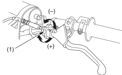
(1) ajustador del extremo del cable (+) aumentar el juego libre (-) reducir el juego libre
