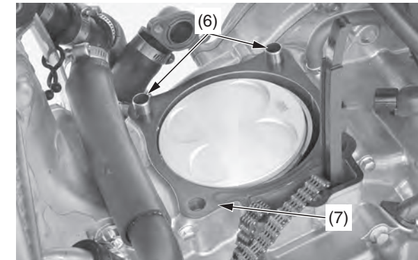
(6) pasadores cónicos (7) empaquetadura del cilindro
