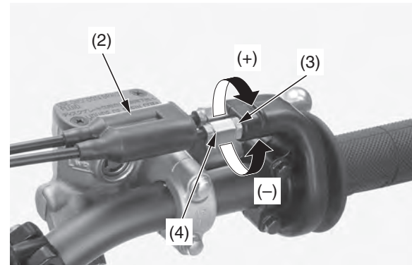
(2) cubierta contra el polvo (+) incrementar (3) contratuerca (–) reducir (4) ajustador
