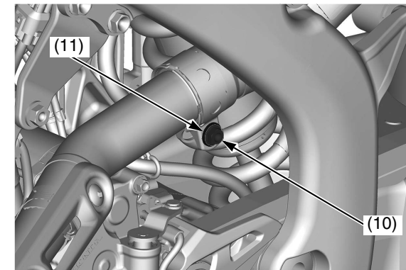
(10) tornillo de la abrazadera (11) arandela del silenciador izquierdo
