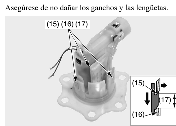
(15) ganchos (16) lengüetas
