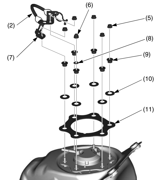
(2) cable de tope (5) tuercas de montaje de la bomba de combustible (6) tuerca de sombrerete de montaje de la bomba de combustible (7) guía del cable de tope (8) arandela (9) casquillos (10) arandelas de muelle cónicas (11) placa de la bomba de combustible
