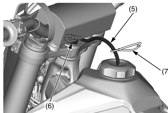
(5) respiradero (7) abrazadera de manguera (6) tuerca del vástago de dirección
