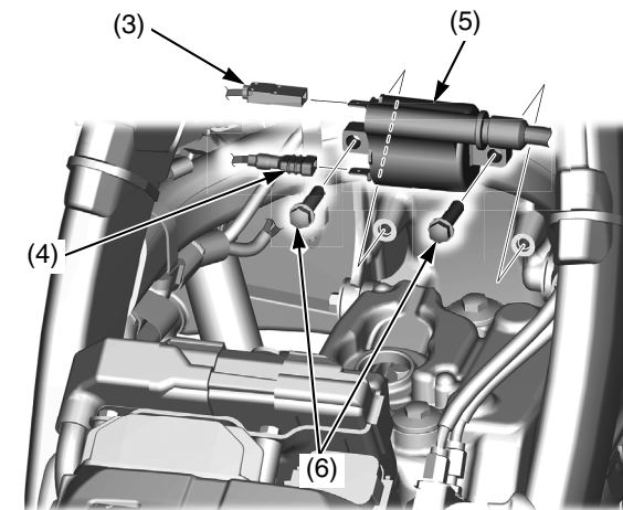
(3) conector A de la bobina de encendido
