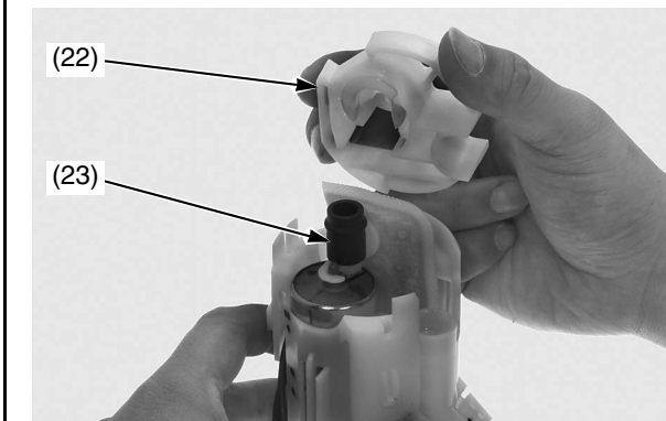
(22) tope de la bomba de combustible (23) amortiguador de goma
