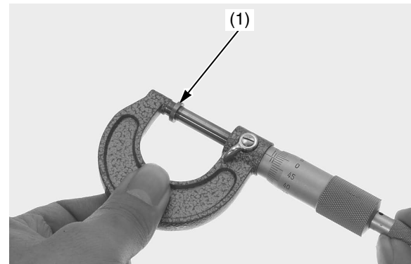
(1) suplemento
