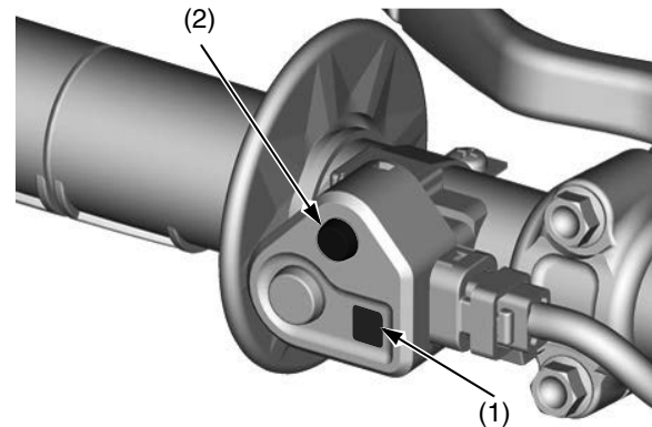
(1) indicador del sistema de control de lanzamiento (morado) (2) botón de selección de modo del motor
