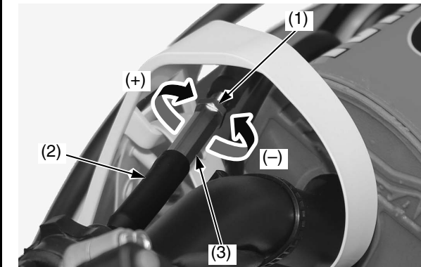
(1) contratuerca (2) funda de goma (3) mando de ajuste de cable integral (+) aumento de holgura (-) reducción de holgura
