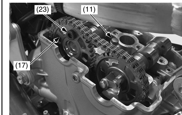
(11) tornillo de tope del eje del balancín (17) corona del árbol de levas de admisión (23) tornillo de la corona del árbol de levas
