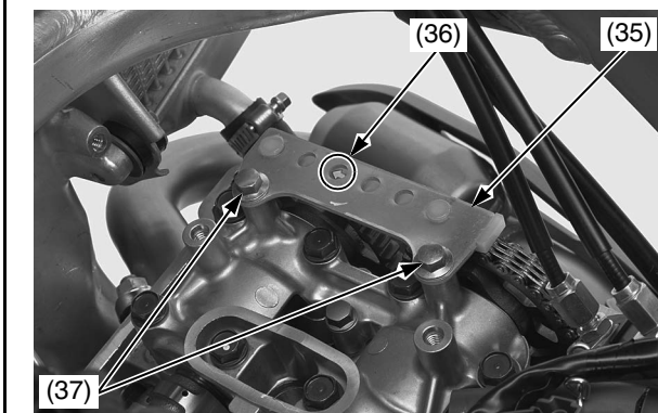
(35) guía de la cadena de distribución (36) marca “↔” (37) tornillos guía de la cadena de distribución
