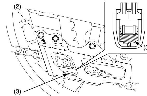
(2) deslizadera de la guía (3) límite de desgaste de la cadena
