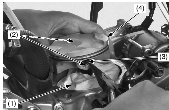
(1) trapo de taller (2) clips del bulón del pistón (3) bulón del pistón (4) pistón
