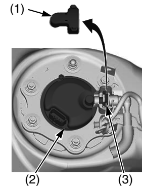
(1) tapa del racor del conector rápido de combustible (2) bomba de combustible (3) racor del conector rápido de combustible
