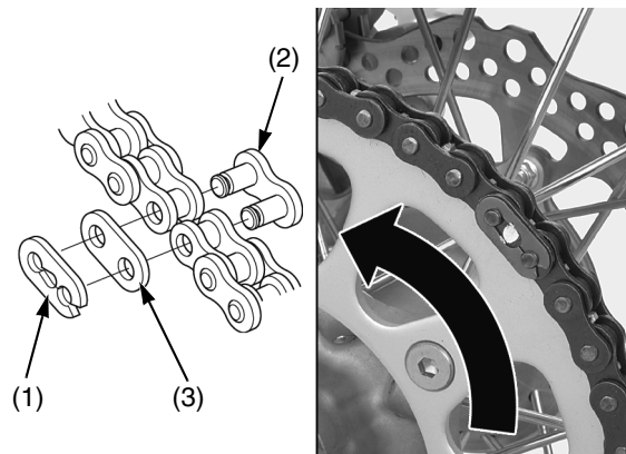
(1) circlip del eslabón de cierre (3) placa de eslabón (2) eslabón de cierre
