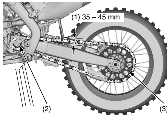
(1) holgura de la cadena de transmisión (2) piñón (3) corona
