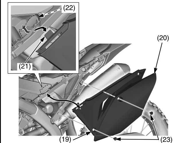
(19) tapa del filtro de aire (20) tapa lateral (21) pestaña de la tapa del filtro de aire (22) ranura de la base de soporte del asiento (23) tornillos
