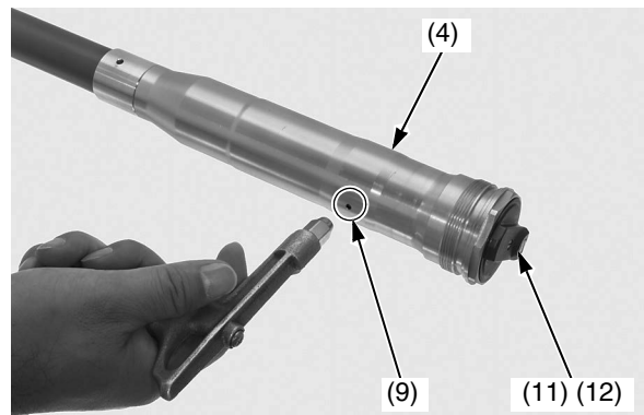
(4) conjunto del amortiguador de la horquilla (9) orificio de lubricación (11) tornillos de liberación de la presión de aire (12) juntas tóricas (nuevas)
