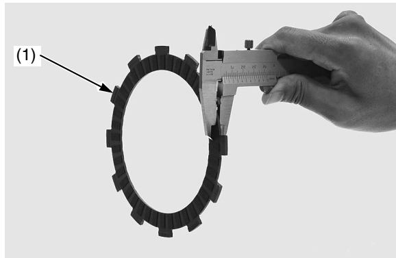
(1) disco del embrague
