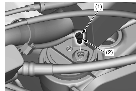
(1) tornillo de liberación de la presión de aire (2) junta tórica (nueva)
