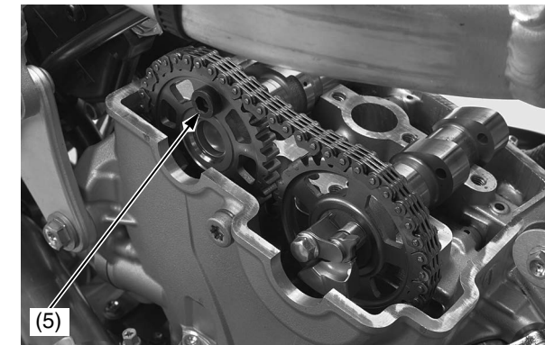
(5) tornillo de la corona del árbol de levas
