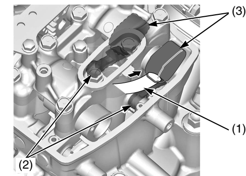
(1) galga de espesores (3) lóbulos de leva del árbol de levas (2) balancines de admisión
