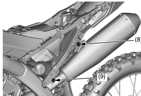
(8) tornillo B de montaje del silenciador izquierdo (9) tornillo A de montaje del silenciador izquierdo
