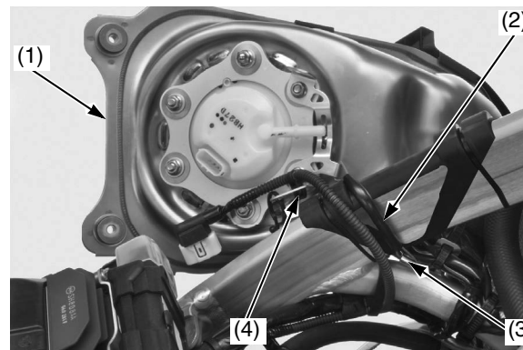
(1) depósito de combustible (2) cable de tope (3) gancho del bastidor (4) clip de la abrazadera del mazo de cables
