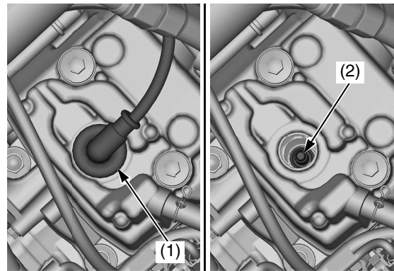
(1) pipa de la bujía
