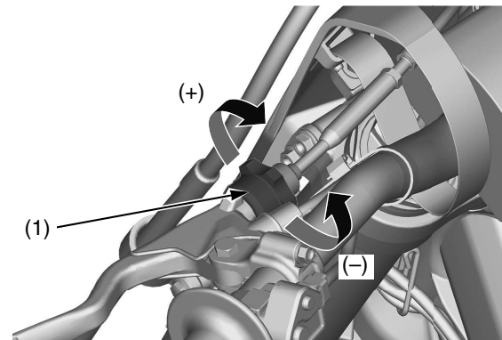
(1) mando de ajuste del extremo del cable (+) aumento de holgura (-) reducción de holgura
