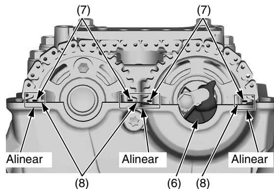
(6) peso del descompresor (7) marcas de sincronización (8) superficie de contacto de la culata
