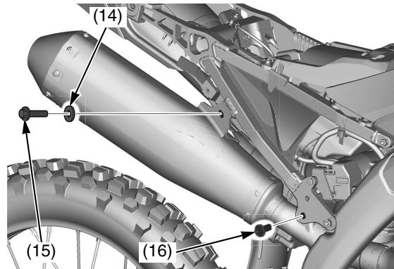
(14) arandela (15) tornillo de montaje B del silenciador derecho (16) tornillo de montaje A del silenciador derecho
