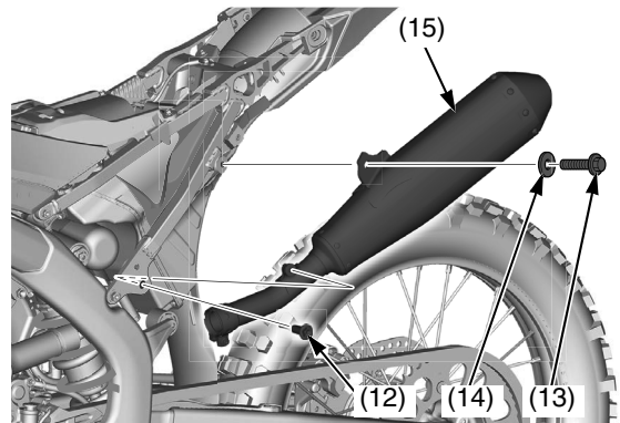
(12) tornillo A de montaje del silenciador izquierdo (13) tornillo B de montaje del silenciador izquierdo (14) arandela (15) silenciador izquierdo
