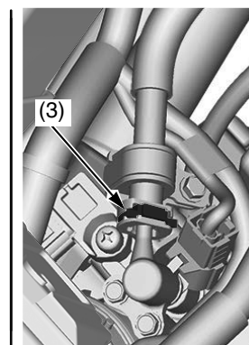
(1) tapa del racor del conector rápido de combustible (2) bomba de combustible (3) racor del conector rápido de combustible
