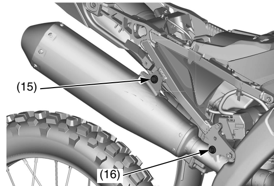
(15) tornillo de montaje B del silenciador derecho (16) tornillo de montaje A del silenciador derecho
