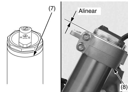
(7) ranura
