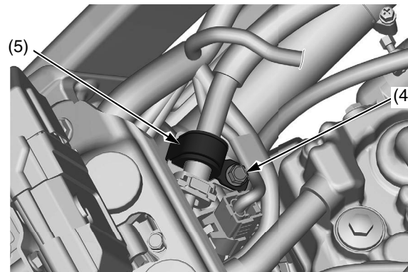
(4) tornillo (5) abrazadera y goma de ajuste
