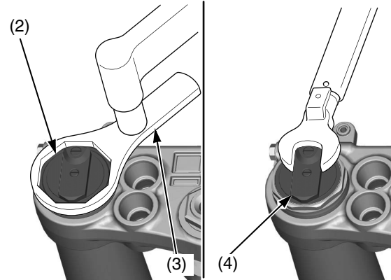
(2) conjunto del amortiguador de la horquilla (3) llave para contratuercas (4) conjunto de tornillos de la horquilla
