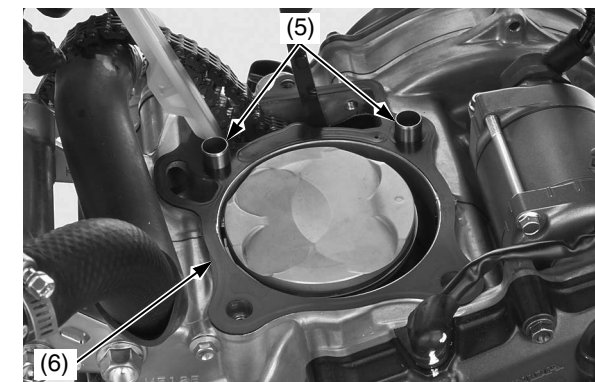
(5) pasadores de espiga (6) junta del cilindro
