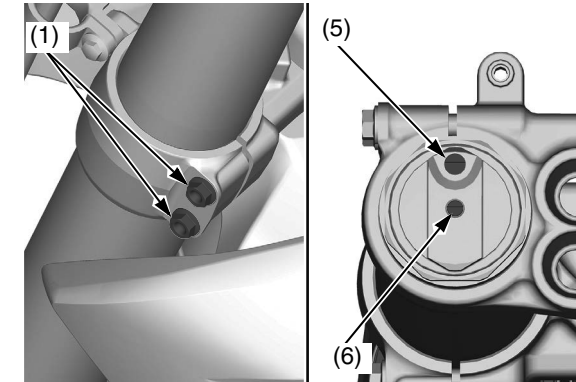
(1) tornillos de bloqueo inferiores del puente de la horquilla (5) tornillo de liberación de la presión de aire (6) mando de ajuste de amortiguación en compresión
