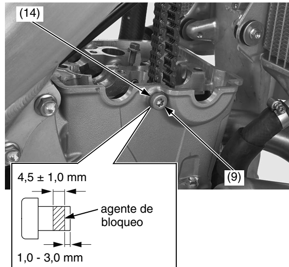
(9) tornillo de sellado (14) arandela de sellado (nueva)
