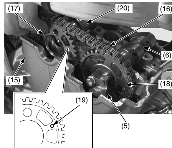
(5) peso del descompresor (17) corona del árbol de levas de admisión (6) árbol de levas de escape (18) corona del árbol de levas de escape (15) culata (19) marca "O" (16) cadena de distribución (20) árbol de levas de admisión
