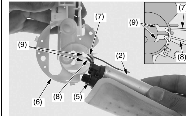
(2) conjunto de la bomba de combustible (7) cable rojo (5) junta tórica (nueva) (8) cable negro (6) soporte de la unidad de la bomba de combustible (9) ranuras
