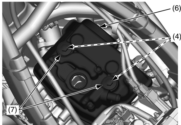
(4) juntas de goma (6) tapa de la culata (7) tornillos huecos de la tapa de la culata
