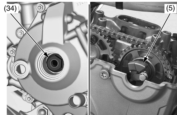
(5) peso del descompresor (34) volante de inercia
