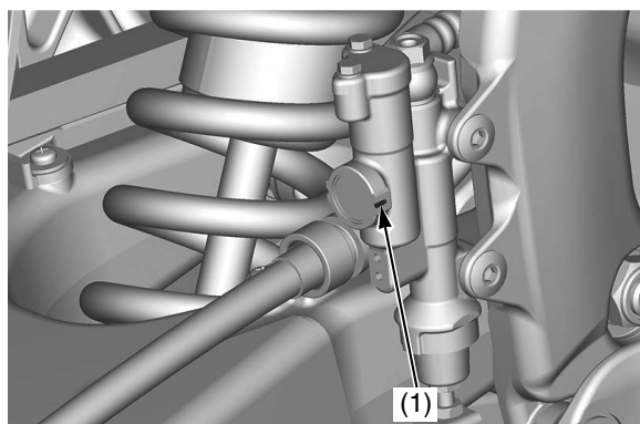
(1) marca LOWER
