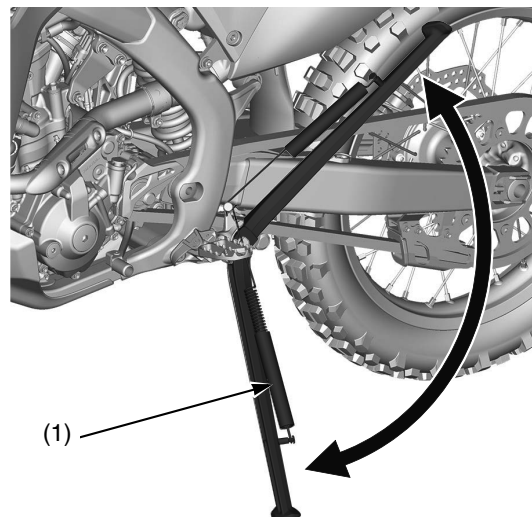
(1) muelle del caballote lateral
