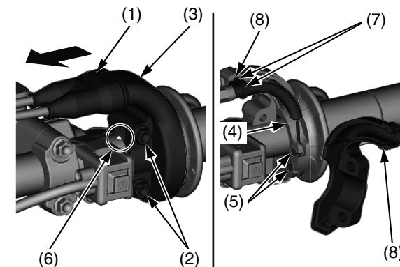
(1) guardapolvo (2) tornillos de la carcasa (3) caja del acelerador (4) tubo del acelerador (5) extremos del cable del acelerador (6) marca de pintura (7) orejetas (8) ranuras
