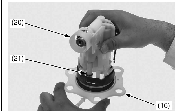
(16) base de la bomba de combustible (20) conjunto del soporte de la unidad de la bomba de combustible (21) junta tórica
