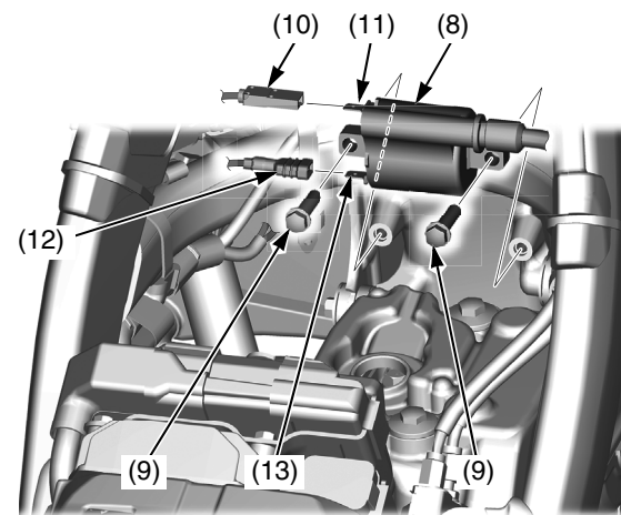
(8) bobina de encendido (9) tornillos de la bobina de encendido (10) conector A de la bobina de encendido (11) terminal azul (12) conector B de la bobina de encendido (13) terminal negro
