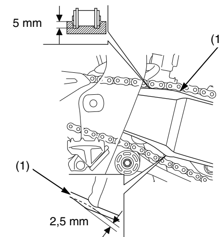
(1) guía de la cadena
