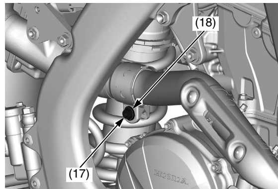
(17) tornillo de fijación del silenciador derecho (18) arandela
