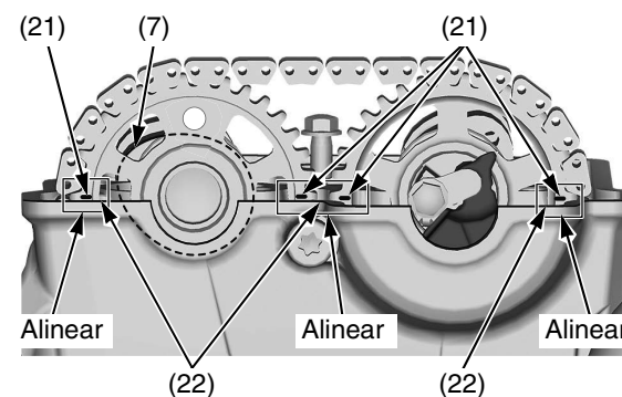
(7) lóbulo de leva del árbol de levas (21) marcas de sincronización (22) superficie de contacto de la culata
