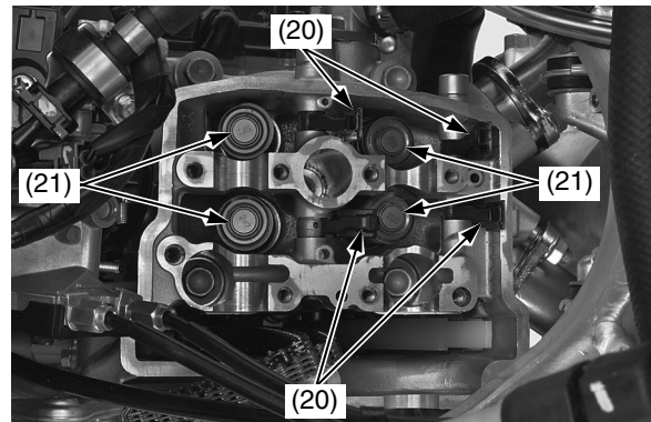
(20) balancines (21) suplementos
