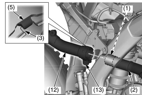
(1) junta (2) tubo de escape (3) recorte (5) lengüeta (12) silenciador derecho (13) abrazadera del silenciador derecho
