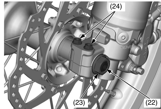
(22) eje delantero (23) tuerca del eje delantero (24) tornillos de bloqueo izquierdos del eje
