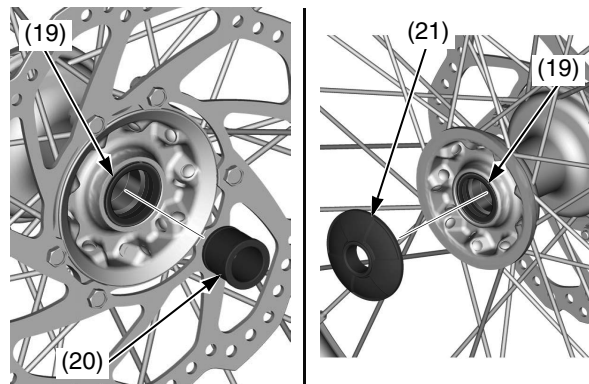
(19) labios del guardapolvos (20) casquillo del lado izquierdo
