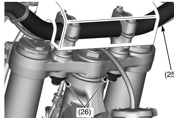
(25) manillar (26) monturas de goma, arandelas y tuercas del soporte inferior del manillar
