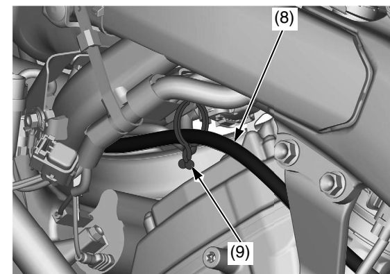
(8) manguito de rebose (9) abrazadera
