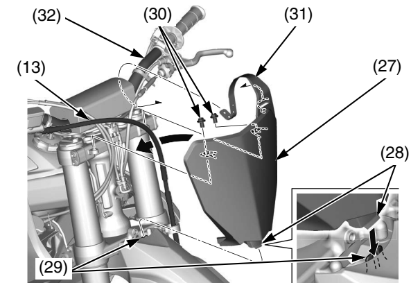
(13) latiguillo de freno (27) placa de matrícula (28) lengüeta (29) ranura (30) tornillos de la placa de matrícula (31) lengüeta de la placa de matrícula (32) manillar
