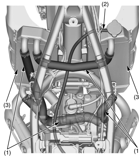
(1) manguitos del radiador (3) aletas del radiador (2) manguito de rebose
