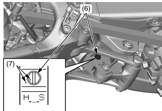
(6) mando de ajuste de amortiguación en extensión (7) marcas de punzón
