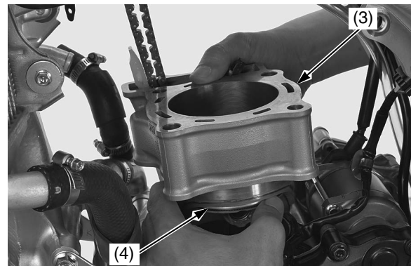
(3) cilindro (4) pistón
