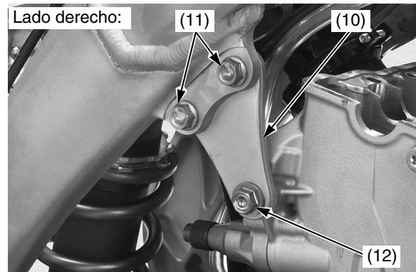
(9) placa izquierda del anclaje de la culata izquierda (10) placa derecha del anclaje de la culata (11) tornillos de las placas del anclaje de la culata (12) tornillos del anclaje de la culata
