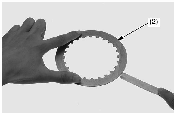
(2) placa del embrague
