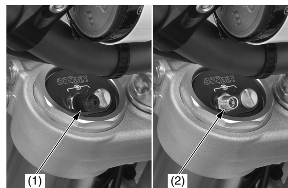
(1) tapón de la válvula (2) válvula de aire de la cámara interior
