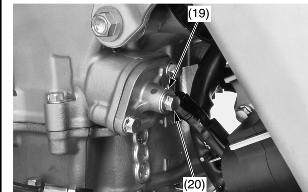
(19) arandela de sellado (nueva) (20) perno de la cubierta del alzador del tensor de la cadena de levas
