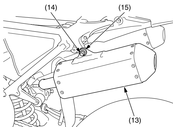
(13) silenciador izquierdo (14) perno de montaje del silenciador izquierdo (15) arandela
