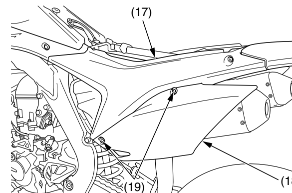
(17) cubiertas del alojamiento del filtro de aire (18) cubiertas laterales (19) pernos
