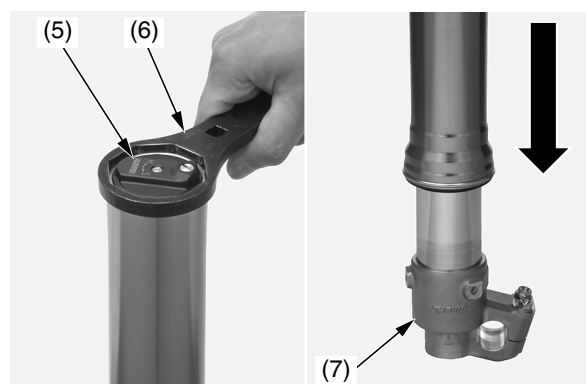
(5) amortiguador de la horquilla (6) llave de contratuercas (7) soporte del eje
