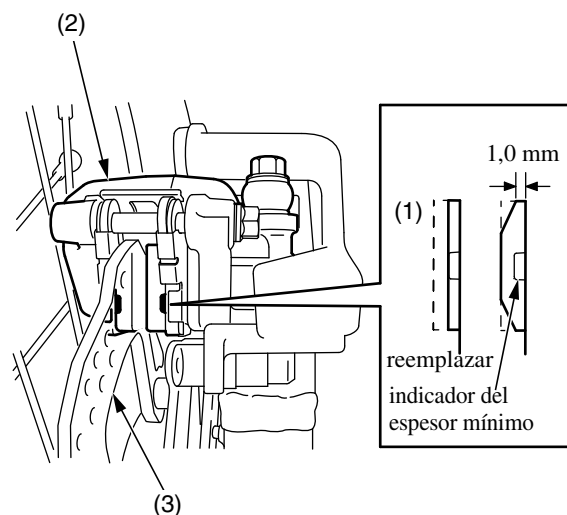
(1) pastillas del freno (3) disco del freno (2) pinza del freno trasero
