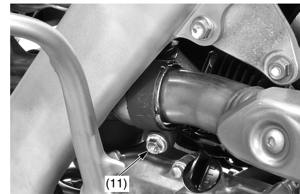
(11) perno de la abrazadera del silenciador derecho
