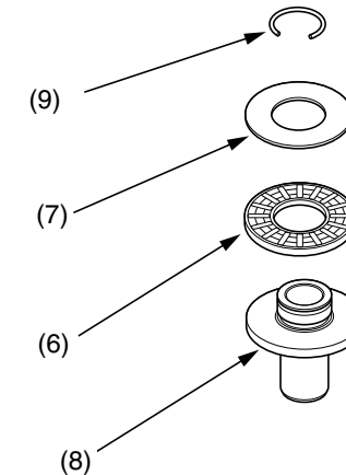
(6) cojinete de agujas (7) arandela (8) alizador del embrague (9) retenedor (nuevo)
