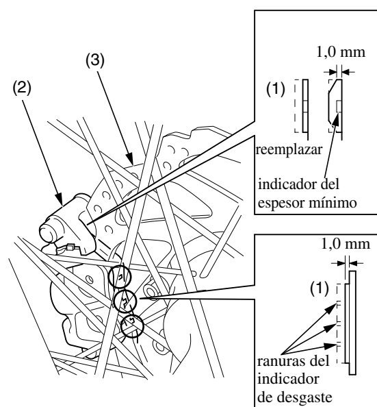
(1) pastillas del freno (3) disco del freno (2) pinza del freno delantero
