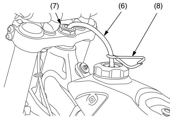
(6) tubo del respiradero (7) tuerca del vástago de dirección (8) abrazadera de manguera
