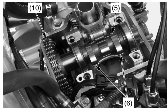
(5) árbol de levas (6) lóbulos de las levas de admisión (10) cadena de levas
