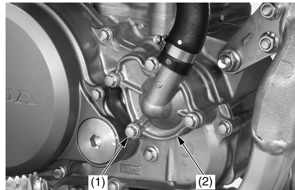
(1) perno de drenaje del refrigerante y arandela de sellado (nuevo) (2) cubierta de la bomba de agua
