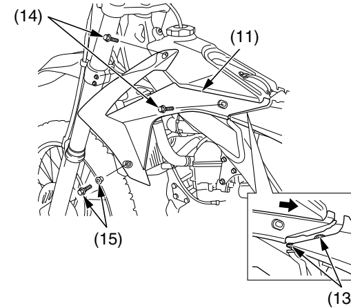
(11) protectores (13) lengüetas de la cubierta de la caja del filtro de aire (14) pernos B de los protectores (15) collares y pernos A de los protectores
