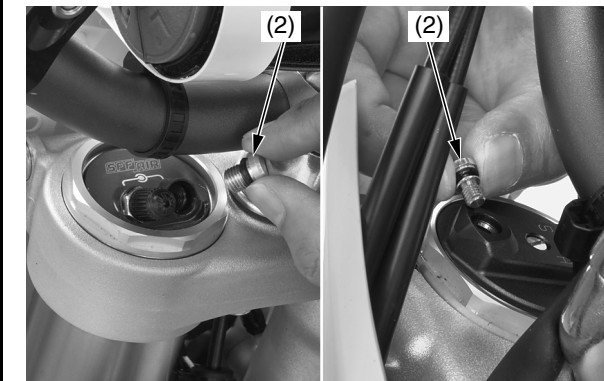
(2) tornillos de liberación de la presión
