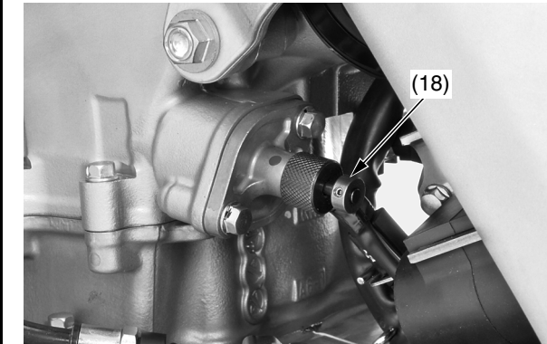
(18) tope del tensor
