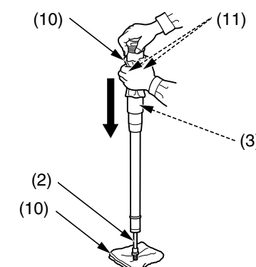
(2) barra del pistón del amortiguador de la horquilla (3) cámara de aceite del amortiguador de la horquilla (10) paño de taller (11) orificios de aceite
