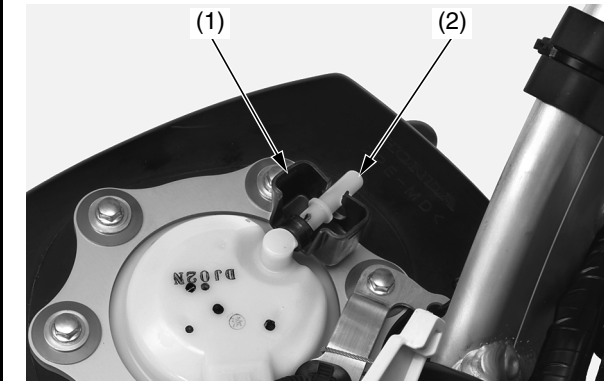
(1) cubierta de goma (2) junta de combustible
