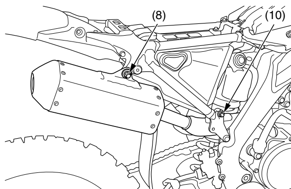
(8) perno B de montaje del silenciador derecho (10) perno A de montaje del silenciador derecho
