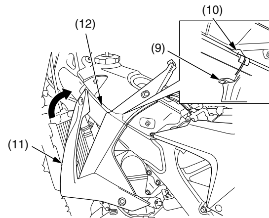
(9) ganchos de los protectores (10) huecos (11) protectores (12) bastidor
