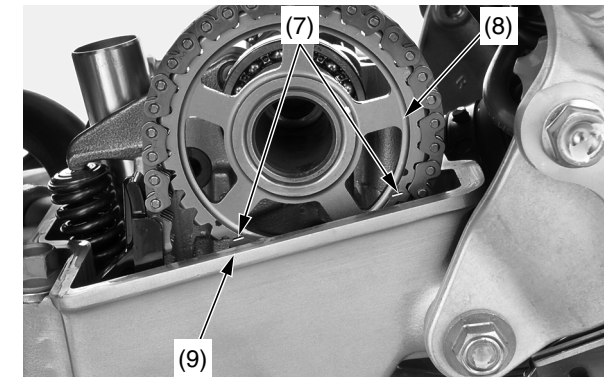
(7) marcas de distribución (8) rueda dentada de levas (9) cubierta de la culata
