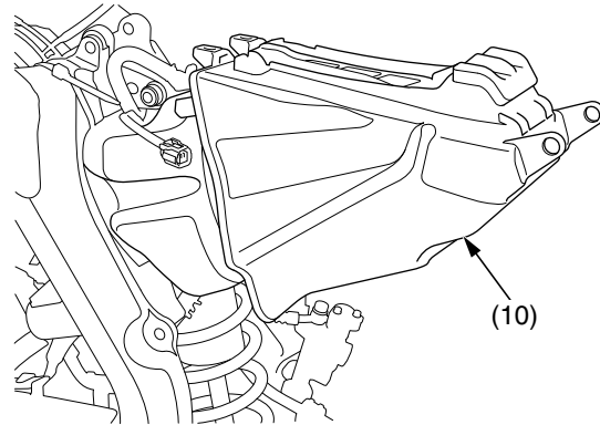
(10) caja del filtro de aire
