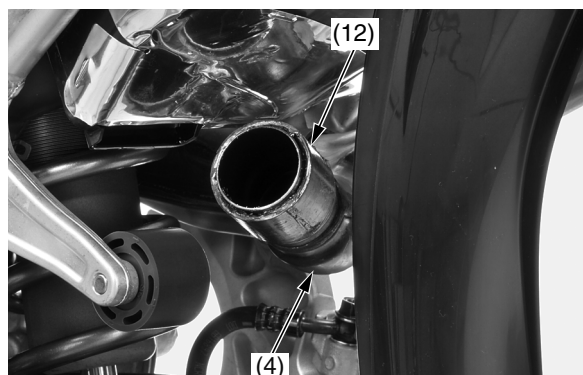
(4) silenciador derecho (12) empaquetadura (nueva)
