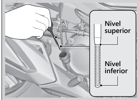
Tapón de llenado/varilla de aceite
