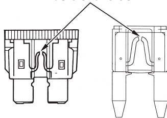
Fusible fundido
