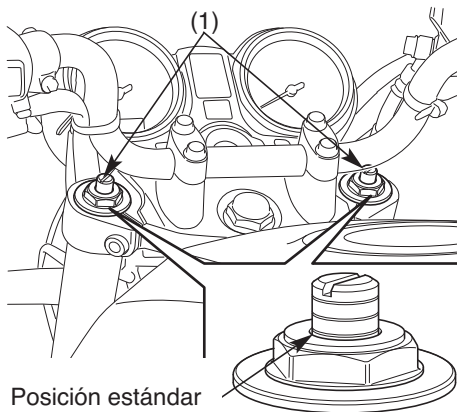
(1) Regulación pre-carga
