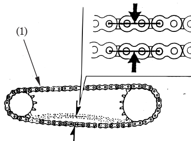
(1) Cadena de transmisión
