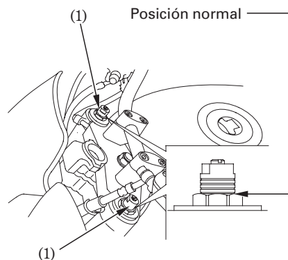
(1) Regulador de precarga
