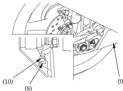
(8) Ranura (10) Lengüeta (9) Horquilla oscilante
