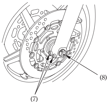
(7) Pernos de retención del eje (8) Eje delantero
