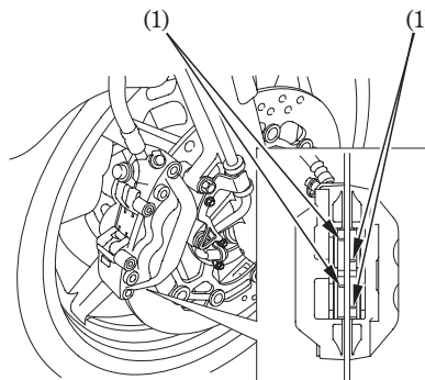
(1) Ranuras indicadoras de desgaste
