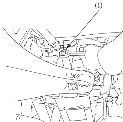
(1) Llave de bujías
