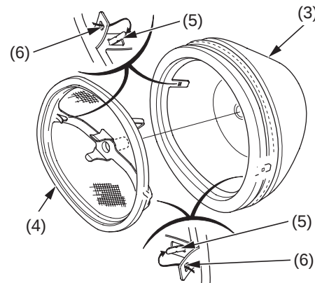
(3) elemento del filtro de aire (5) lengüetas del soporte (4) soporte del filtro de aire (6) orificios
