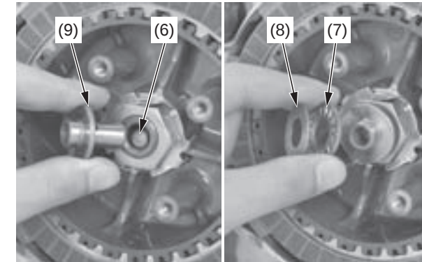
(6) barra del alzador del embrague (7) cojinete de agujas (8) arandela (9) alzador del embrague
