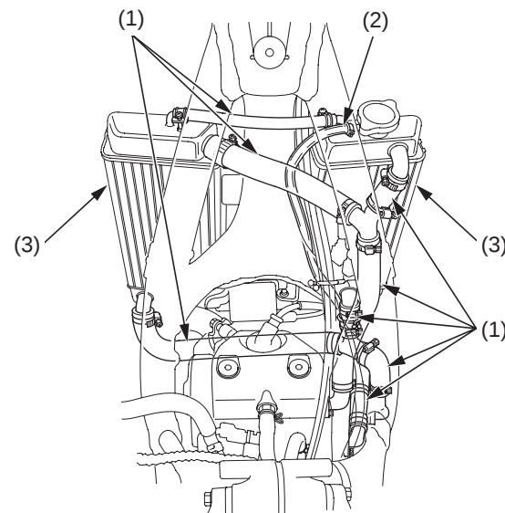
(1) mangueras de agua (3) aletas del radiador (2) manguera de rebose
