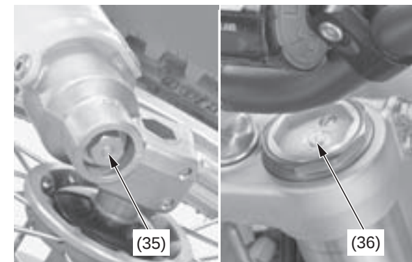
(35) ajustador de la amortiguación de expansión (36) ajustador de la amortiguación de compresión
