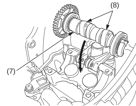
(7) árbol de levas (8) lóbulos de las levas de admisión
