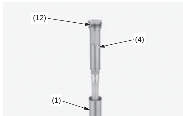
(1) conjunto de la horquilla (12) junta tórica (4) conjunto del amortiguador de la horquilla
