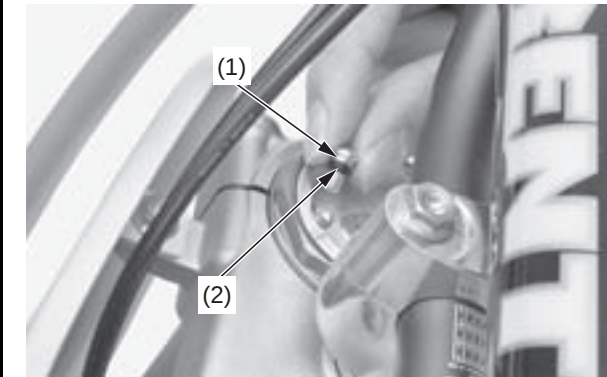
(1) tornillo de liberación de presión de aire de la horquilla (2) junta tórica
