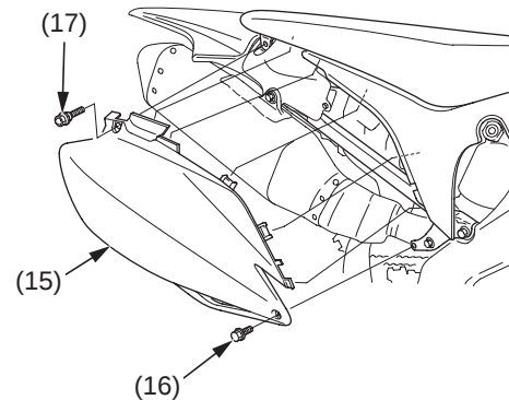
(15) cubierta lateral derecha (16) perno (17) perno de montaje del asiento
