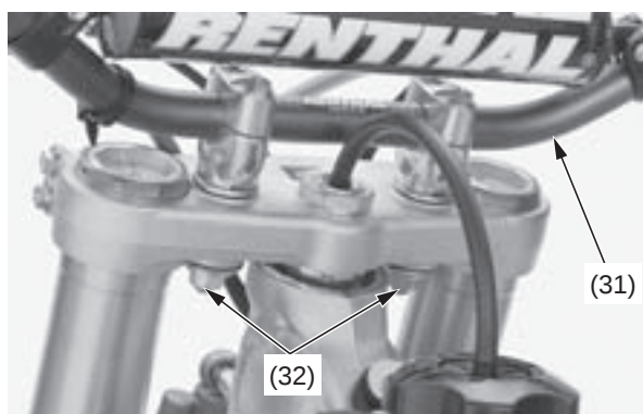
(31) manillar (32) gomas de montaje, arandelas y tuercas del soporte inferior del manillar
