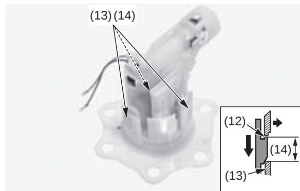
(12) ganchos (13) lengüetas
