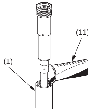
(1) conjunto de la horquilla (11) aceite de la horquilla
