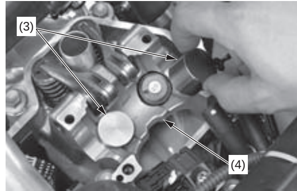
(3) alzávalvulas (4) culata
