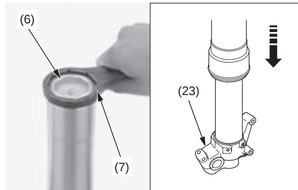
(6) amortiguador de la horquilla (7) llave de contratuerzas
