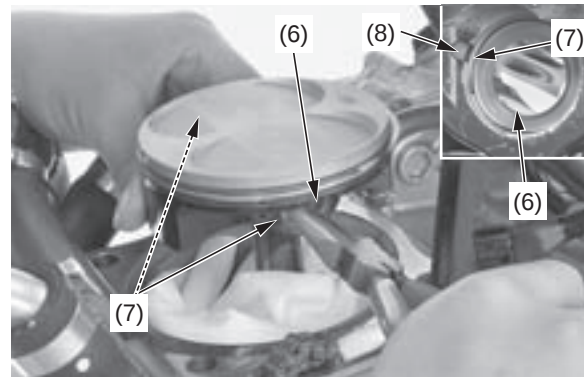
(6) pasador del pistón (8) corte del pistón (7) retenedores del pasador del pistón
