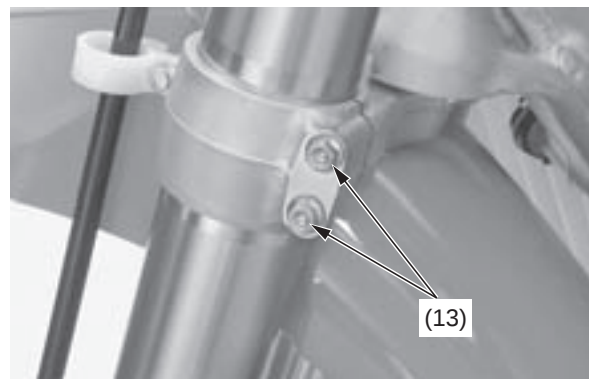
(13) pernos de fijación inferiores del puente de la horquilla
