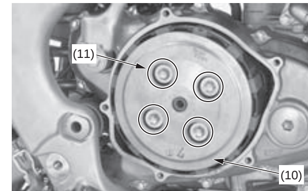
(10) placa de presión del embrague (11) resortes y pernos del embrague
