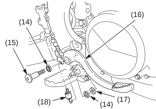
(14) sellos contra el polvo (15) perno del pivote del pedal del freno (16) pedal del freno trasero (17) arandela (18) resorte de retorno del pedal del freno
