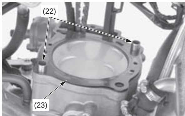
(22) pasadores cónicos (23) empaquetadura de la culata
