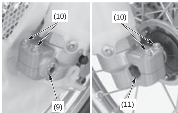
(9) tuerca del eje delantero (10) pernos de fijación del eje
