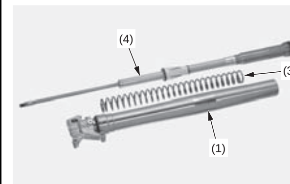
(1) conjunto de la horquilla (3) resorte de la horquilla (4) conjunto del amortiguador de la horquilla
