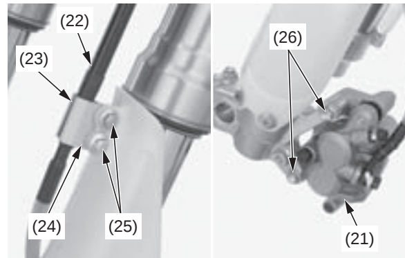
(21) pinza del freno (22) manguera del freno (23) soporte B (24) soporte A (25) pernos de la abrazadera de la manguera del freno (26) pernos de montaje de la pinza del freno
