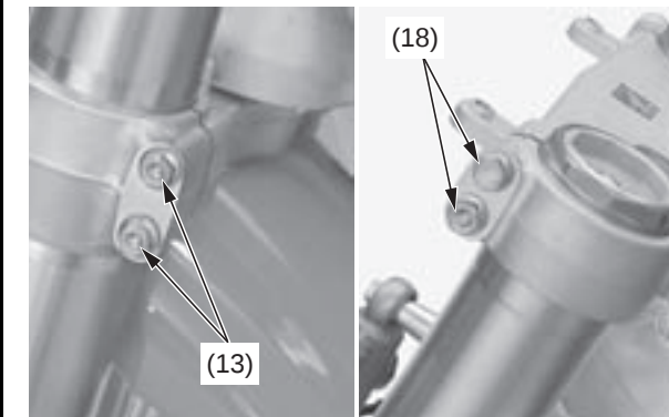
(13) pernos de fijación inferiores del puente de la horquilla (18) pernos de fijación superiores del puente de la horquilla
