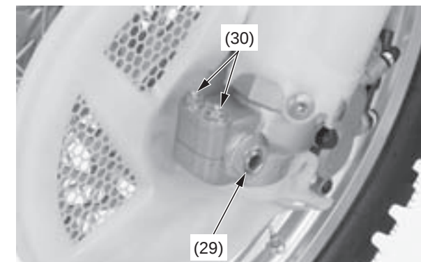
(29) tuerca del eje delantero (30) pernos de fijación del eje izquierdo
