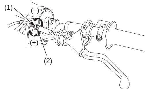
(1) contratuerca (+) aumentar el juego libre (2) ajustador del cable integral (-) reducir el juego libre
