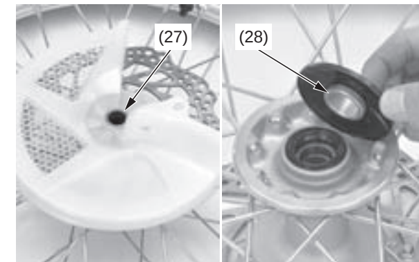
(27) cubierta del disco/collar (28) collar del lado derecho
