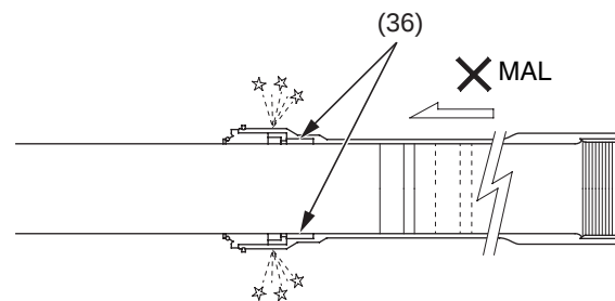
(36) bujes de la guía
