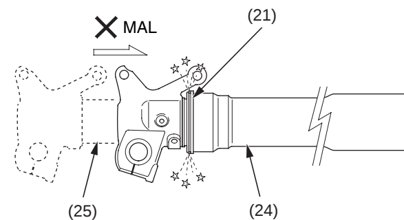
(21) sello contra el polvo de la horquilla (24) tubo exterior
