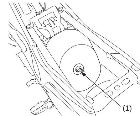
(1) perno de retención del filtro de aire
