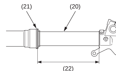
(20) superficie de deslizamiento (21) sello contra el polvo de la horquilla
