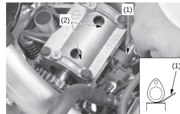
(1) calibre de espesores (2) alzaválvulas y lóbulos de leva
