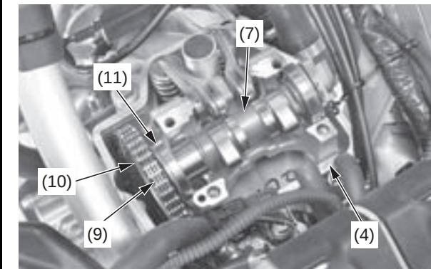
(4) culata (7) árbol de levas (9) cadena de levas (10) rueda dentada de levas (11) cojinete del árbol de levas izquierdo
