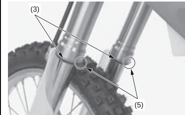
(3) anillos de desgaste (5) huelgos del extremo
