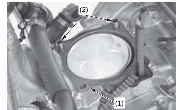
(1) empaquetadura del cilindro (2) pasadores cónicos
