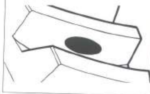
③ FALSCH (Kontakt an Zahnfuß)
