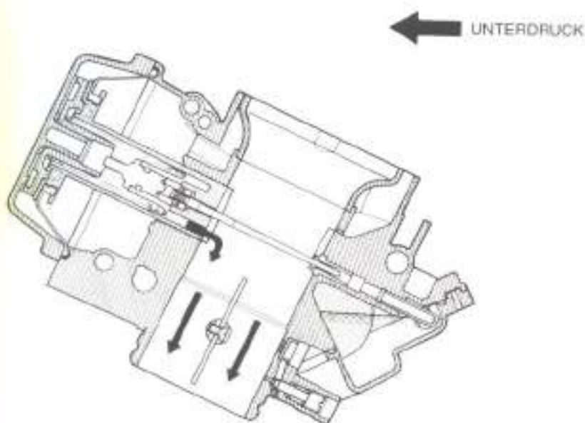
OBERE POSITION DES KOLBENSCHIEBERS
