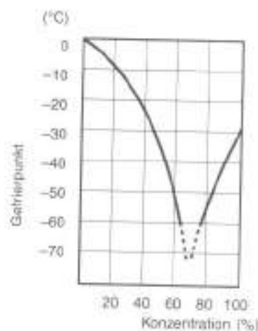
Abb. 1 Kühlmittel-Dichte/Gefrierpunktkurve.
