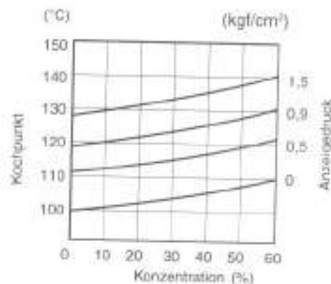
Abb. 2 Kühlmittel-Konzentration/Kochpunktkurve.
