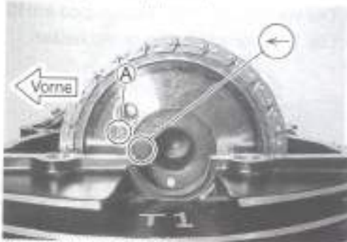
Vorderer Zylinderkopf (Nr. 2)
