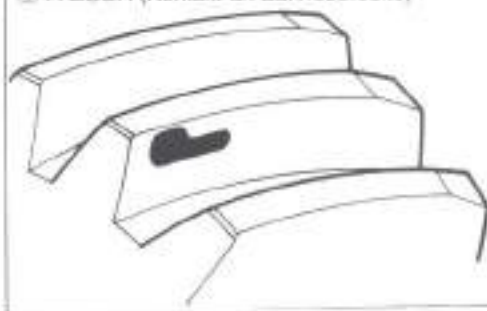
① FALSCH (Kontakt an Zahnoberseite)
