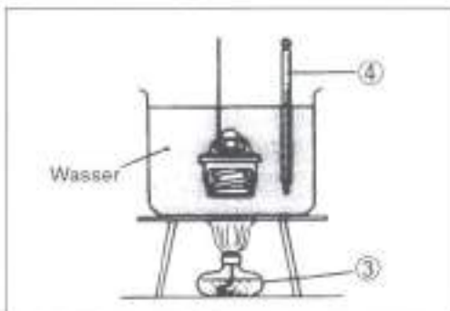
③ Heizgerät ④ Thermometer
