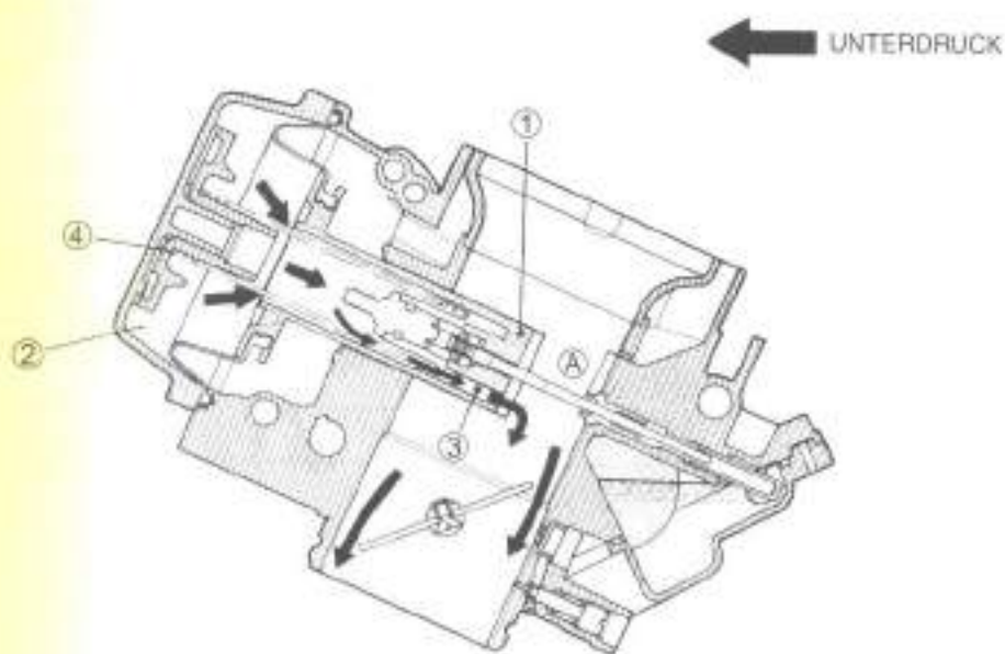
UNTERE POSITION DES KOLBENSCHIEBERS
