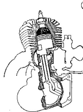
Abb. 5. Arbeitsschema des DKW-Zweitaktmotors mit Umkehrspülung.
