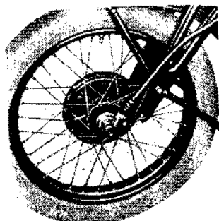
Abb. 42. Demontage des Vorderrades u. Tachometerantriebes: Man löst die beiden Achsmuttern und öffnet die eine Kabelscheide vorsichtig etwas m. dem Schlüssel. Um den Tachometerantrieb zu lösen, braucht man nur den Sperrknopf einzudrücken und kann dann das Kabel herausziehen. Bei Wiedereinsetzen ist darauf zu achten, daß die Kabelführungszunge richtig in die Antriebsführung eingesetzt wird.
