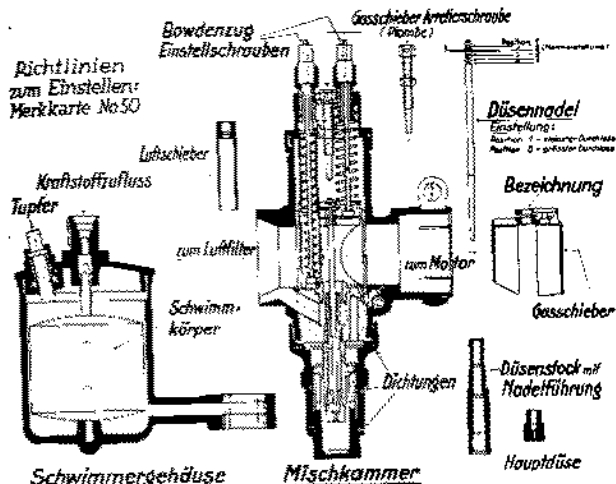
Abb. 23. Amal-Vergaser: Am Vergaser rechts seitlich liegt die Luftregulierungsschraube, etwas darüber die Gasschieberanschlagschraube. Die Handhabung ist auf Seite 27 genau erklärt.
