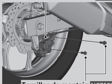
Tornillos de montaje NC750XD
