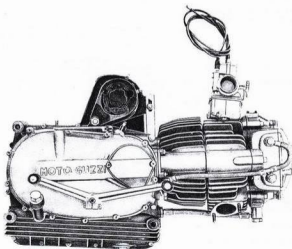
Abb. 5 - Antriebsseite
