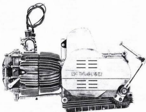
Abb. 4 - Schwungradseite
