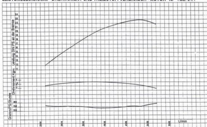
LEISTUNGSDIAGRAMM - DREHMOMENT UND TREIBSTOFFVERBRAUCH - MOTOR "NF" Abb. 81/1
