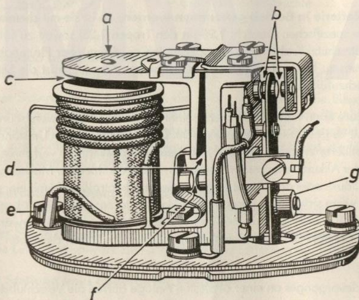
Spannungs-Regler der Lichtmaschine
