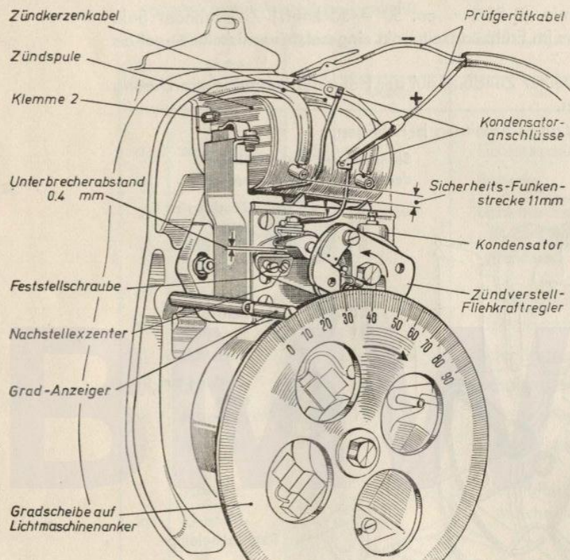
Zündungseinstellung an Zündmagnet R 51/3, R 67 und R 67/2 mit Einstellvorrichtung V 5029
