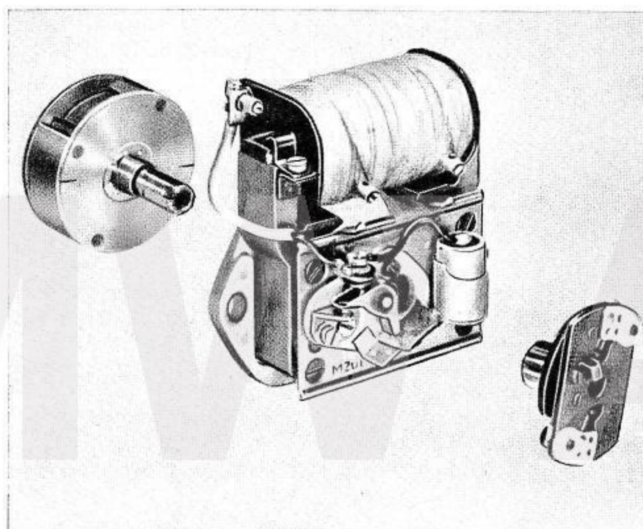
Bild - Fig. 200: Magnetzündler - Magnéto d'allumage - Ignition magneto - Magneto de encendido
