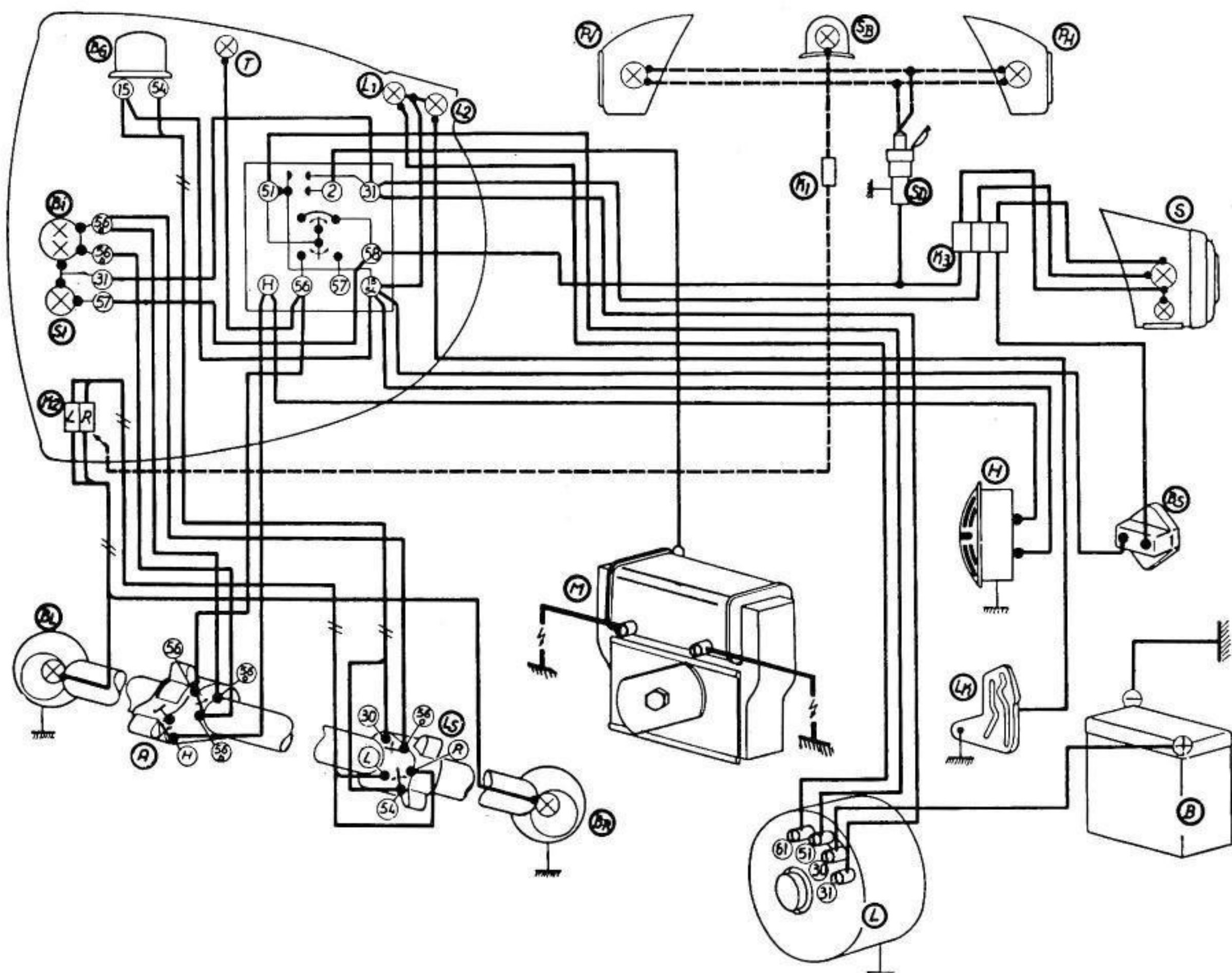
Bild – Fig. 209 Stromlaufplan – Schéma des connections – Wiring Diagram (swivel switch arrangement) – Esquema de conexiones eléctricas
