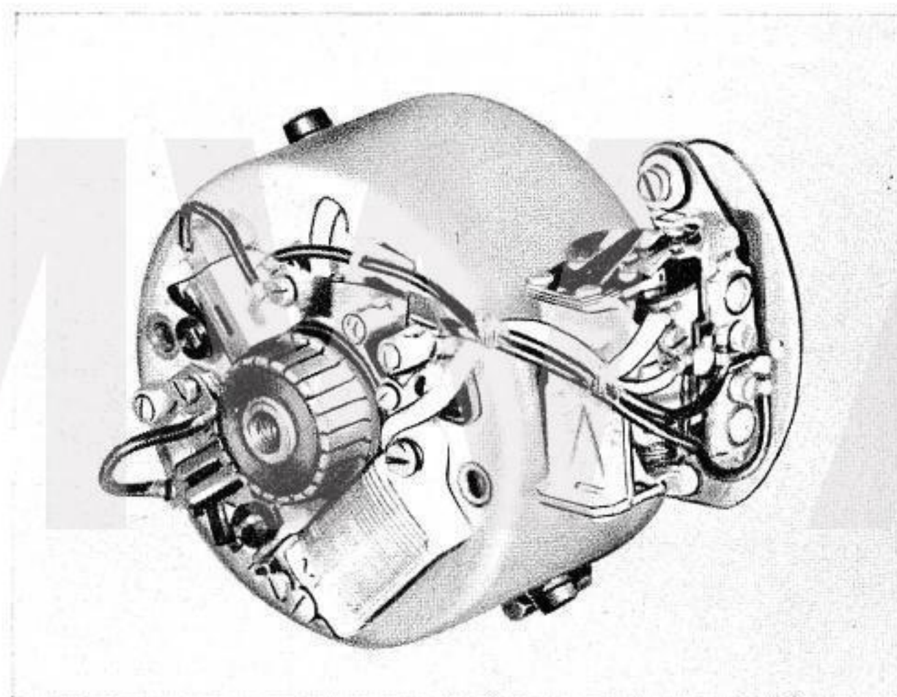
Bild - Fig. 199: Lichtmaschine - Dynamo - Generator - Dinamo
