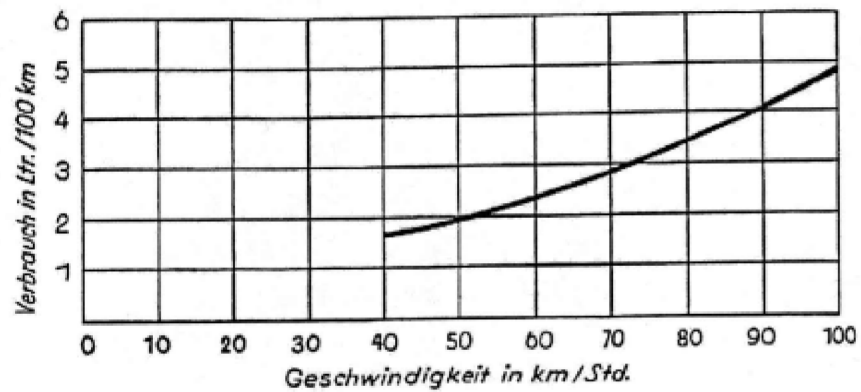
Kraftstoffverbrauchscurve
