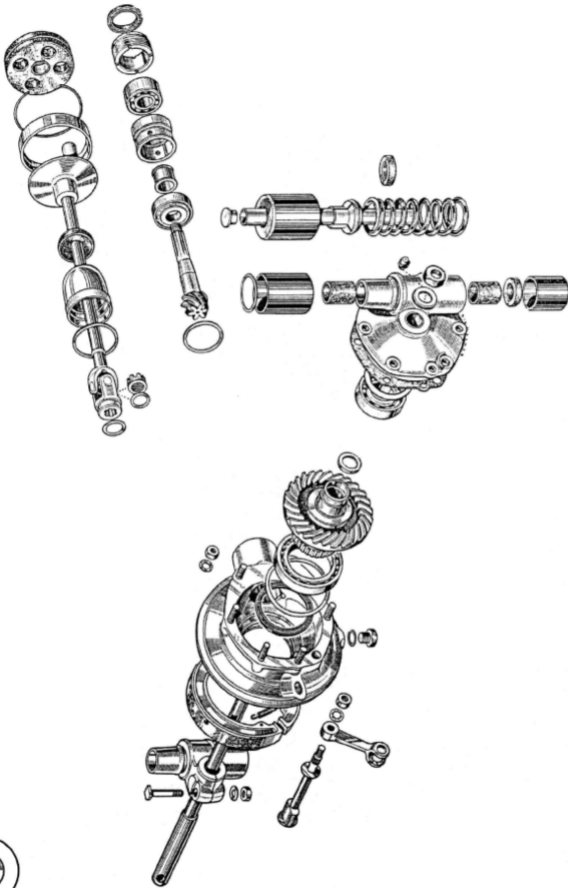
BMW R 25 Kardantrieb und Hinterradfederung.
