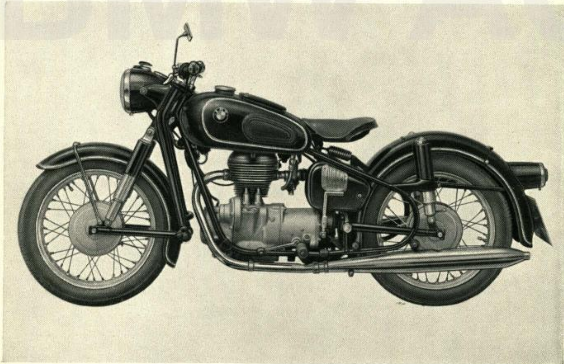
BMW R 27 mit Schwebemotor Ansicht von links
