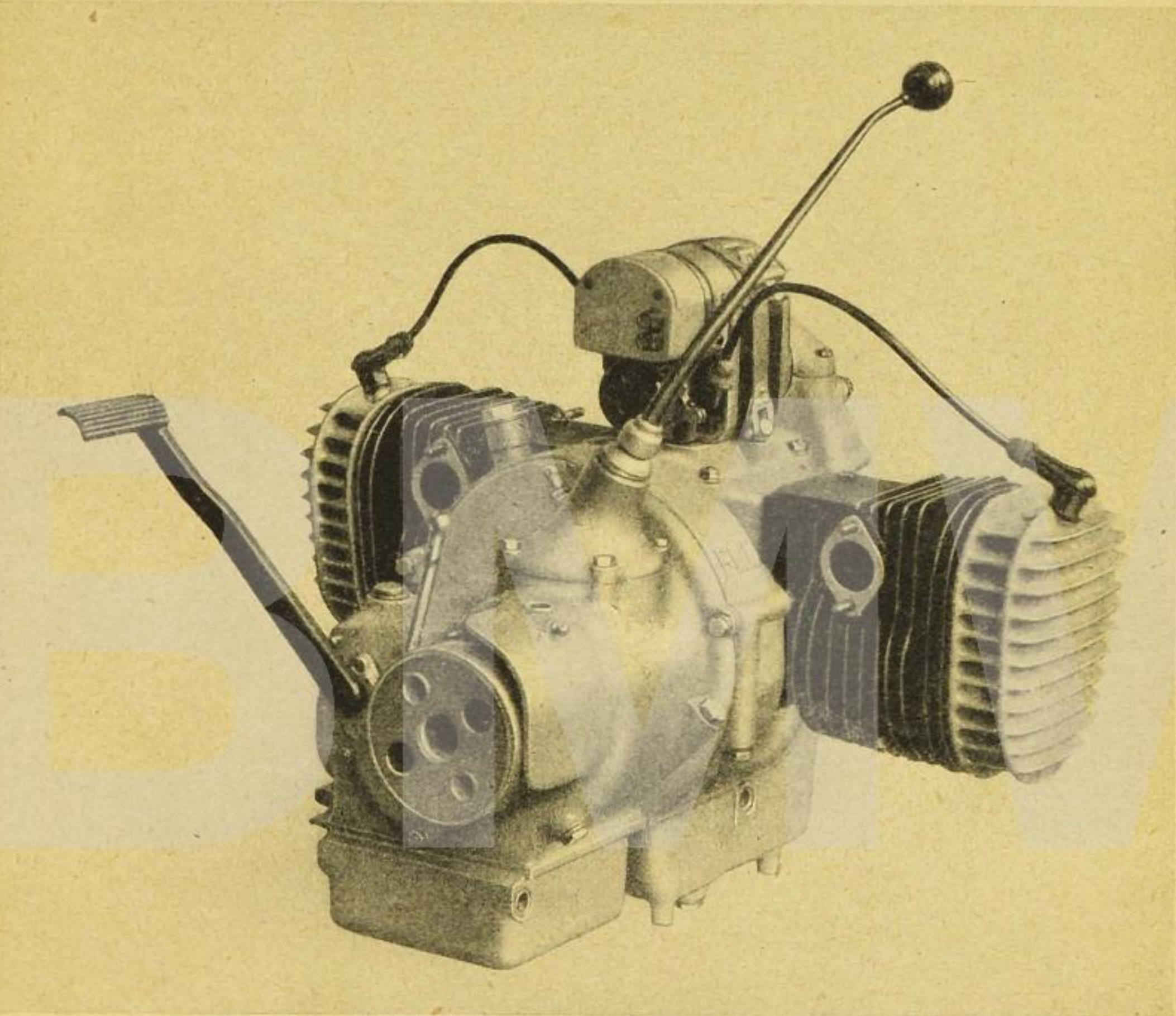
Tafel 1, Gruppe M: Motor und Getriebe
