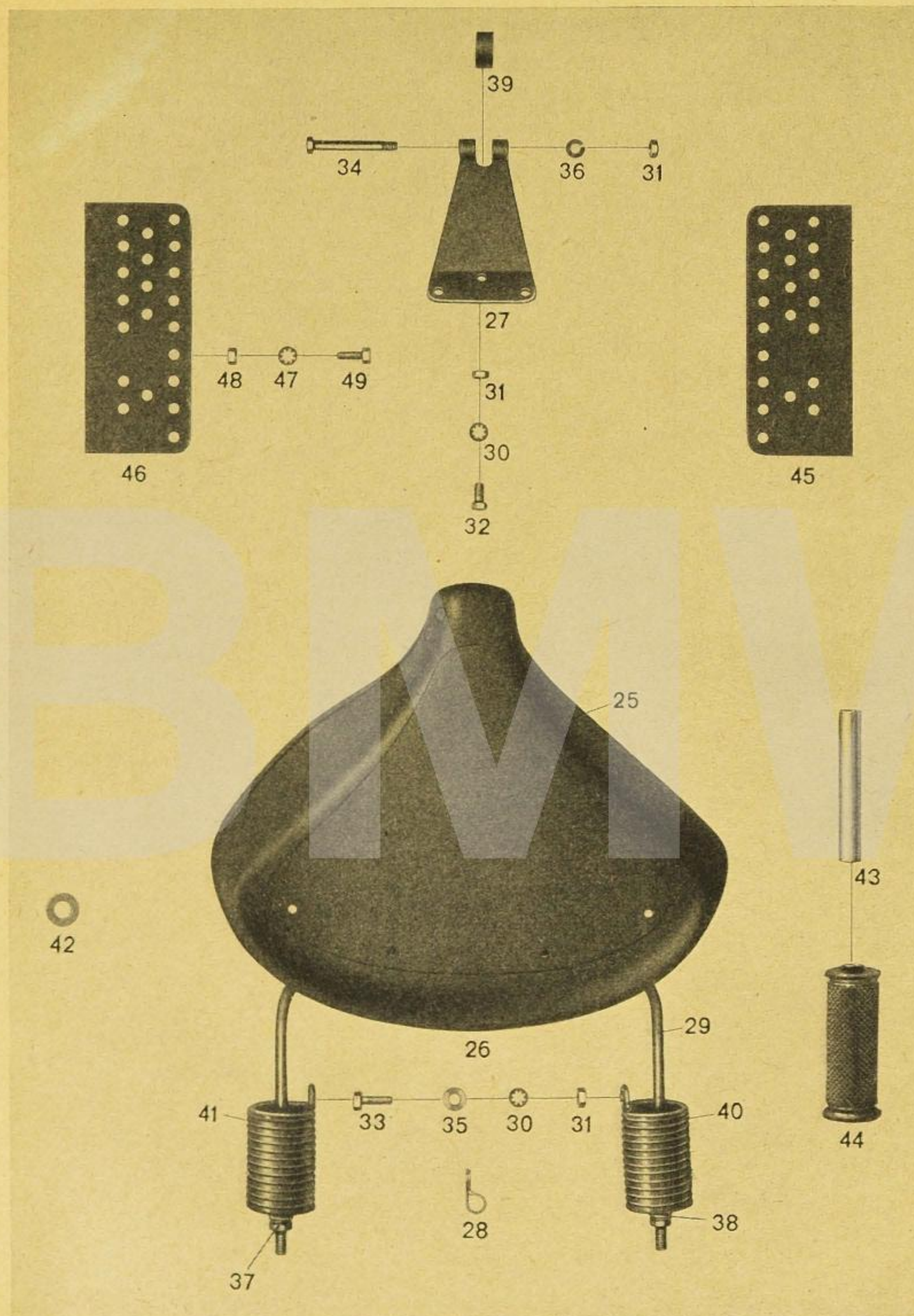
Tafel 13, Gruppe R: Sattel, Fußrasten
