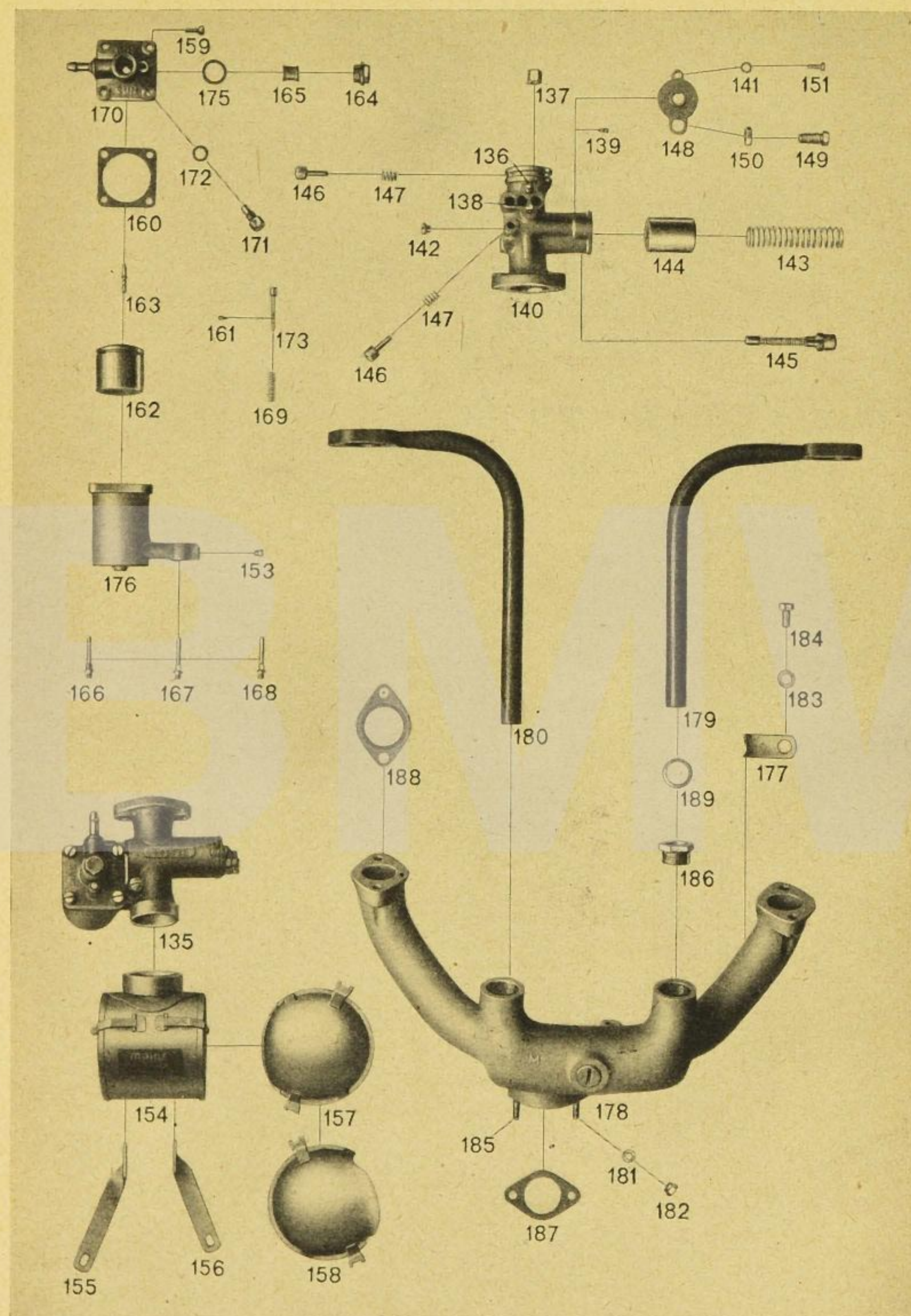
Tafel 7, Gruppe M: a) Motor, Vergaser mit Saugleitungen
