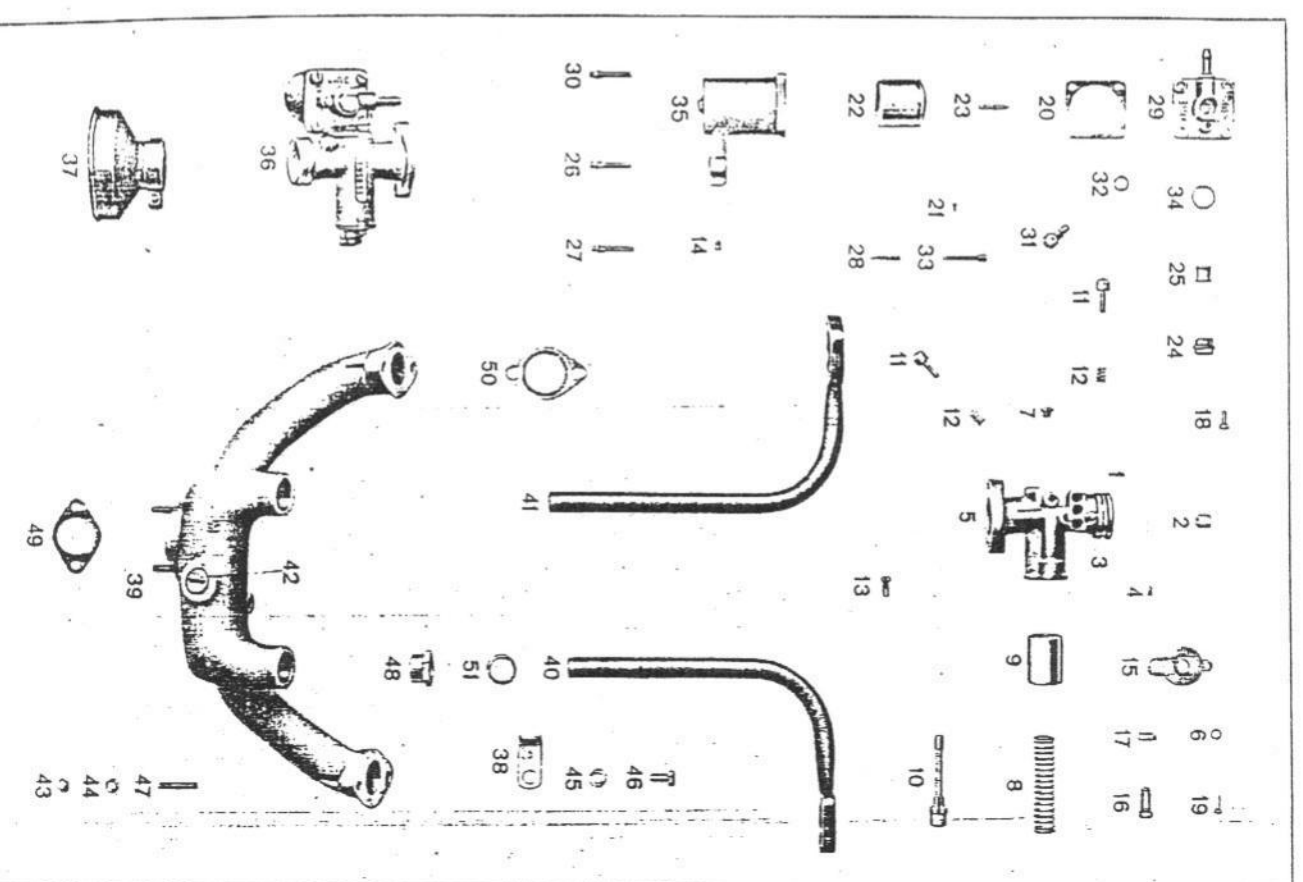
Tafel 20 Sum-Vergaser (Einvergaser-Maschine)
