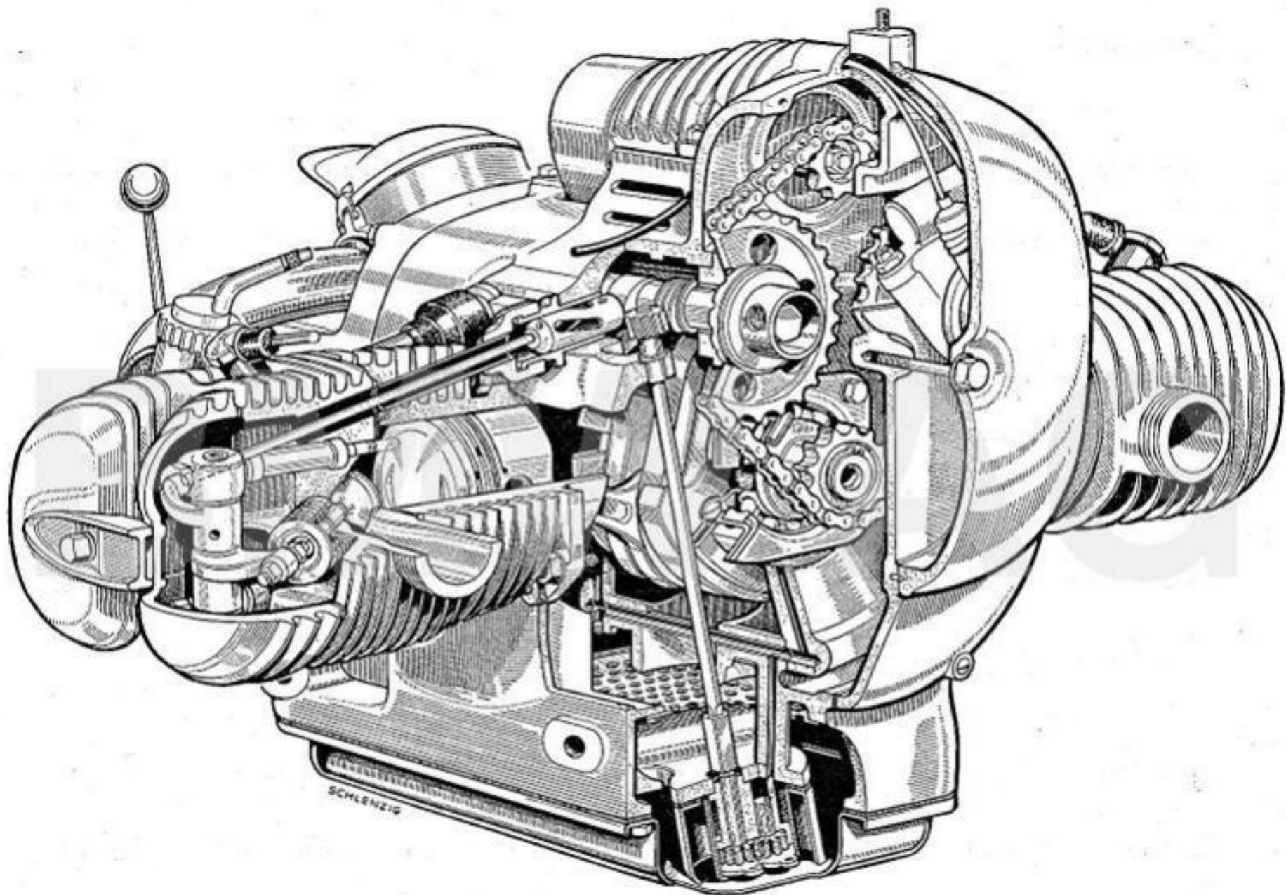
Schnitt durch den BMW Motor R 51/2
