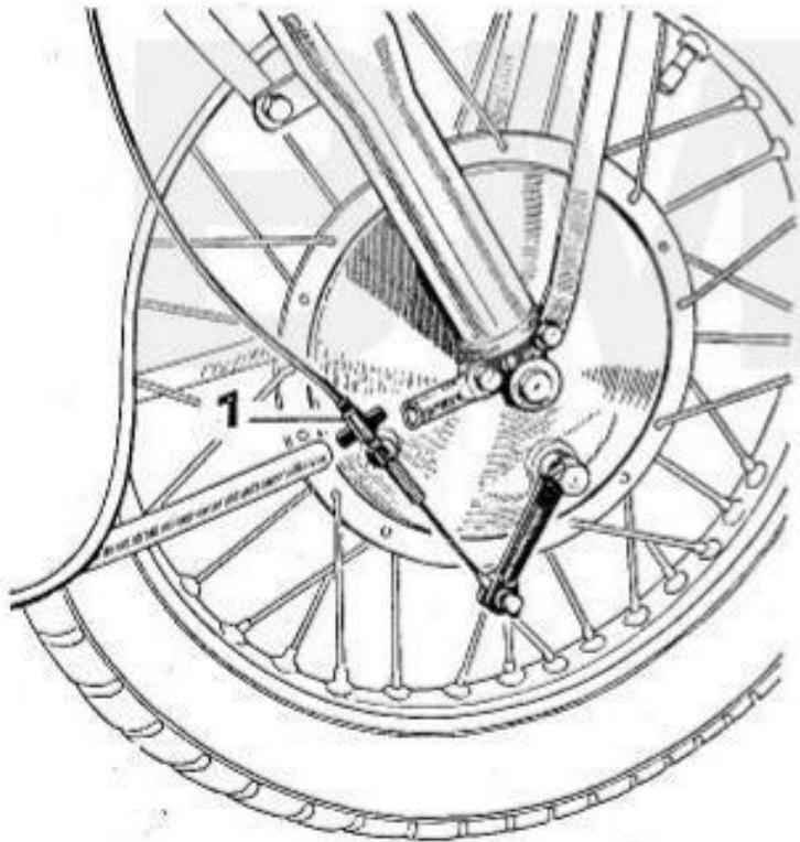
Nachstellen der Vorderradbremse
