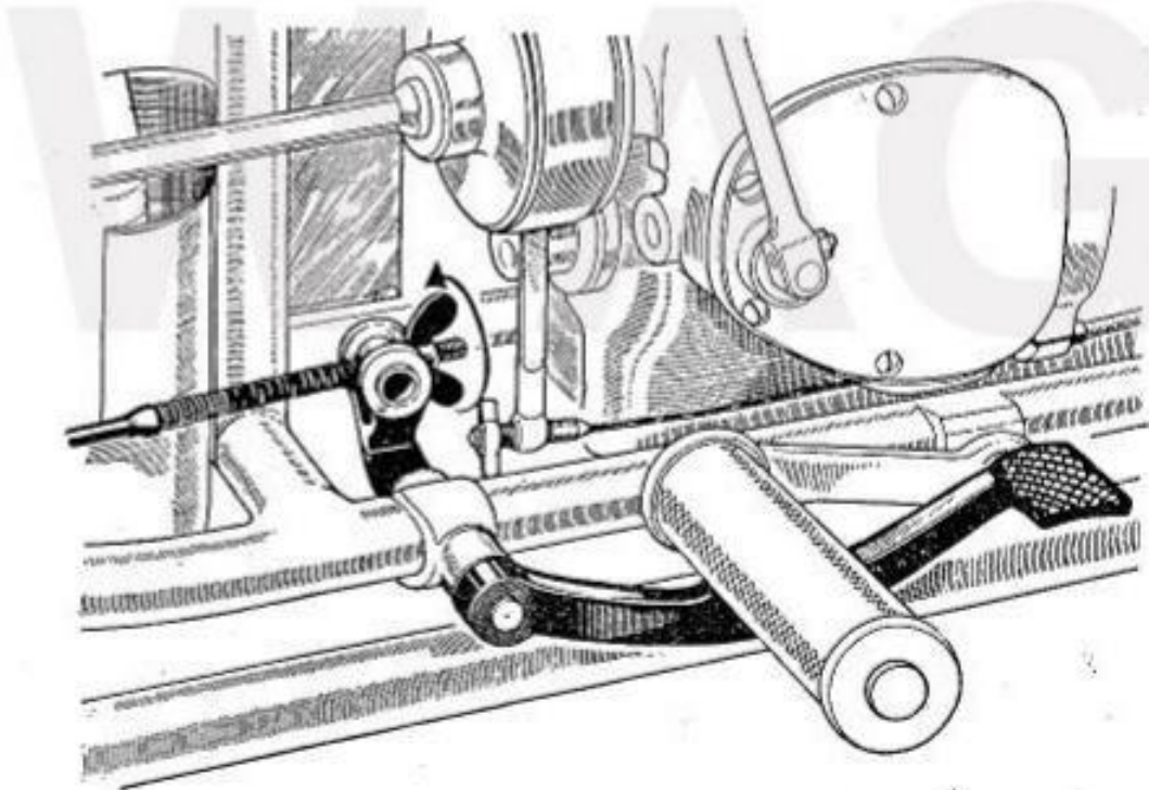
Nachstellen der Hinterradbremse
