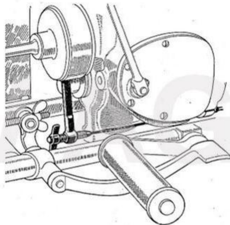
Kupplungs-Nachstellung
