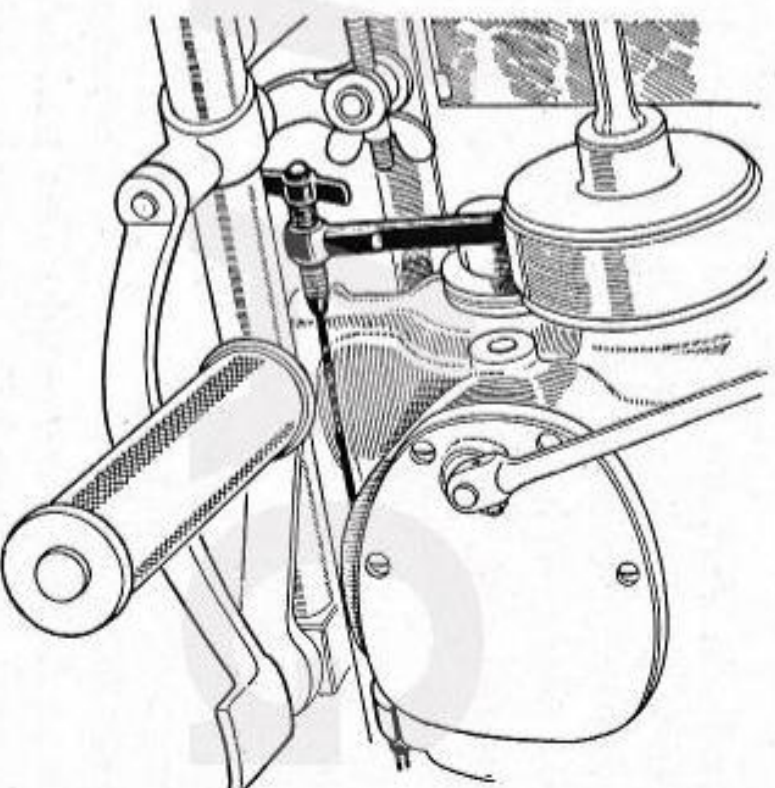
Kupplungs-Nachstellung
