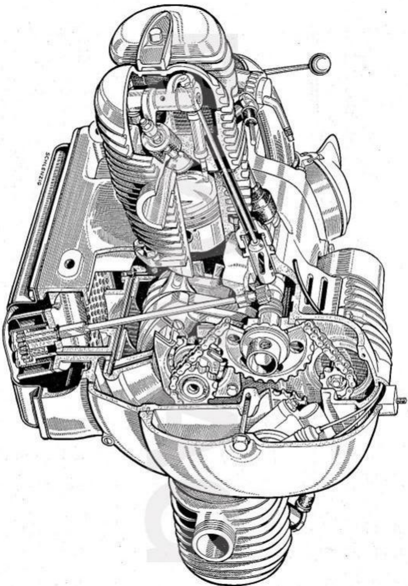
Schnitt durch den BMW Motor R 51/2
