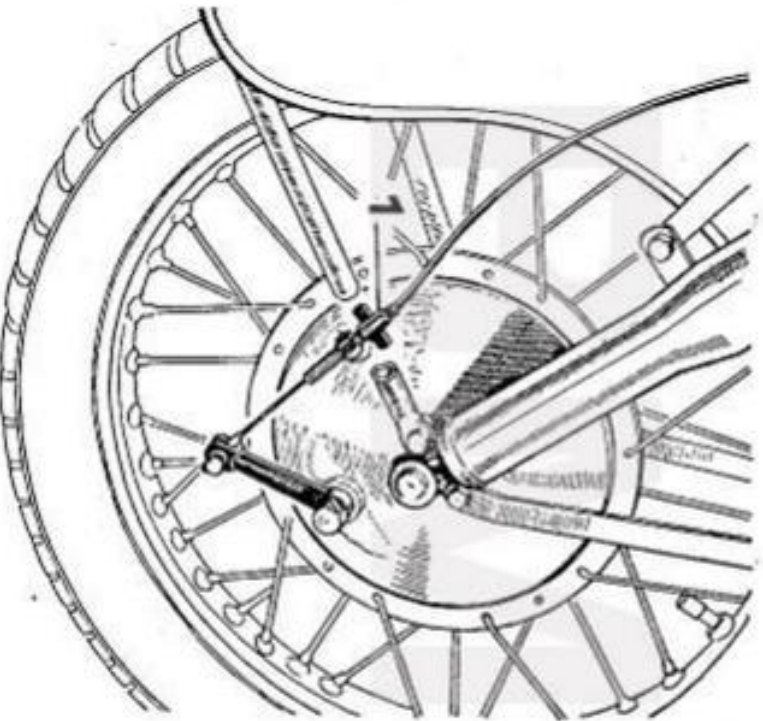
Nachstellen der Vorderradbremse
