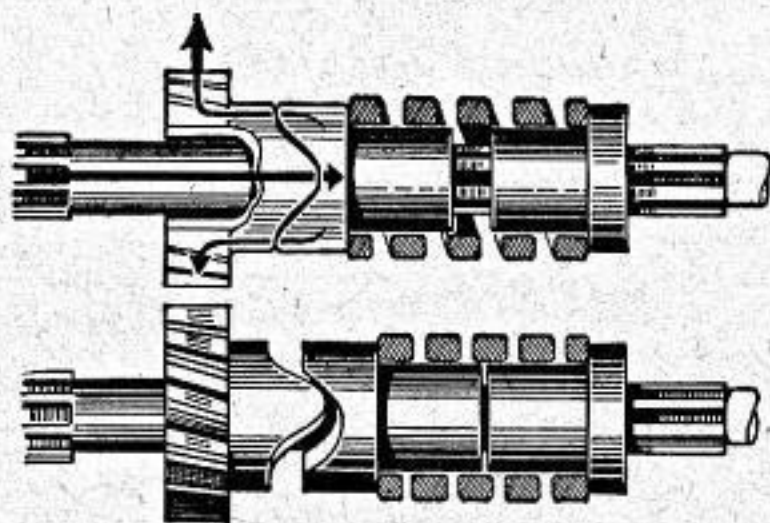
Schema der federnden Hauptwelle im Getriebe
