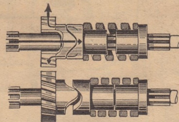
Schema der federnden Hauptwelle im Getriebe
