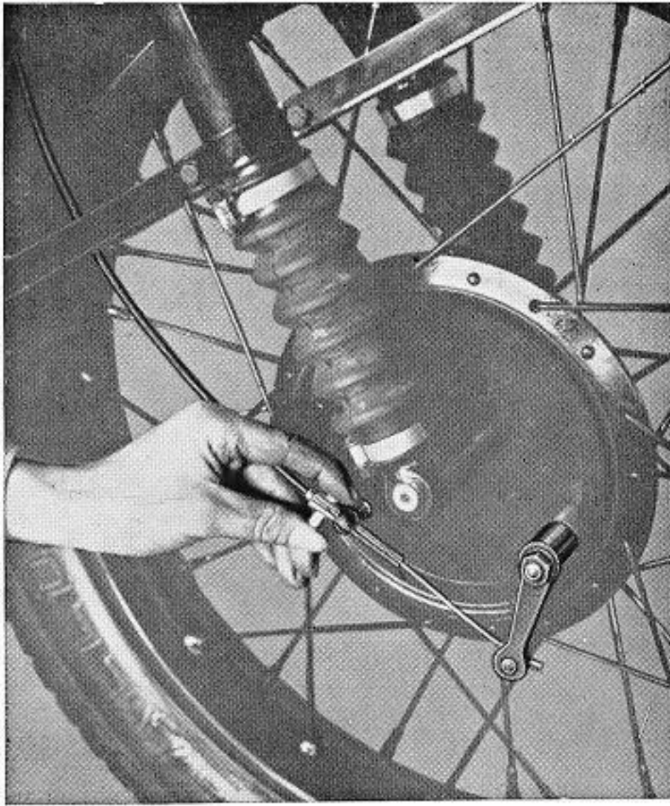
Bild 12. Nachstellen der Vorderradbremse
