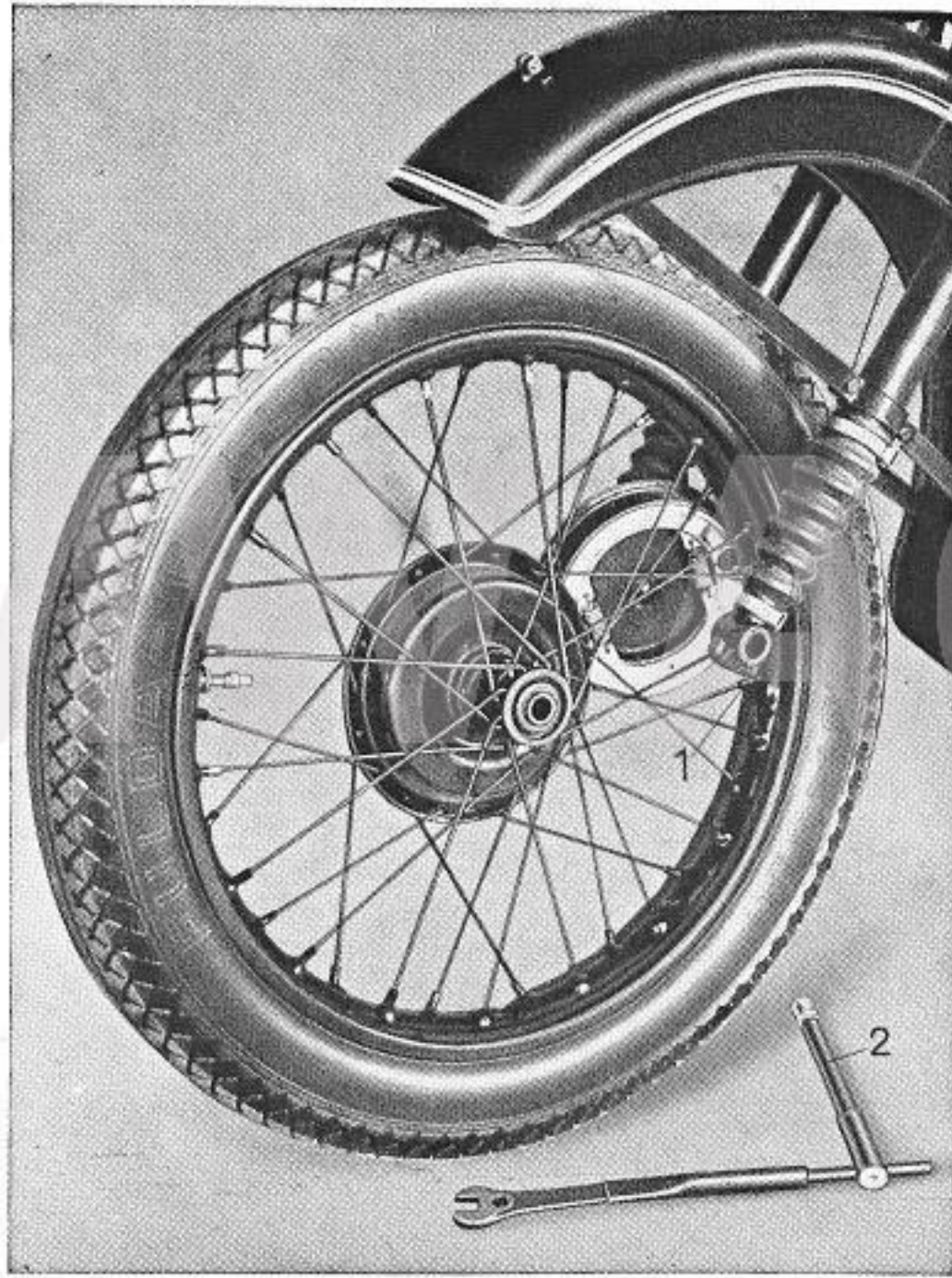
Bild 5. Ausbau des Vorderrades
