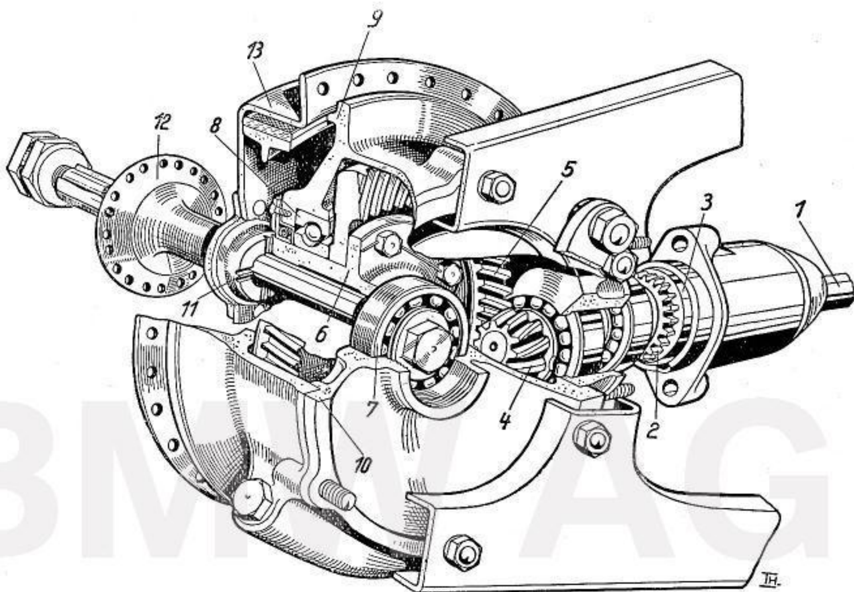
Bild 15. Hinterradantrieb
