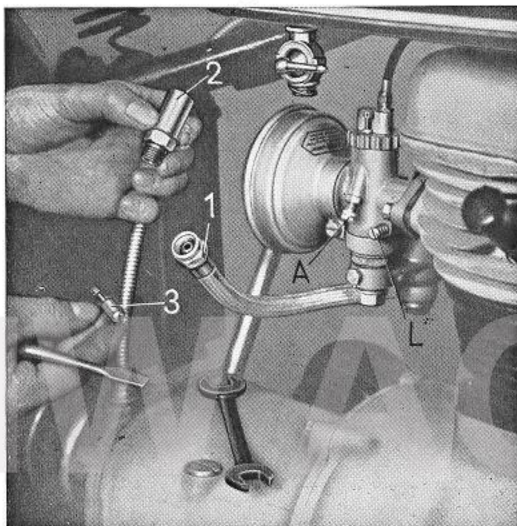
Bild 7. Reinigen des Kraftstoffhahnes
