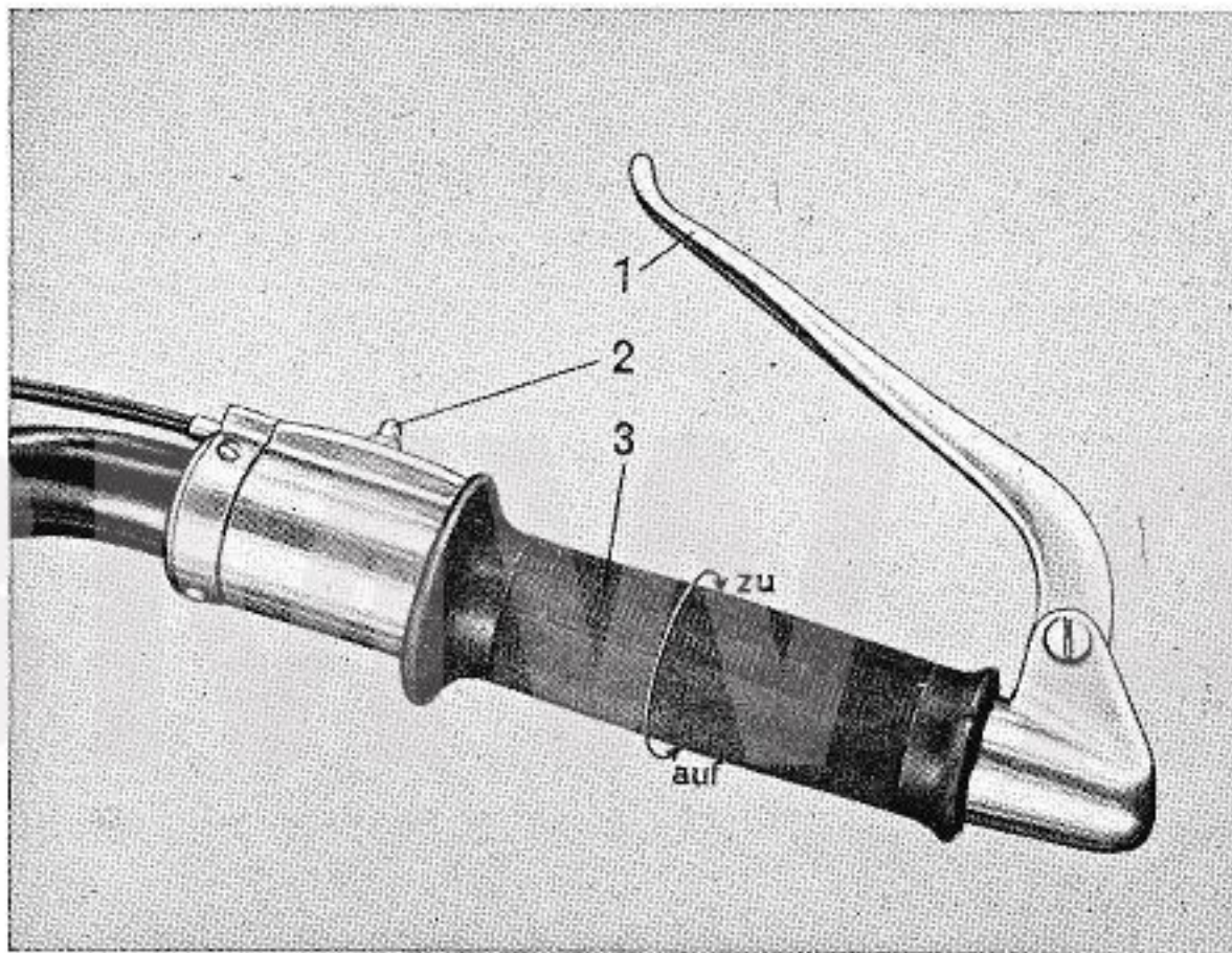
Bild 4. Rechtes Lenkerende
