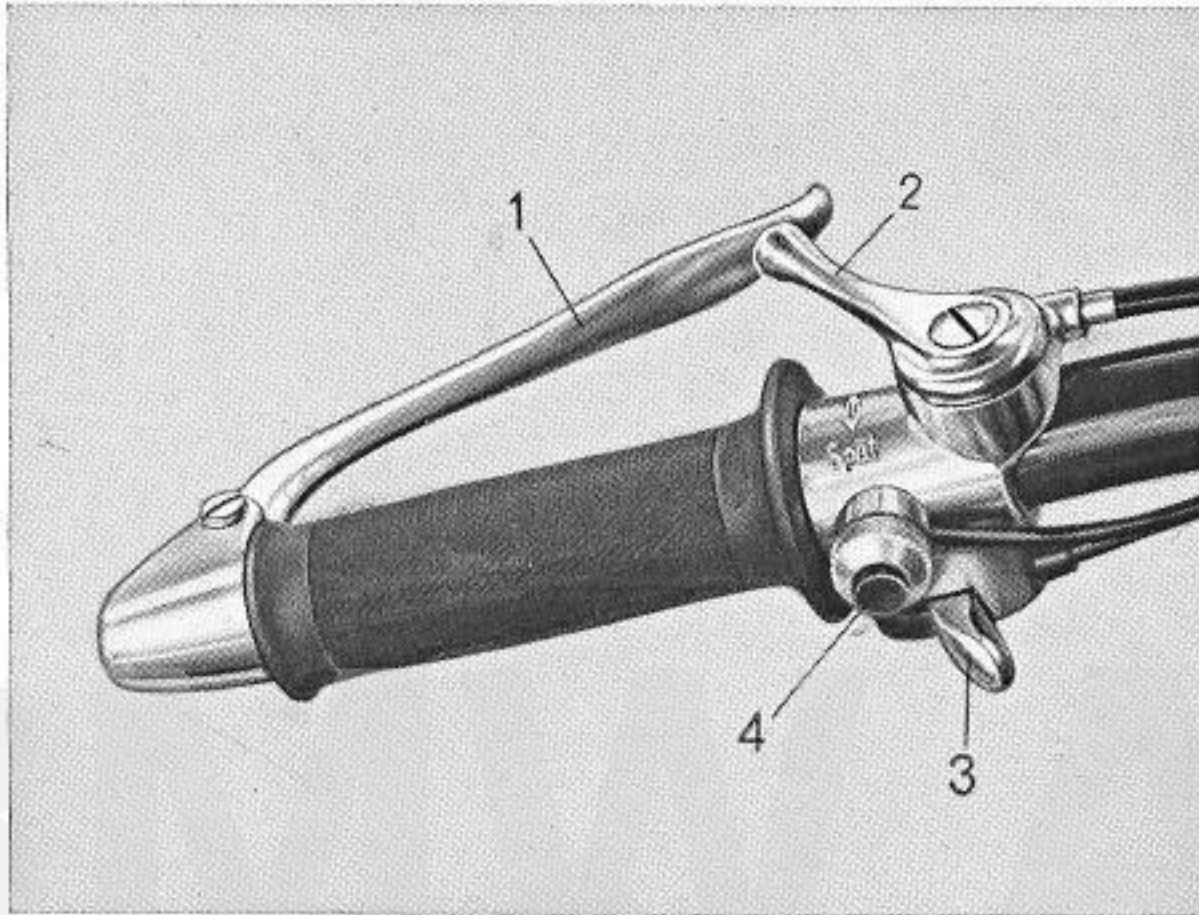
Bild 2. Linkes Lenkerende
