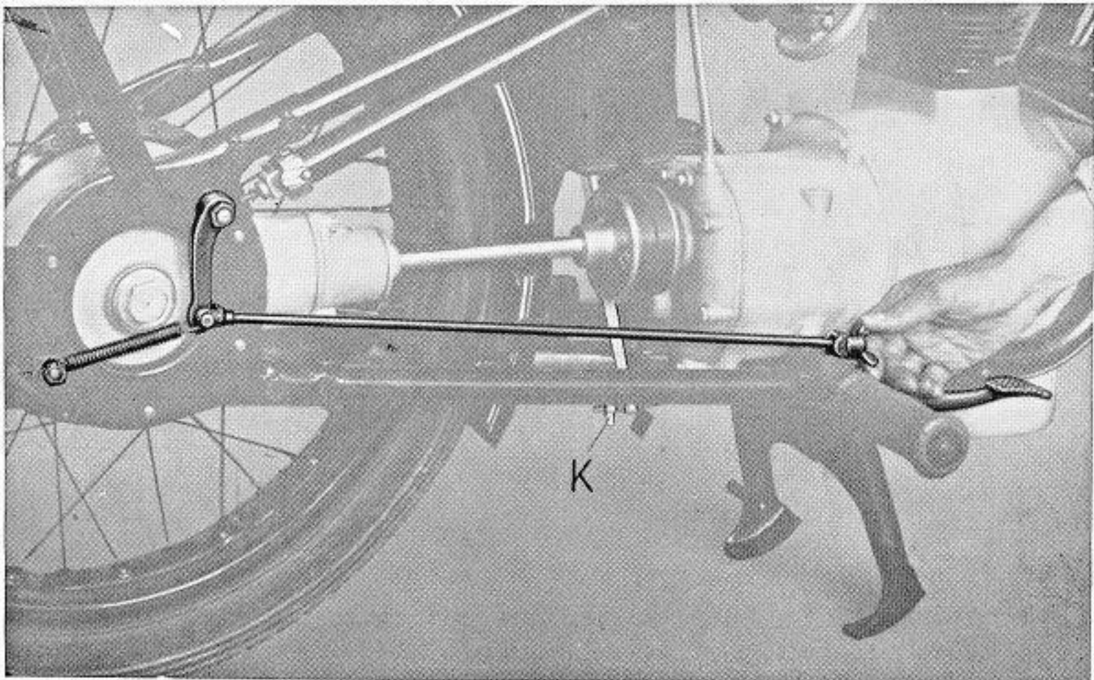
Bild 13. Nachstellen der Hinterradbremse
