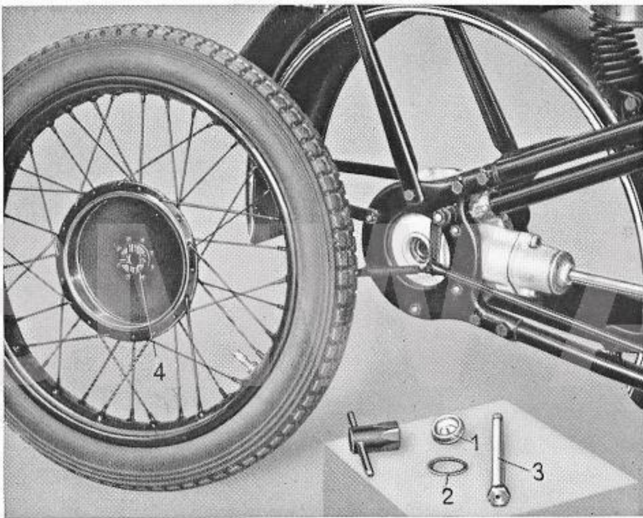
Bild 6. Ausbau des Hinterrades
