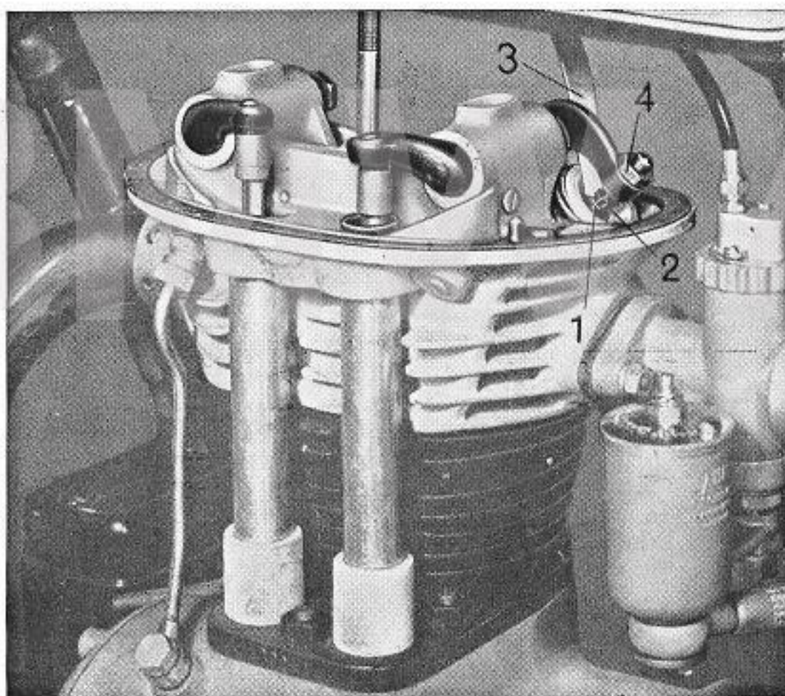
Bild 10. Einstellen des Ventilspieles
