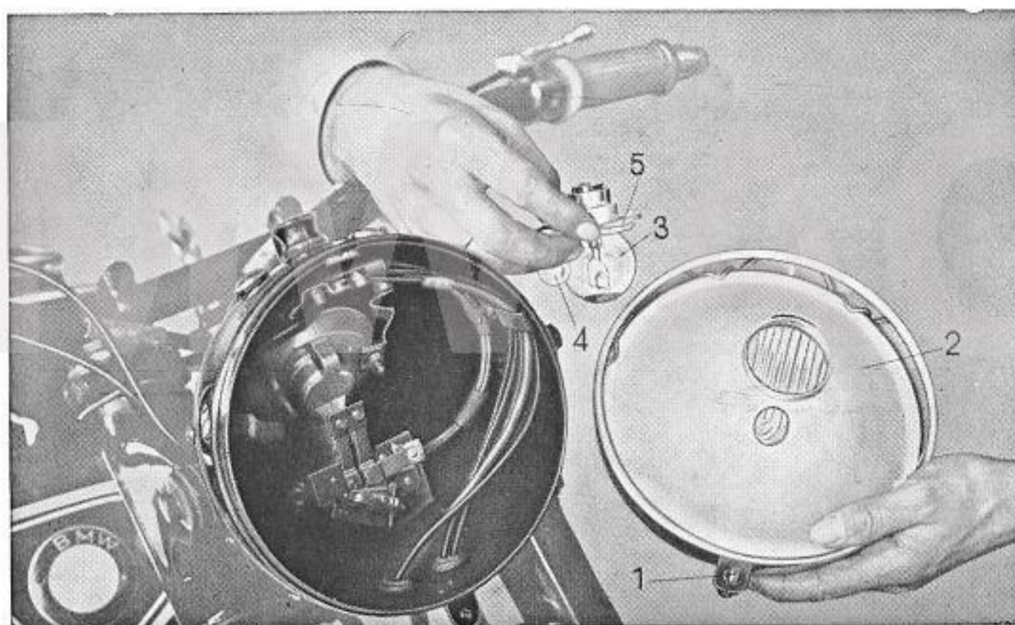
Bild 17. Ausbau der Scheinwerferlampe
