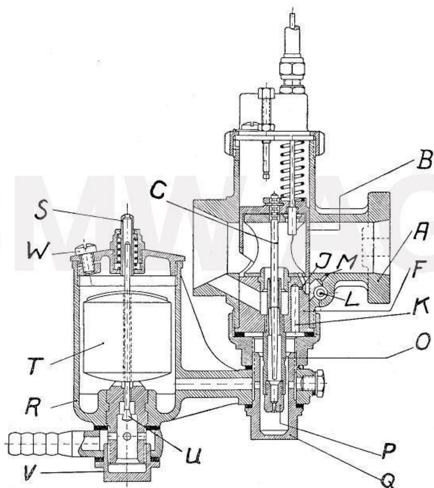
Bild 14. Schnitt durch den Vergaser
