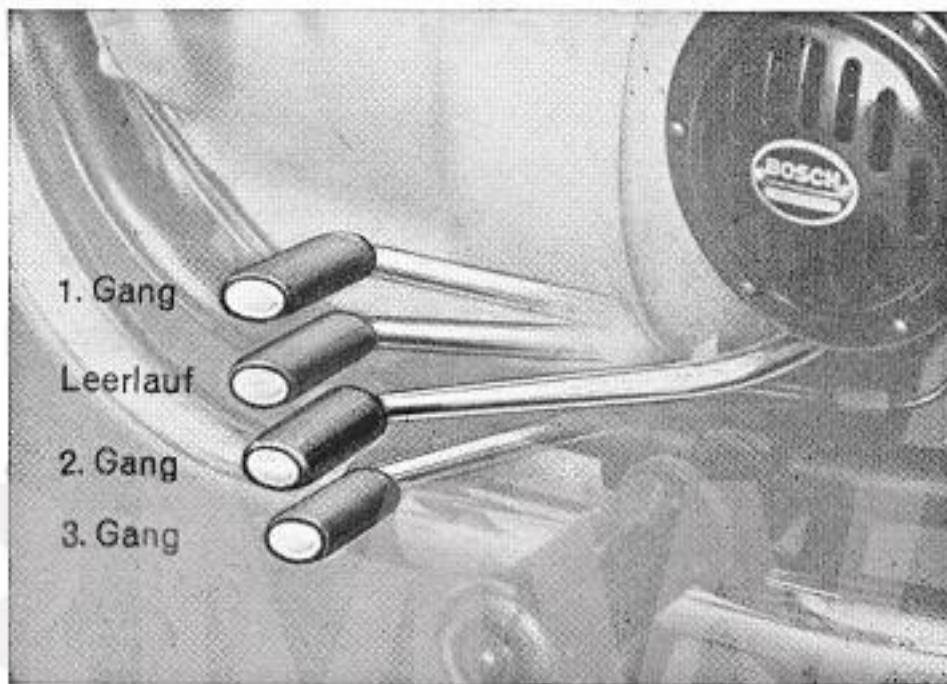
Bild 3. Fußschalthebel
