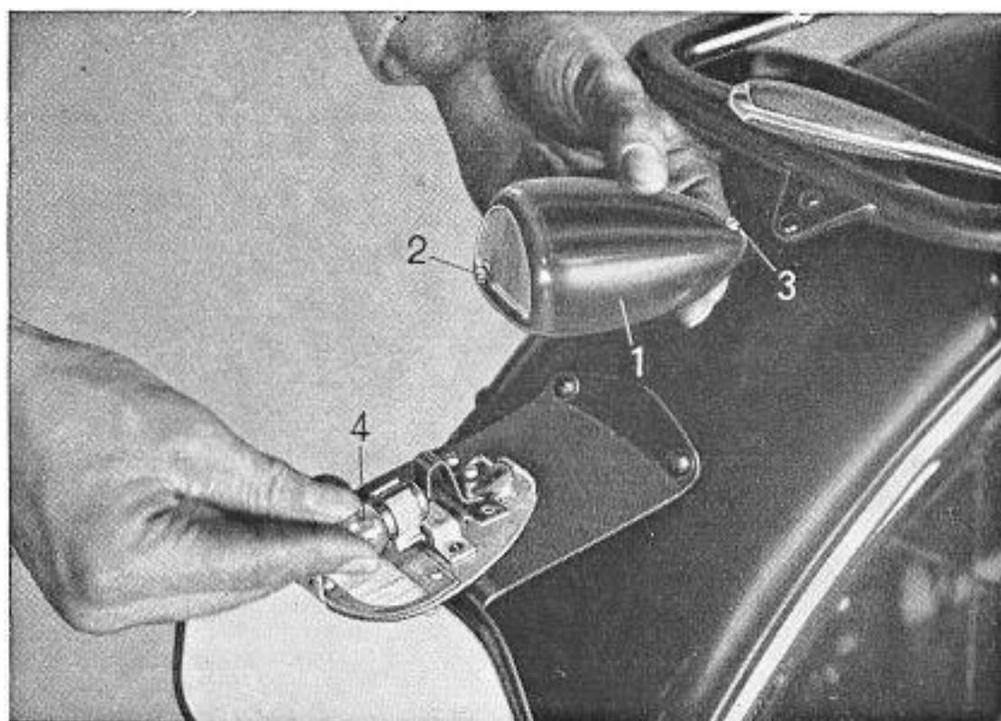
Bild 18. Ausbau der Schlußlichtlampe
