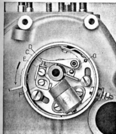
Abb. 13. Unterbrecherkontakte
