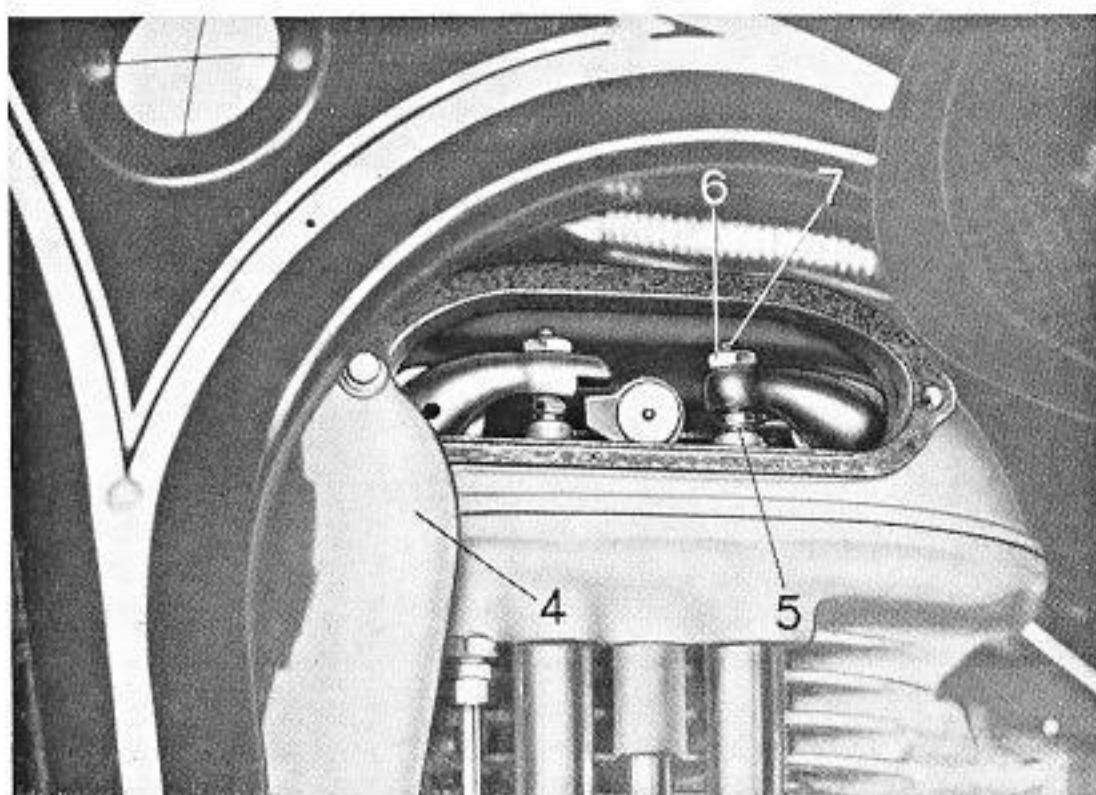
Abb. 16. Kipphebel der R 4-Maschine
