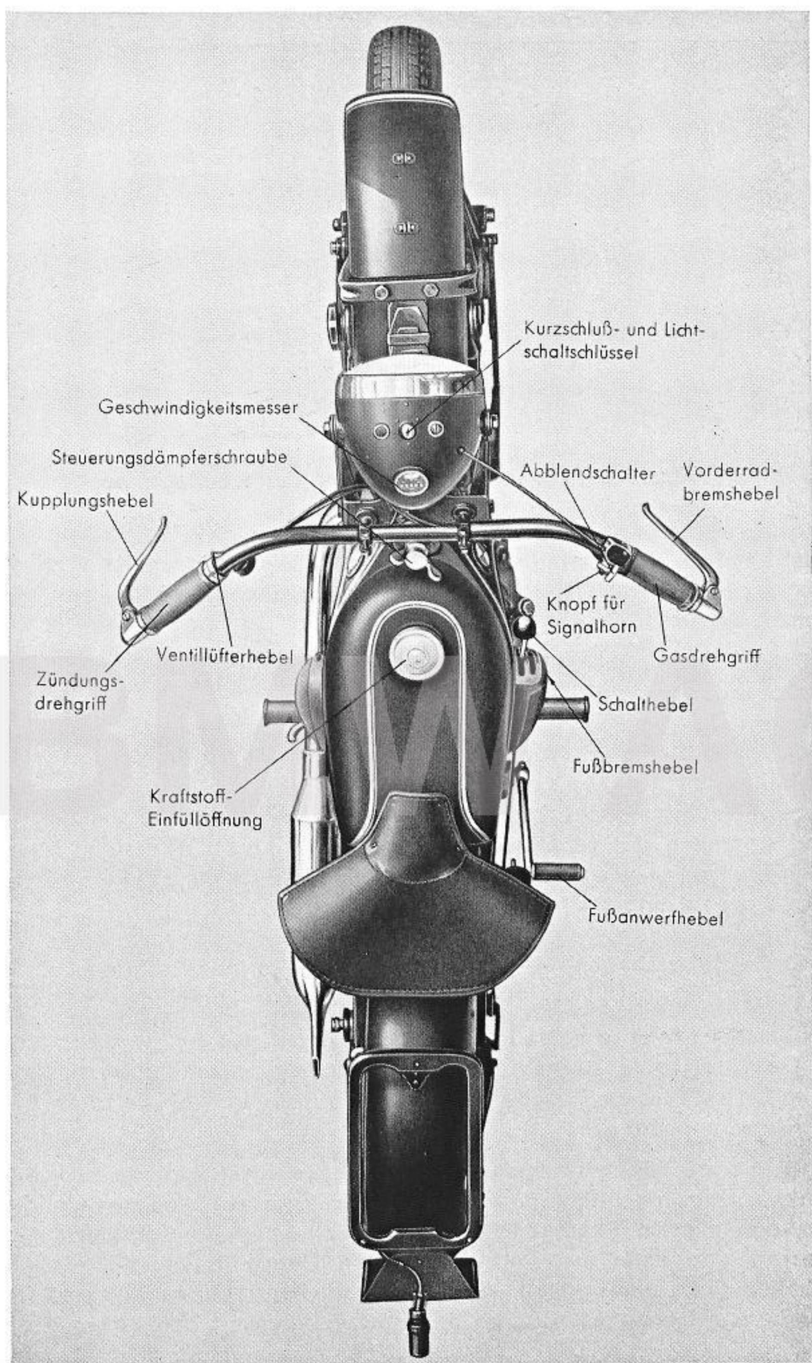
Abb. 6 Die Bedienungshebel der R 4-Maschine
