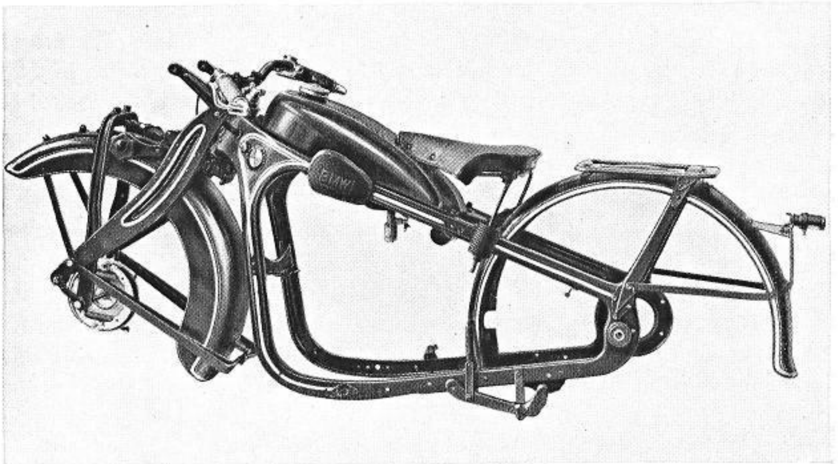
Abb. 30. Rahmen der R 4-Maschine
