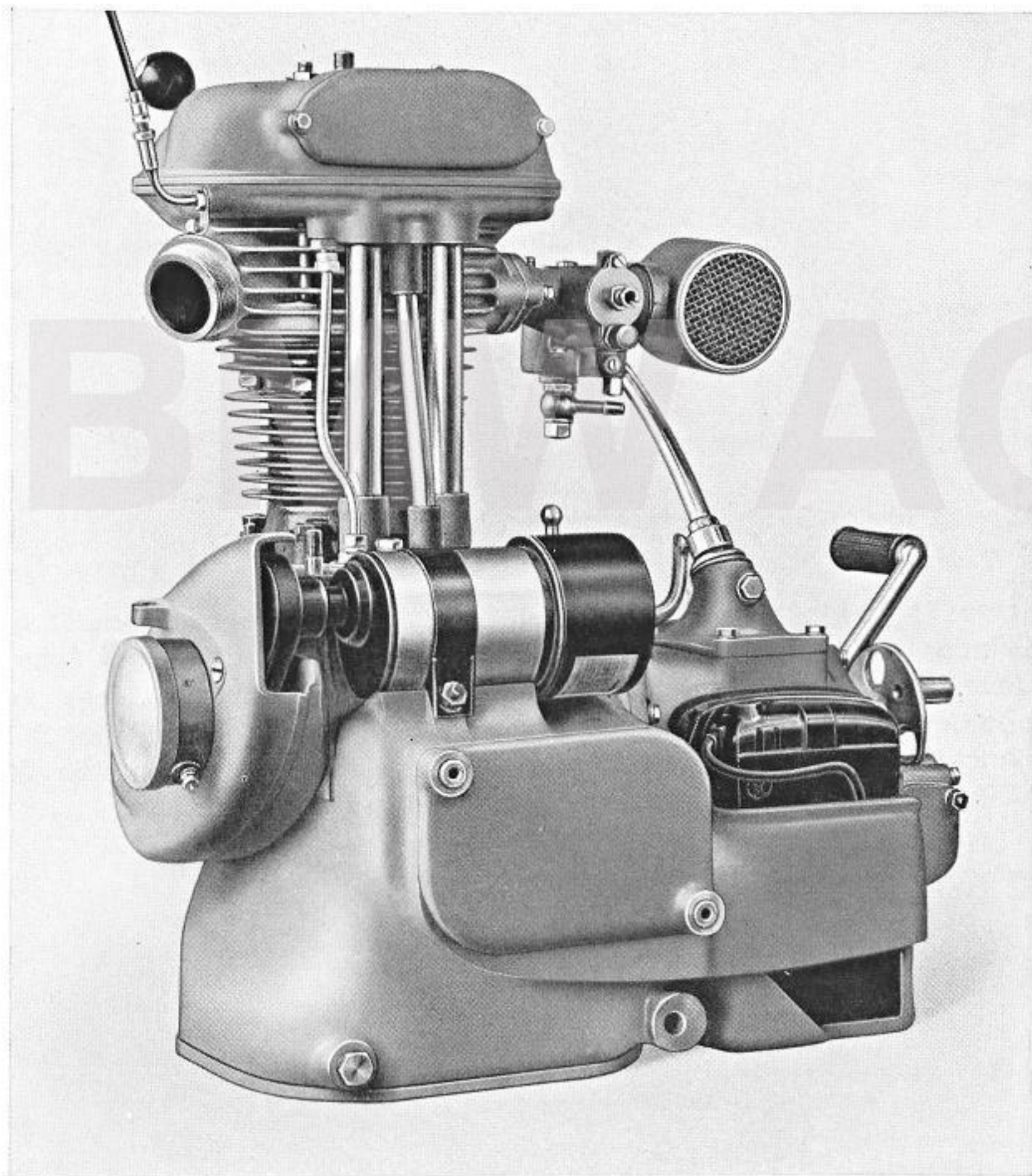
Abb. 17. Motor-Getriebeblock der R 4-Maschine
