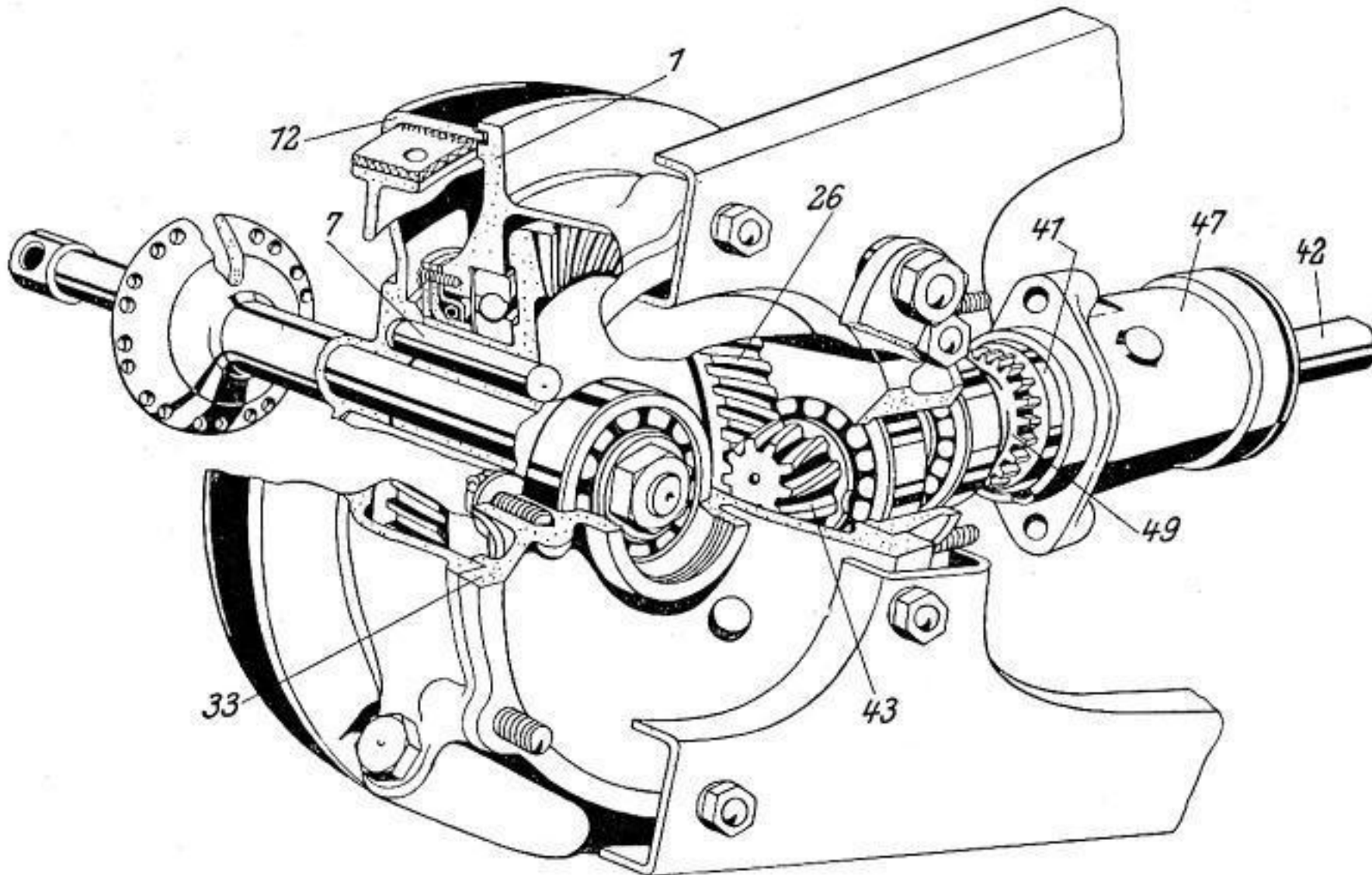
Abb. 29. Kraftübertragung im Kardangehäuse
