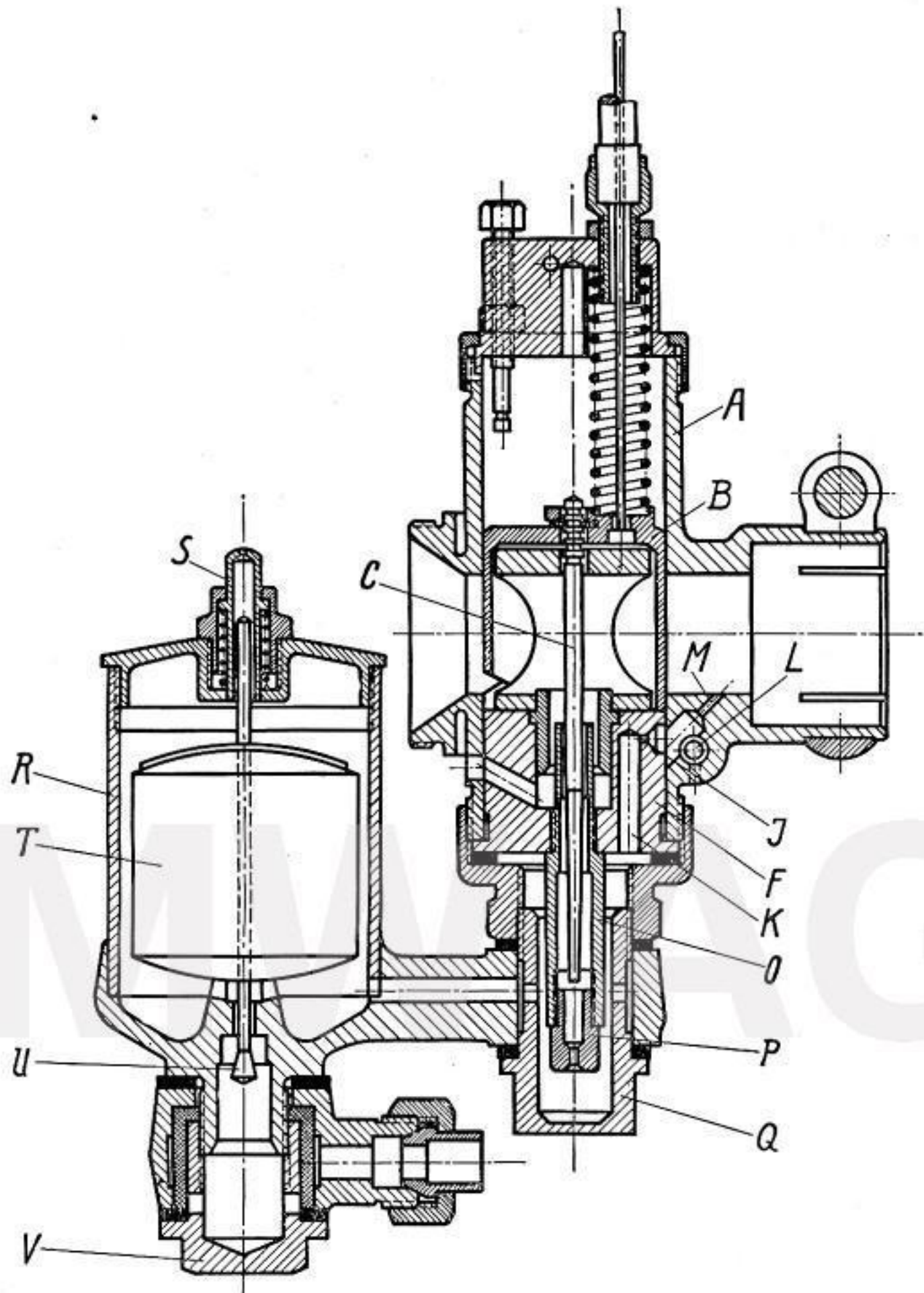
Abb. 23. Vergaser der R 2-Maschine
