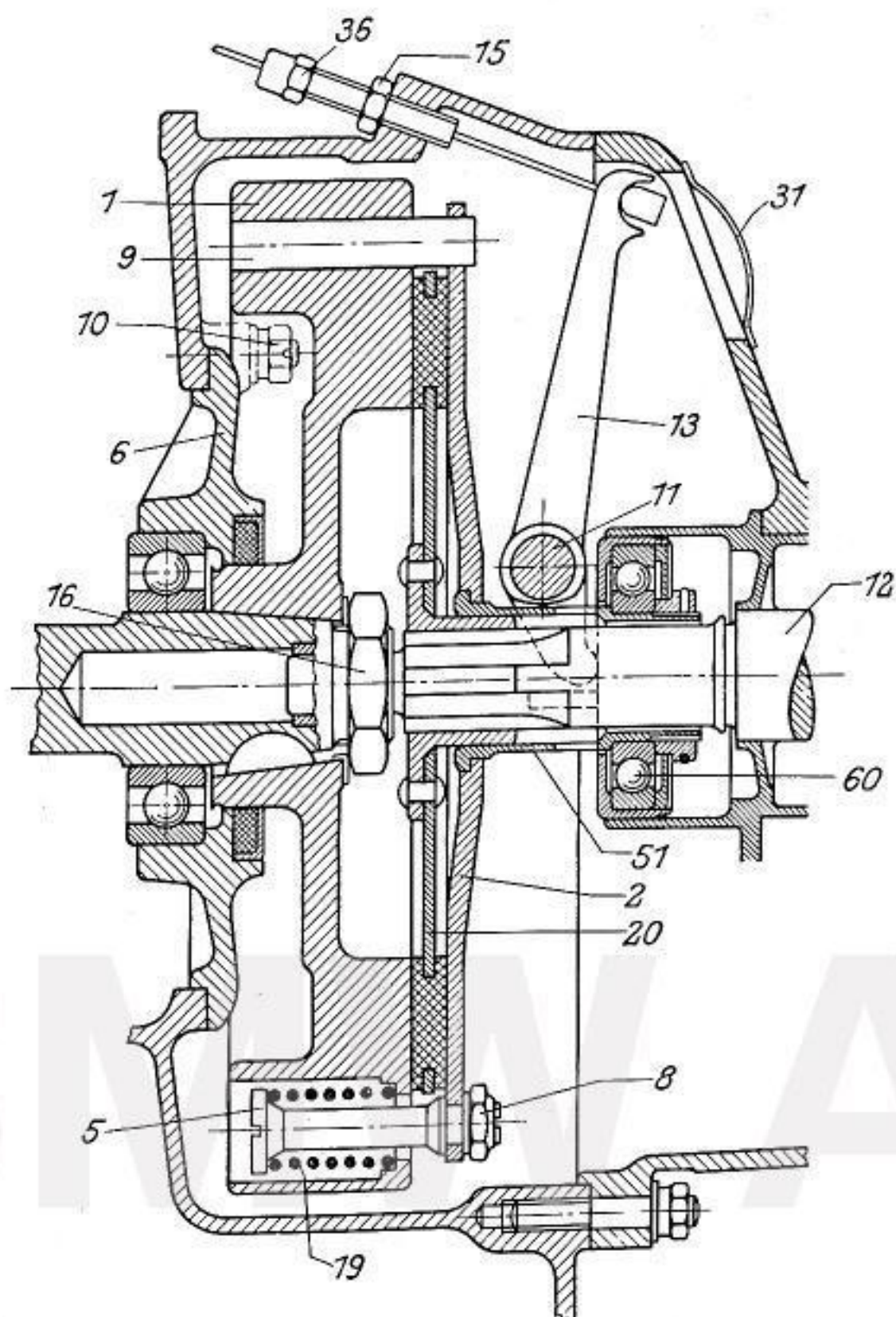
Abb. 25. Kupplung der R 2-Maschine
