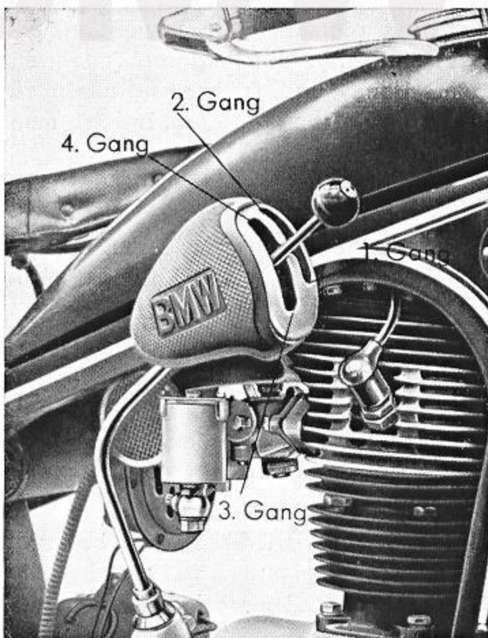
Abb. 9 Schalthebelstellungen bei der R 4-Maschine
