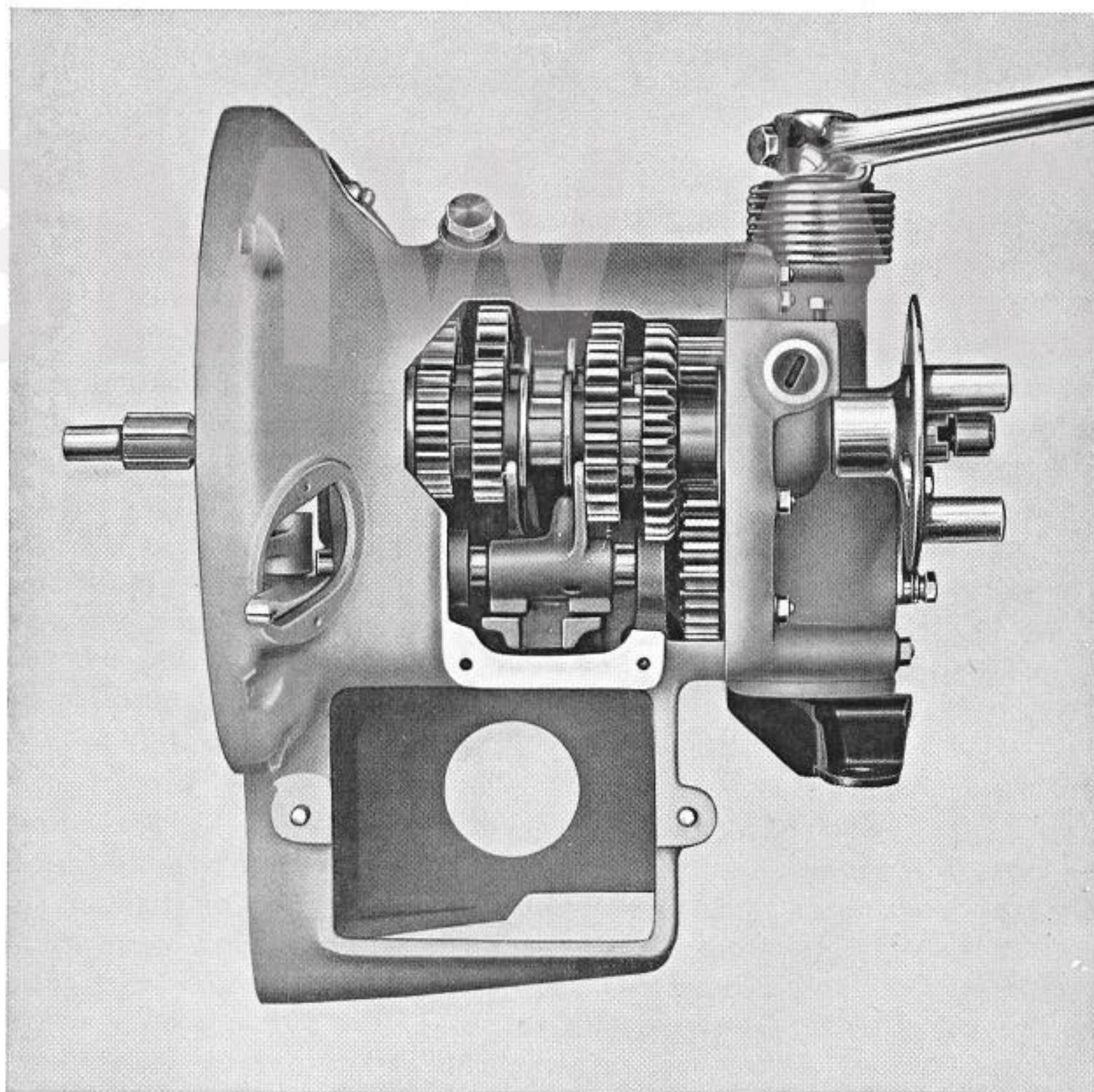
Abb. 28. Getriebe der R 4-Maschine
