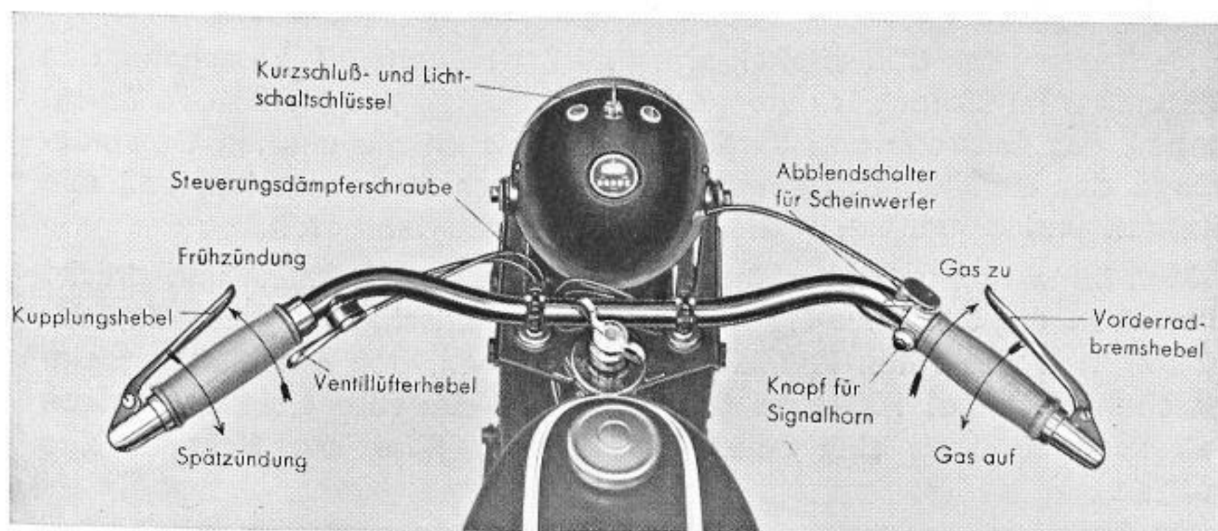
Abb. 8 Lenker und Scheinwerfer der R 4-Maschine
