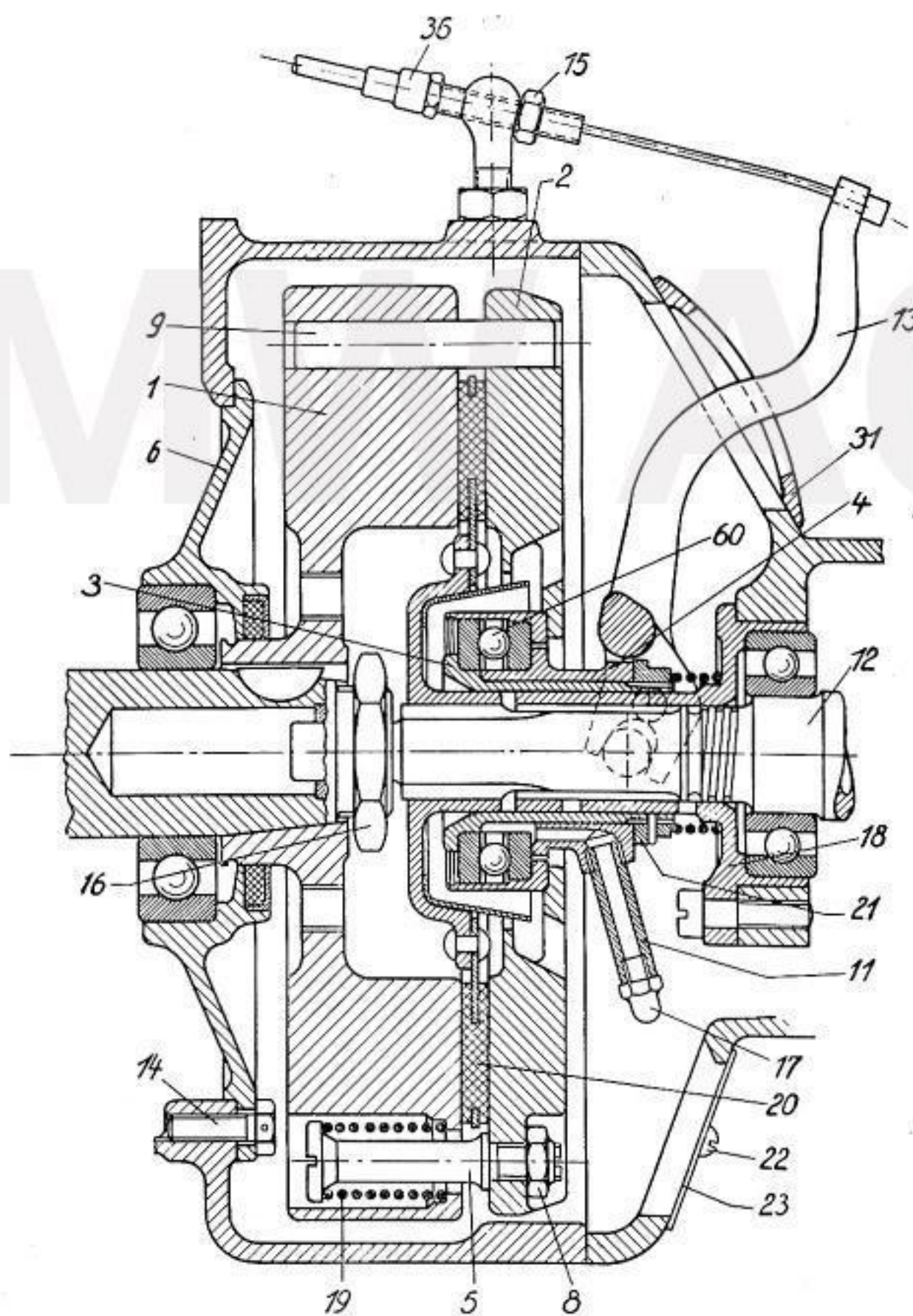
Abb. 26. Kupplung der R 4-Maschine
