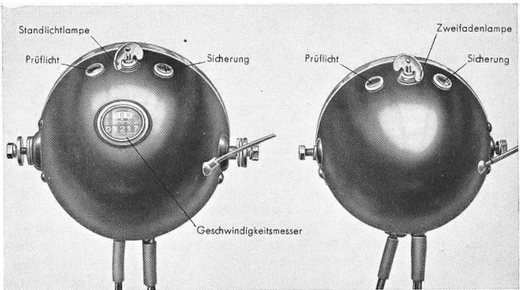
Abb. 32. Scheinwerfer der R 2-Maschine
