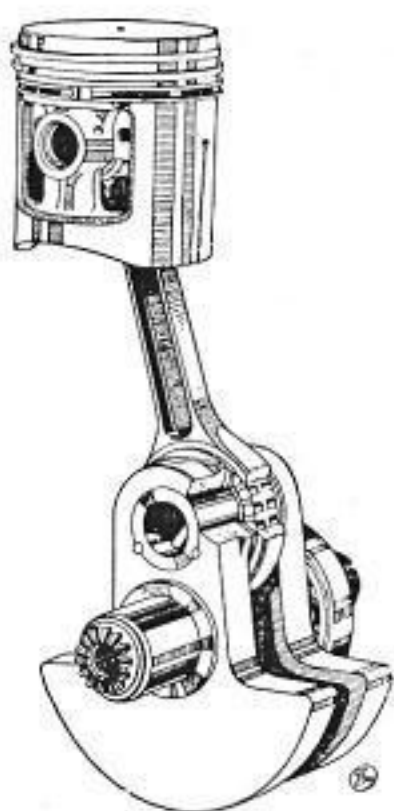
Abb. 20 Kurbelwelle, Pleuel und Kolben
