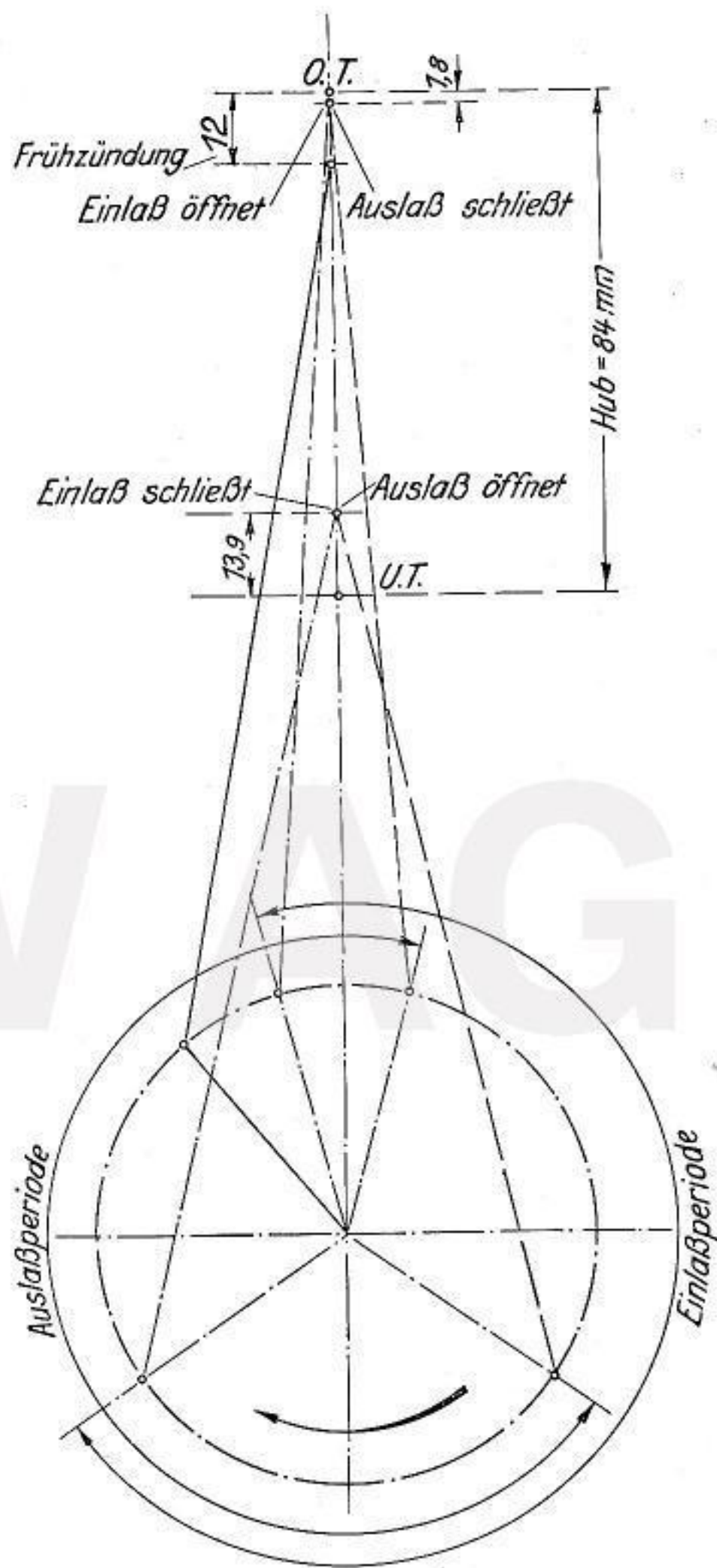
Abb. 34. Einstellschaubild der R 4-Maschine
