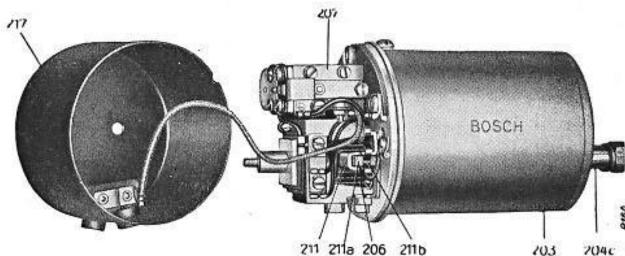
Abb. 12. Lichtmaschine mit abgenommenem Schutzdeckel
