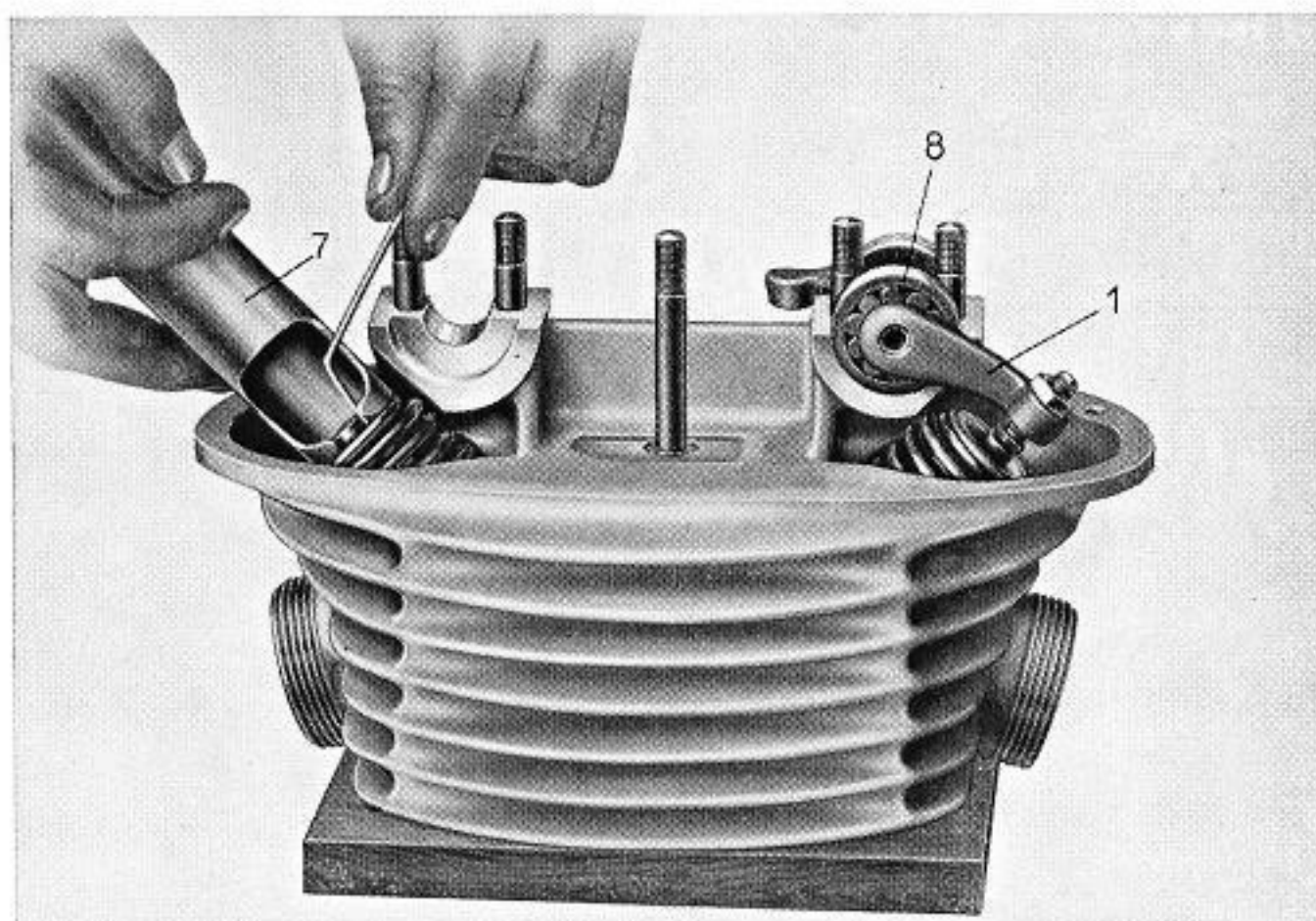
Abb. 35 Ausbau der Ventile bei der R 17-Maschine
