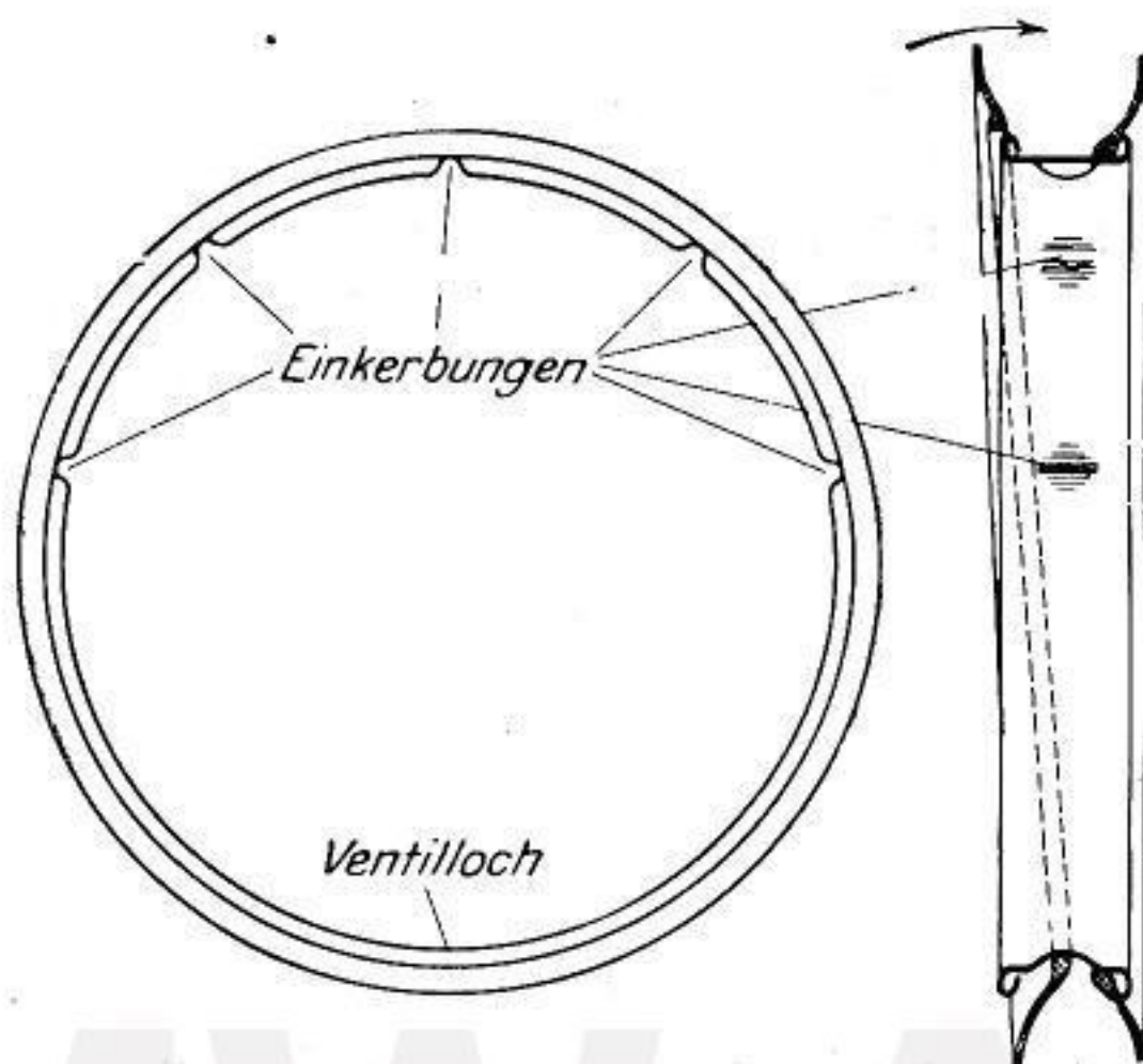
Abb. 42 Aufziehen von Drahtseilreifen auf Tiefbettsicherheitsfelgen
