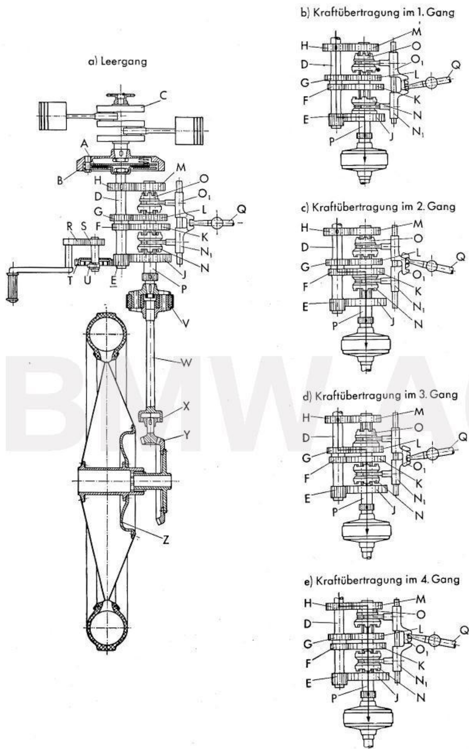
Abb. 27 Schema des Antriebes
