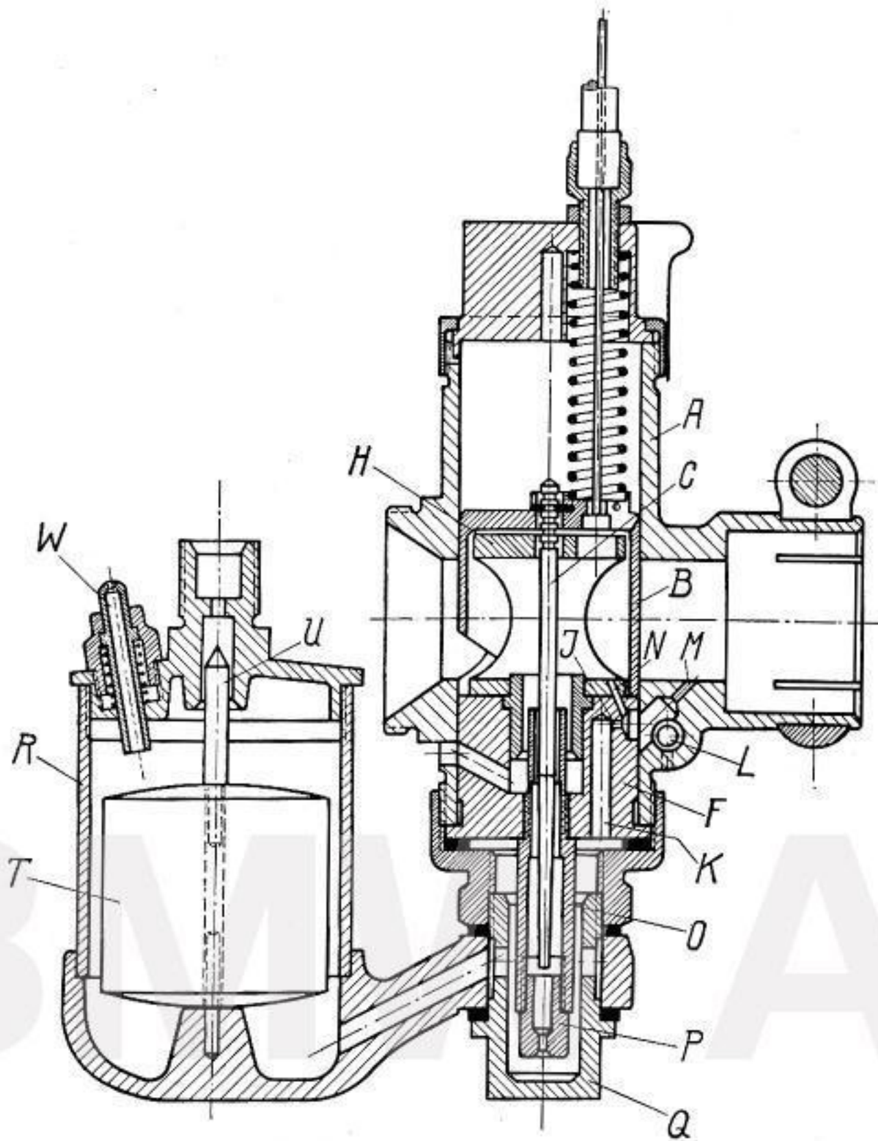
Abb. 25 Vergaser der Sportmaschine
