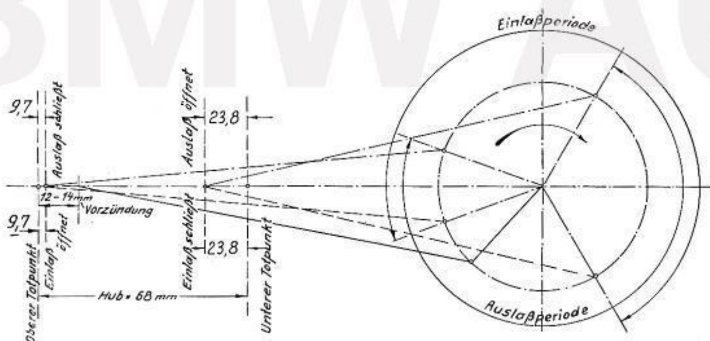
Abb. 38 Einstellschaubild für die Sportmaschine
