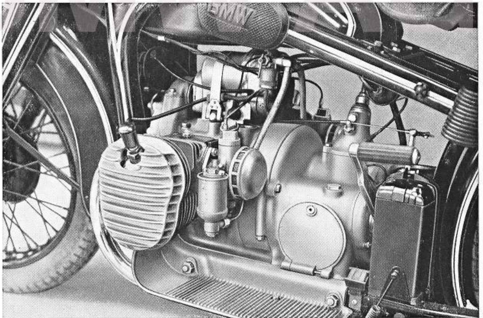
Abb. 16 Motor und Getriebe der R 12-Zweivergaser-Maschine
