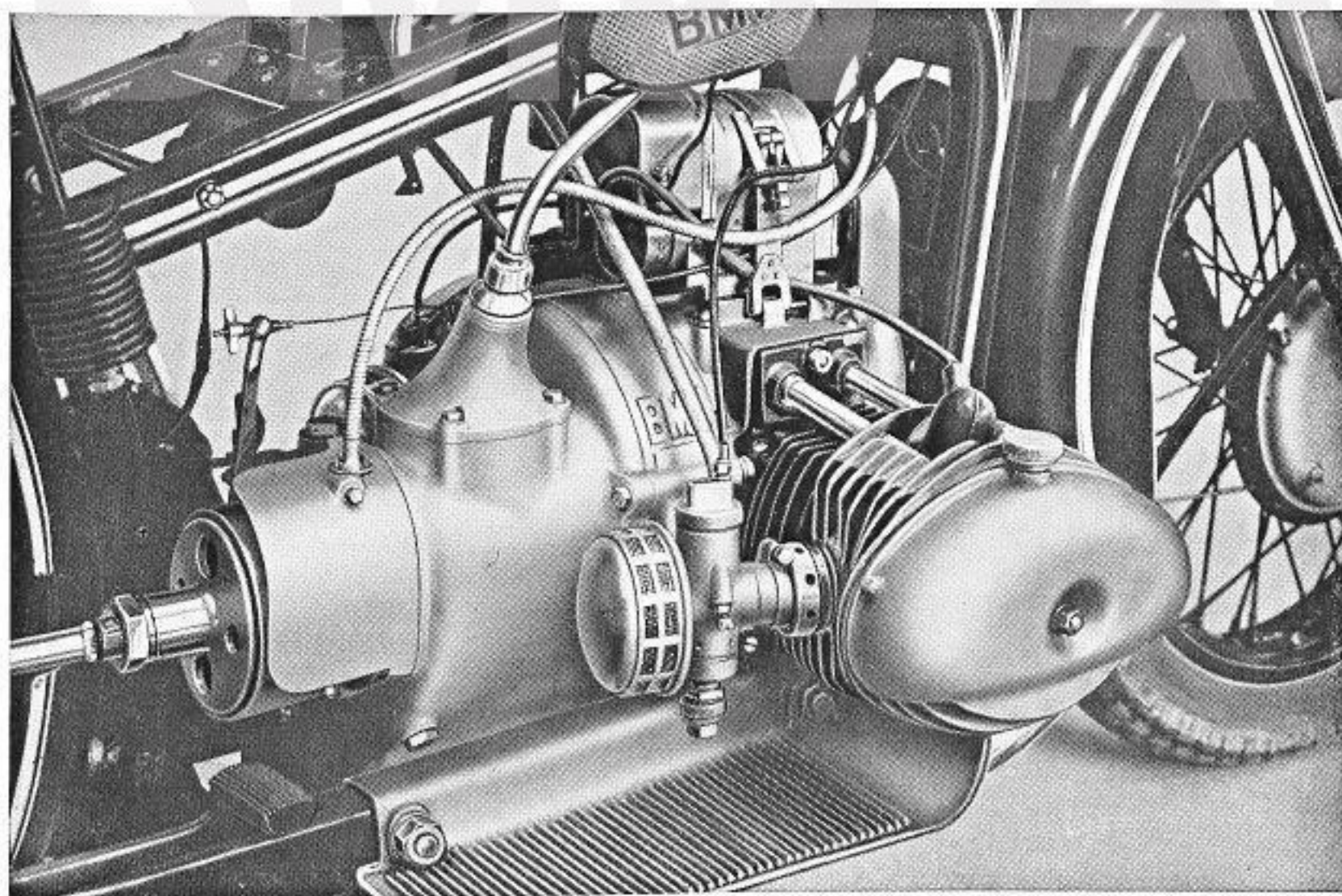
Abb. 17 Motor und Getriebe des R 17-Sportrades
