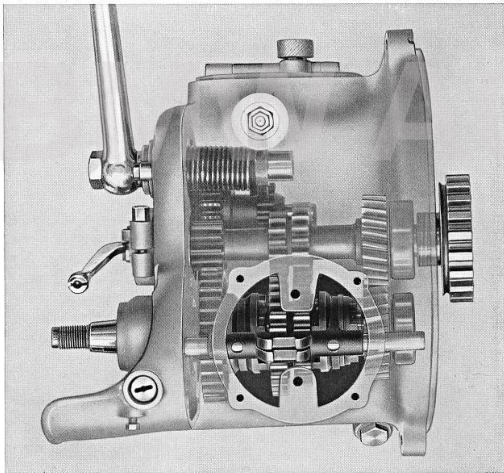
Abb. 28. Getriebe der Baumuster R 12 und R 17.
