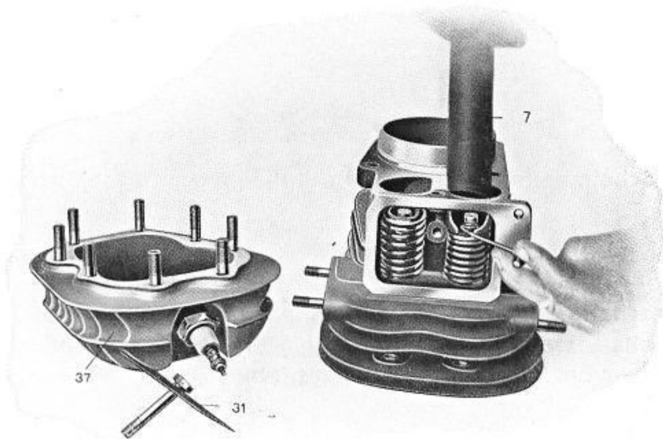
Abb. 34 Ausbau der Ventile bei der R 12-Maschine
