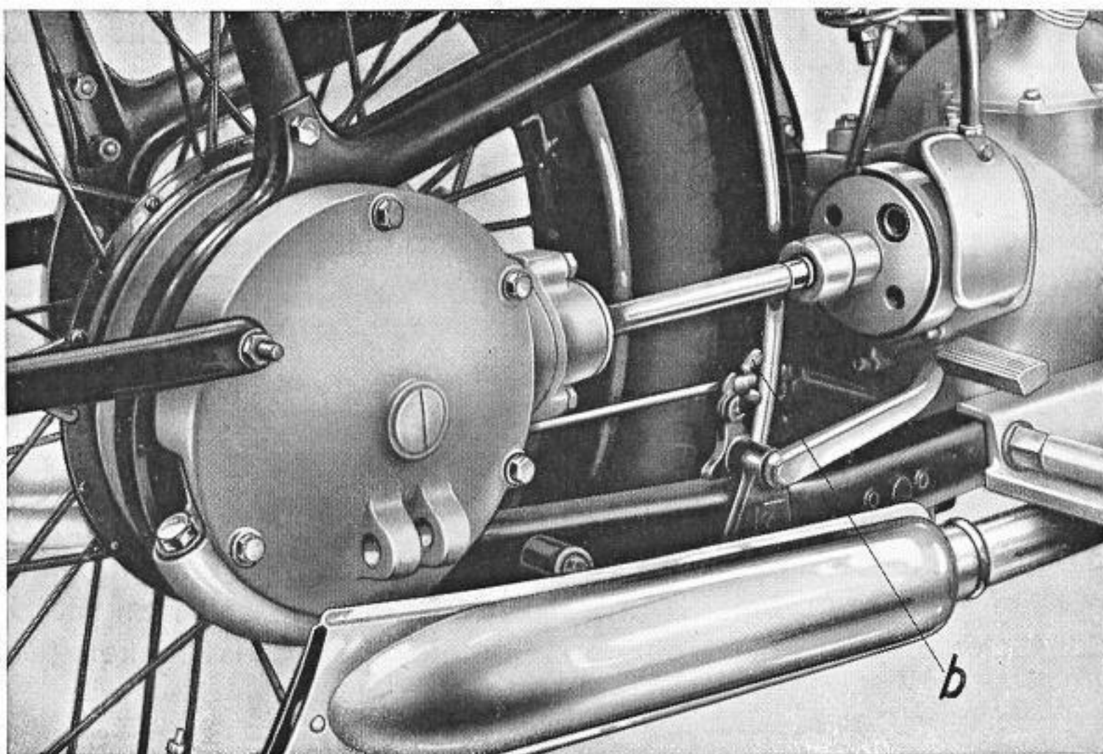
Abb. 11. Hinterradbremse
