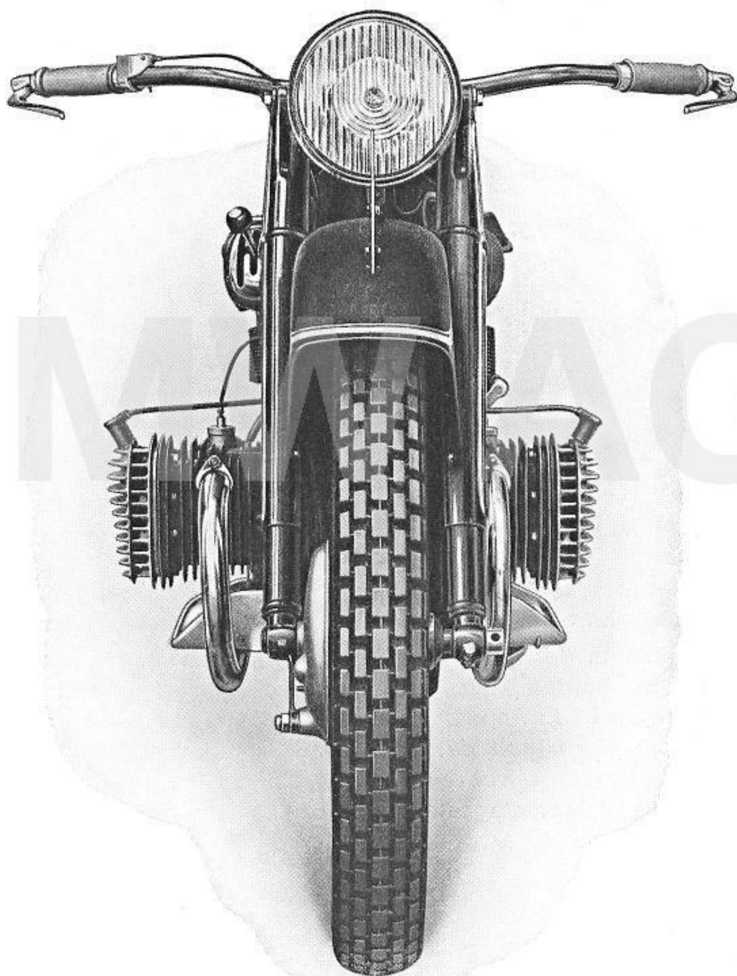
Abb. 31 Vorderansicht des R 12-Tourenrades
