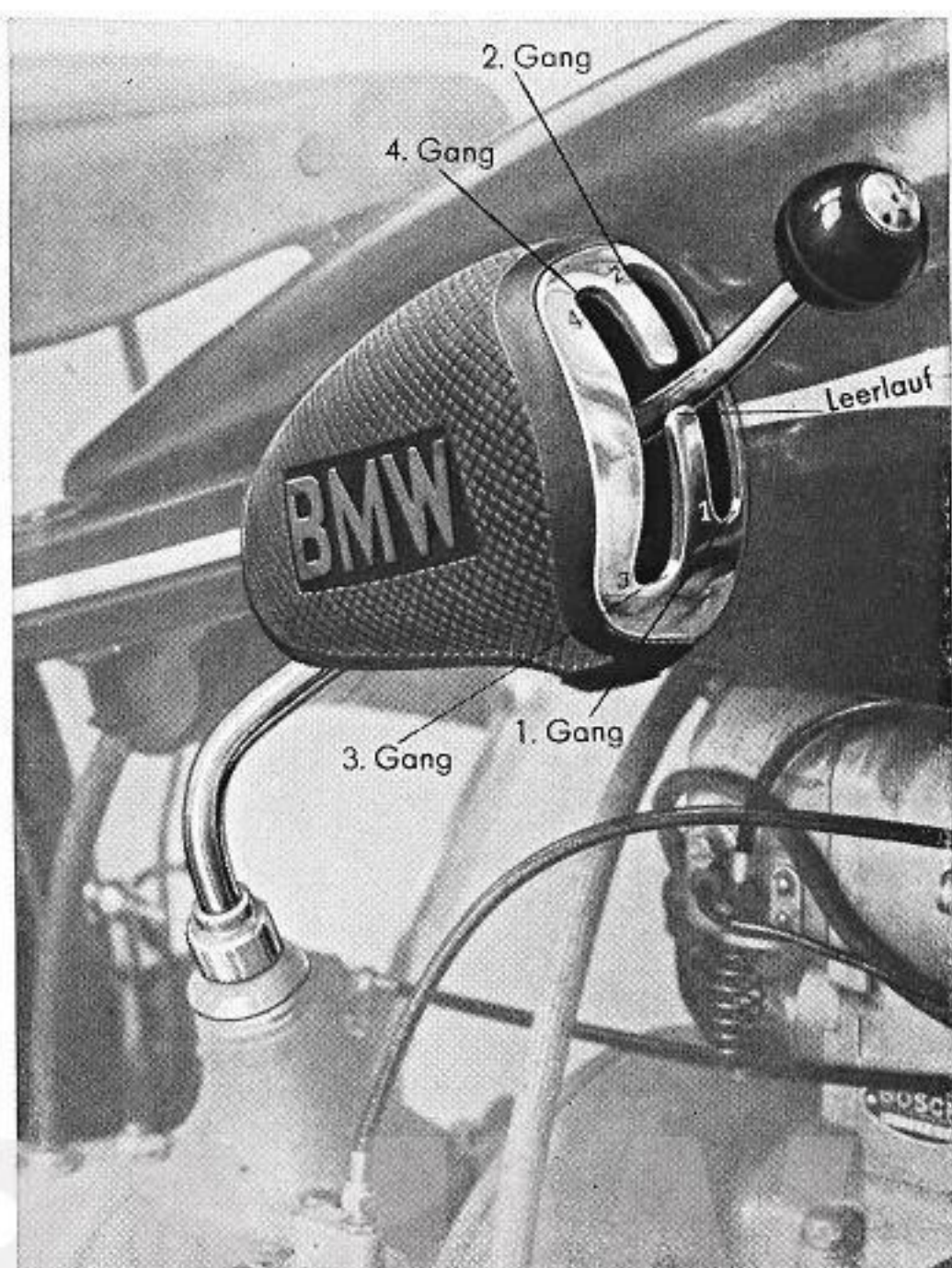
Abb. 8 Getriebebeschaltethebel
