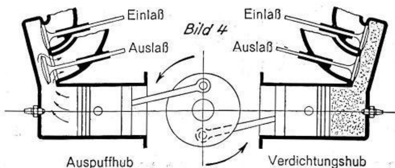
Abb. 19 Schaubildliche Darstellung der Arbeitsweise des Motors der R 12-Tourenmaschine
