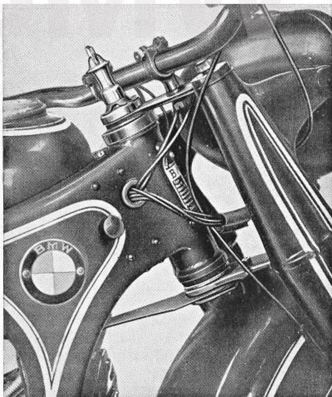
Abb. 29 Steuerkopf und Steuerungsdämpfer
