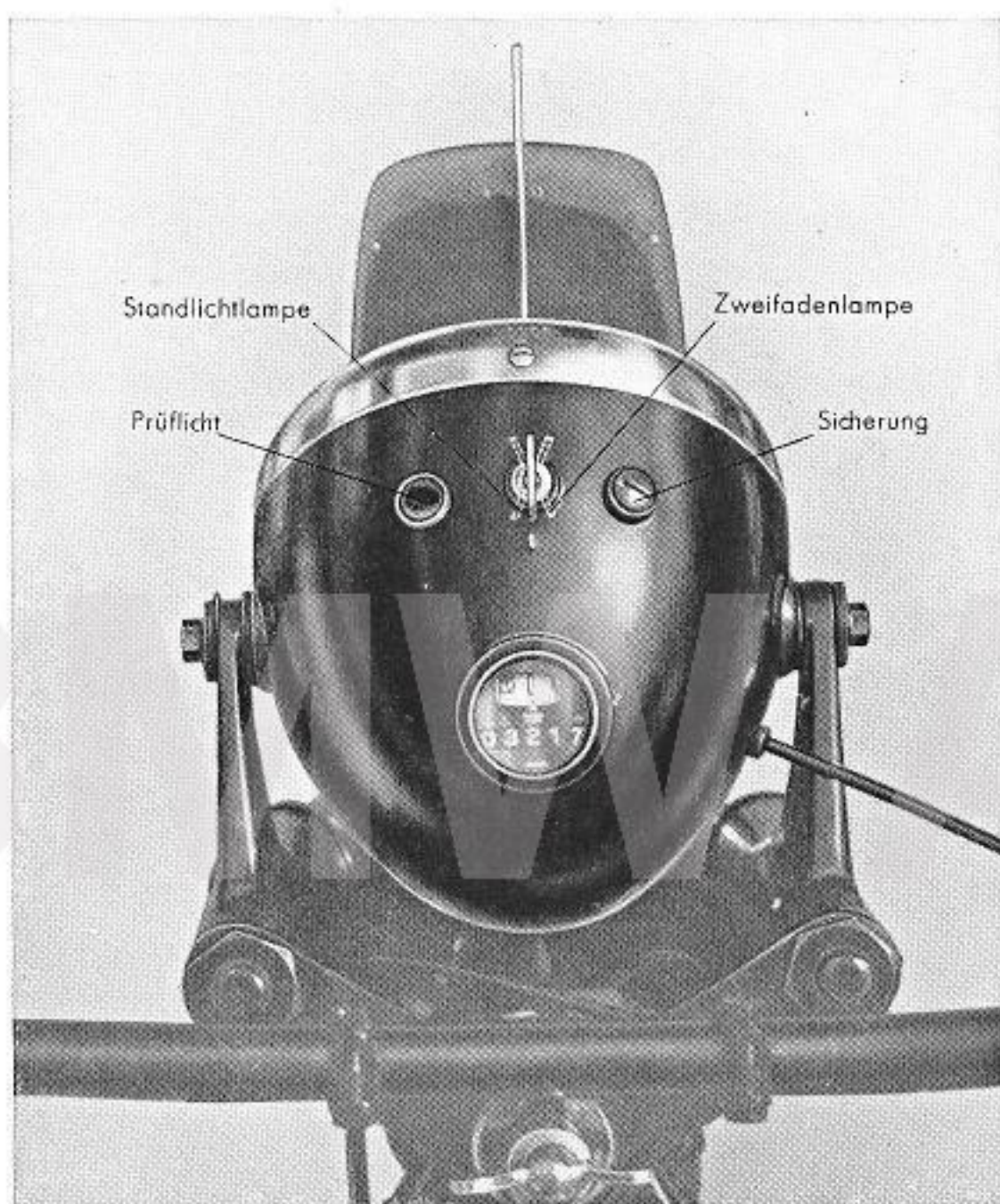
Abb. 33 Scheinwerfer von oben mit Stellungen des Schaltschlüssels
