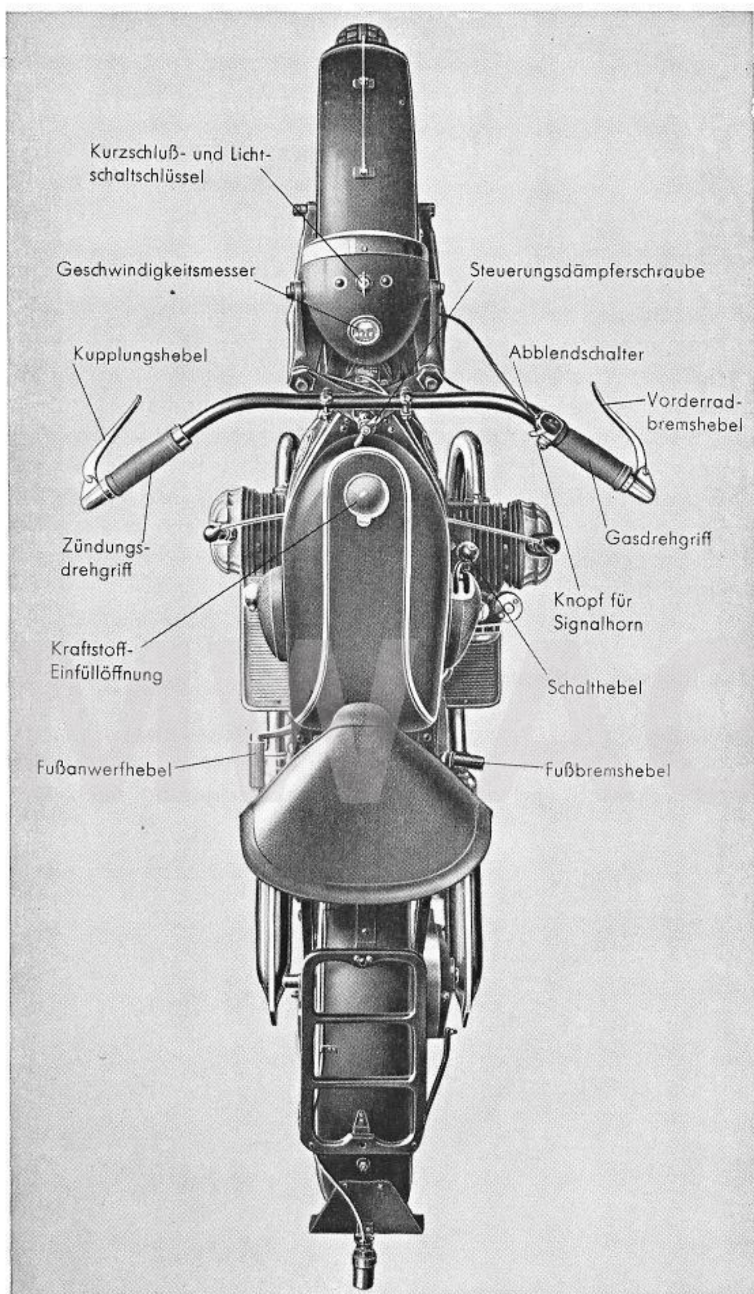
Abb. 6 Die Bedienungshebel am BMW-Kraftrad
