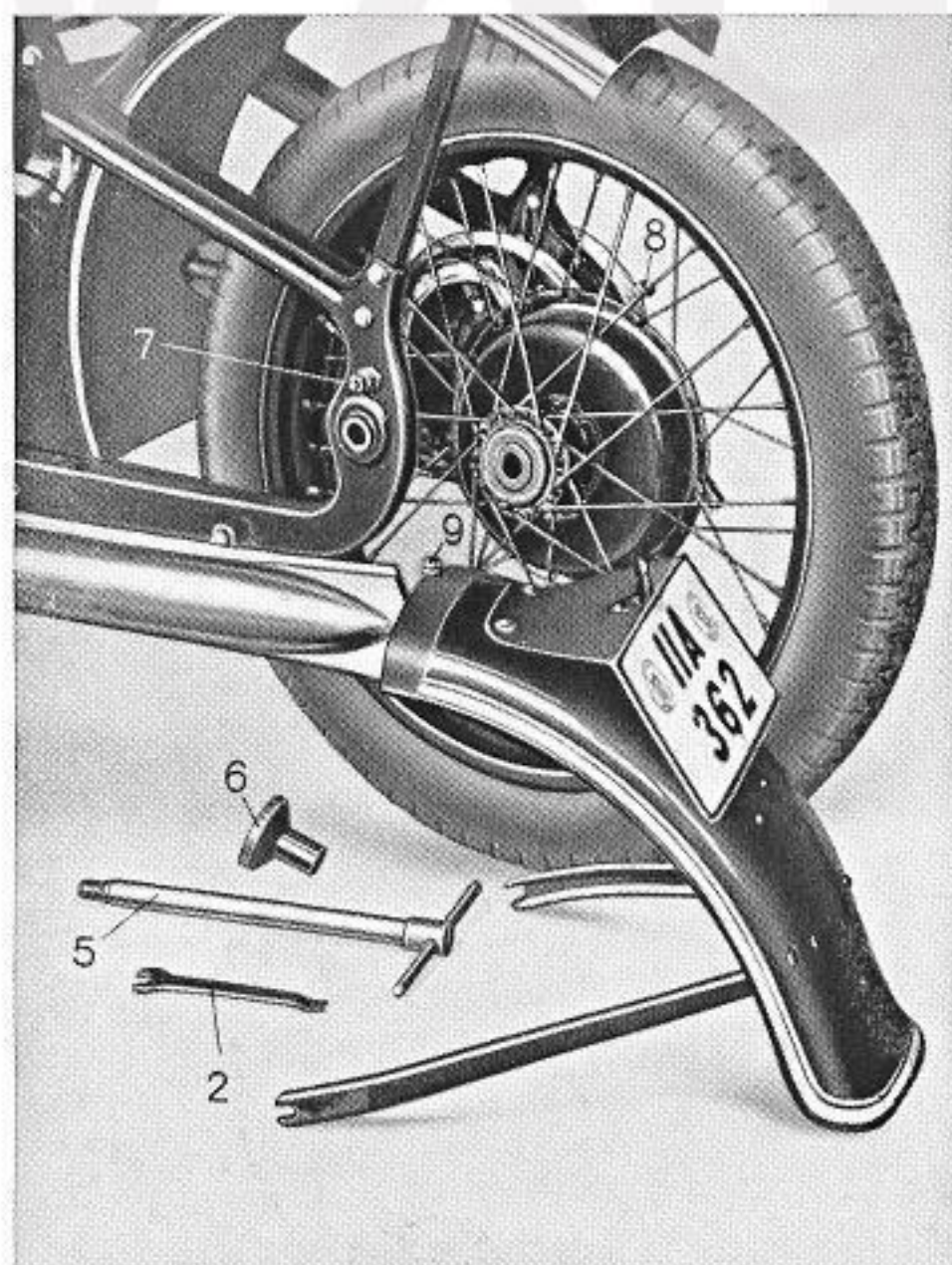
Abb. 41 Ausbau des Hinterrades bei Seitenwagenmaschinen
