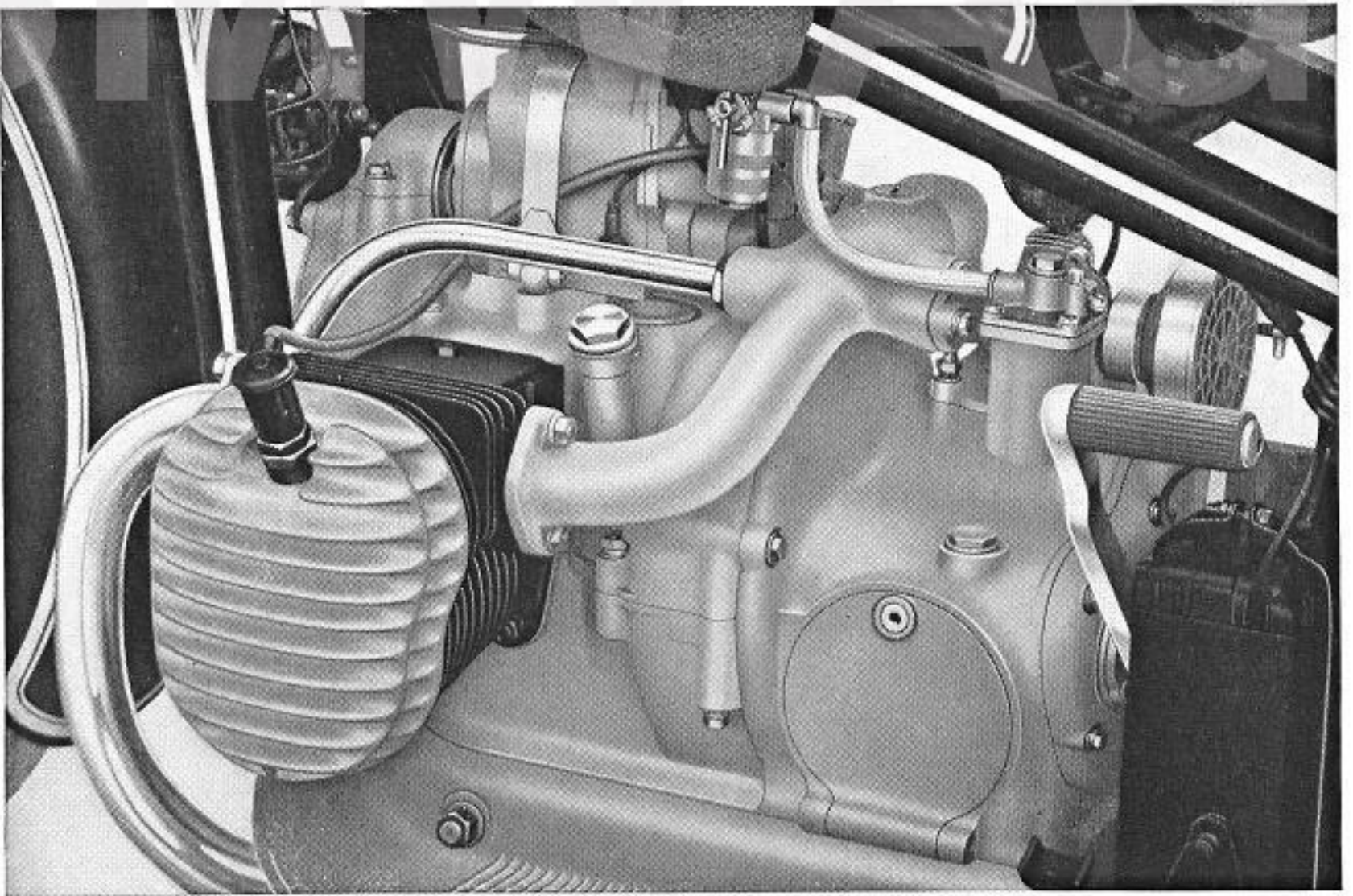
Abb. 18 Motor und Getriebe der R 12-Einvergaser-Maschine
