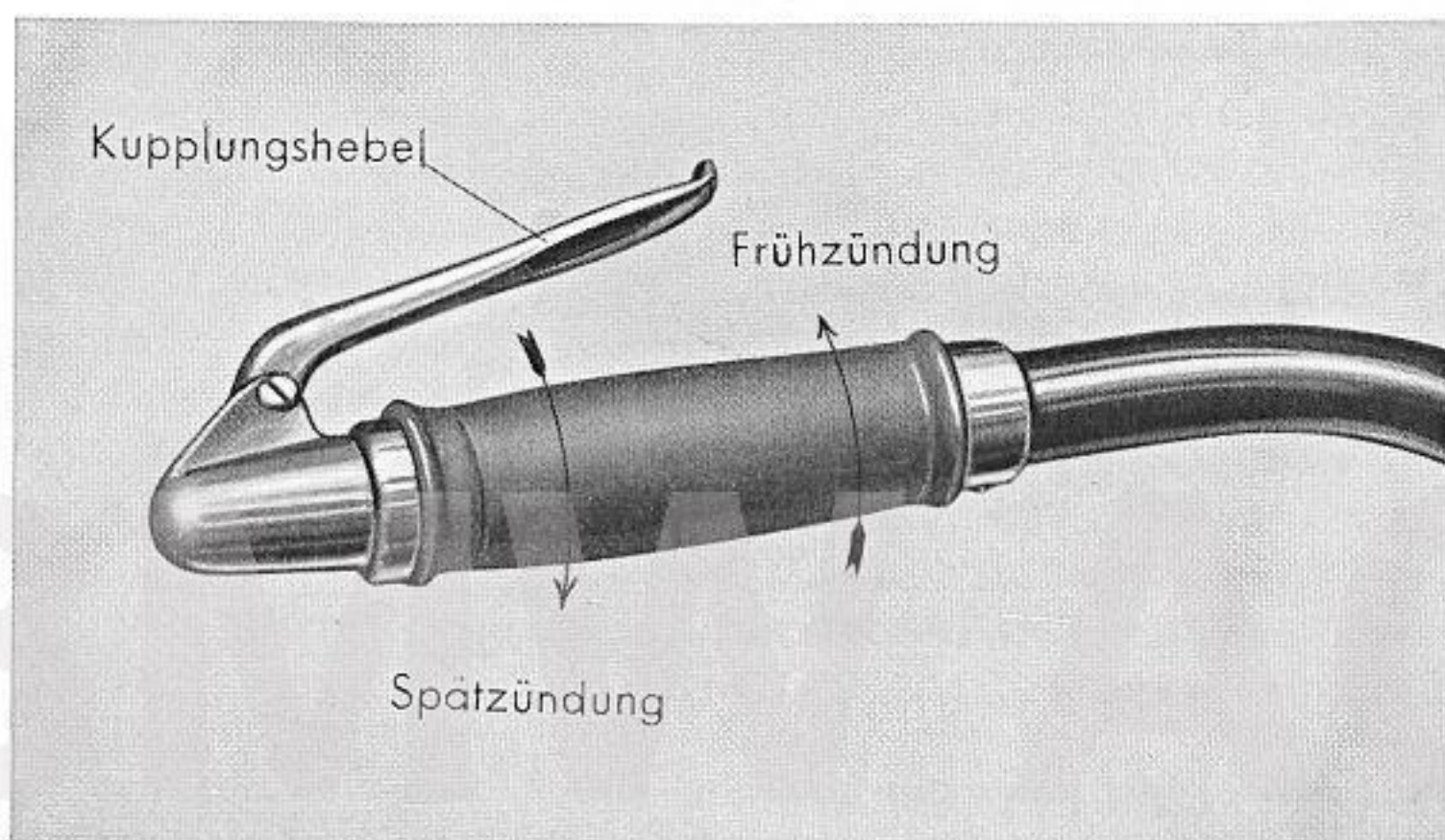
Abb. 7 Linkes Lenkerende (Zündungsdrehgriff)
