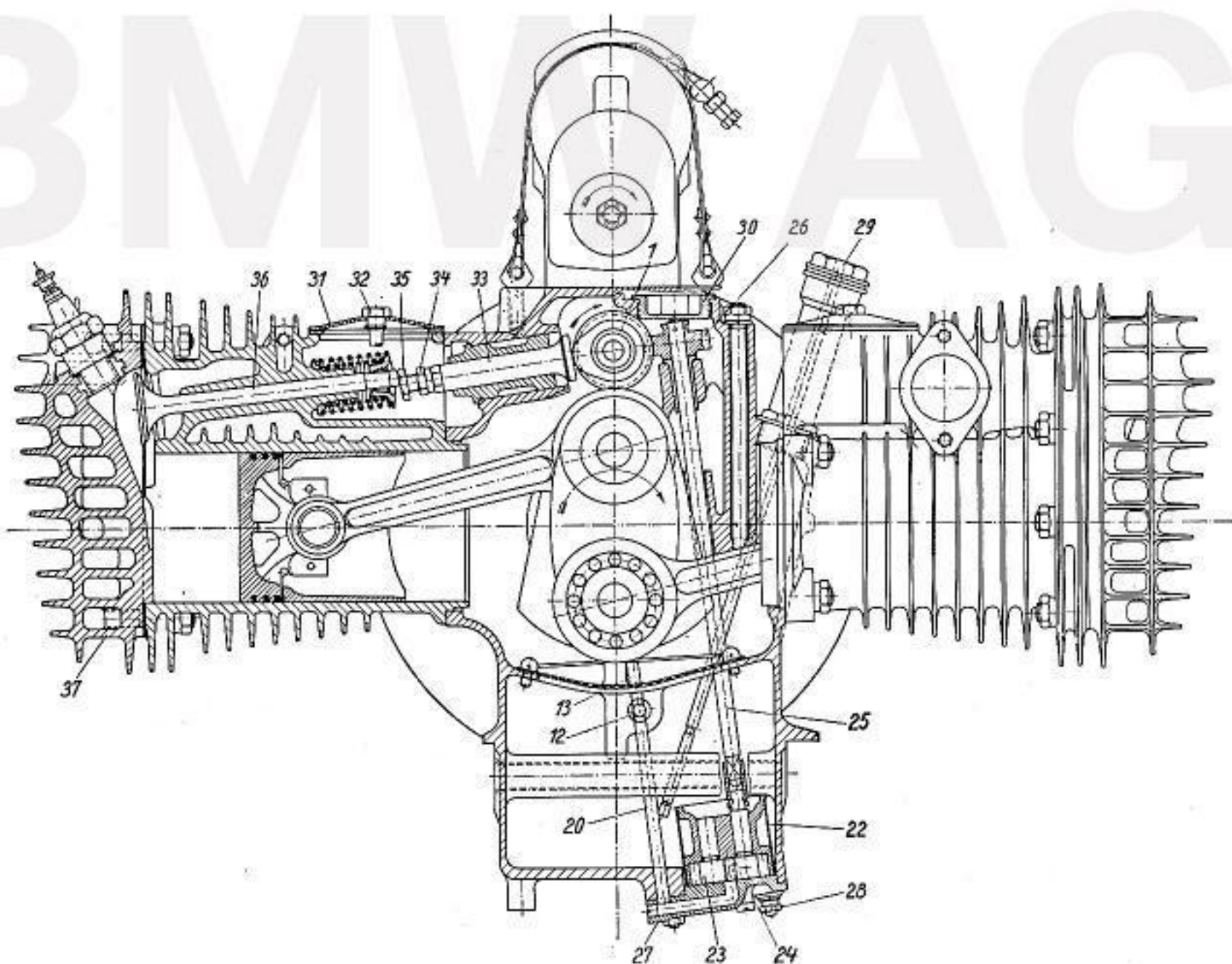
Abb. 36 Tourenmotor mit teilweisem Querschnitt durch die Zylindermittle
