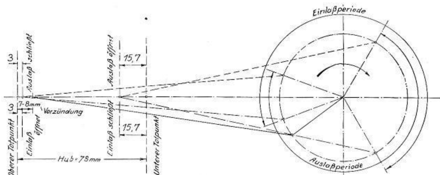
Abb. 37 Einstellschaubild für die Tourenmaschine
