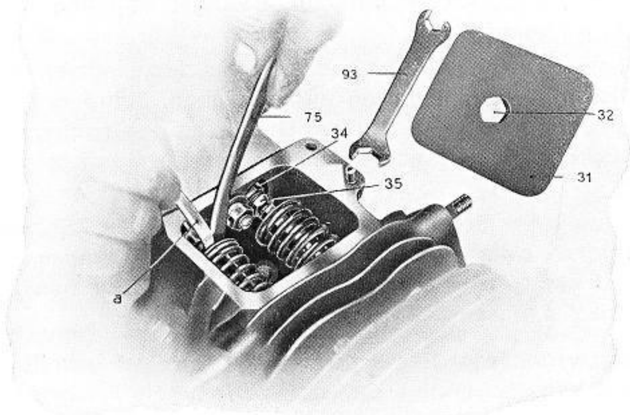
Abb. 14 Einstellen des Ventilspieles der Tourenmaschine
