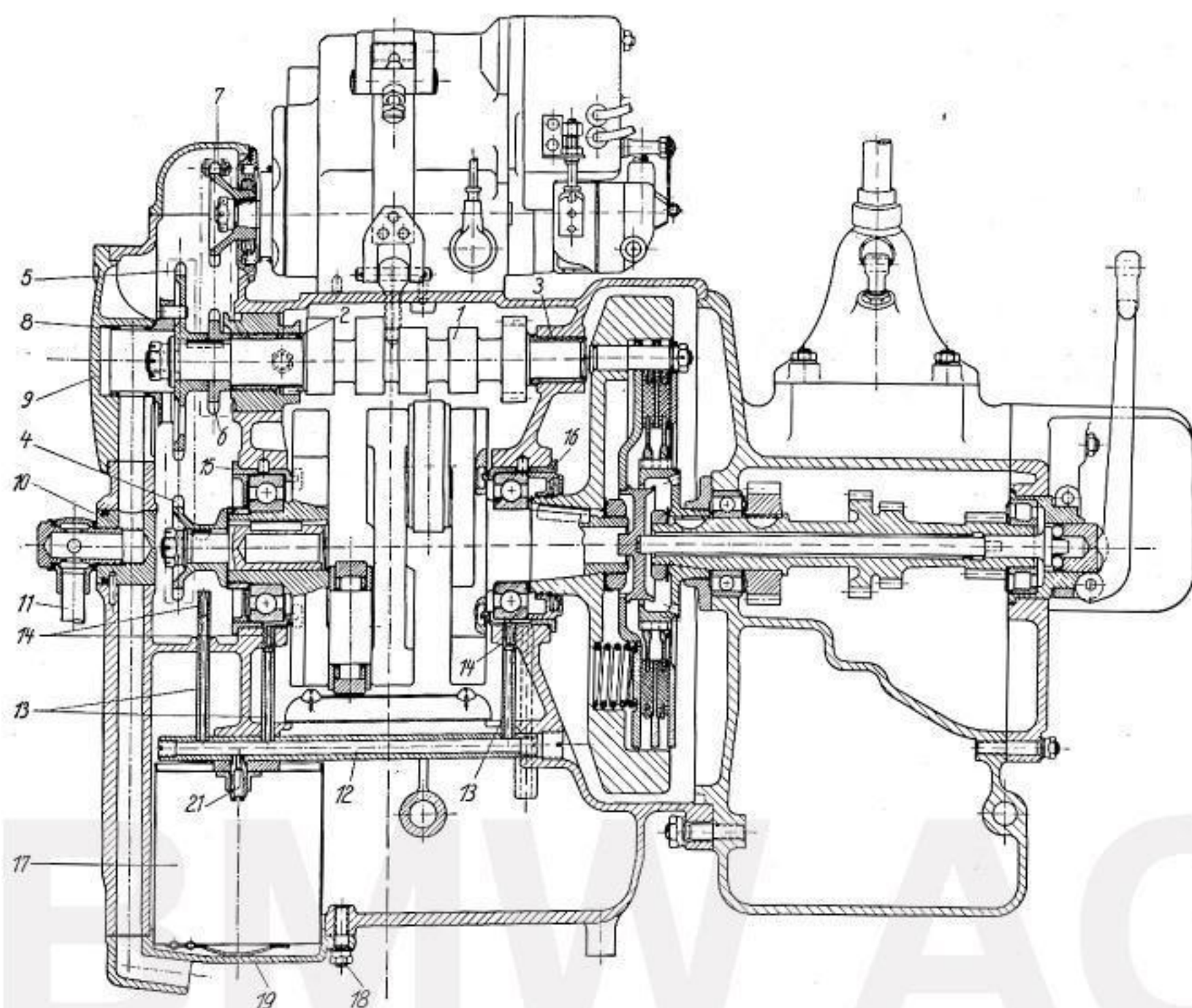
Abb. 22 Längsschnitt durch Motor und Getriebe
