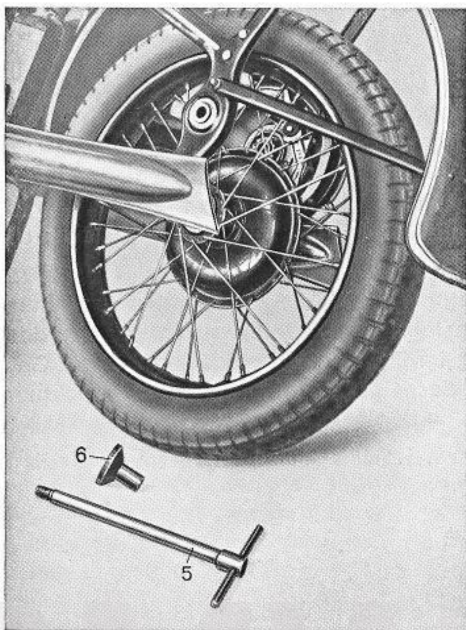
Abb. 40 Ausbau des Hinterrades bei Einzelmaschinen
