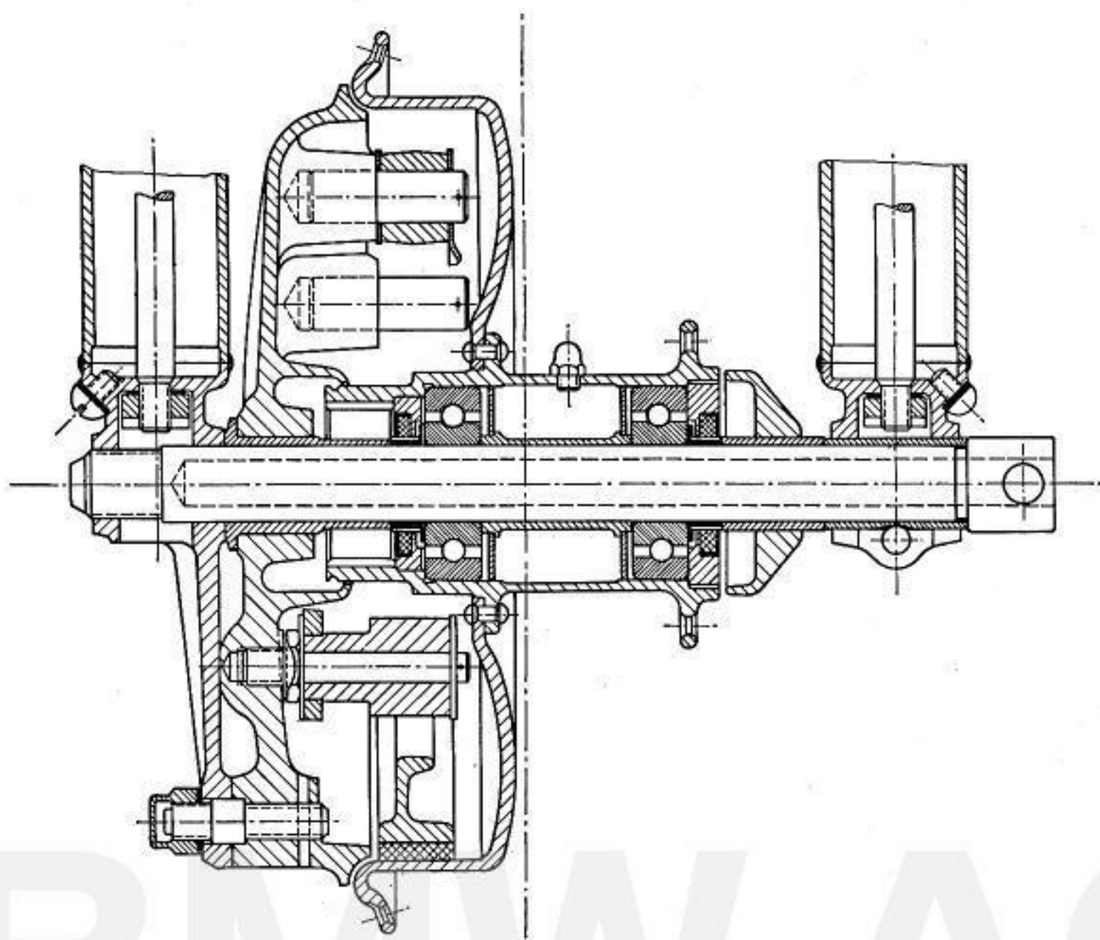
Abb. 32 Schnitt durch die Vorderradnabe und -bremse
