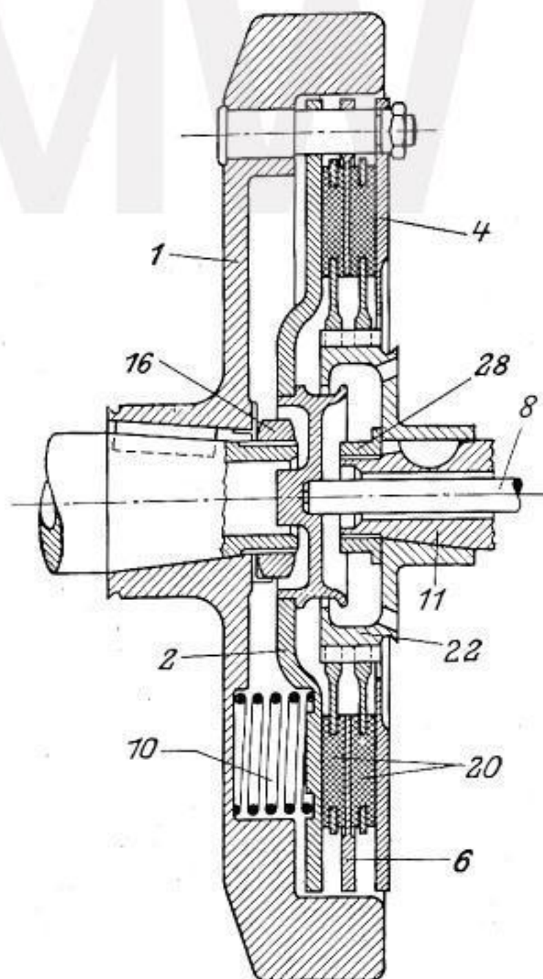
Abb. 26 Zweischeiben- Reibungskupplung
