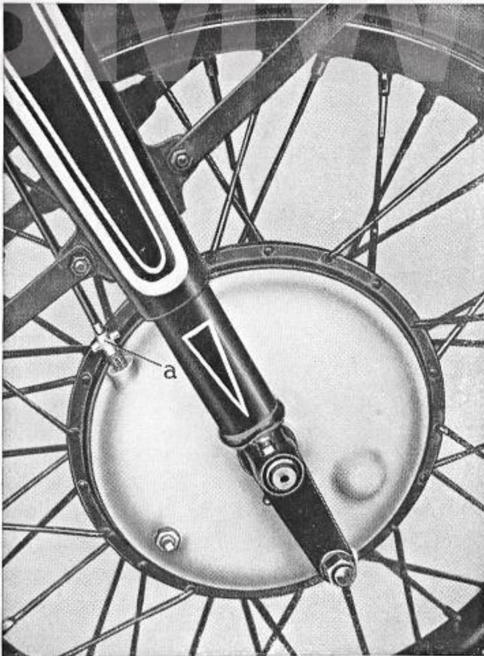
Abb. 10. Vorderradbremse
