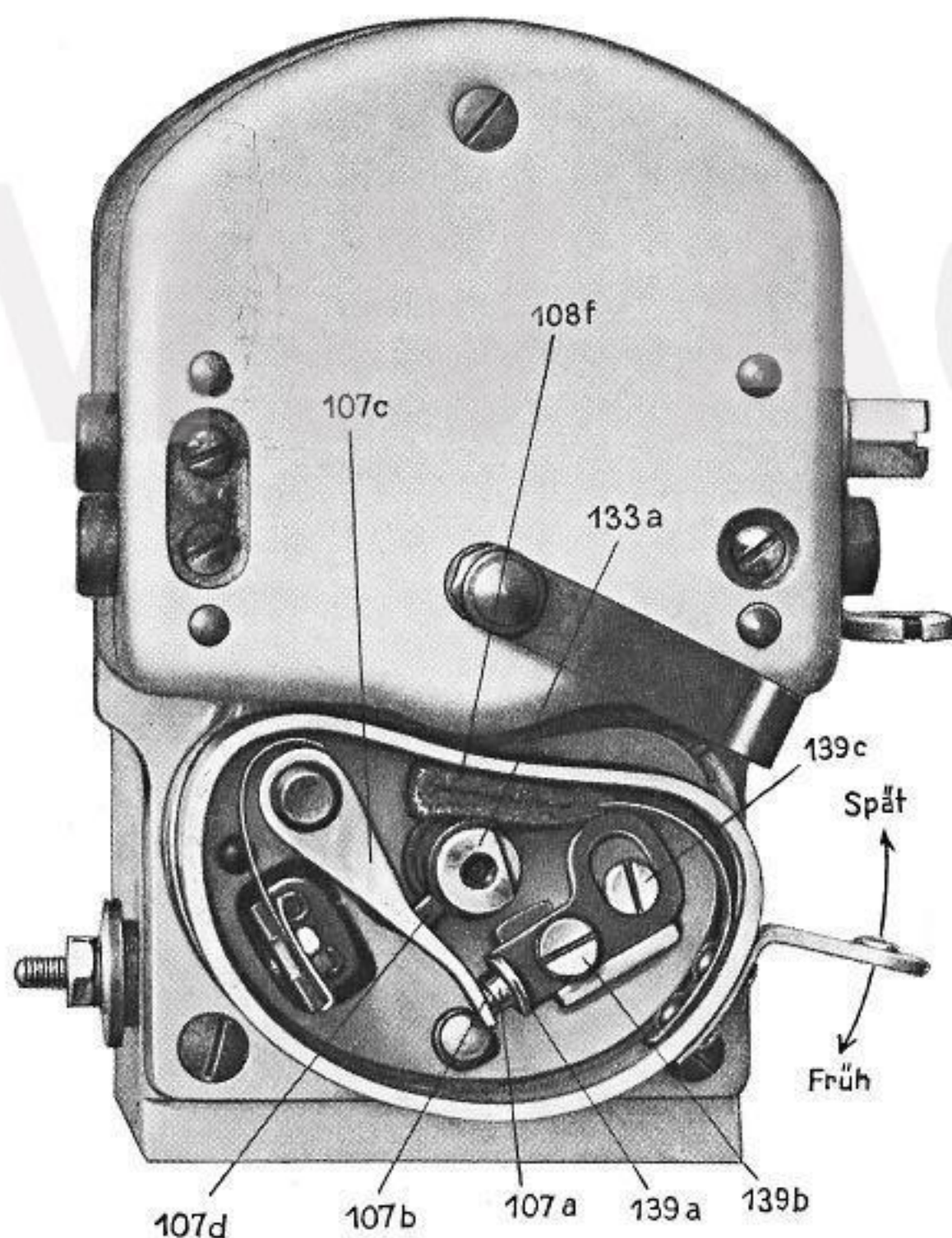
Abb. 12 Unterbrecher des Lichtbatteriezünders
