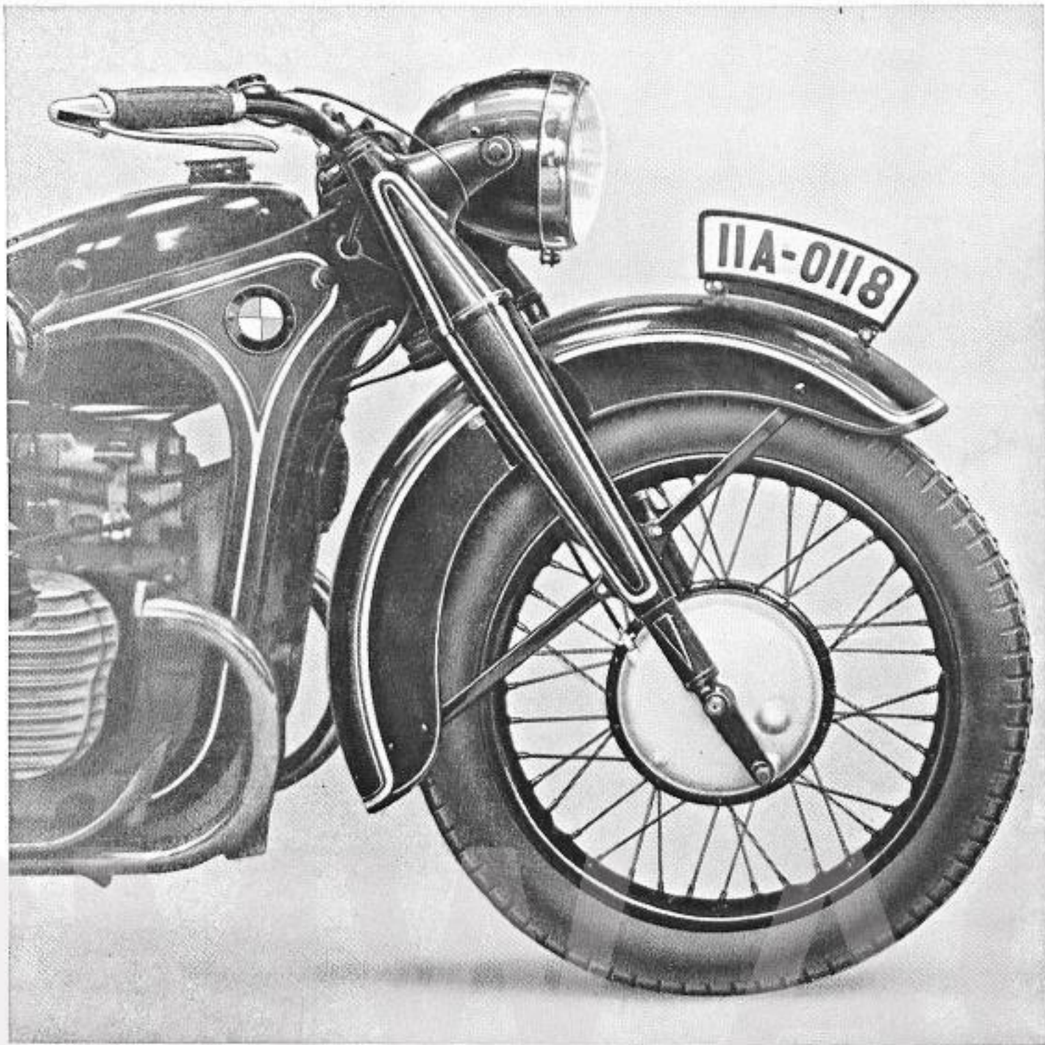
Abb. 30 Vorderrad mit Gabel und Scheinwerfer
