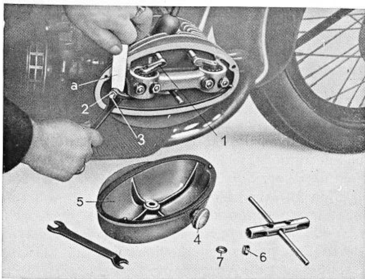
Abb. 15 Einstellen des Ventilspieles der Sportmaschine
