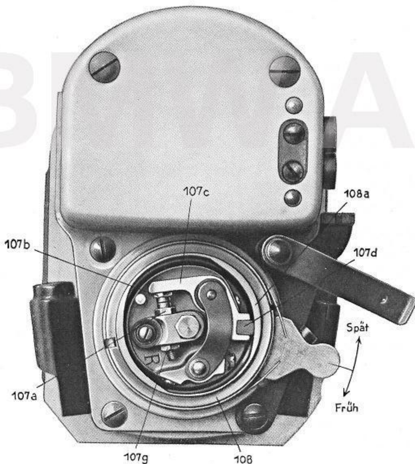
Abb. 13 Unterbrecher des Lichtmagnetzünders
