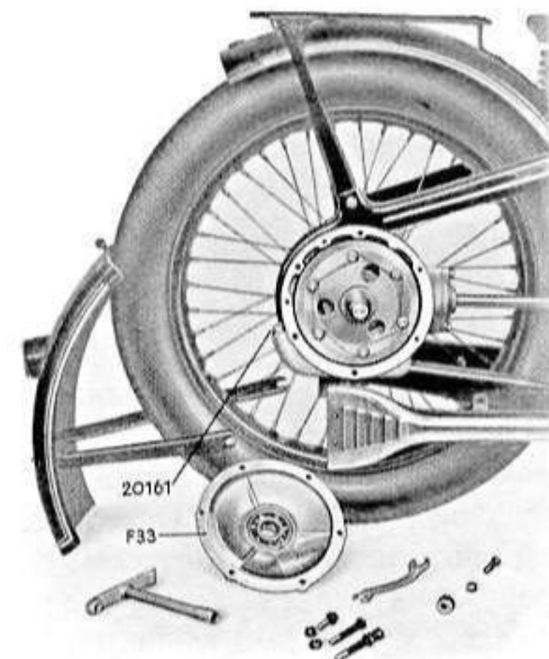
Abb. 18 Abnehmen des Kardangehäusedeckels
