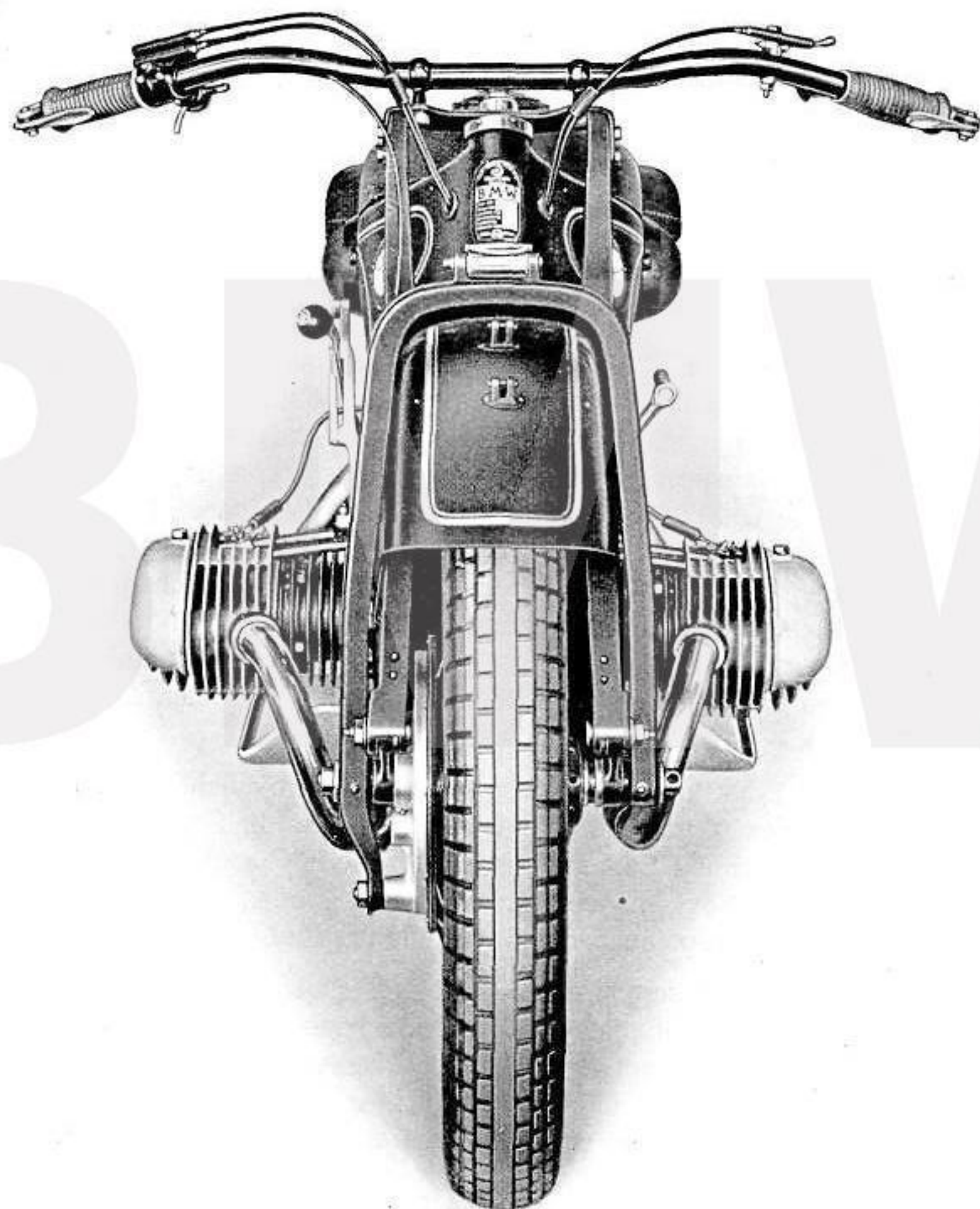
Abb. 3. Vorderansicht des Sportrades R 16
