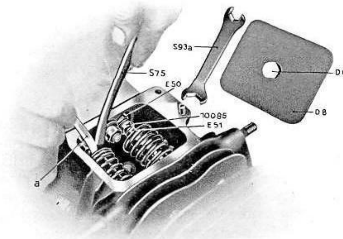
Abb. 22 Einstellen des Ventilspieles der Tourenmaschine
