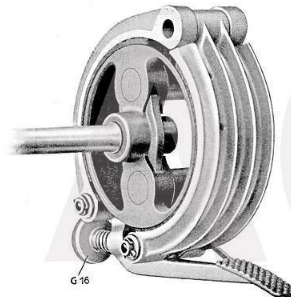
Abb. 20 Kardan-Fußbremse
