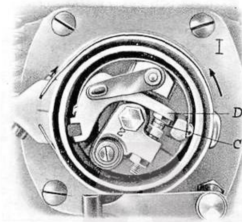
Abb. 28 Unterbrecher
