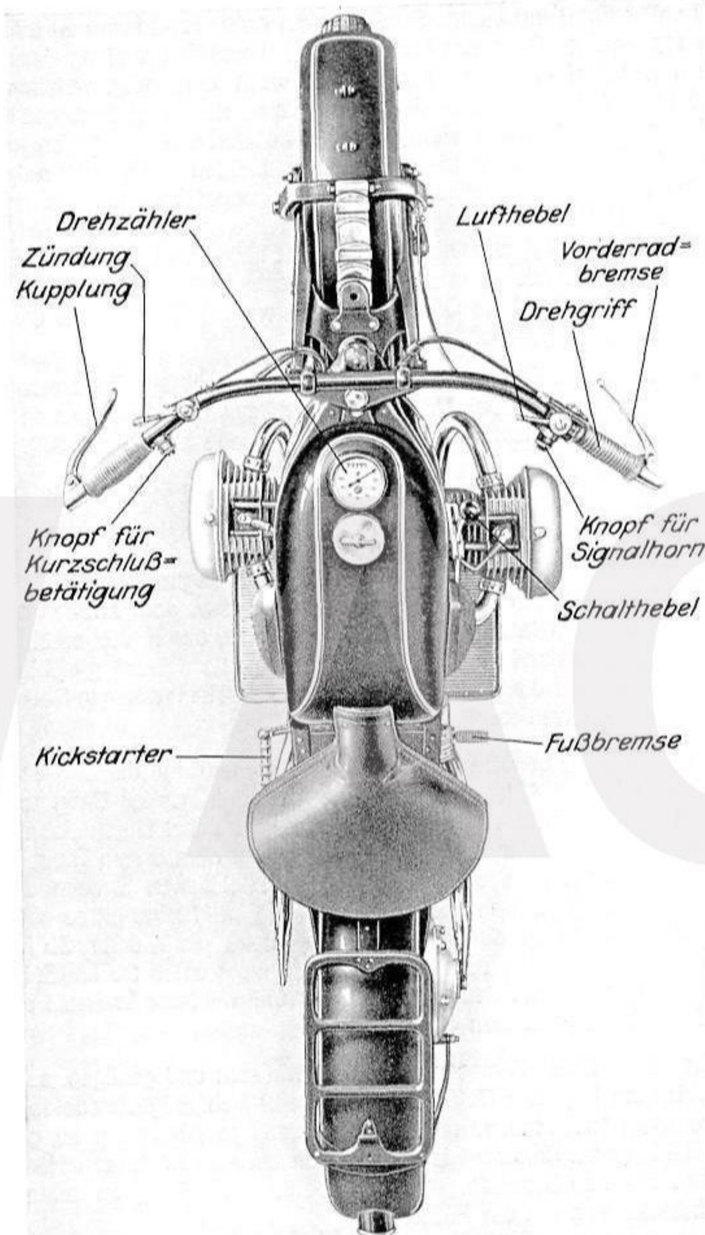
Abb. 34 Die Bedienungshebel am BMW-Kraftrad
