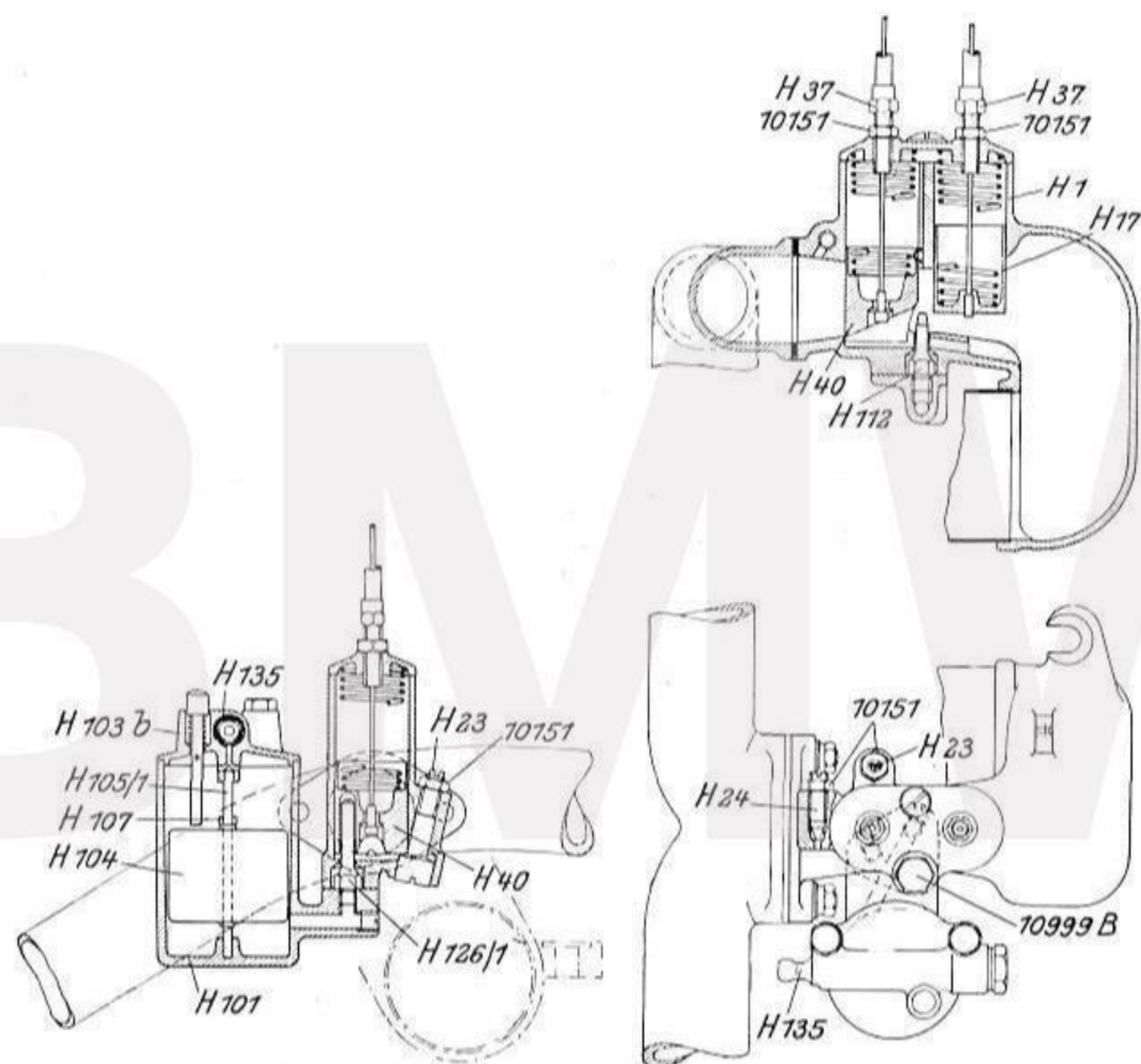
Abb. 13 BMW-Vergaser mit Schwimmer
