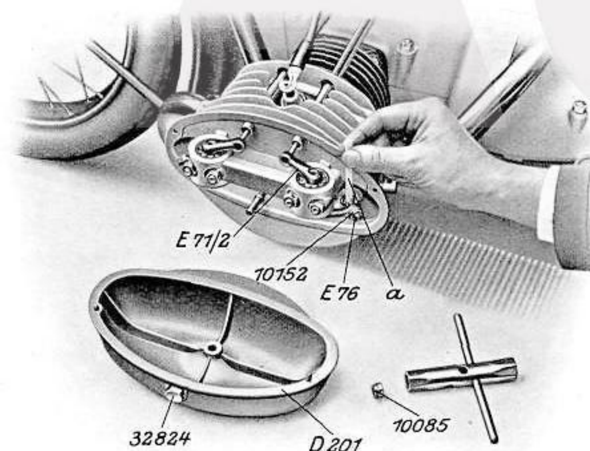
Abb. 23 Einstellen des Ventilspieles der Sportmaschine
