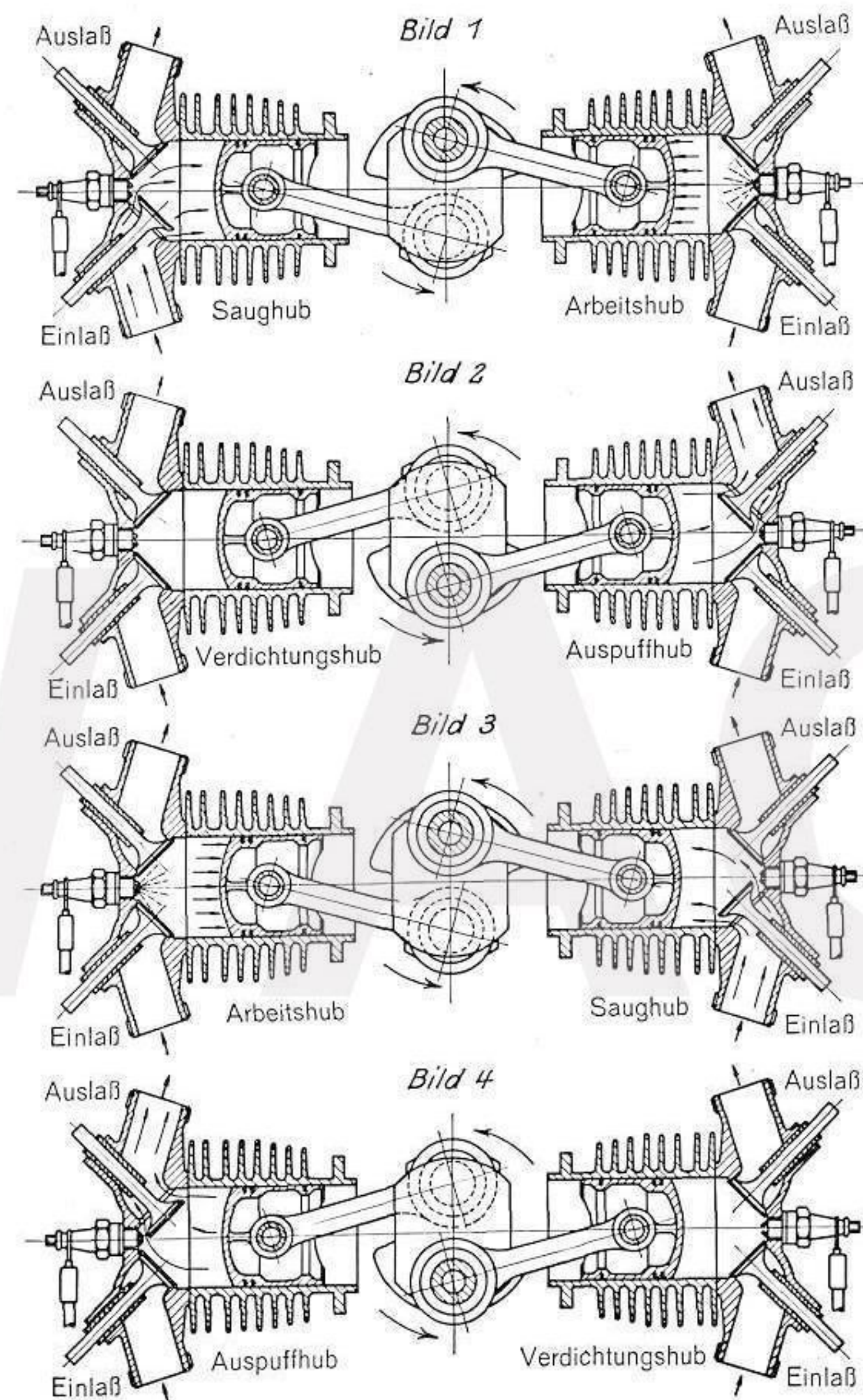
Abb. 9 Schematische Darstellung der Arbeitsweise des Motors der Sportmaschine R 16
