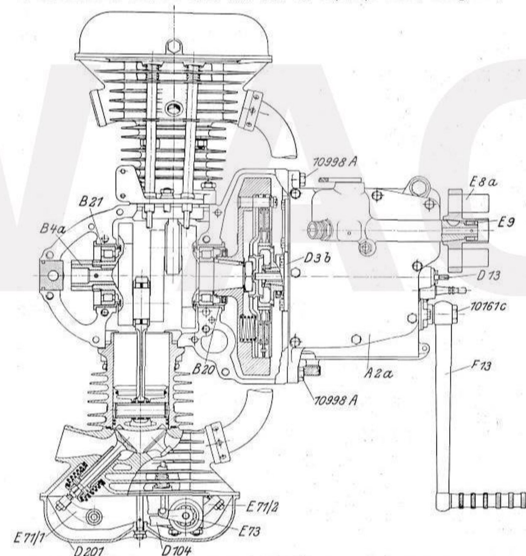
Abb. 15 Sportmotor mit teilweisem Horizontalschnitt durch die Zylindermitte
