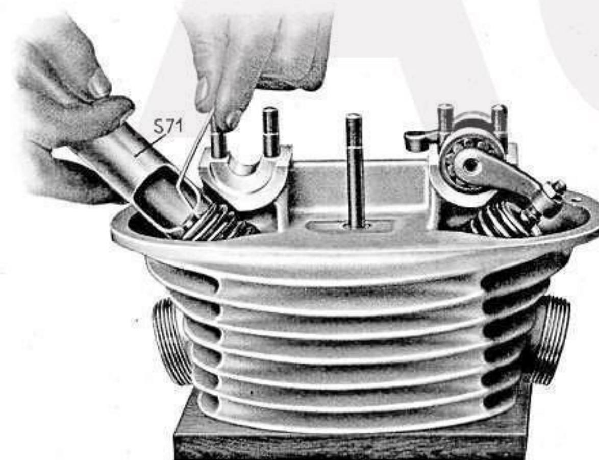
Abb. 25 Ausbau der Ventile bei der Sportmaschine
