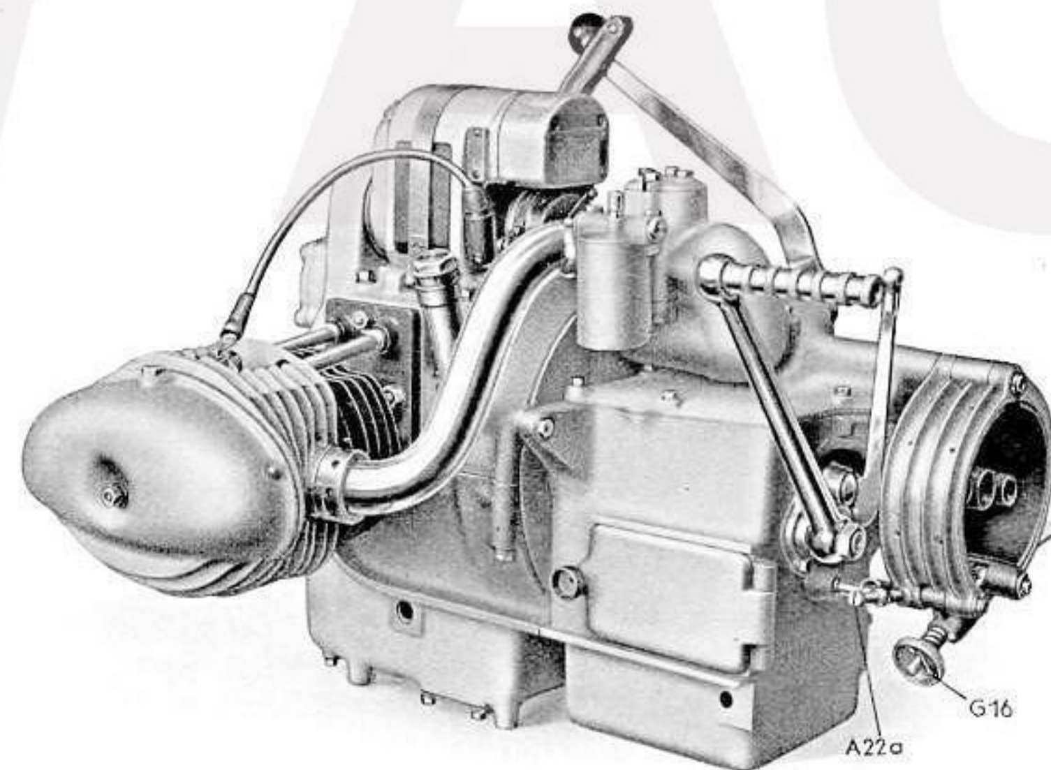
Abb. 5 Motor des Sportrades
