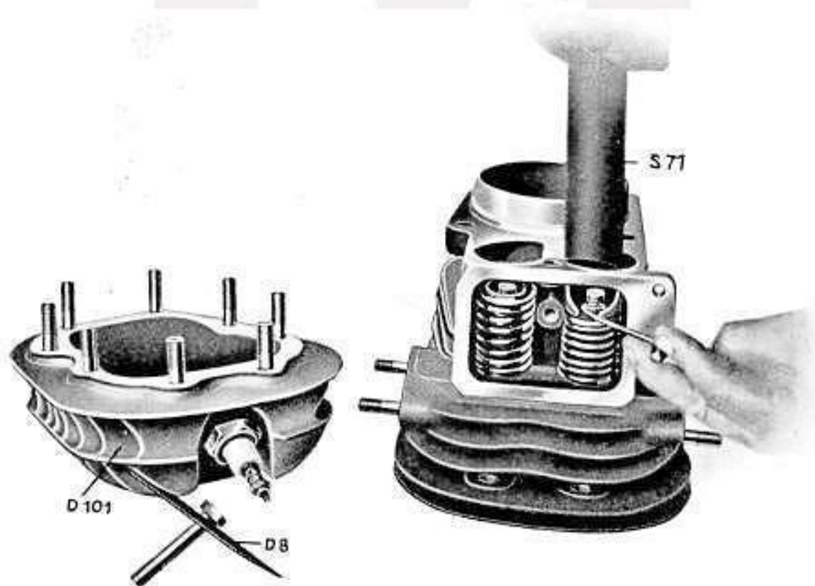
Abb. 24 Ausbau der Ventile bei der Tourenmaschine
