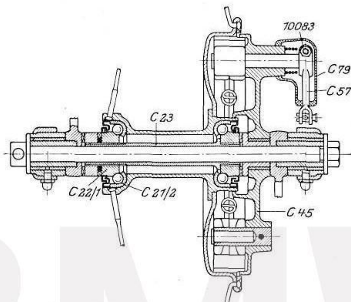
Abb. 21 Schnitt durch die Vorderradbremse
