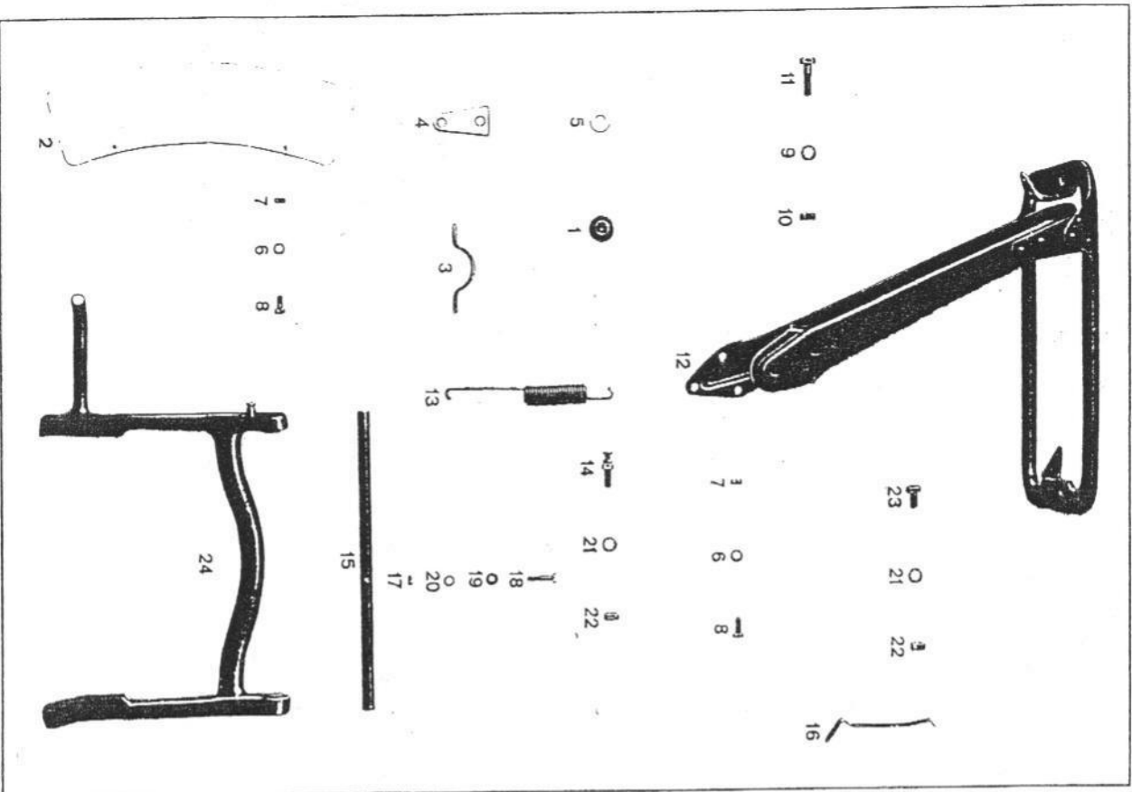
Tafel 6 Vorder- und Hinterradschutzblech, Gepäckträger und Kippständer
