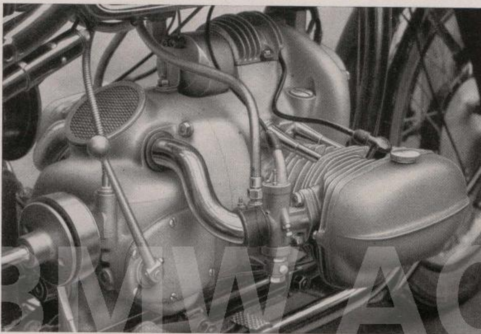
Bild 13. Motorblock R 51
