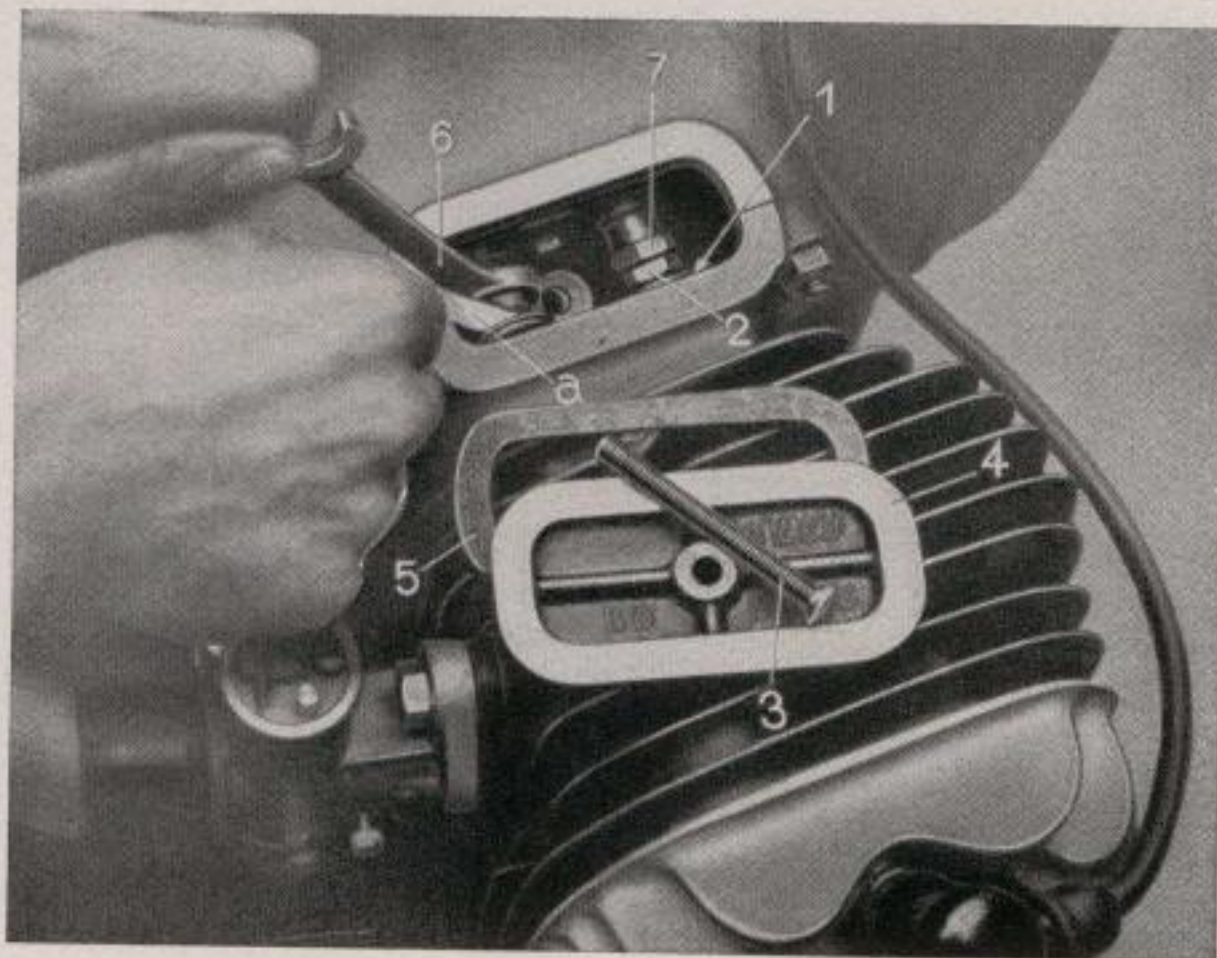
Bild 7. Ventilmachstellung R 61 (R 71)
