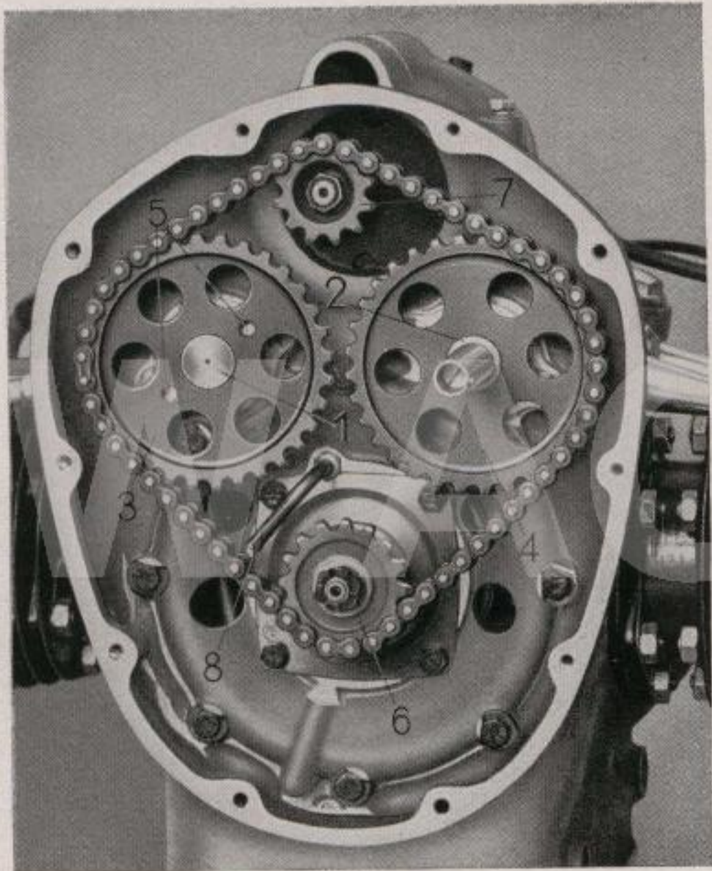
Bild 14. Stirnräderantrieb R 51
