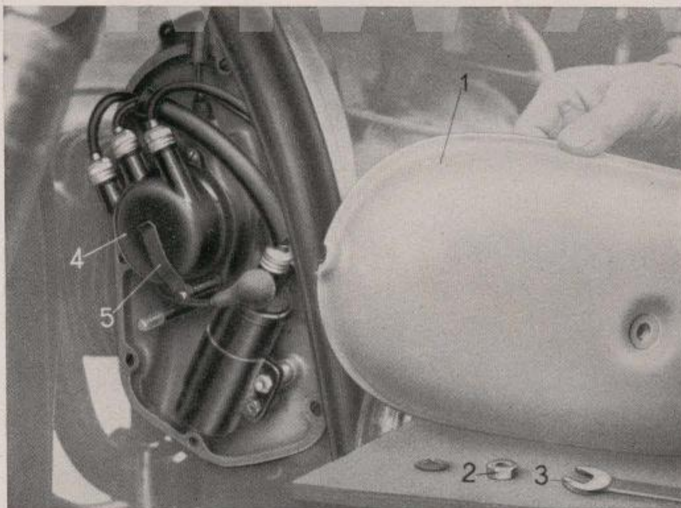
Bild 8. Zündanlage R 61 (R 66—71)
