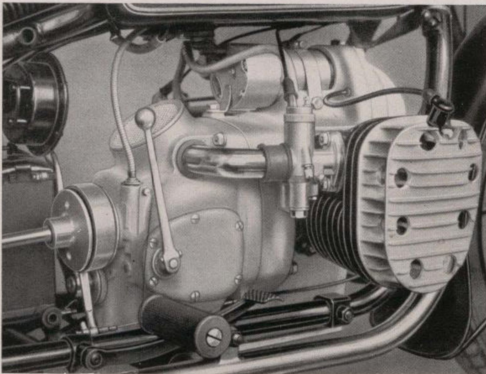
Bild 5. Motoranlage R 71
