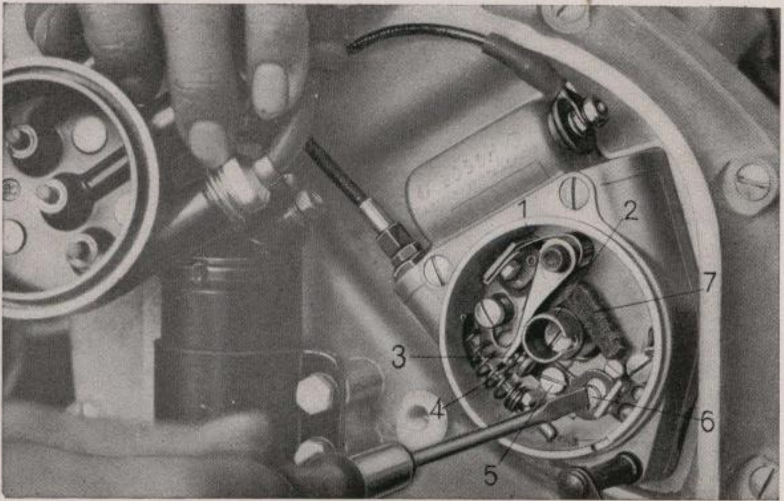
Bild 9. Unterbrecher
