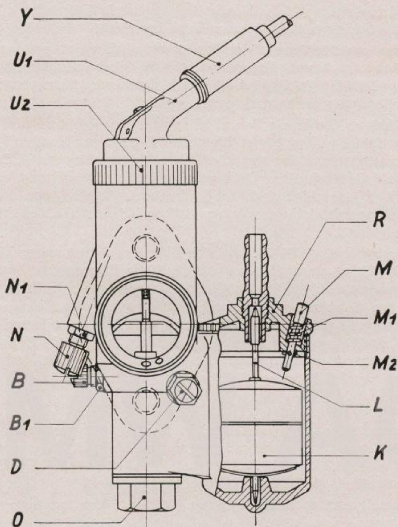
Bild 18. Vergaser R 71
