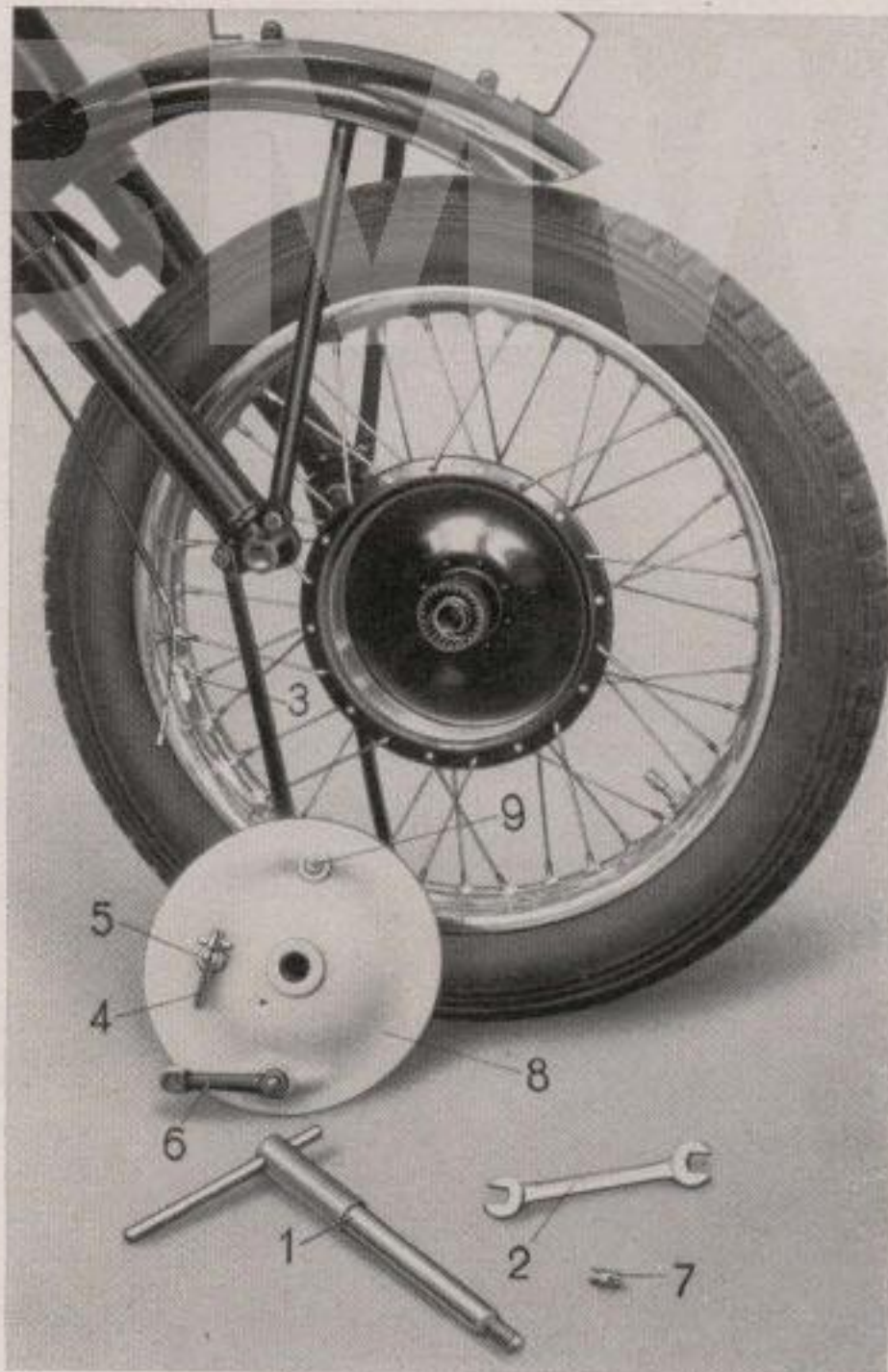
Bild 1. Ausbau des Vorderrades
