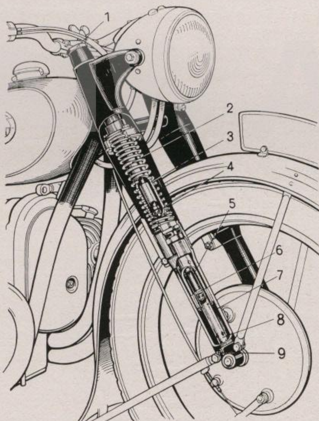
Bild 21. Vorderradgabel
