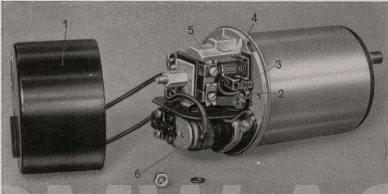
Bild 10. Lichtmaschine
