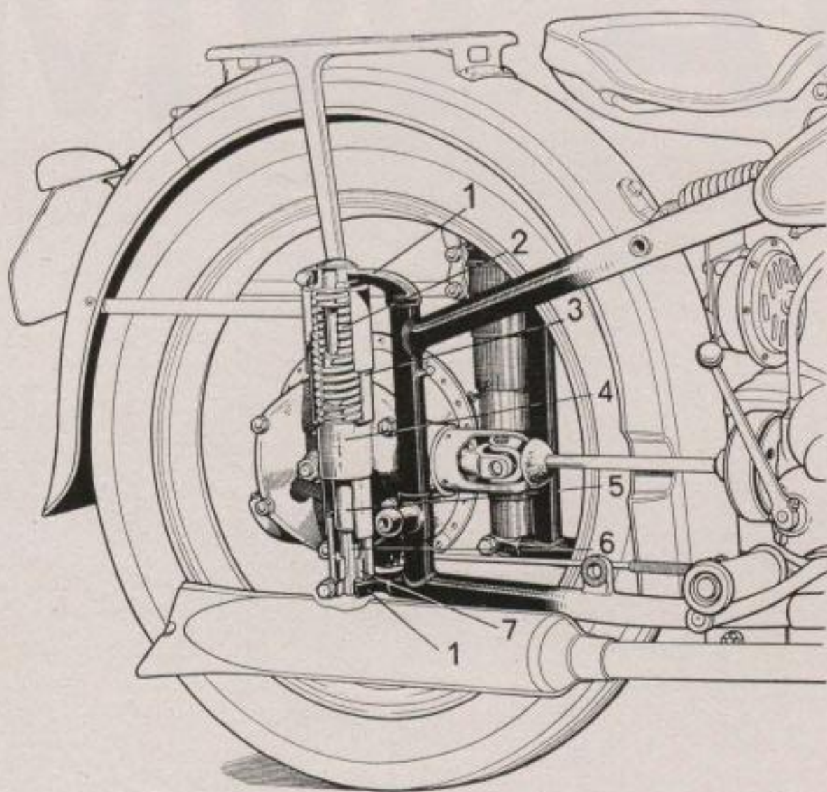
Bild 22. Hinterradfederung
