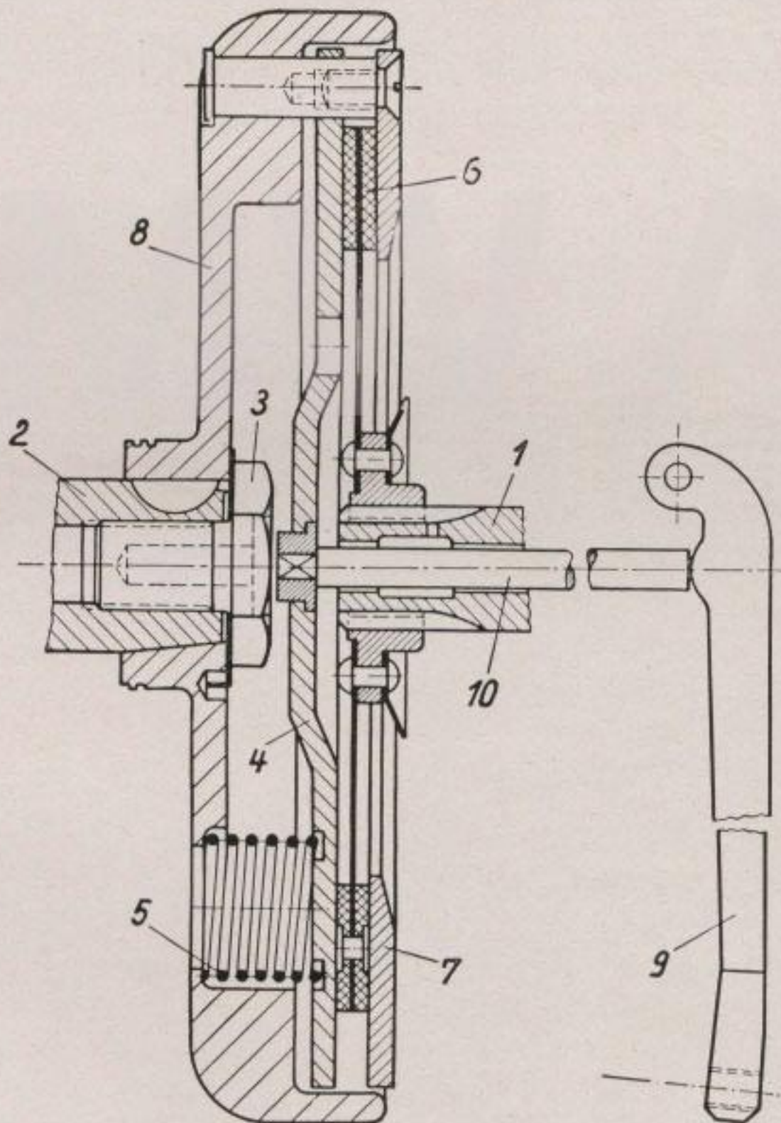
Bild 19. Kupplung
