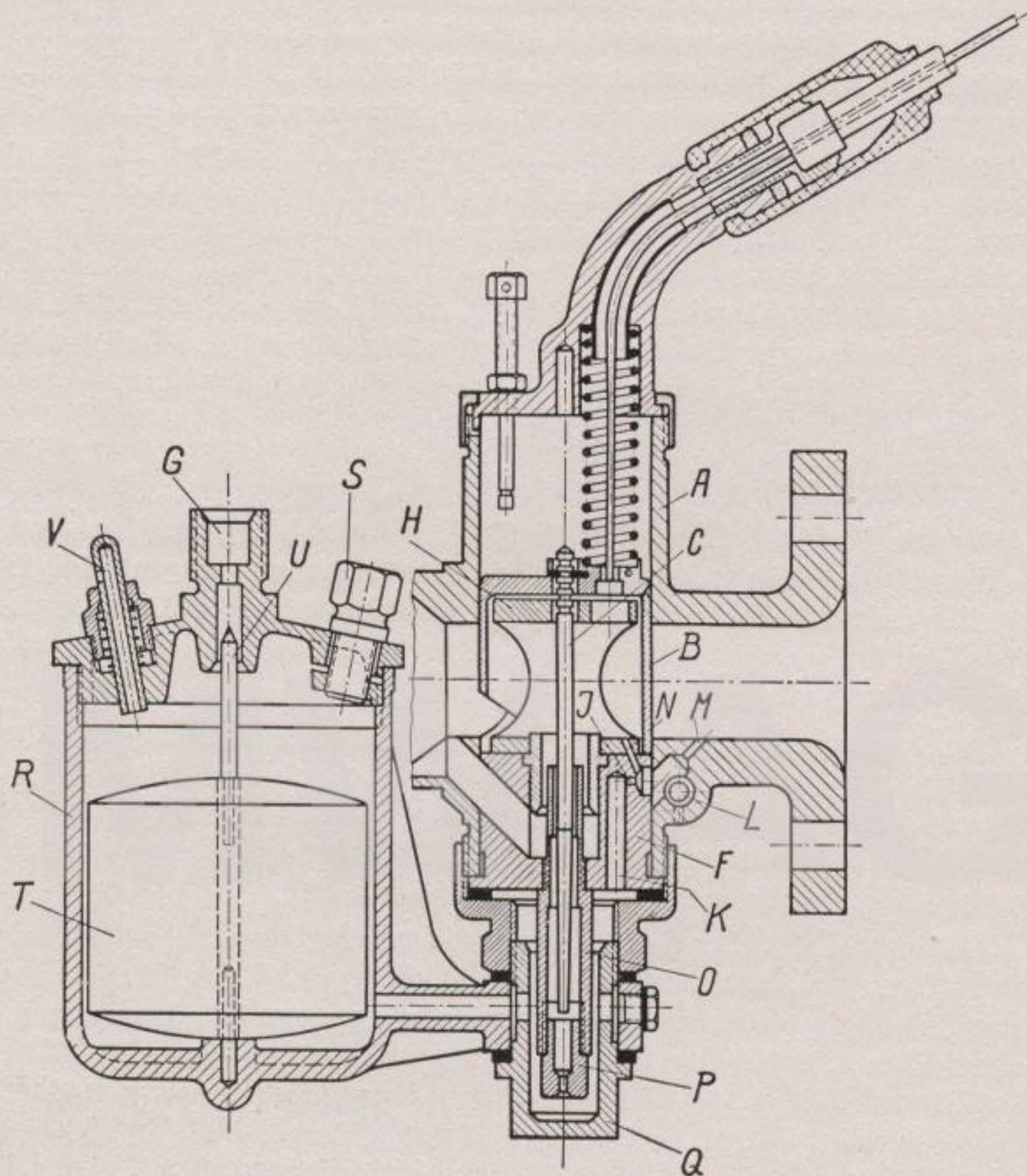
Bild 16. Vergaser R 51 (R 61 und 66)
