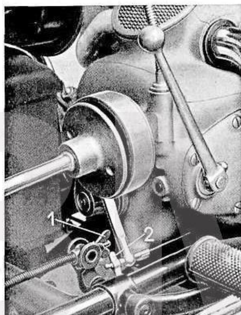
Bild 12. Brems- und Kupplungsnachstellung
