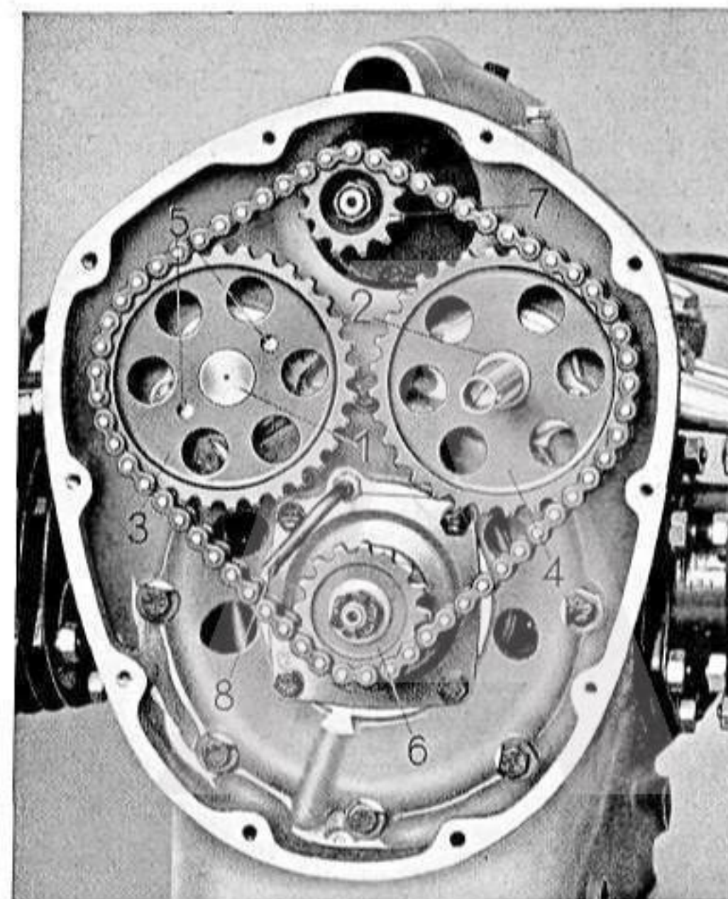
Bild 14. Stirnräderantrieb R 51
