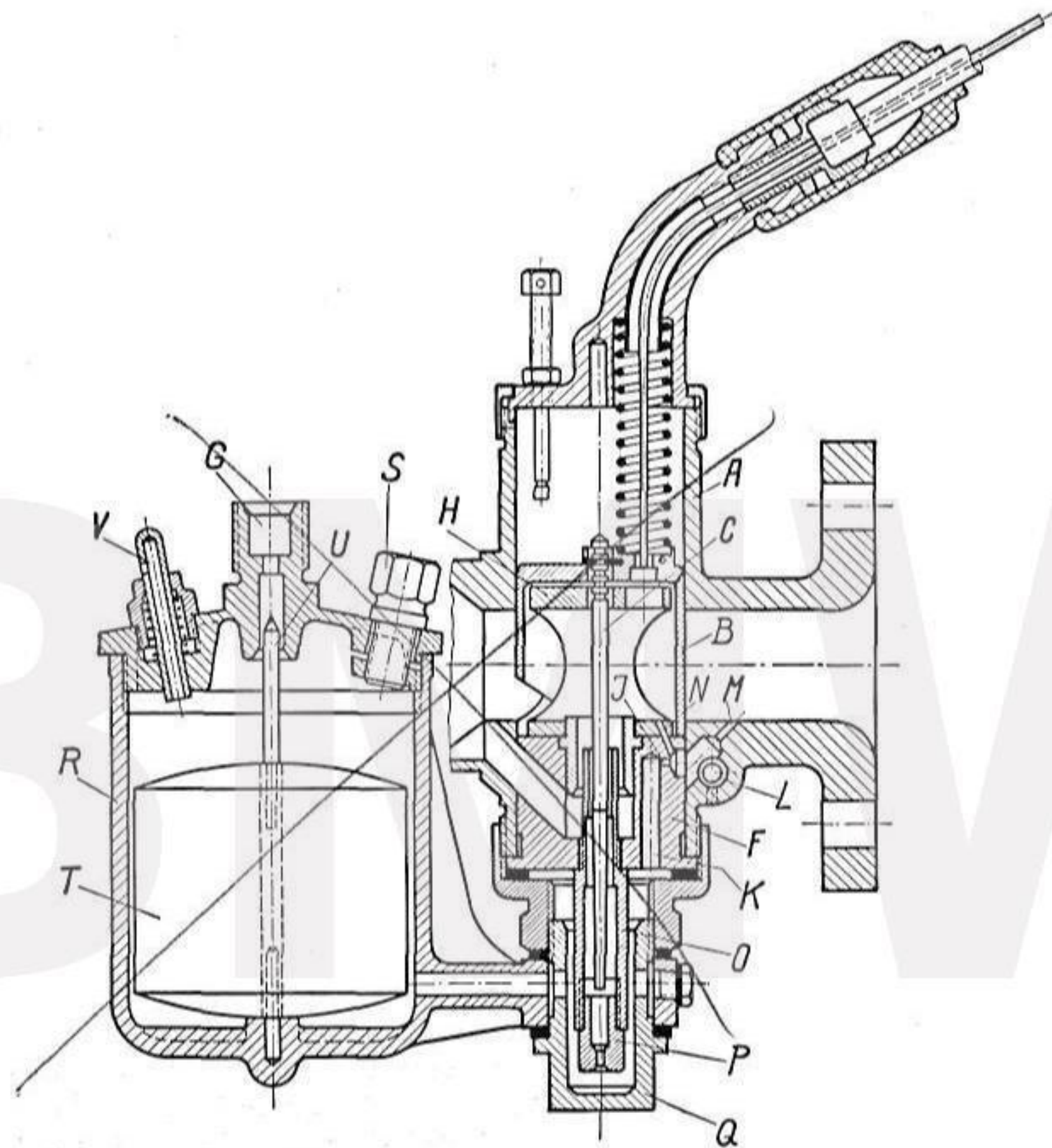
Bild 16. Vergaser R 51 (R 61 und 66)
