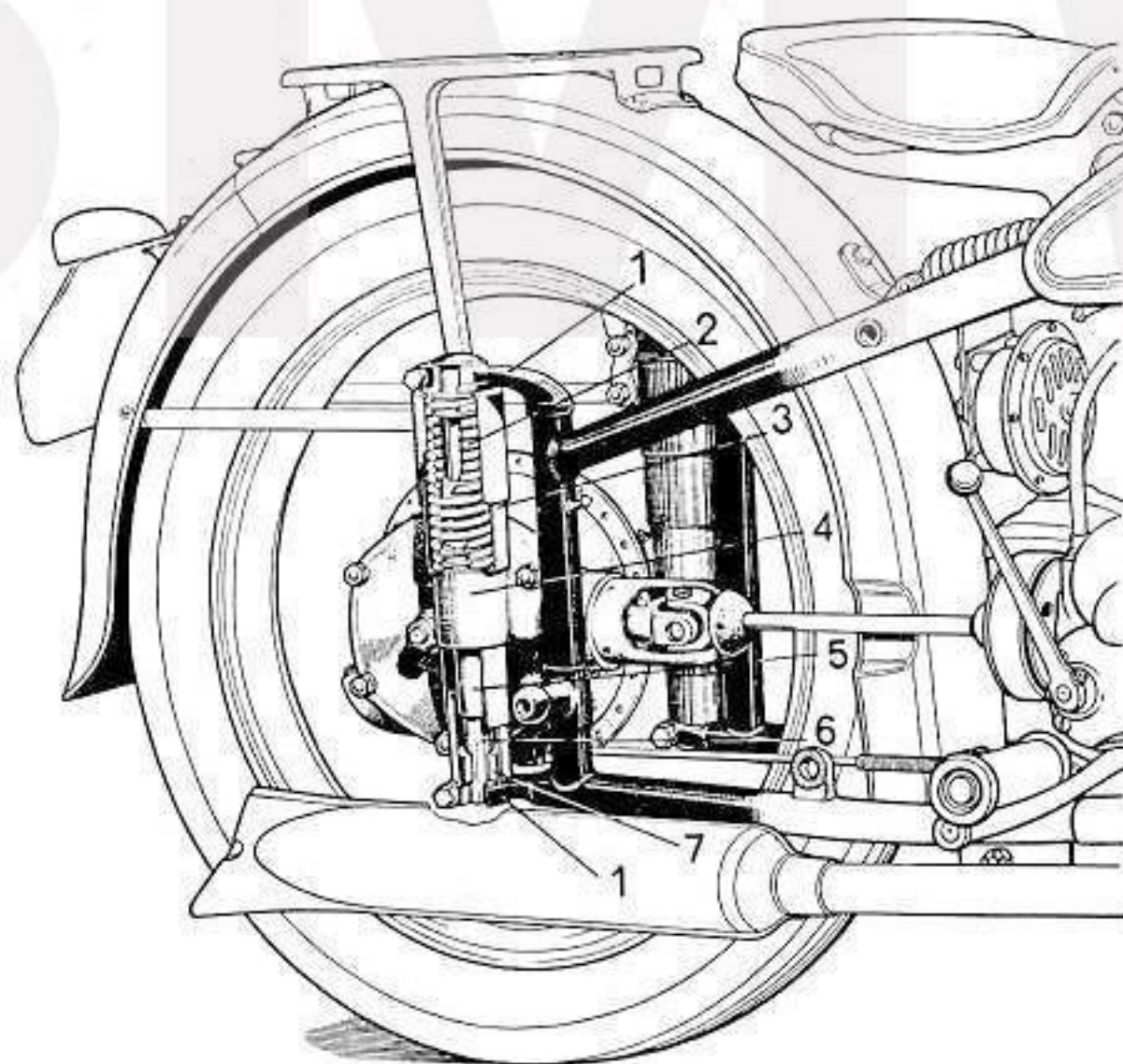
Bild 22. Hinterradfederung
