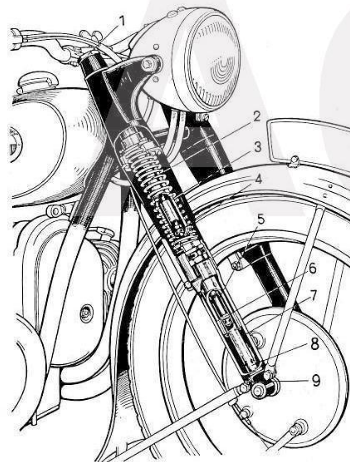
Bild 21. Vorderradgabel
