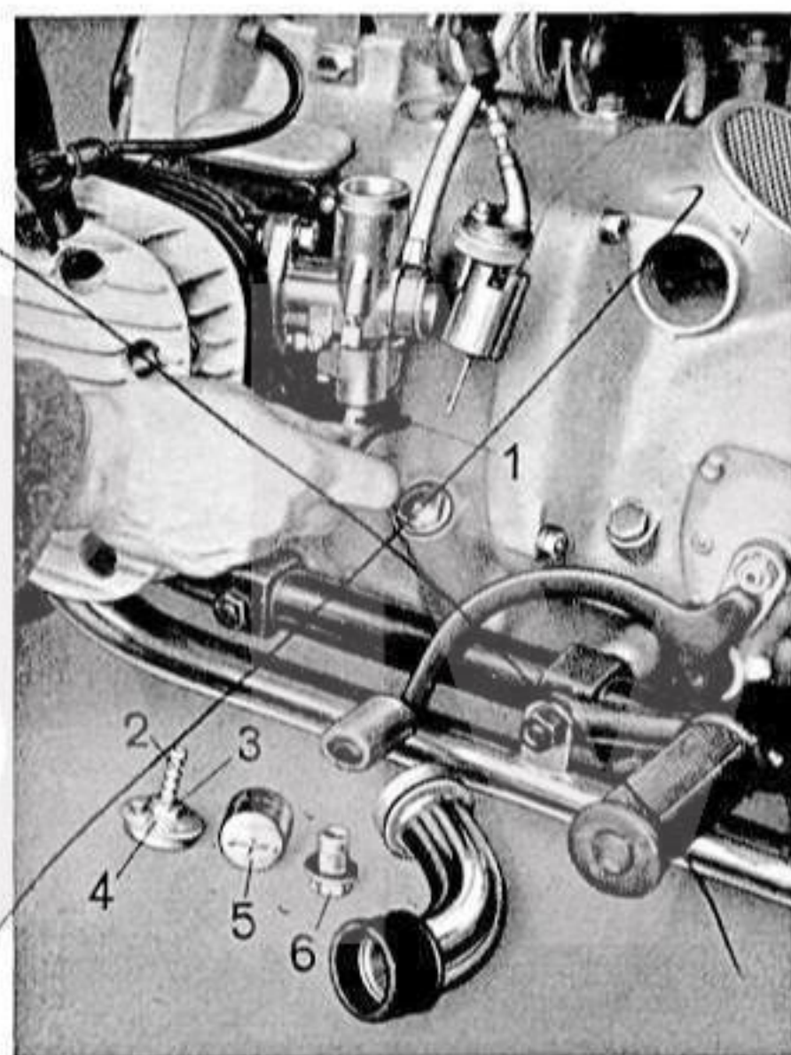
Bild 4. Vergaser R 71
