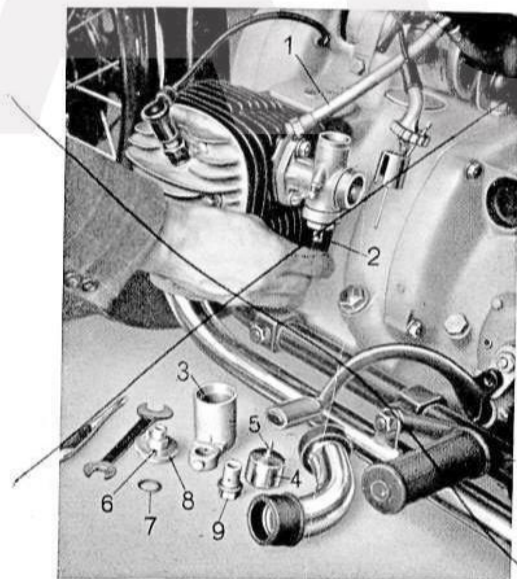
Bild 3. Vergaser R 51/61/66
