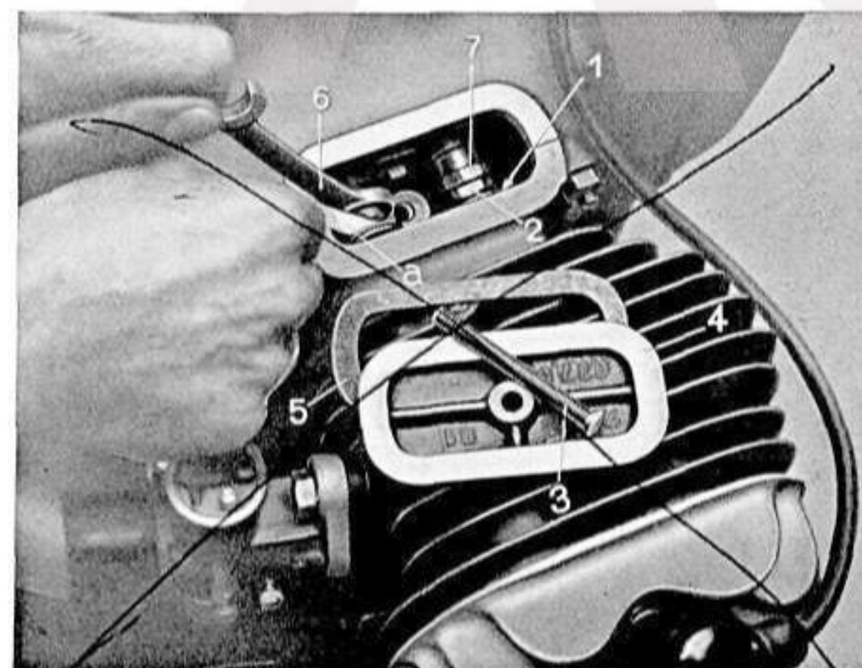
Bild 7. Ventilaachstellung R 61 (R 71)
