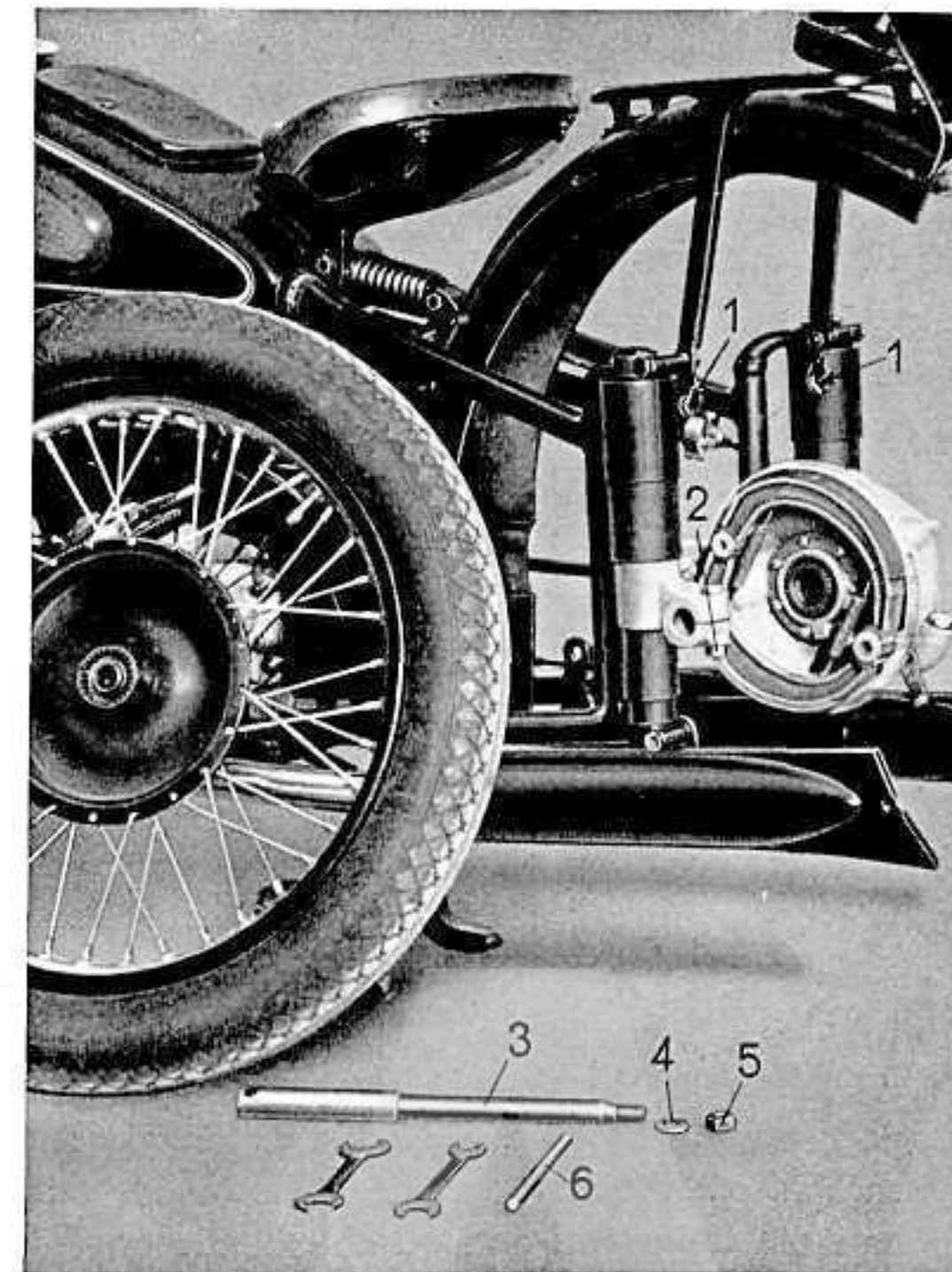
Bild 2. Ausbau des Hinterrades
