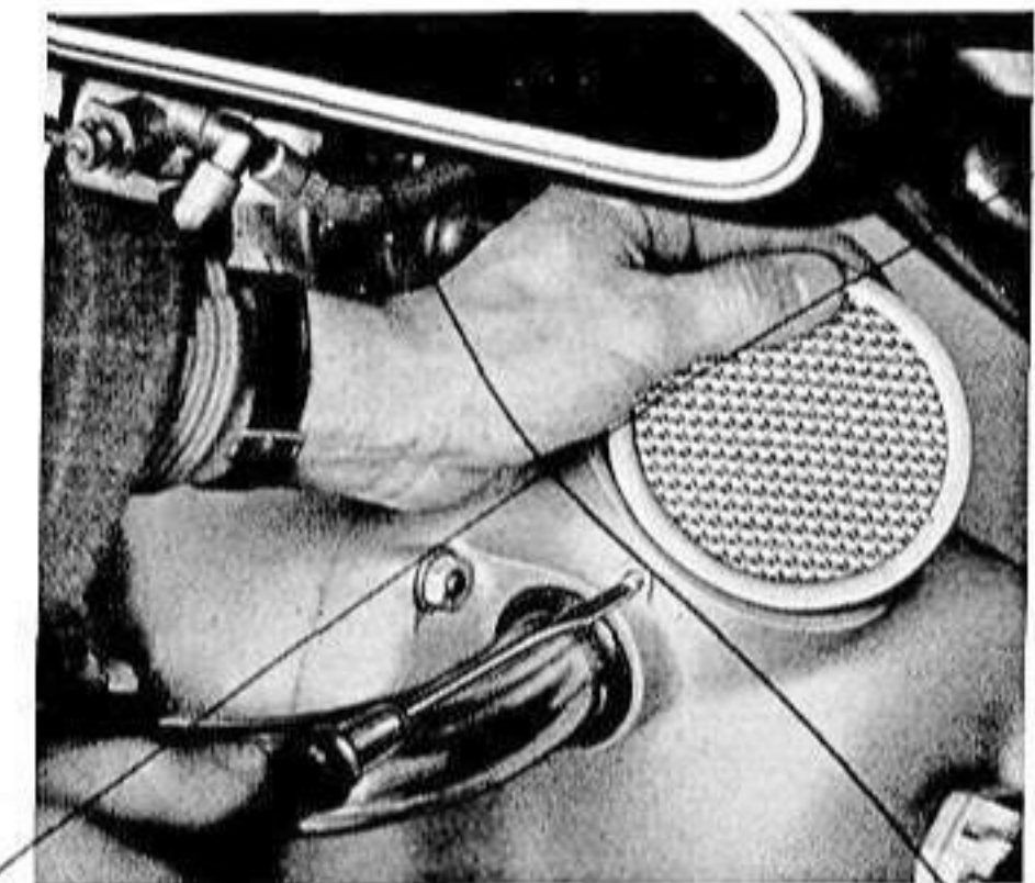
Bild 17. Luftfilter (R 51, 66, 61, 71)
