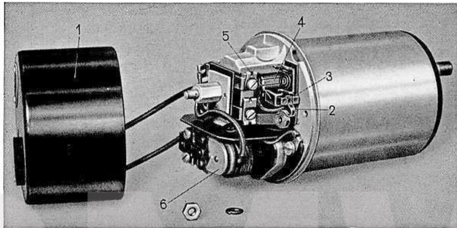
Bild 10. Lichtmaschine
