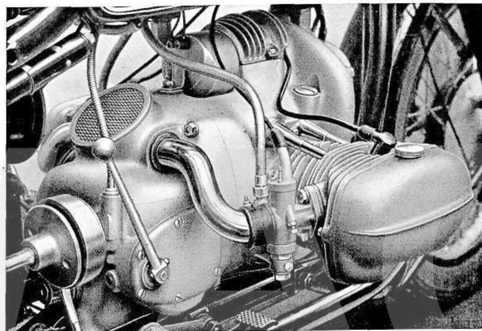
Bild 13. Motorblock R 51
