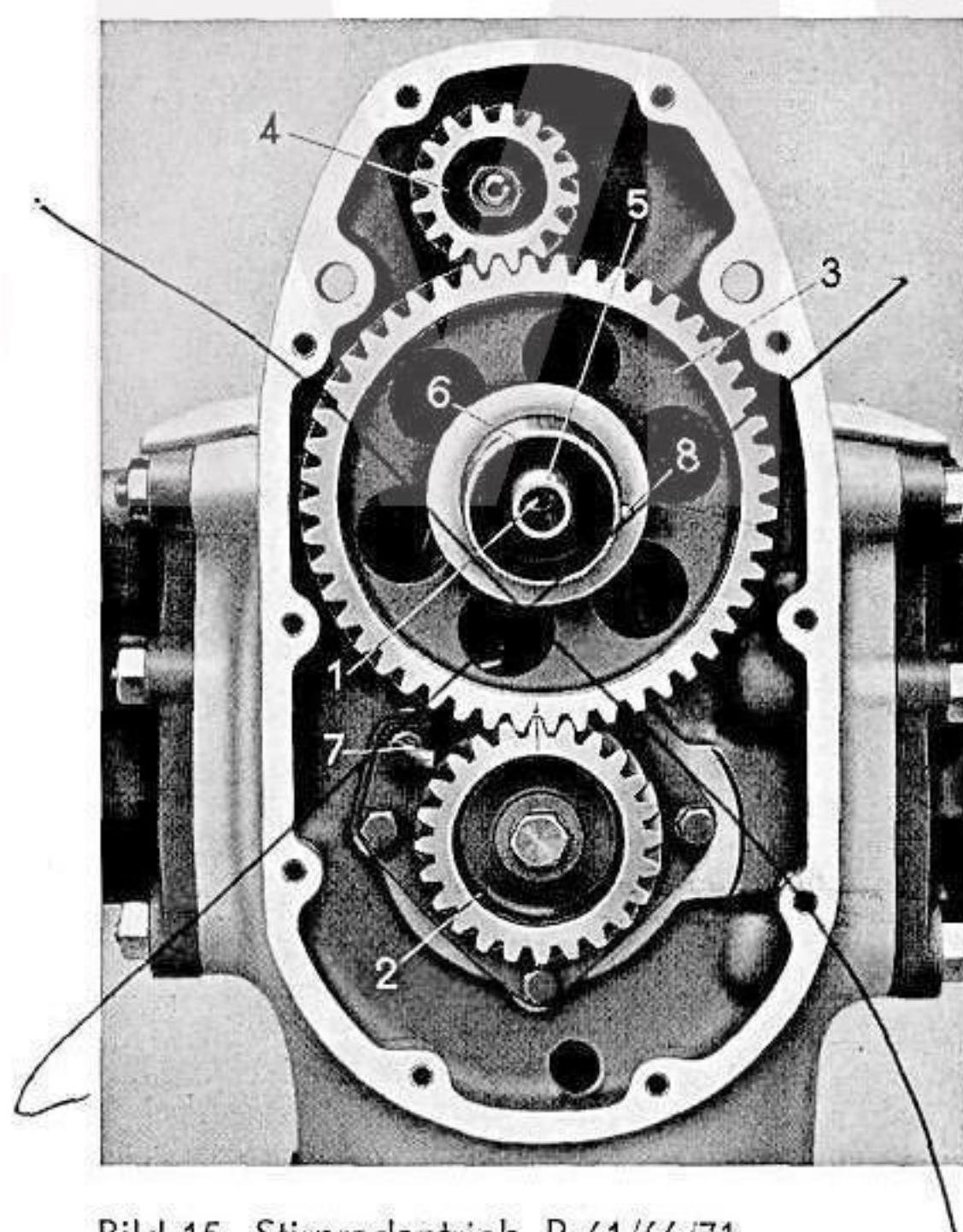
Bild 15. Stirnradantrieb R 61/66/71
