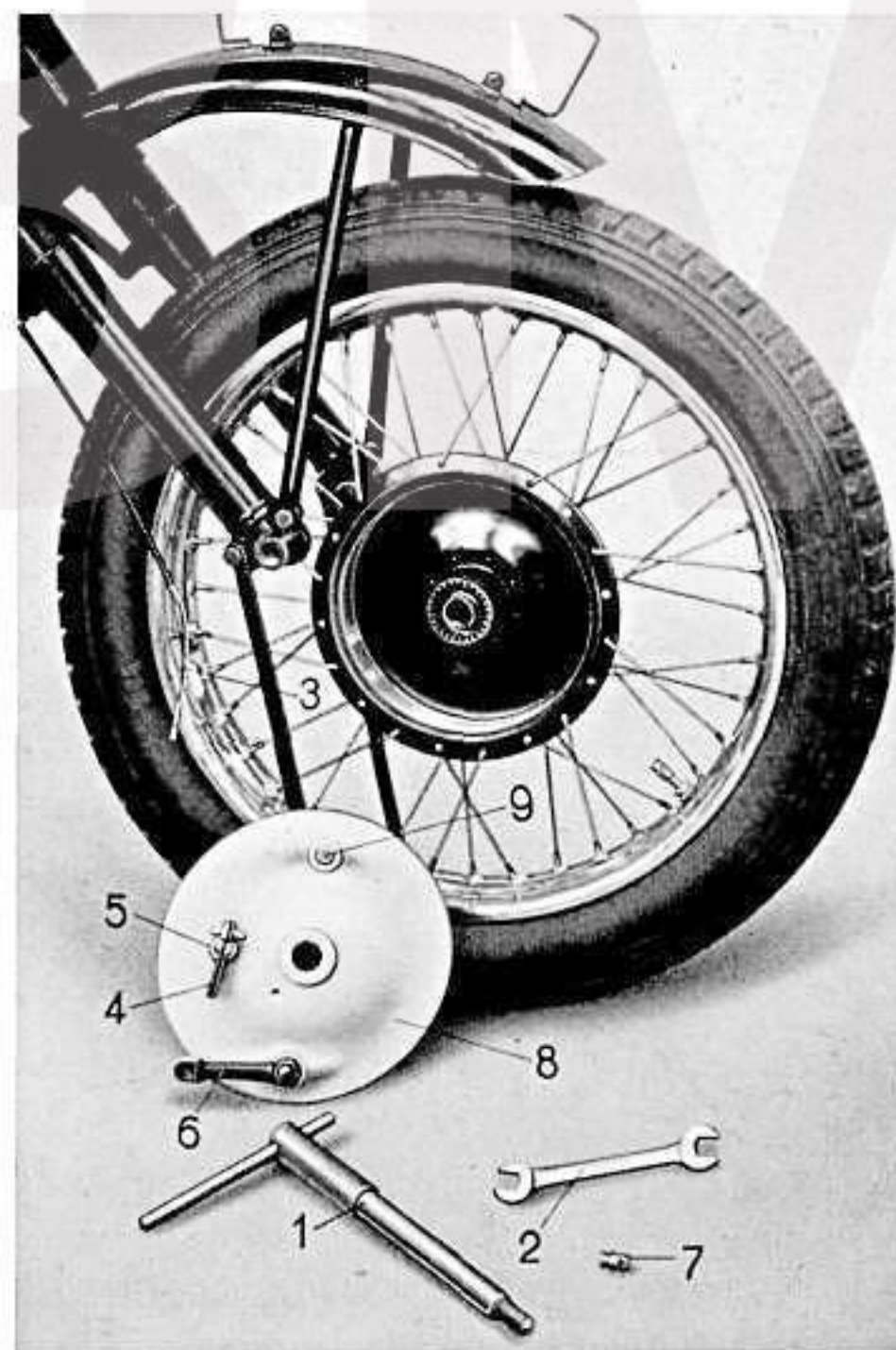
Bild 1. Ausbau des Vorderrades
