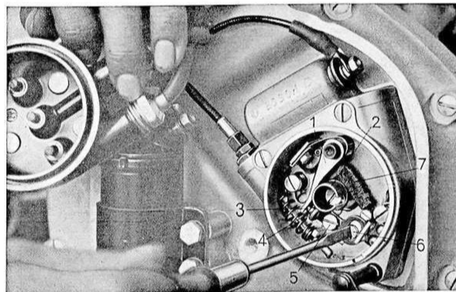
Bild 9. Unterbrecher
