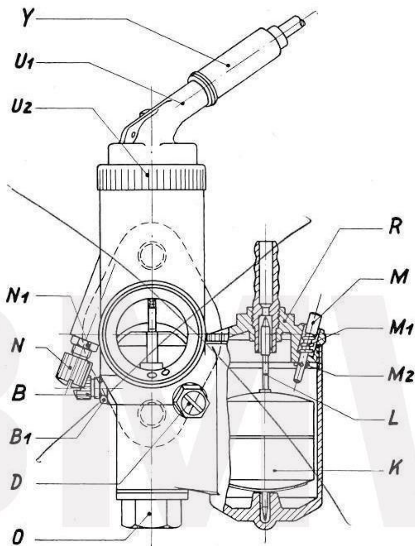
Bild 18. Vergaser R 71
