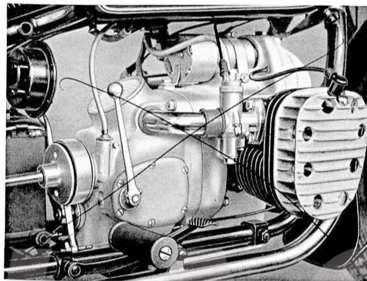
Bild 5. Motoranlage R 71
