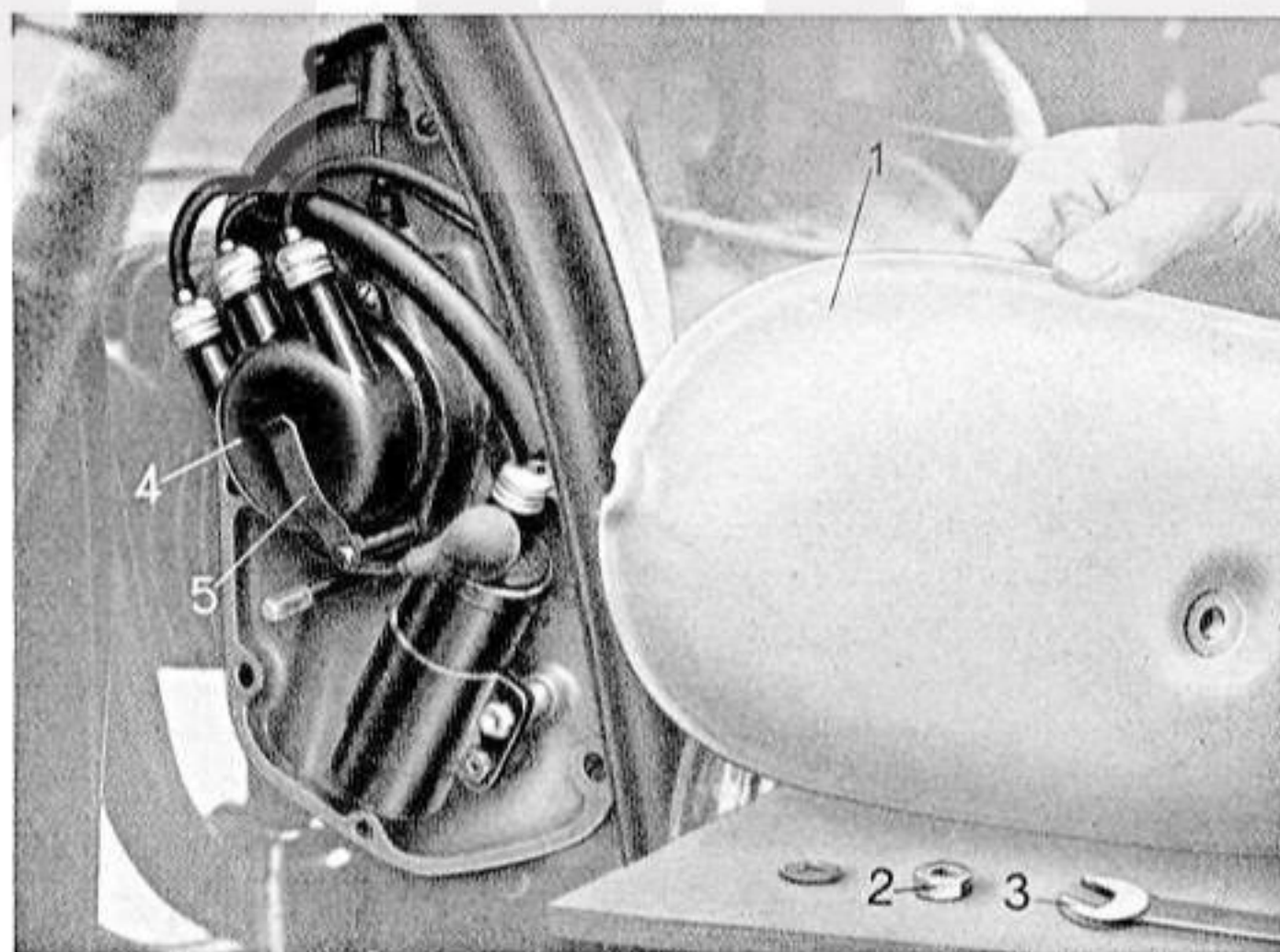
Bild 8. Zündanlage R 61 (R 66 - R 71)
