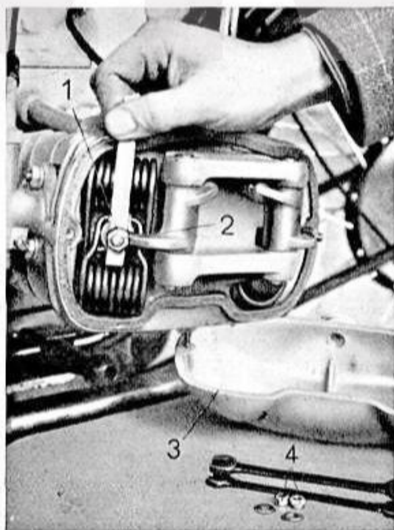
Bild 6. Zylinder-Kopf R 66 (R 55)
