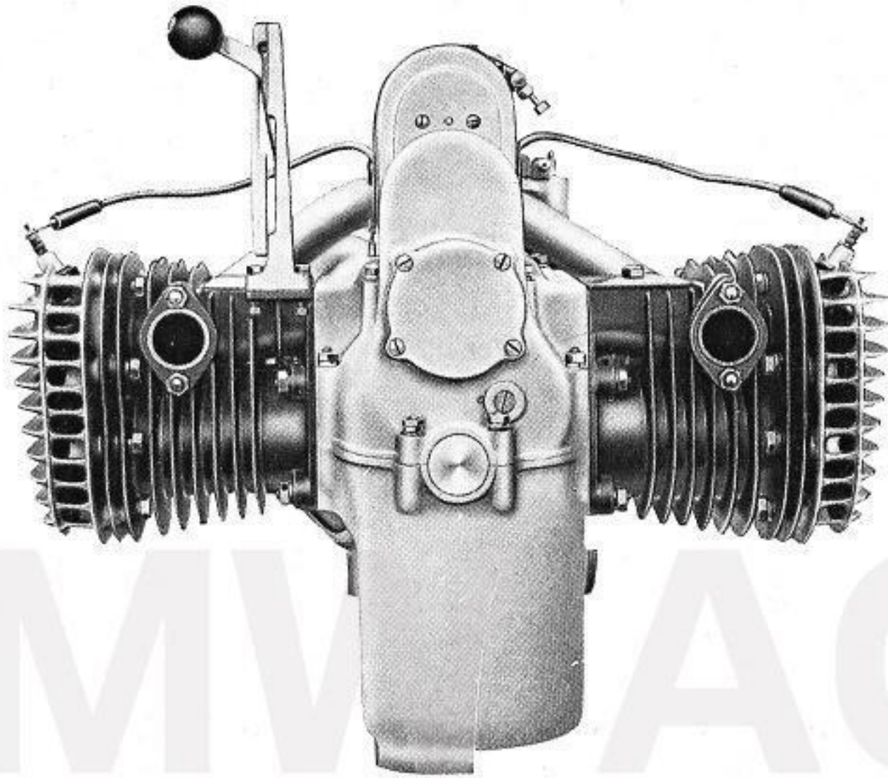
Abb. 8 Vorderansicht des Motors M 56 für Rad R 62
