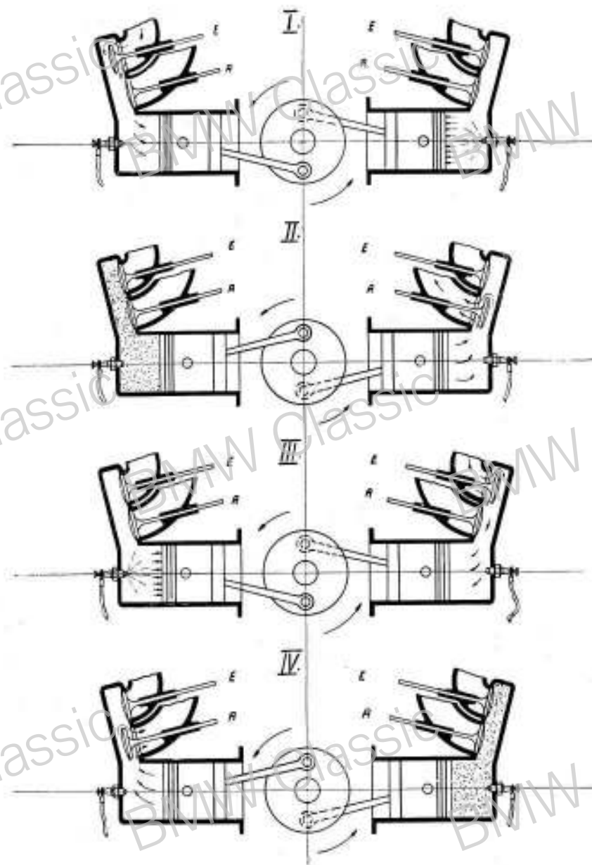
Abb. 5. Schematische Darstellung der Arbeitsweise des Motors.
