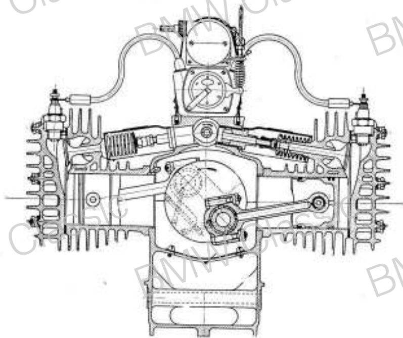
Abb. 15 Schnitt durch den Motor.
