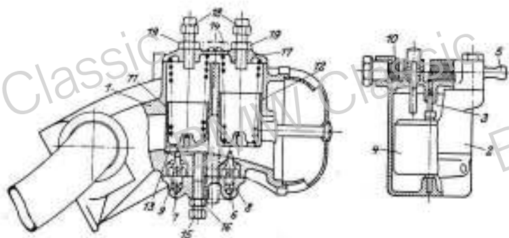
Abb. 7. Schnitt durch den B.M.W.-Vergaser.
