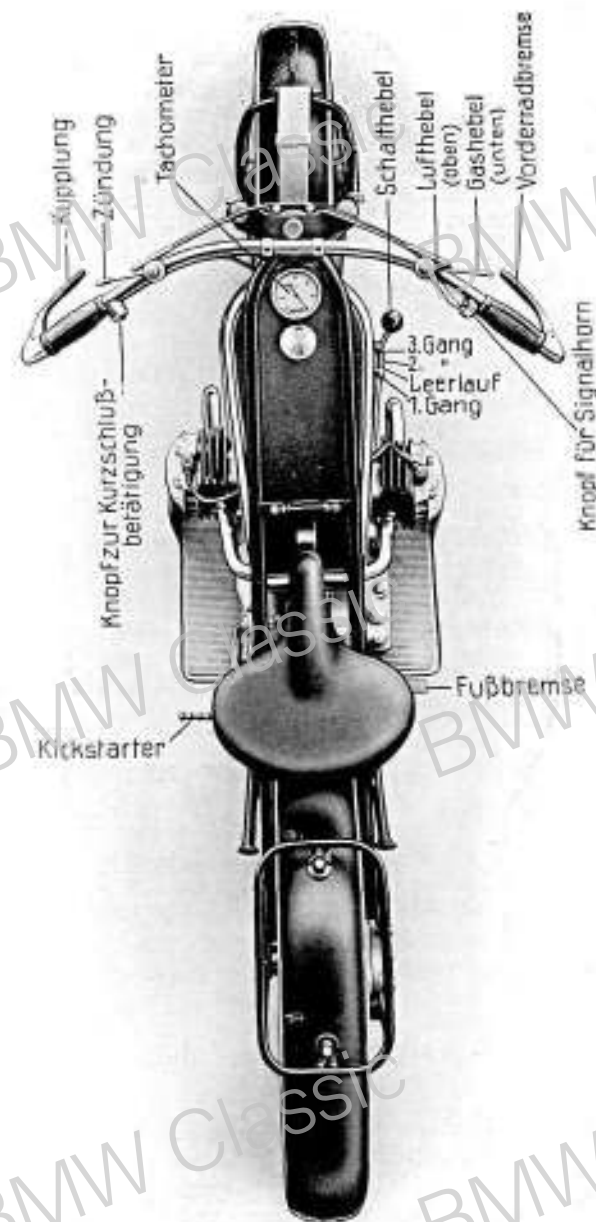
Abb. 27. Die Bedienungshebel am B.M.W.-Rade.
