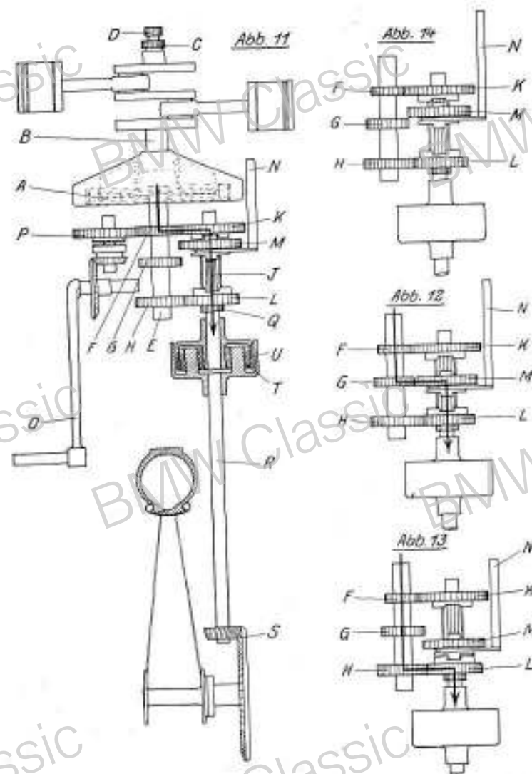
Abb. 11, 12, 13 und 14. Schematische Darstellung des Antriebes.
