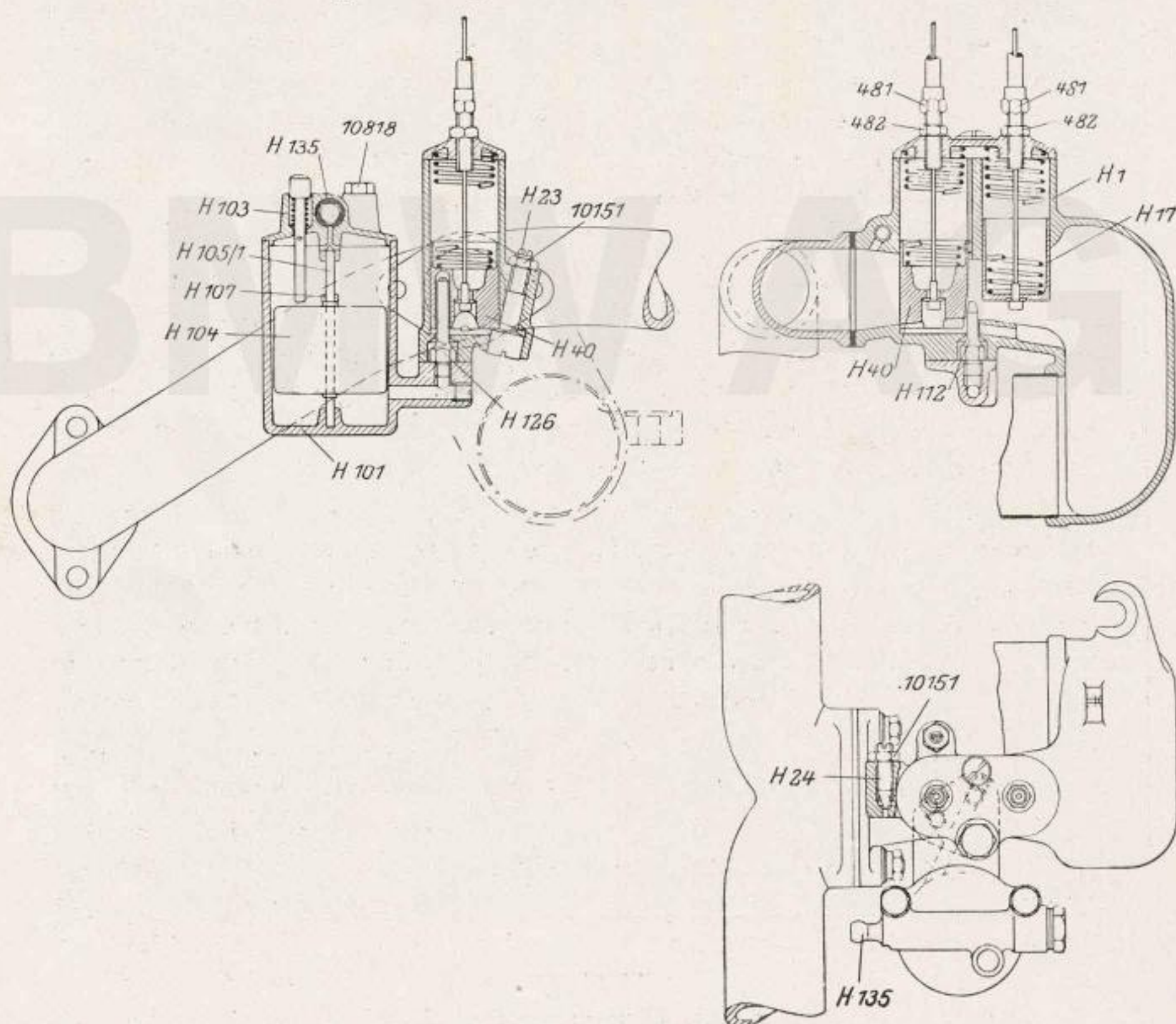
Abb. 7. BMW-Vergaser mit Schwimmergehäuse.
