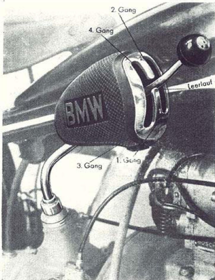
Abb. 8 Getriebebeschaltethebel
