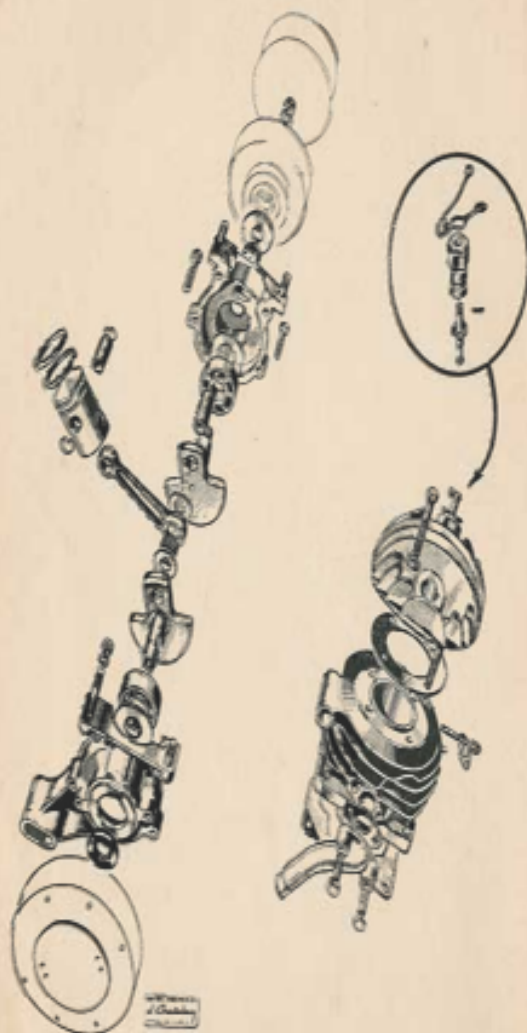
Vue éclatée du Moteur
