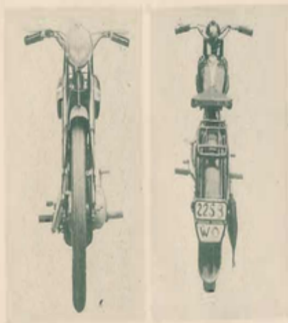
QUELQUES ASPECTS DE LA 125 TERROT
