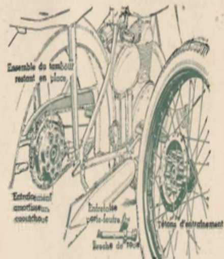
VUE DU MOYEU ARRIERE
