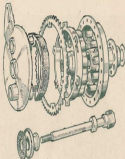
VUE DU MOYEU ARRIERE
