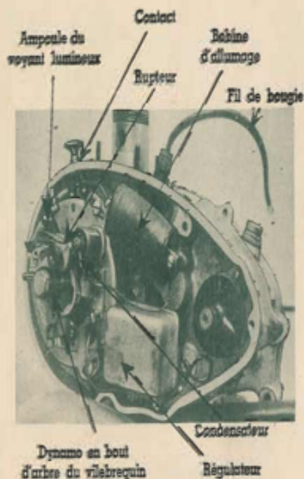
VUE DE L'EQUIPEMENT ELECTRIQUE DE LA 125 TERROT
