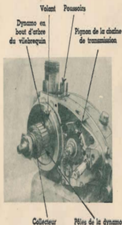
Volant et induit de la dynamo
