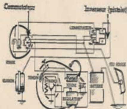
Schémas d'équipement électrique au 125 Terrot.
