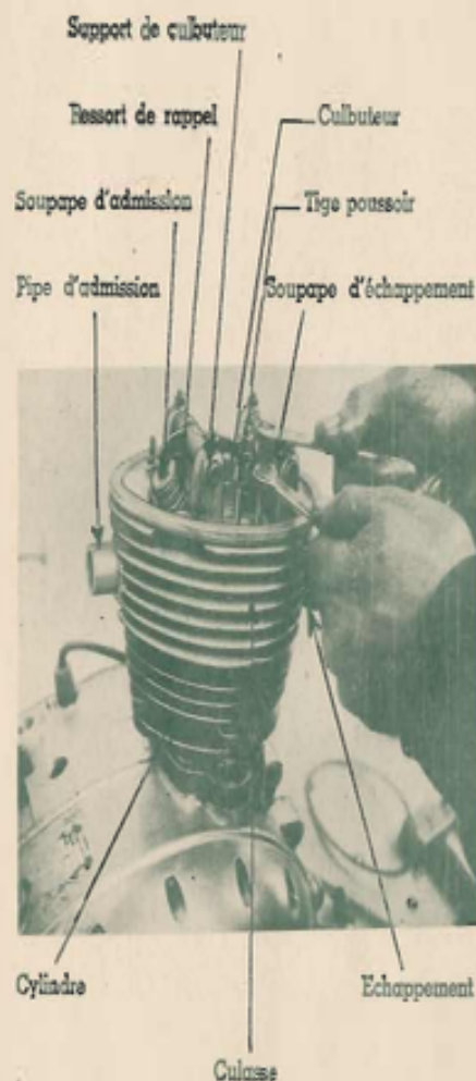
REGLAGE DU JEU AUX CULBUTEURS
