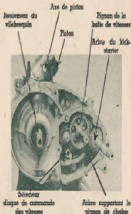
LE MOTEUR EN COURS DE DEMONTAGE (côté gauche)
