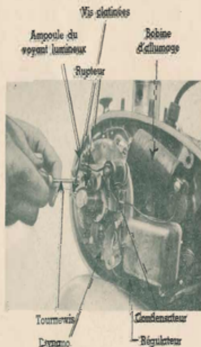
REGLAGE DE L'EQUIPEMENT DES VIS PLATINEES
