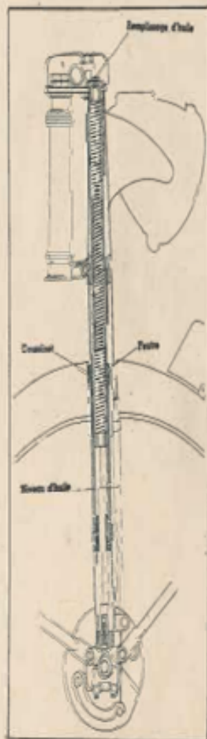
COUPE DE LA FOURCHE TELESCOPIQUE DE LA MOYNETTE 125 cmc. TERROT TYPE E.T.D.
