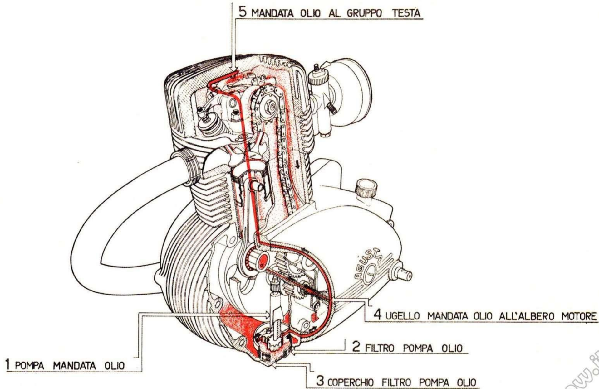
Fig. 3 - Schema circolazione olio.
