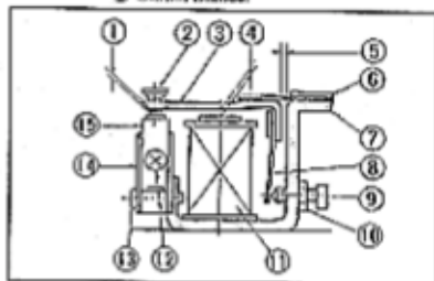
Fig. 5-52 ① Apertura puntine. ② Controalzo. ③ Contatto superiore. ④ Avvolgimento. ⑤ Armatura. ⑥ Vite registrazione apertura puntine. ⑦ Apertura del nucleo. ⑧ Vite registrazione apertura nucleo. ⑨ Apertura della interlasciatura. ⑩ Gruppo di contatto. ⑪ Molla. ⑫ Contatto inferiore. ⑬ Inclinatura. ⑭ Molla di registro. ⑮ Vite regolazione voltaggio.
