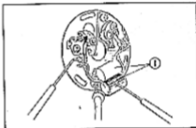
Fig. 5-73 ① Condensatore.
