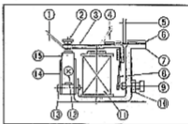
Fig. 5-61 ① Apertura puntino. ② Contatto inferiore. ③ Armatura. ④ Apertura del nucleo. ⑤ Molla. ⑥ Intalsatura. ⑦ Molla di registrazione. ⑧ Vite regolazione voltaggio. ⑨ Controdado. ⑩ Avvolgimento. ⑪ Vite regolazione apertura puntino. ⑫ Vite regolazione apertura nucleo. ⑬ Gruppo di contatto. ⑭ Contatto superiore.
