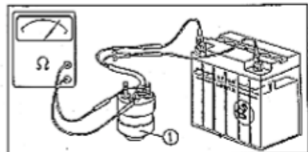
Fig. 5-22 ① Interruttore magnetico di avviamento.
