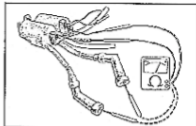
Fig. 5-58 Prova della continuità della bobina.
