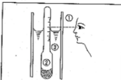
Fig. 5-63 ① Livello dell'occhio. ② Densimetro. ③ Elettrolito.
