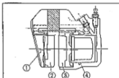
Fig. 4-22 ① Pinza H. ② Pastiglia A. ③ Pastiglia B. ④ Pinza A.
