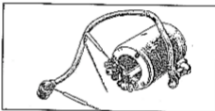
Fig. 5-26 Controllo della continuità dell'avvolgimento di campo.
