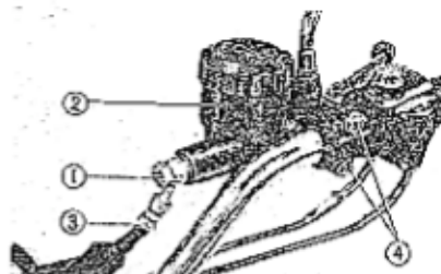
Fig. 4-17 ① Bullone di attacco. ② Complesso del cilindro principale. ③ Cassetto del liquido del freno. ④ Attacco al manubrio.
