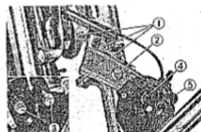
Fig. 4-15 ① Bulloni di montaggio della pinza. ② Bullone di registro. ③ Pinza B. ④ Bulloni di unione della pinza. ⑤ Pinza A.
