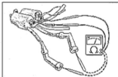
Fig. 5-27 Controllo della continuità della bobina di accensione.
