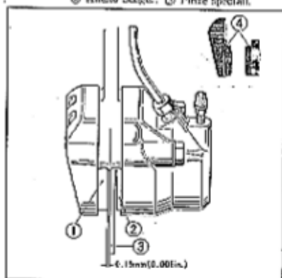
Fig. 4-19 ① Pastiglia B. ② Disco. ③ Pastiglia A. ④ Indicatore del limite di usura.
