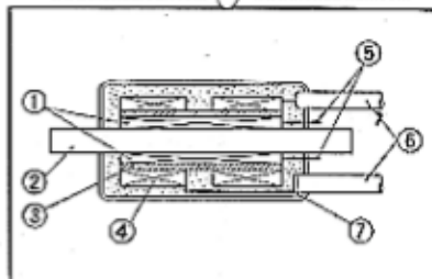
Fig. 5-26 ① Avvolgimento primario. ② Nucleo di ferro. ③ Roccetto. ④ Avvolgimento secondario. ⑤ Terminali primario. ⑥ Cavetti ad alta tensione. ⑦ Terminali del secondario.
