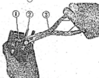
Fig. 4-29 ① Corpo del cilindro principale. ② Anello Seeger. ③ Pinze speciali.
