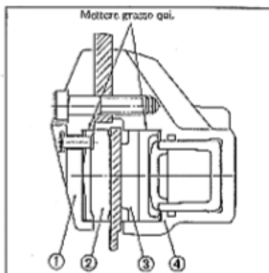
Fig. 4-33 ① Pinza B. ③ Pastiglia A. ② Pastiglia B. ④ Pinza A.
