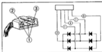
Fig. 5-17 ① Cavetti gialli. ② Cavetto rosso/bianco. ③ Cavetto verde.
