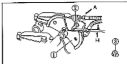
Fig. 2-15 ① Leva del gas. ② Contro dado. ③ Pernetto del fermo.
