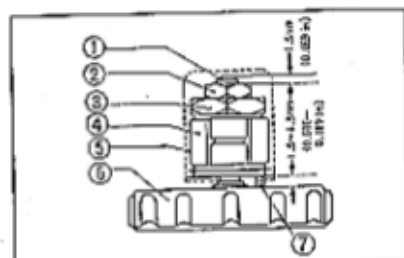
Fig. 2-29 ① Aletta filettata. ② Controdado. ③ Dado di regolazione. ④ Braccetto di comando. ⑤ Cassina di getto. ⑥ Parte superiore del carburatore. ⑦ Svucometro.
