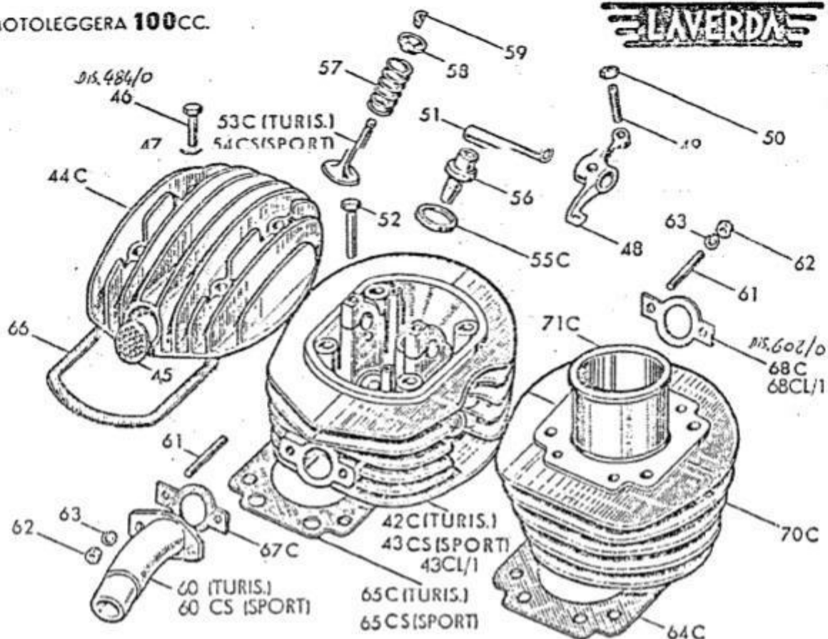
2 - TESTA - CILINDRO
