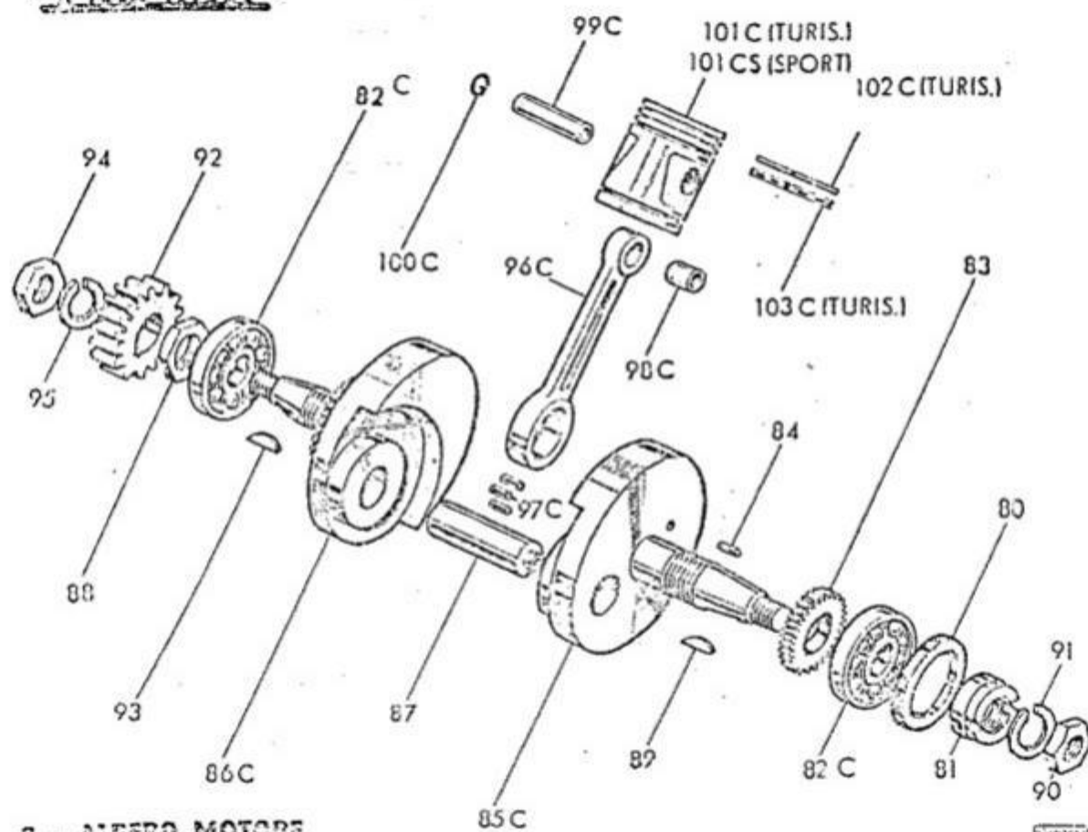
3 - ALBERO MOTORE
