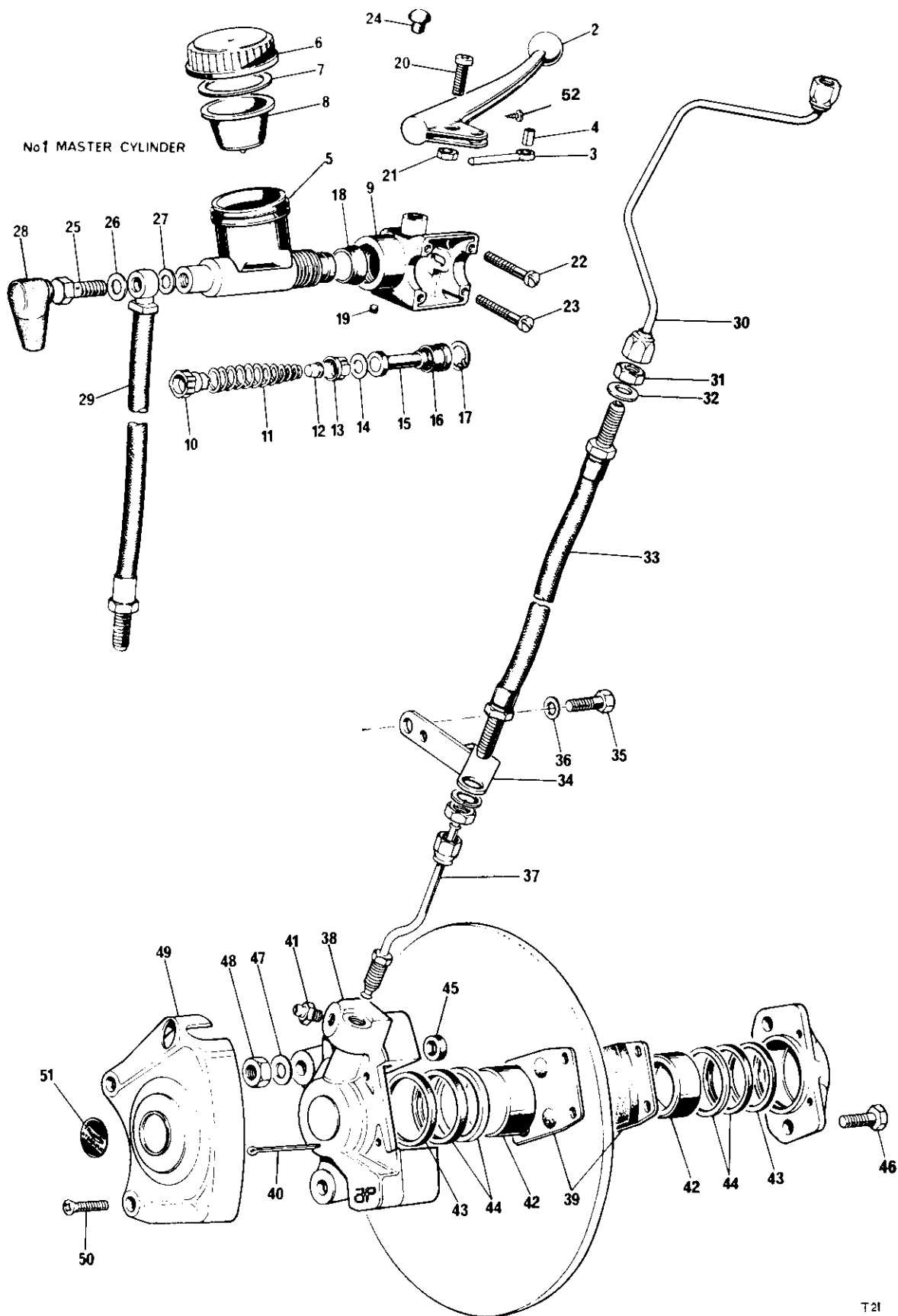
Fig. 21. FRONT BRAKE
