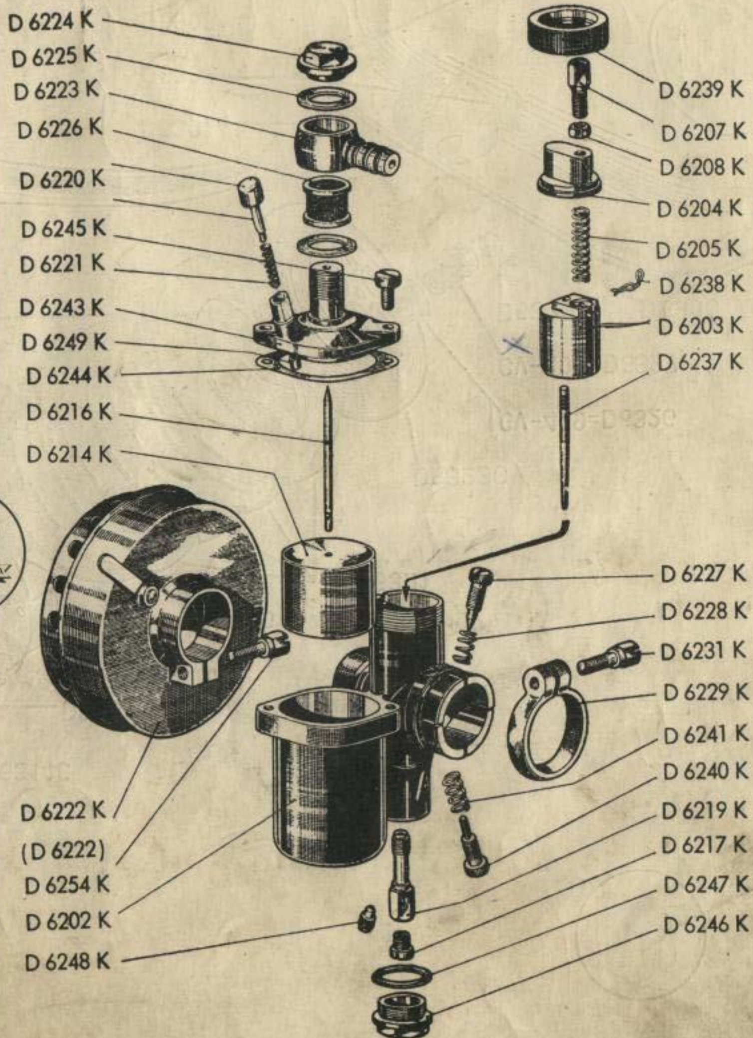
CARBURADOR IRZ - Tipo 18 - AE
