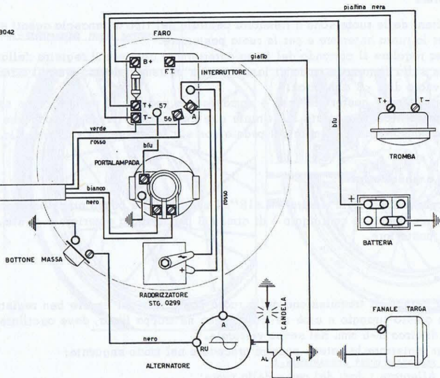
Fig. 5 - Schema impianto elettrico 125 T.R.L.
