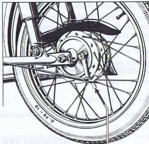
B - REGISTRAZIONE FRENO POSTERIORE
